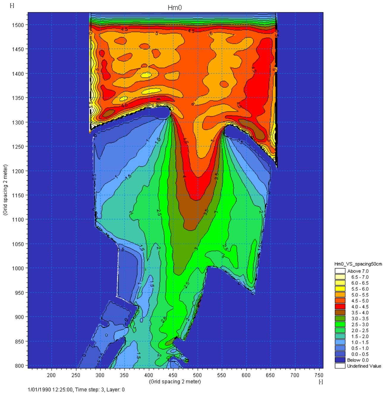
Figuur 2 - Contourplot significante golfhoogte H_{m0,GI} na 100-jarige storm met kortkruinige golven uit richting NW
