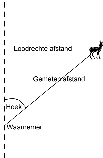
Figuur 3 Berekeningsmethode voor het berekenen van de loodrechte afstand tussen het waargenomen ree en het waarnemingstraject (in het geval het dier zich niet loodrecht t.o.v. de waarnemer en het traject bevindt).
