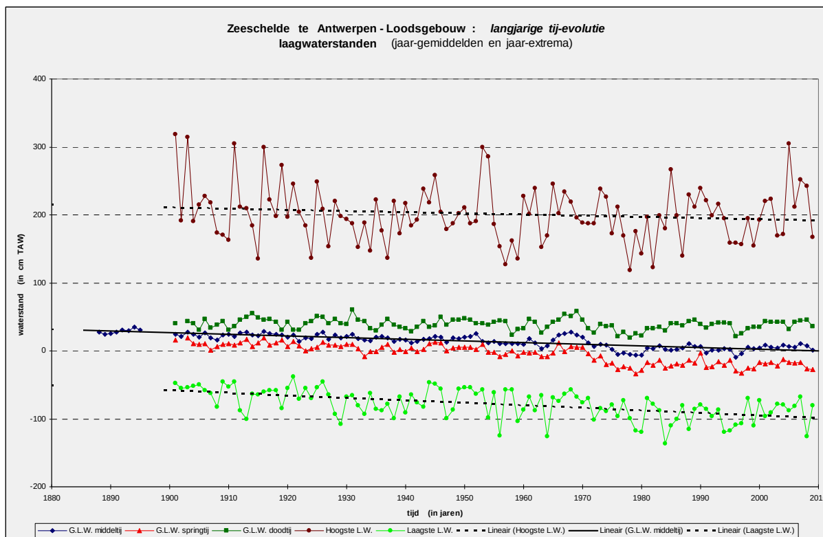
Figuur 29 - Zeeschelde te Antwerpen-Loodsgebouw: evolutie sinds 1885 (resp. 1900) van jaargemiddeld laagwater middeltij, springtij en doortij, aangevuld met de jaarlijks hoogste en de jaarlijks laagste laagwaterstanden
