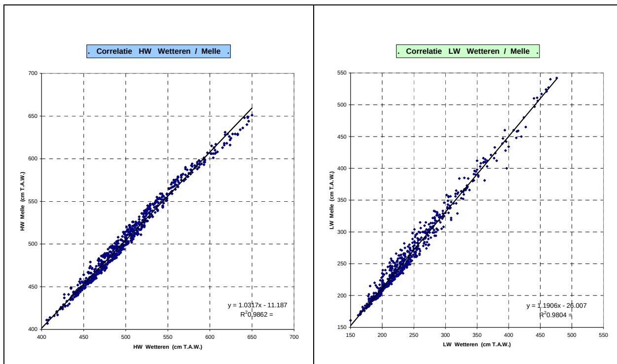
Figuur 7 - correlaties van hoogwater (links) en laagwater (rechts) over een kalenderjaar tussen de geburige meetposten Wettersen en Melle
