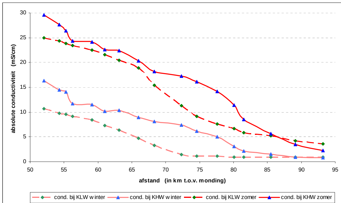
Figuur 85 - Westerschelde en Zeescheldebekken tussen Bath en Rupelmonde : langsvaart bij kentering laag- en hoogwater op typische winter- en zomer-omstandigheden 2009 - verloop van de conductiviteit
