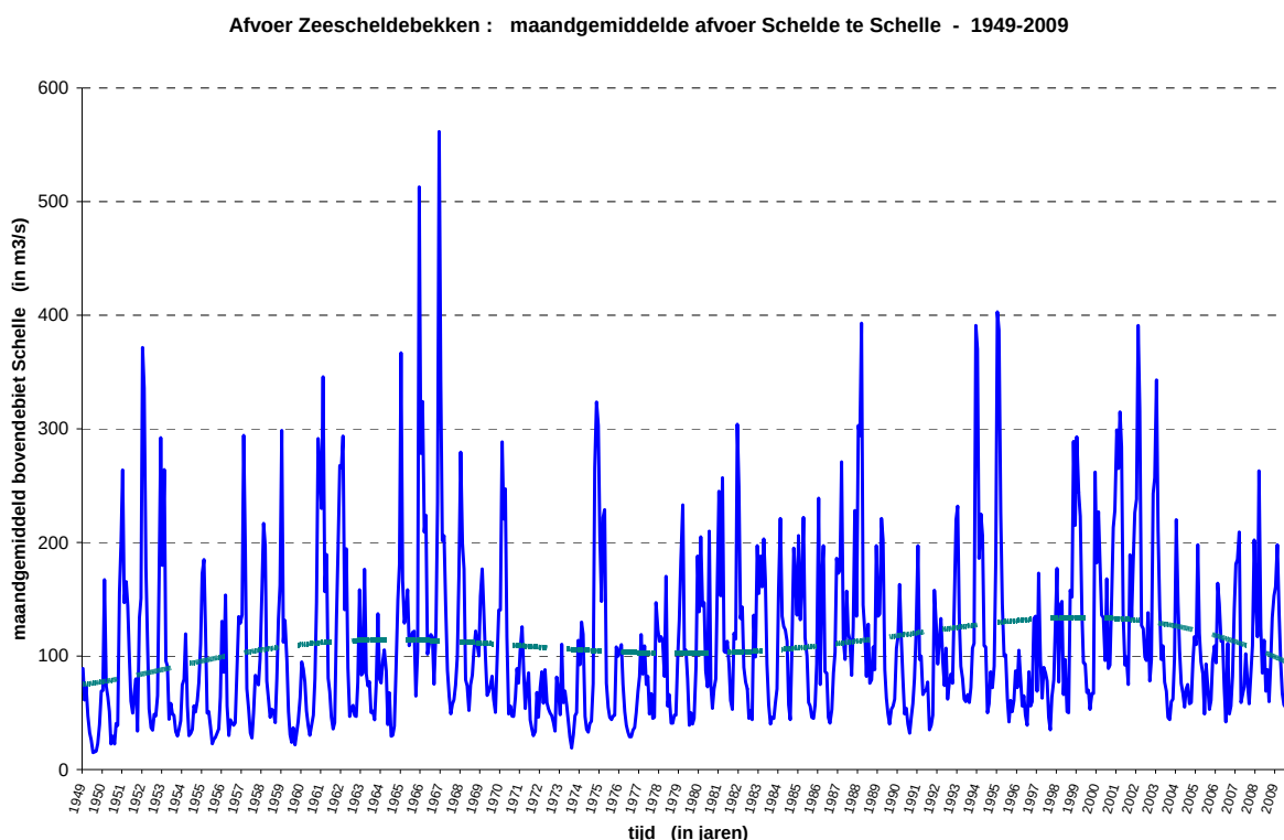
Figuur 48 - Zeescheldebekken: afvoer "Schelde te Schelle" over de periode 1949 à 2009 op basis van maandgemiddelde waarden
