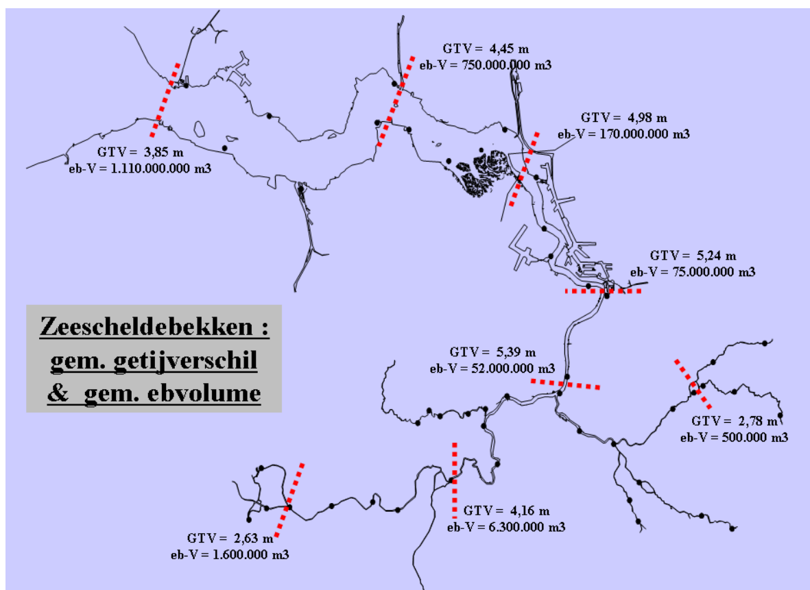
Figuur 5 - Zeescheldebekken: algemeen liggingplan met aanduiding van gemiddelde tijverschillen (GTV) (in m) en gemiddelde eb-volumes (in m³) op enkele kenmerkende locaties
