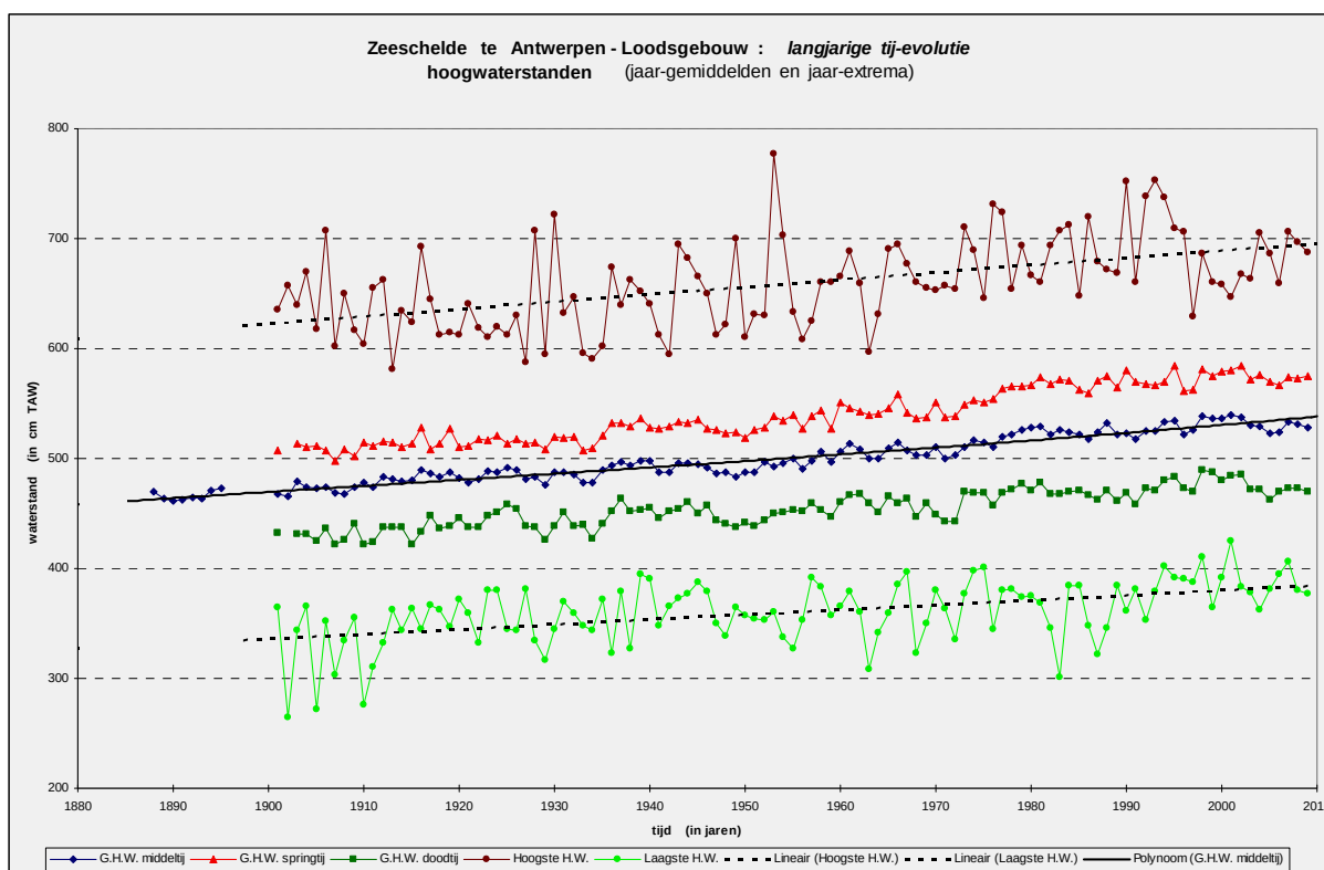
Figuur 22 - Zeeschelde te Antwerpen-Loodsgebouw: evolutie sinds 1885 (resp. 1900) van jaargemiddeld hoogwater middeltij, springtij en doottij, aangevuld met de jaarlijks hoogste en de jaarlijks laagste hoogwaterstanden
