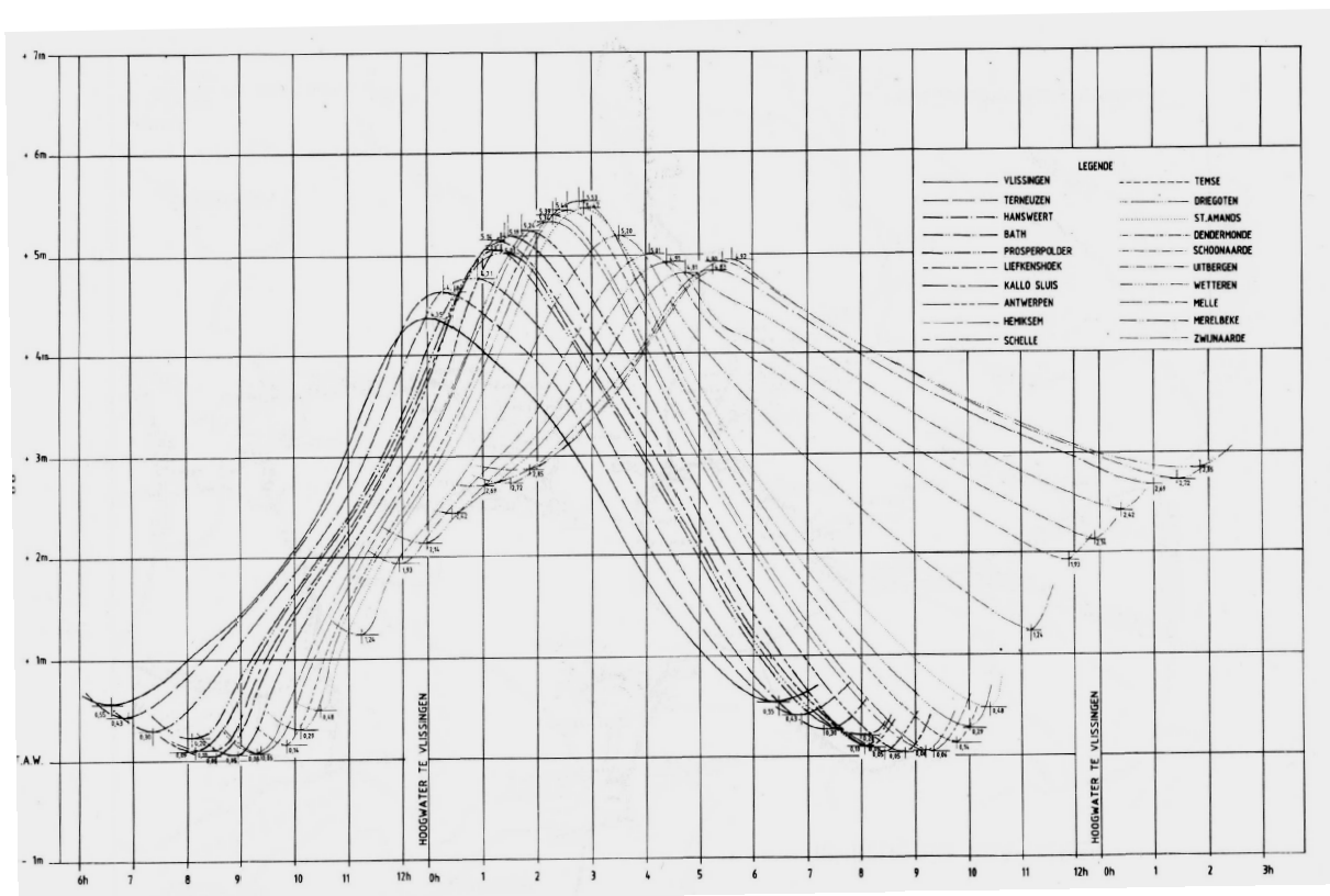
Figuur 4 - Zeescheldebekken: uittekening van de gemiddelde (middel-)tijden van (bijna) alle meetlocaties in Westerschelde en Zeescheldebekken. De tijkrommen zijn alle met hun vertraging t.o.v. het tijdstip van hoogwater te Vlissingen gezet
