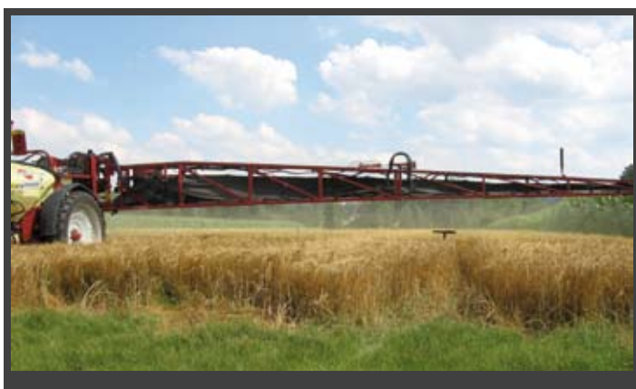
Veldmeting voor het bepalen van het effect van het gewastype op de hoeveelheid spuitdrift
