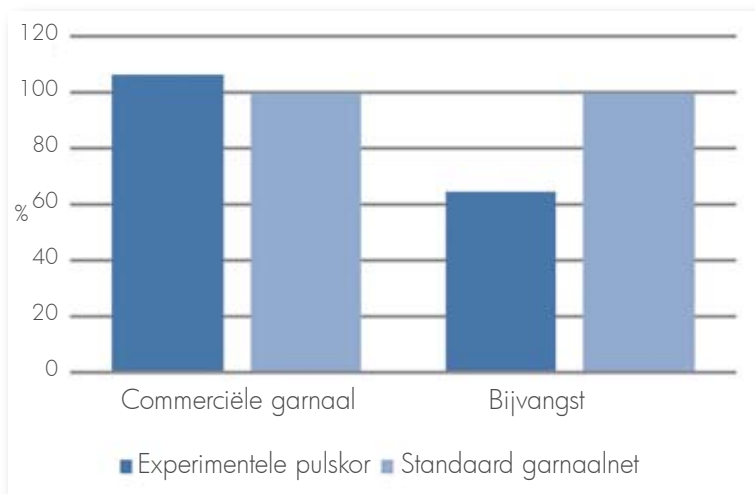
Figuur 8: Vangstvergelijking van de pulskor met de traditionele garnaalboomkor voor commerciële garnaal en bijvangst
