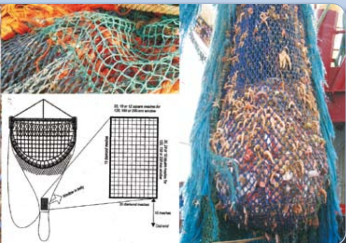
Figuur 2: Technische aanpassingen aan de alternatieve boomkor
