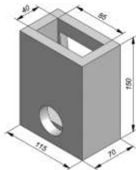
Figuur 3-42-11: uitstroombak type RA03 Eindstuk (voor taludgreppel DE02, aansluitingen en talud te bepalen, maten in cm)
