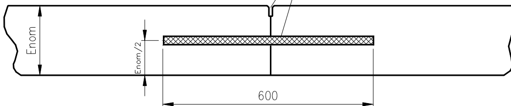
Figuur 6-1-10: dwarse werkvoeg, doorsnede A – A' (alle maten in mm)
