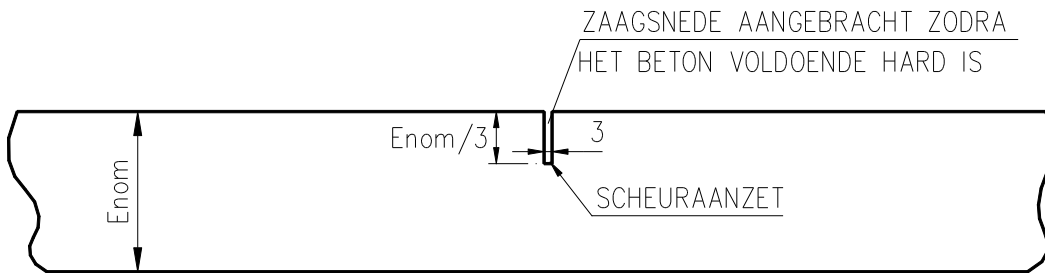
Figuur 6-1-8: doorsnede A – A' (alle maten in mm) dwarse krimpvoeg type 3: met zaagsnede zonder sponning en zonder vulvulling voor vrijliggende fietspaden, vrijliggende zijstroken en voetpaden
