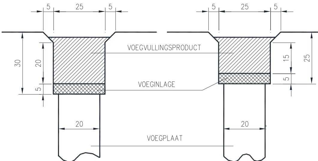
Figuur 6-1-3: dwarse uitzettingsvoeg, doorsnede A – A' (alle maten in mm)
