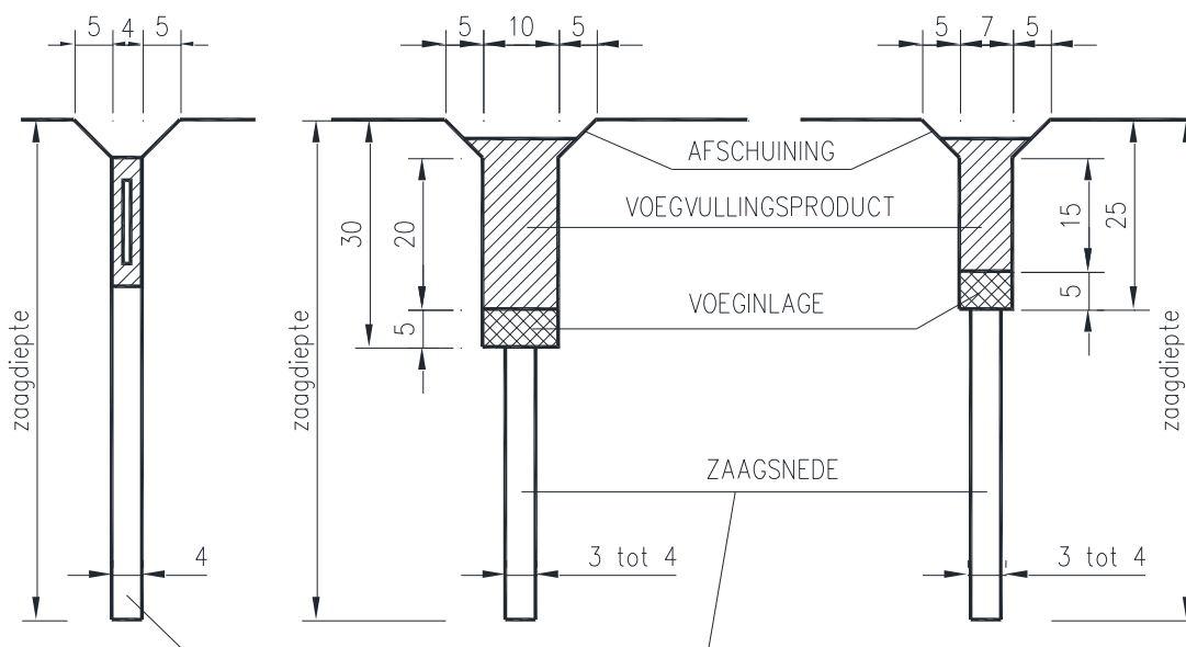
Figuur 6-1-13: langse buigingsvoeg, doorsnede A – A' (alle maten in mm)
