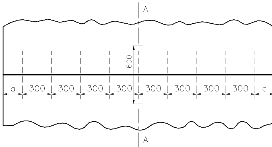
Figuur 6-1-5: bovenaanzicht dwarse krimpvoeg (alle maten in mm), 150 \leq a < 300 ZAAGSNEDEN AANGEBRACHT ZODRA HET BETON VOLDOENDE VERHARD IS
