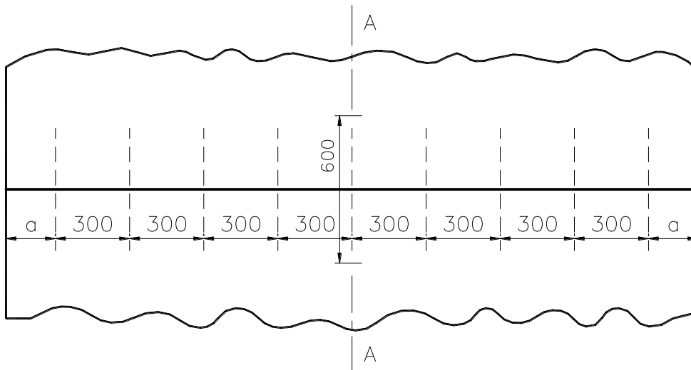
Figuur 6-1-9: bovenaanzicht dwarse werkvoeg (alle maten in mm), 150 \leq a < 300 ZAAGSNEDE AANGEBRACHT ZODRA HET BETON VOLDOENDE VERHARD IS SCHEURVORMINGSAANZET MET SPONNING DEUVEL \varnothing 25 IN GLAD STAAL BE 220
