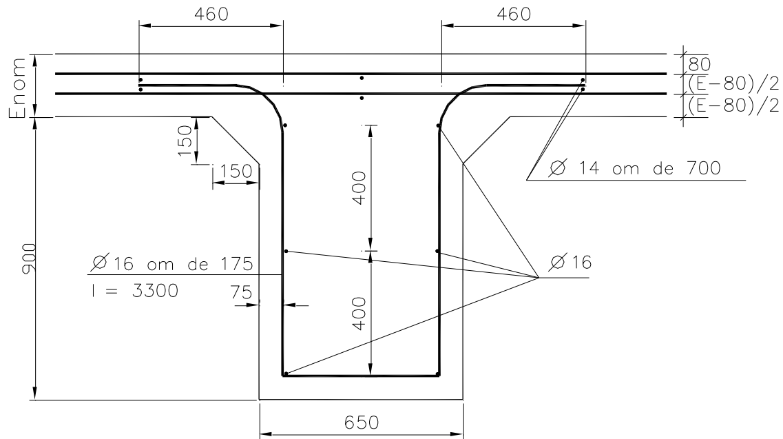
Figuur 6-1-21: dwarsdoorsnede van een rib van het verankeringslandhoofd (alle maten in mm)
