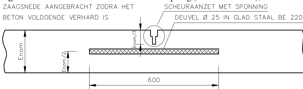
Figuur 6-1-6: doorsnede A – A' (alle maten in mm) dwarse krimpvoeg type 1: met zaagsnede en sponning met voegvulling
