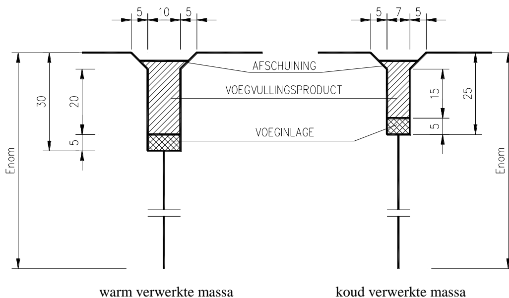
Figuur 6-1-11: detail van de dwarse werkvoeg (alle maten in mm)
