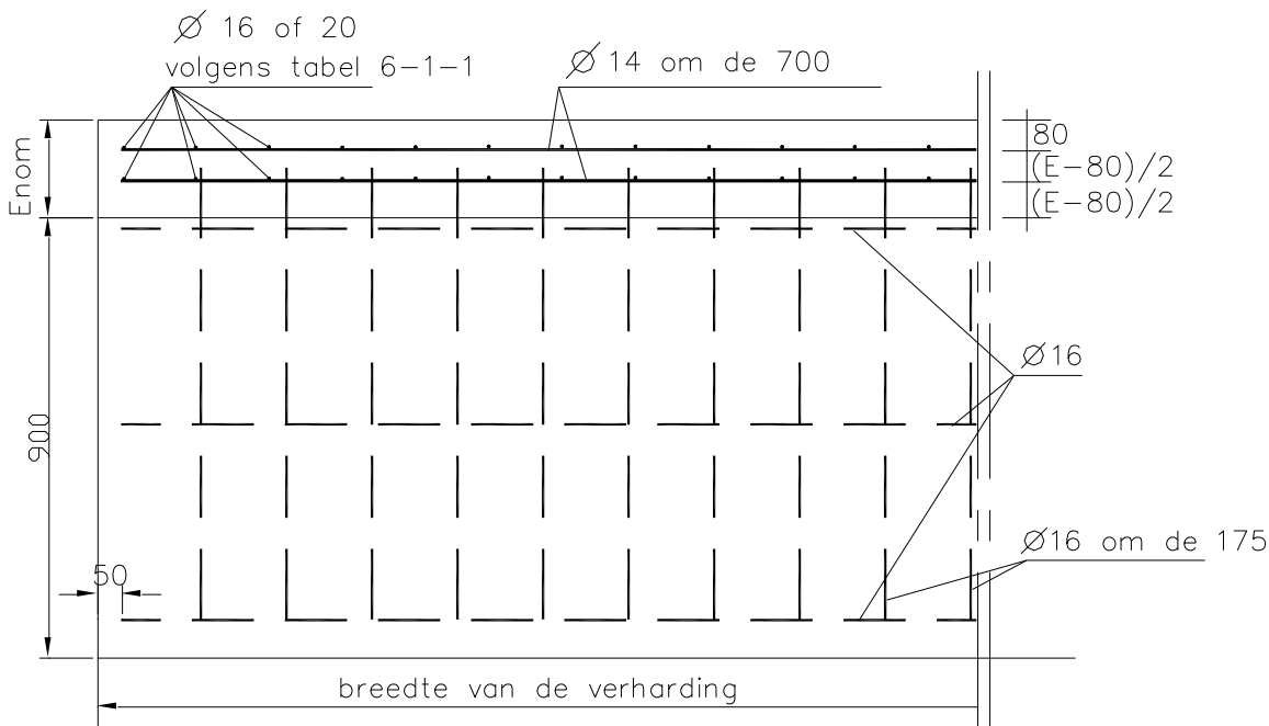
Figuur 6-1-20: dwarsdoorsnede verankeringslandhoofd (alle maten in mm)
