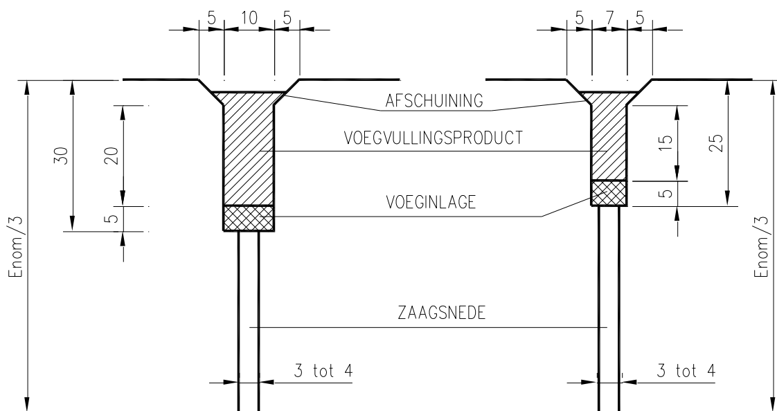
Figuur 6-1-6: doorsnede A – A' (alle maten in mm) dwarse krimpvoeg type 1: met zaagsnede en sponning met voegvulling
