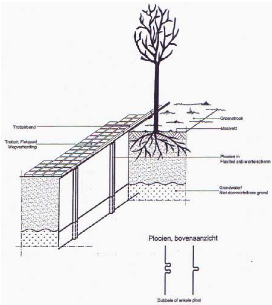
Figuur 9-19-12: detail 3 – plooiën in flexibel anti-wortelscherm Om diepe wortelgroei te stimuleren worden plooiën gevouwen nadat het flexibel anti-wortelscherm verticaal geplaatst is in een lineaire toepassing.
