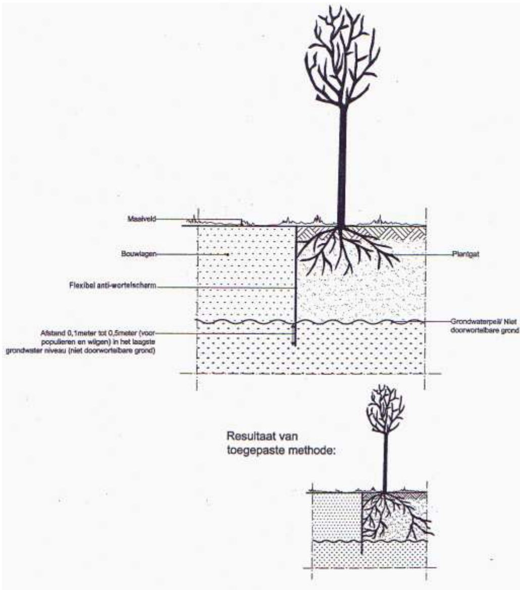
Figuur 9-19-10: detail 2a – diepte niveau flexibel anti-wortelscherm: barriërevorming door diepe toepassing
