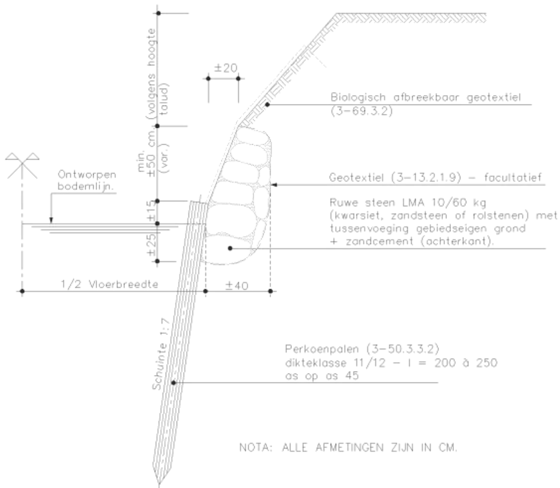
Figuur 13-2-1: taludversteving
