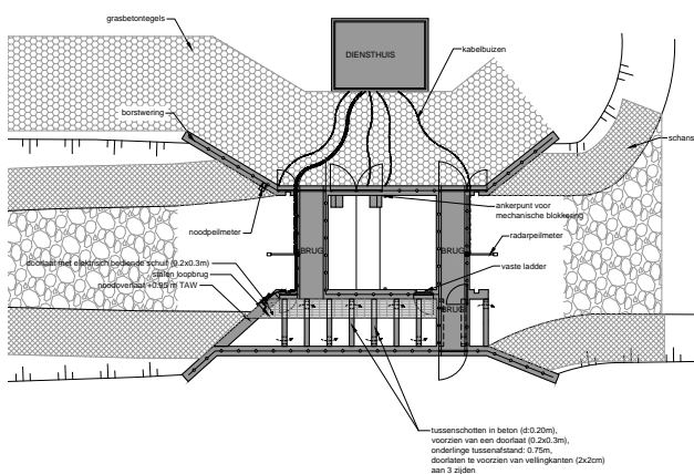
Ontwerp stuw aan Sluisstraat (fase 1)
