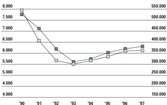
7.17 Geladen tonnenmaat en tonkilometer van de Vlaamse districten (1990-1997). Bron: dienst Regeling Binnenscheepvaart. Linkerkolom: tonnenmaat. Rechterkolom: tonkm.
