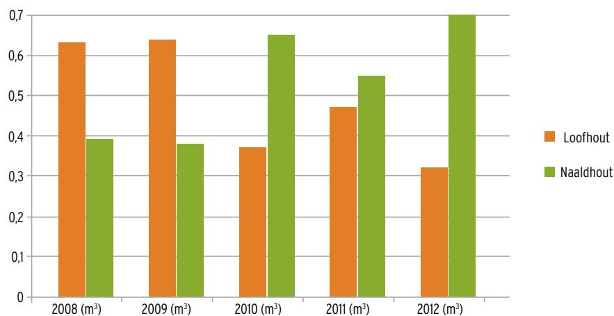
fig. 6 • verhouding loofhout-naaldhout in het verkocht FSC-hout voor de periode 2008-2012
