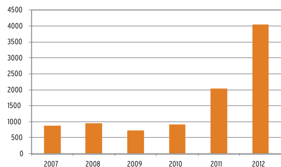
fig. 9 • houtige biomassa vrijgekomen bij werken in eigen regio (ton/jaar)
