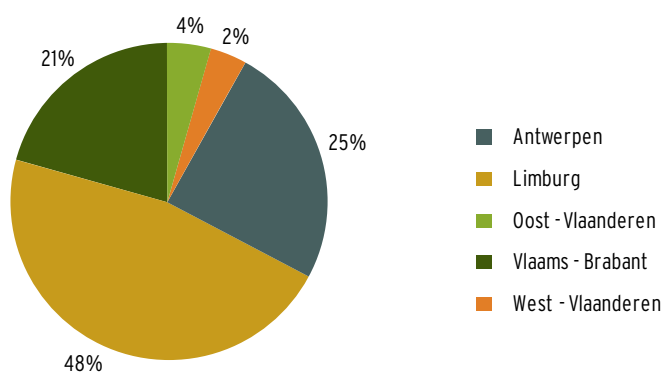
fig. 5 • provinciale spreiding verkocht FSC-hout in 2012
