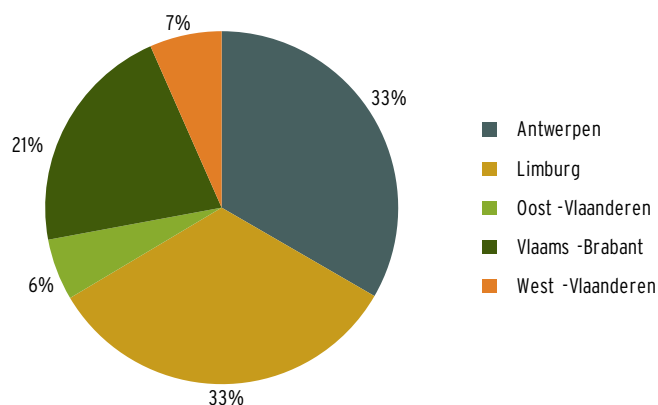
fig. 4 • provinciale spreiding verkochte volumes ANB-domeinen 2012
