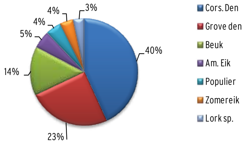
fig. 7 • Drie boomsoorten zijn samen goed voor bijna 80% van het totale gekapte FSC-volume: Corsicaanse den, Grove den en Beuk.
