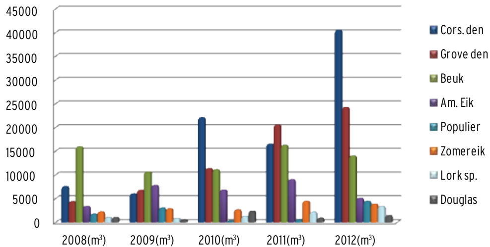
fig. 8 • verkoop aandeel economische belangrijke soorten voor de periode 2008-2012
