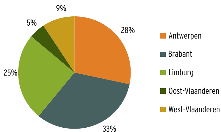
fig. 18 • verdeling verkocht houtvolume over provincies, totaal 411.748m 3
