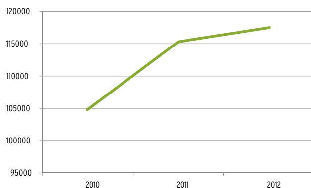
fig. 3 • volume verkochte hout in m 3 - 2010-2012
