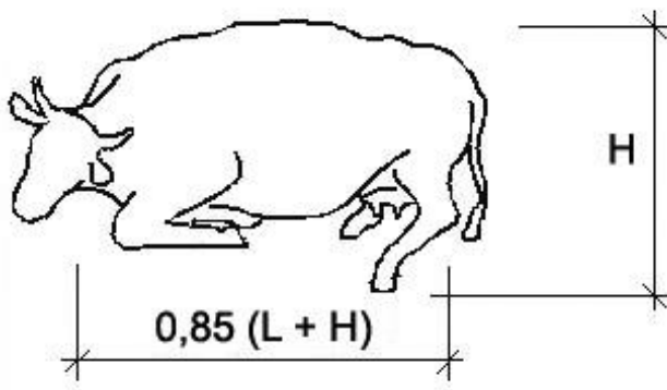
Figuur 16: Minimale ruimtebehoefte voor een liggende koe.
