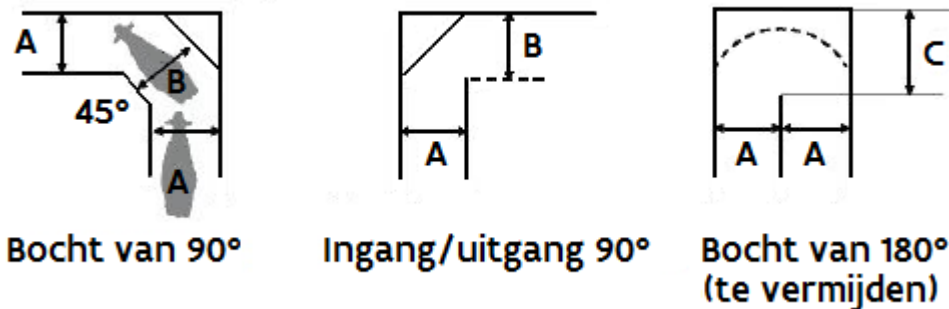
Figuur 73: Minimumbreedtes in bochten met koeverkeer in één richting ( A ). De stippellijn toont een optie om het koeverkeer in een rechte hoek te verbeteren. Bochten van 180^\circ moeten vermeden worden om stroom van dieren te verbeteren en verwondingen te minimaliseren.
