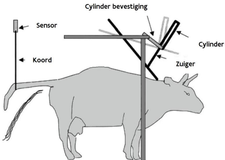
Figuur 29: Mechanisch-pneumatisch systeem (“Aktorik”).
