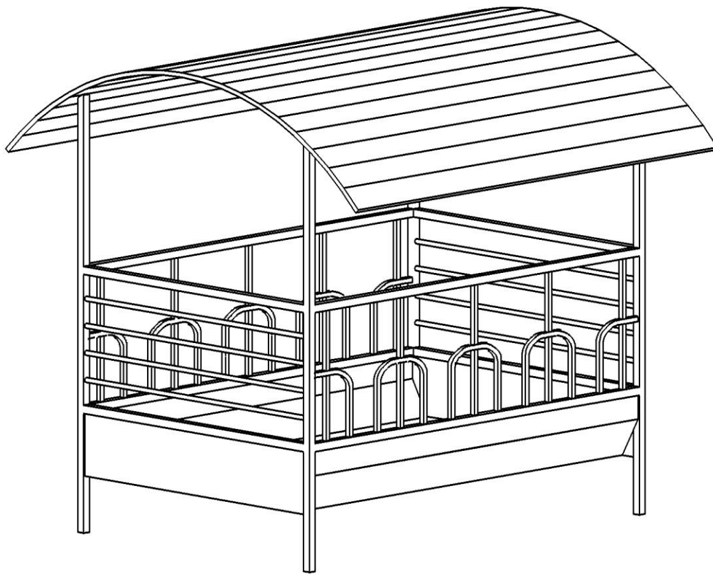
Figuur 41: Voorbeeld van een mobiele hoorruif.
