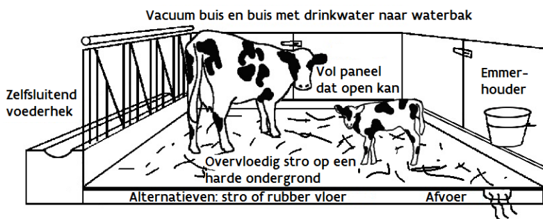
Figuur 75: Voorbeeld van ontwerp en uitrusting van een individuele afkalffox.
