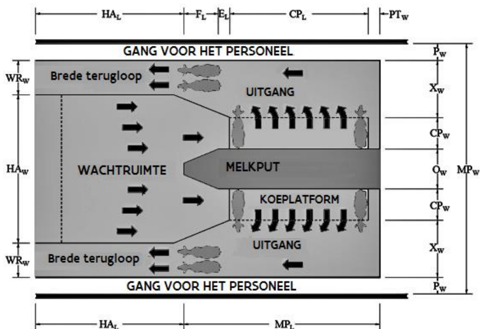
Figuur 58: Zij aan zij melkstal met rapid exit en dubbele terugloopgang (naar DPC 54).
