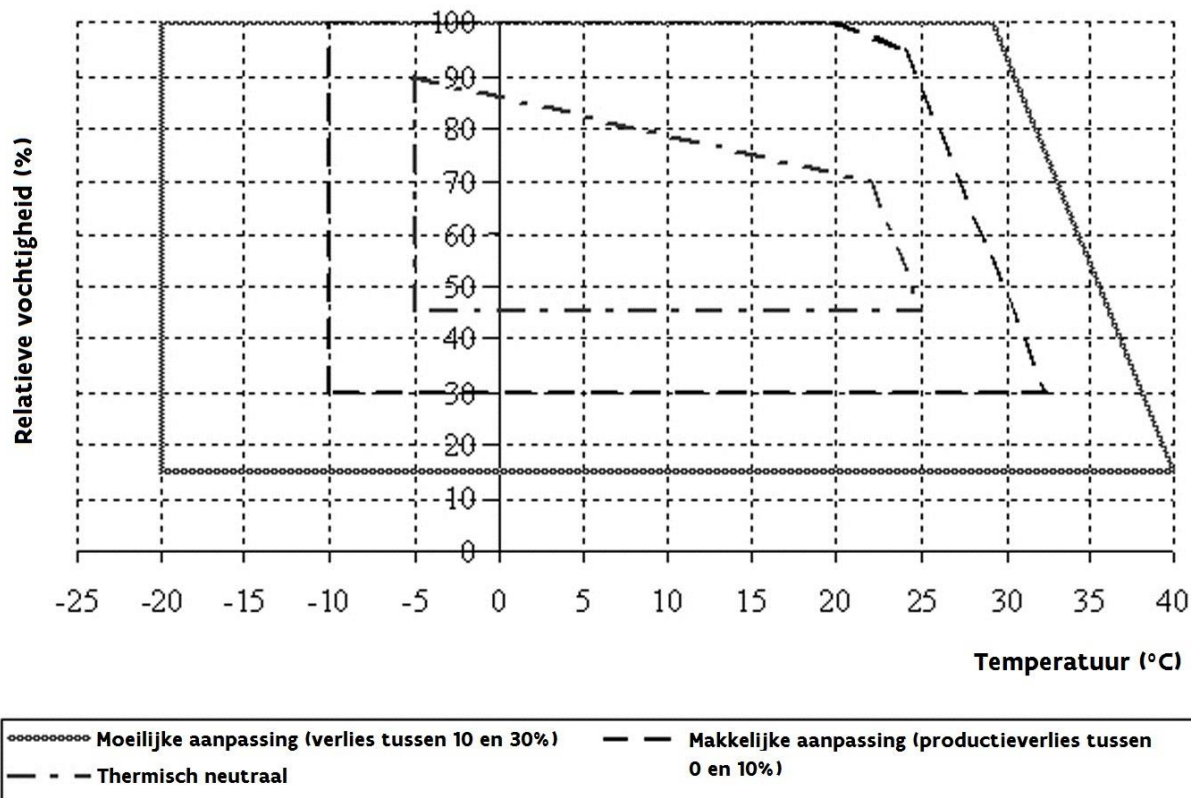
Figuur 5: Grafiek die de limieten van gelijkaardige dierlijke productieve respons weergeeft in functie van luchttemperatuur en relatieve vochtigheid bij een lichtsnelheid van 0,5 m/s.
