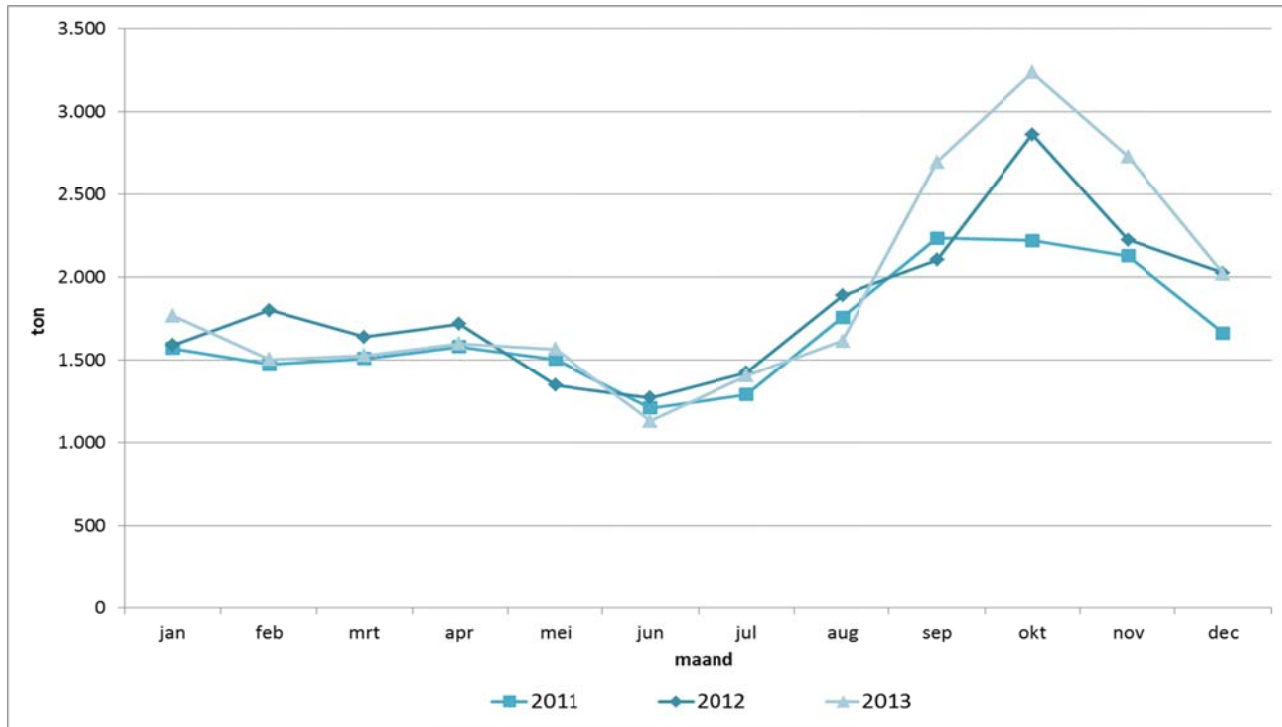
Grafiek 4 : Maandlijks totaal aanvoergewicht in Belgische + vreemde havens
