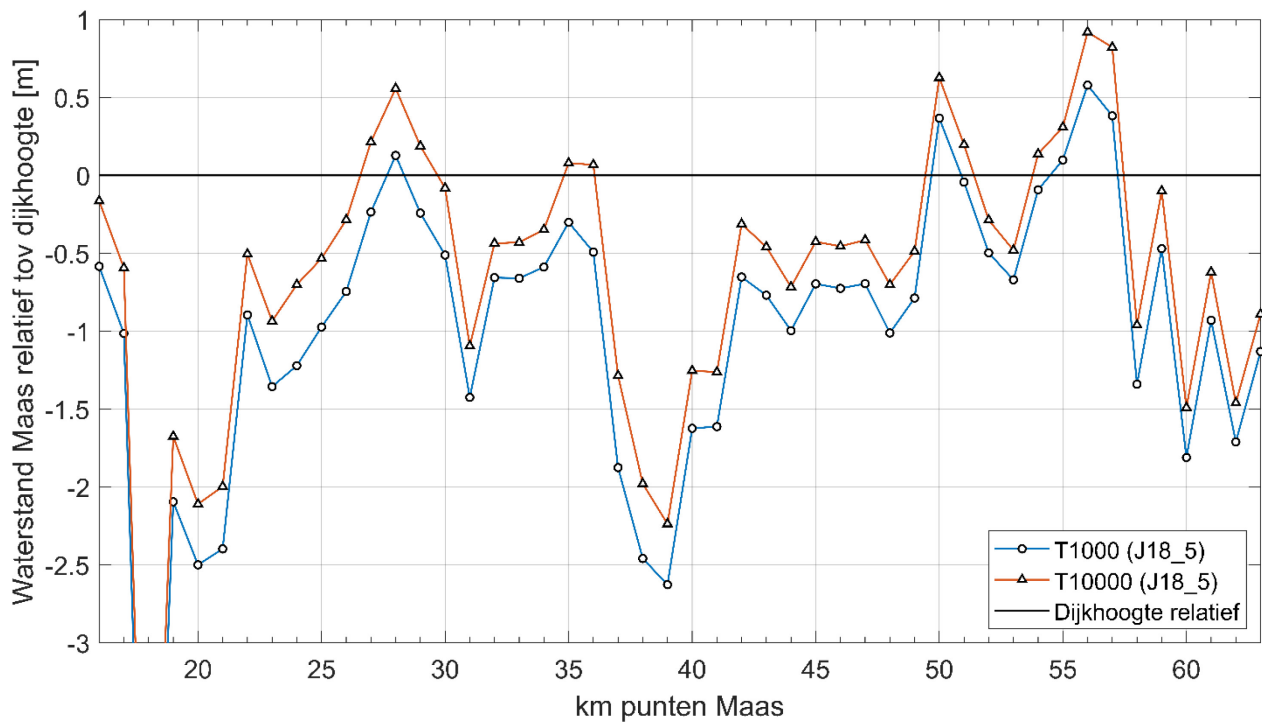
Figuur 4 Waterstand van de Maas voor een T1000 en T10000 (model J18_5) relatief t.o.v. de dijkhoogte.
