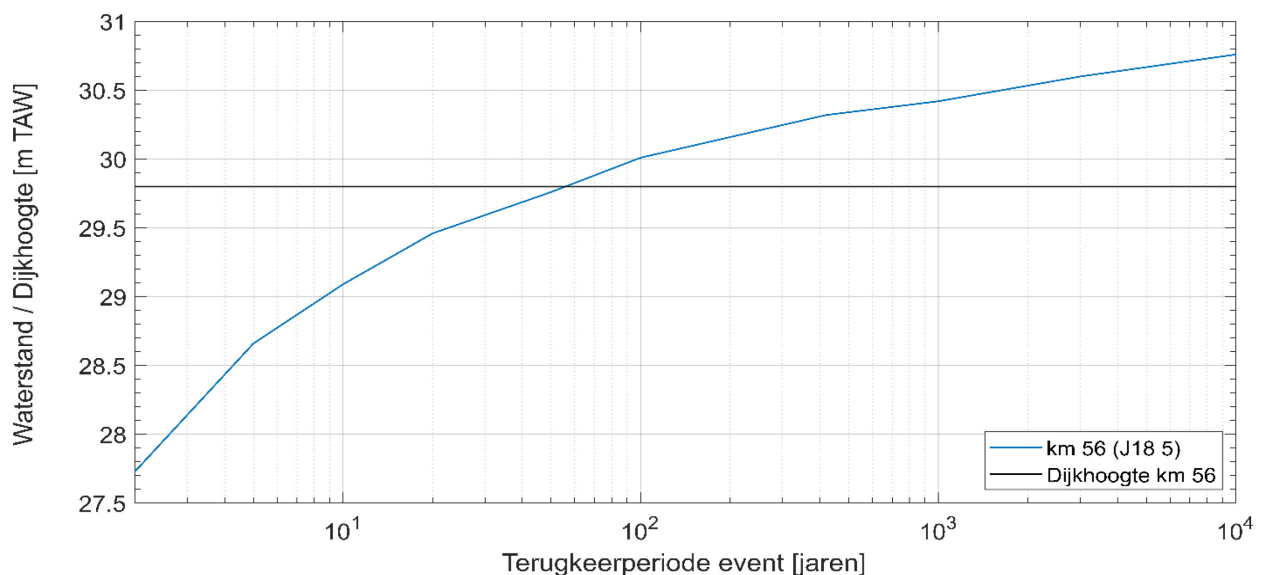
Figuur 7 Waterstanden aan km 56 voor verschillende terugkeerperiodes van events vergeleken met de dijkhoogte op km 56
