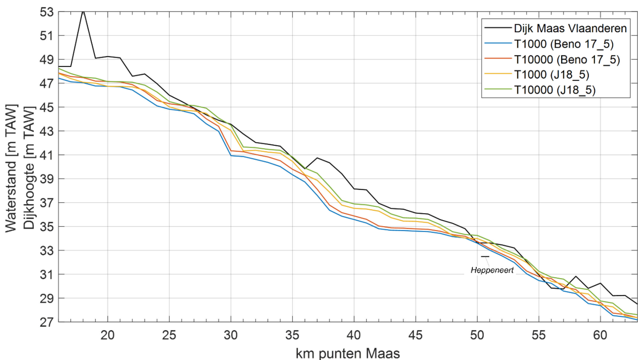
Figuur 3 Waterstanden in WAQUA J18_5 en BenO17_5 voor T1000 en T10000 vergeleken met de hoogtes van de winterdijk in Vlaanderen
