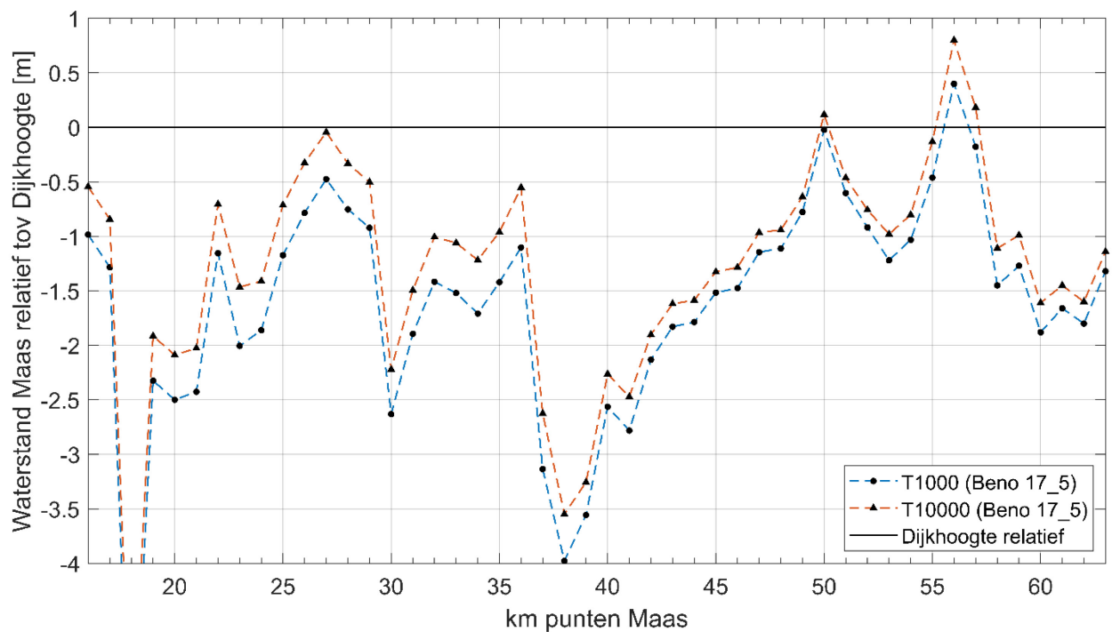
Figuur 5 Waterstand van de Maas voor een T1000 en T10000 (model BenO17_5) relatief t.o.v. de dijkhoogte.
