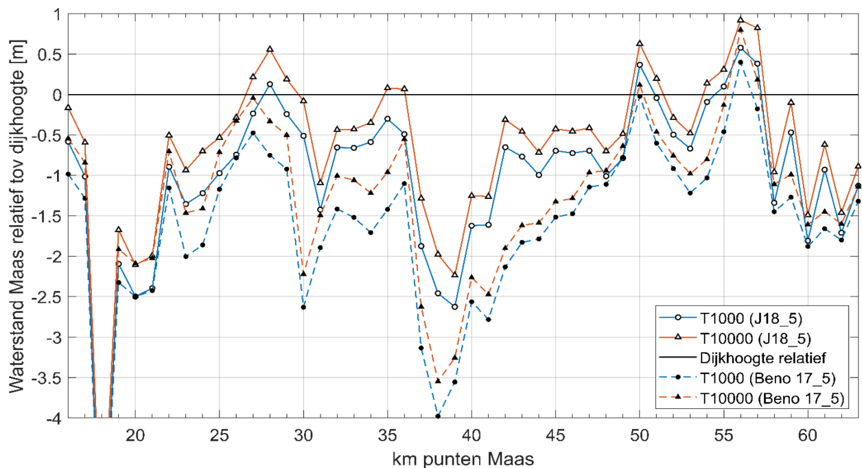
Figuur 6 Waterstand van de Maas voor een T1000 en T10000 (model J18_5 tezamen met BenO17_5) relatief t.o.v. de dijkhoogte.
