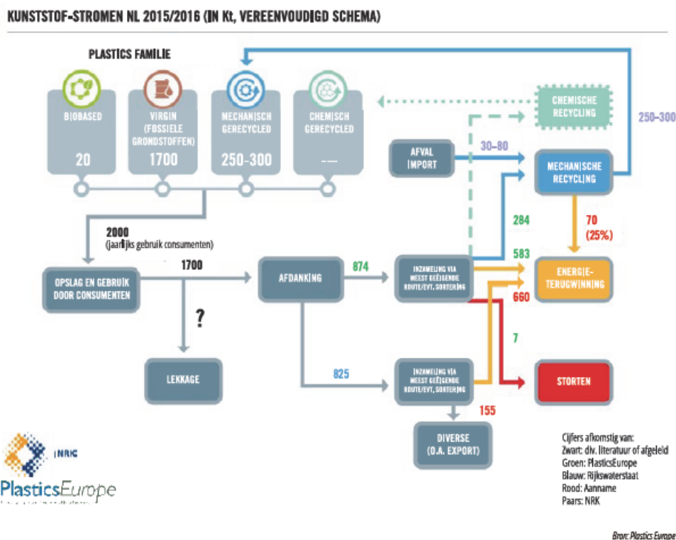
Figuur 4: Kunststofstromen in Nederland (2015/2016, in kT) 23
