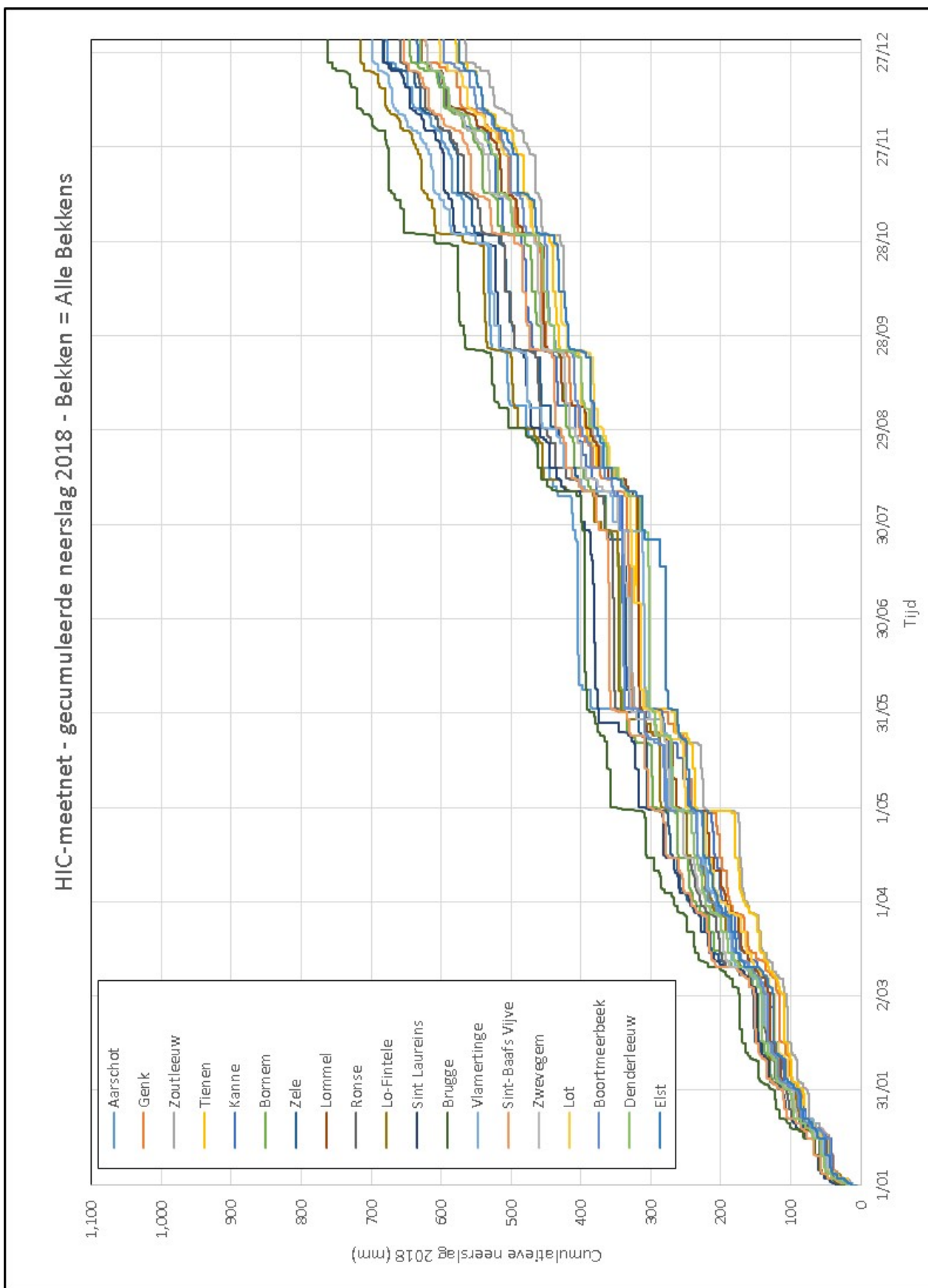
Figuur 2 – Overzicht gecumuleerde neerslag van de 19 HIC stations in 2018 - gevalideerde meetreeksen
