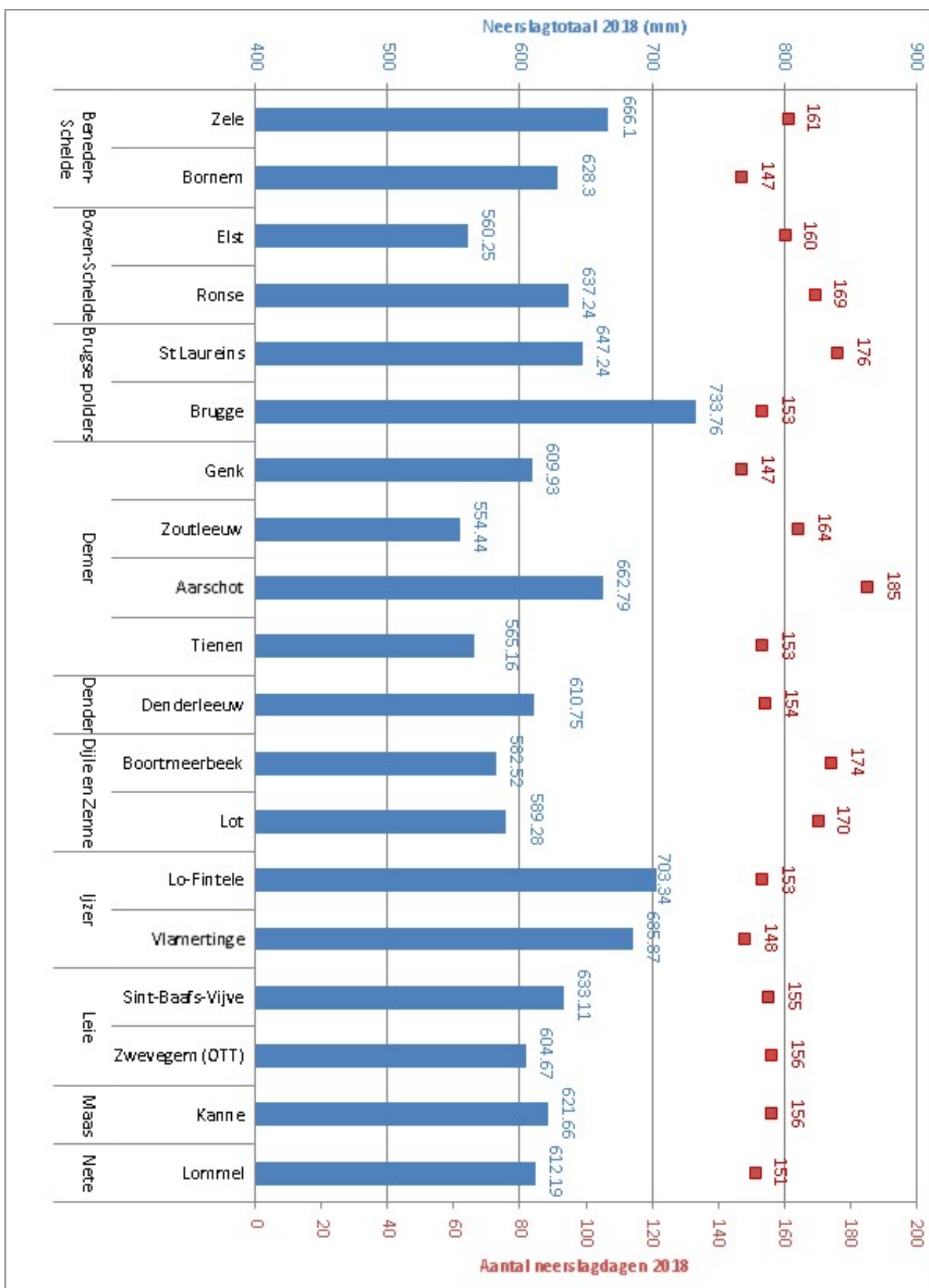
Figuur 1 – Overzicht van de neerslagtotalen en het aantal neerslagdagen van de 19 HIC stations in 2018.
