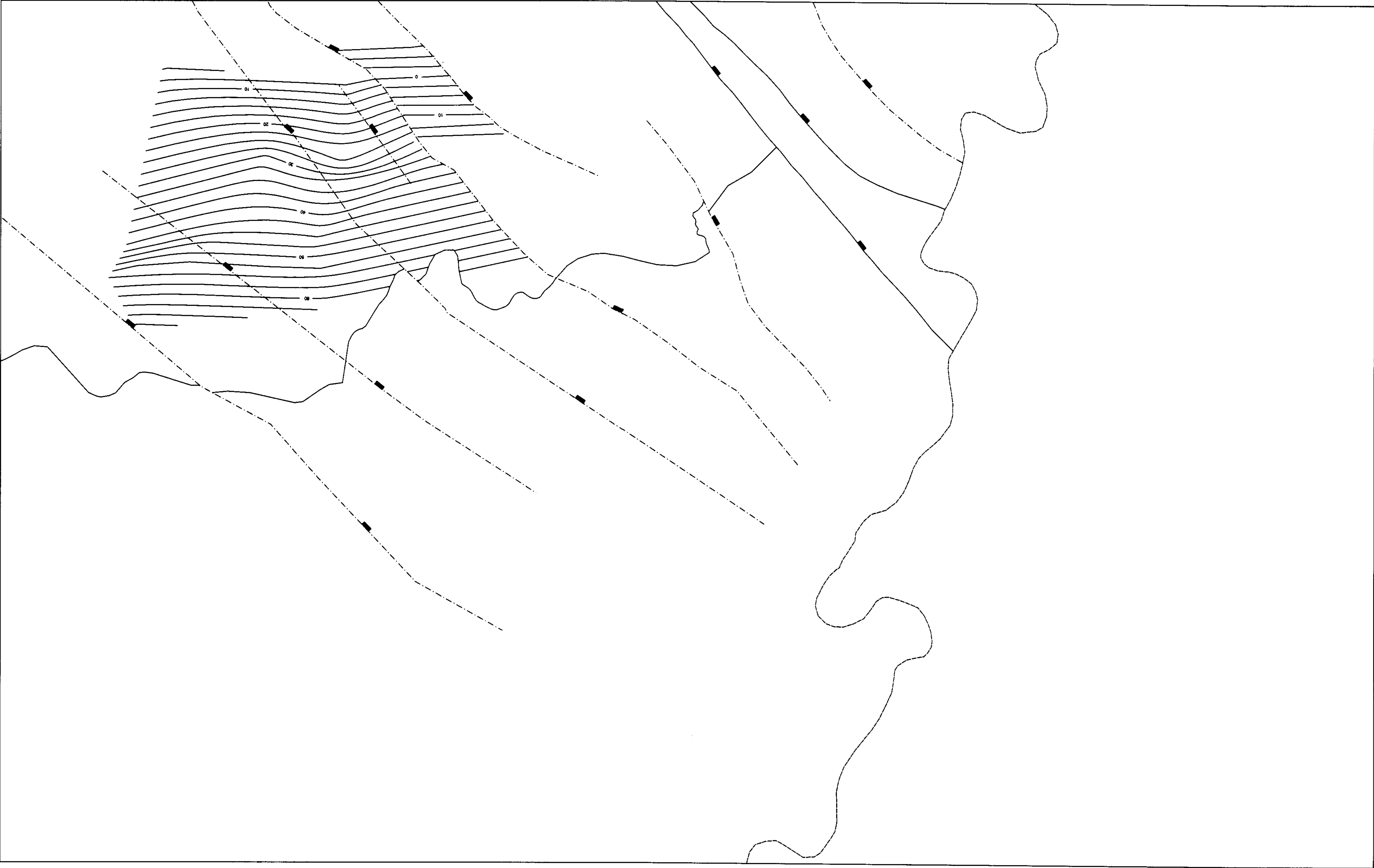
OVERLEGFOLIE 4: ISOHYPSEN VAN DE BASIS VAN DE FORMATIE VAN DIEST
