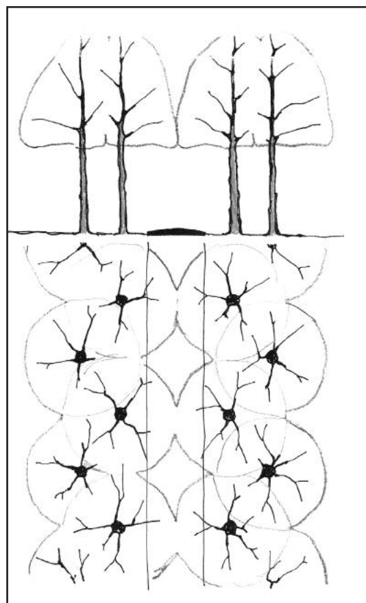
FIG 160 Dubbele dreef met driehoeksverband (tekening: Geert Van der Linden)
