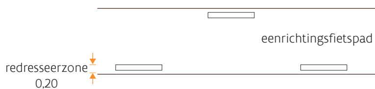
figuur 8: Voorbeeld van toepassing van een randmarkering als onderdeel van de redresseerzone
