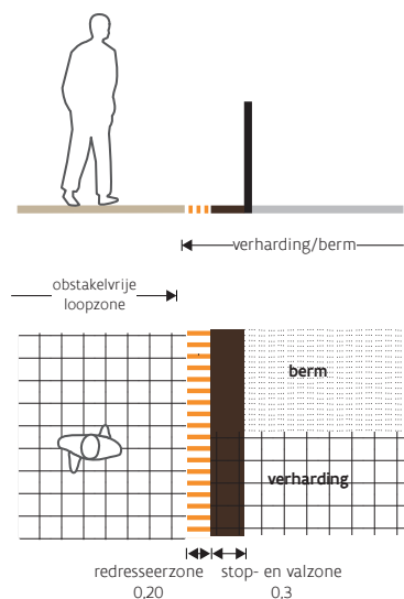
figuur 4: Toepassing redresseerzone en stop- en valzone voor voetgangers
