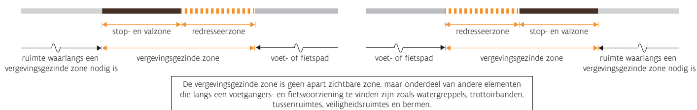
figuur 2: schematische weergave van de vergevingsgezinde zone, redresseerzone en stop- en valzone tussen een rijbaan en een voet- of fietspad
