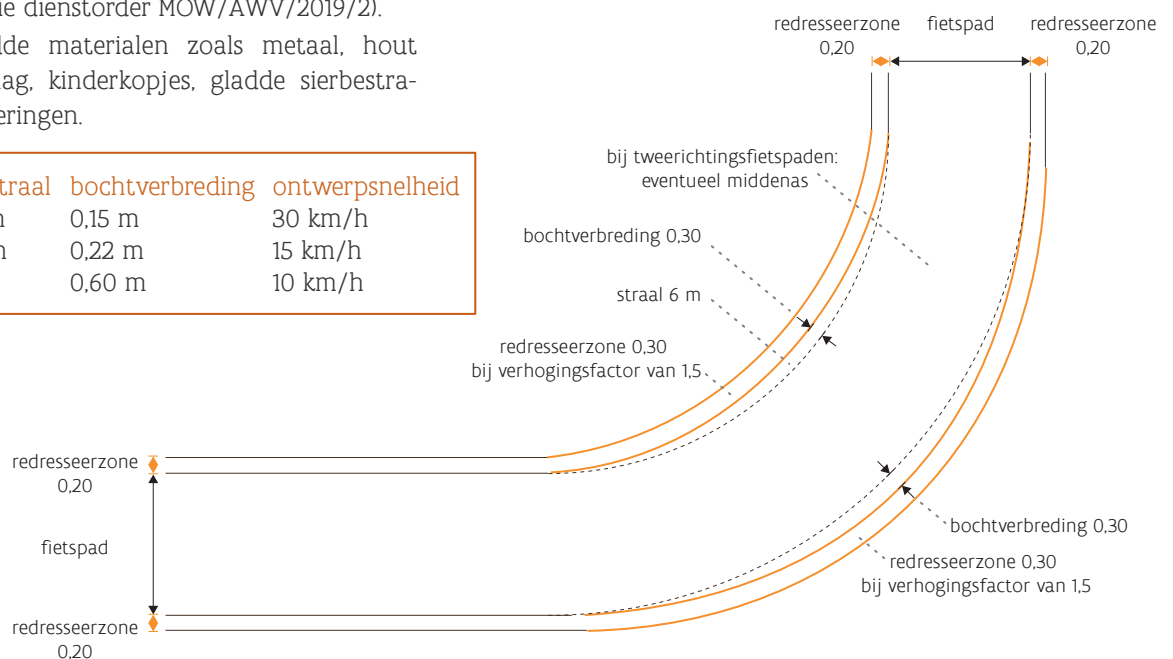
figuur 7: Bochtverbreiding bij een minimale boogstraal van 6 m
