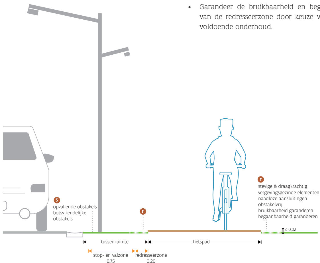
figuur 13: Voorbeeld druk vrijliggend fietspad
