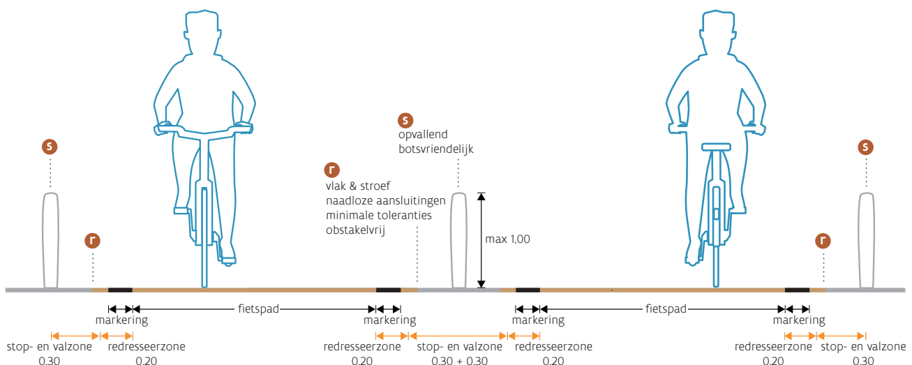
figuur 9 Voorbeeld fietspad met paaltjes
