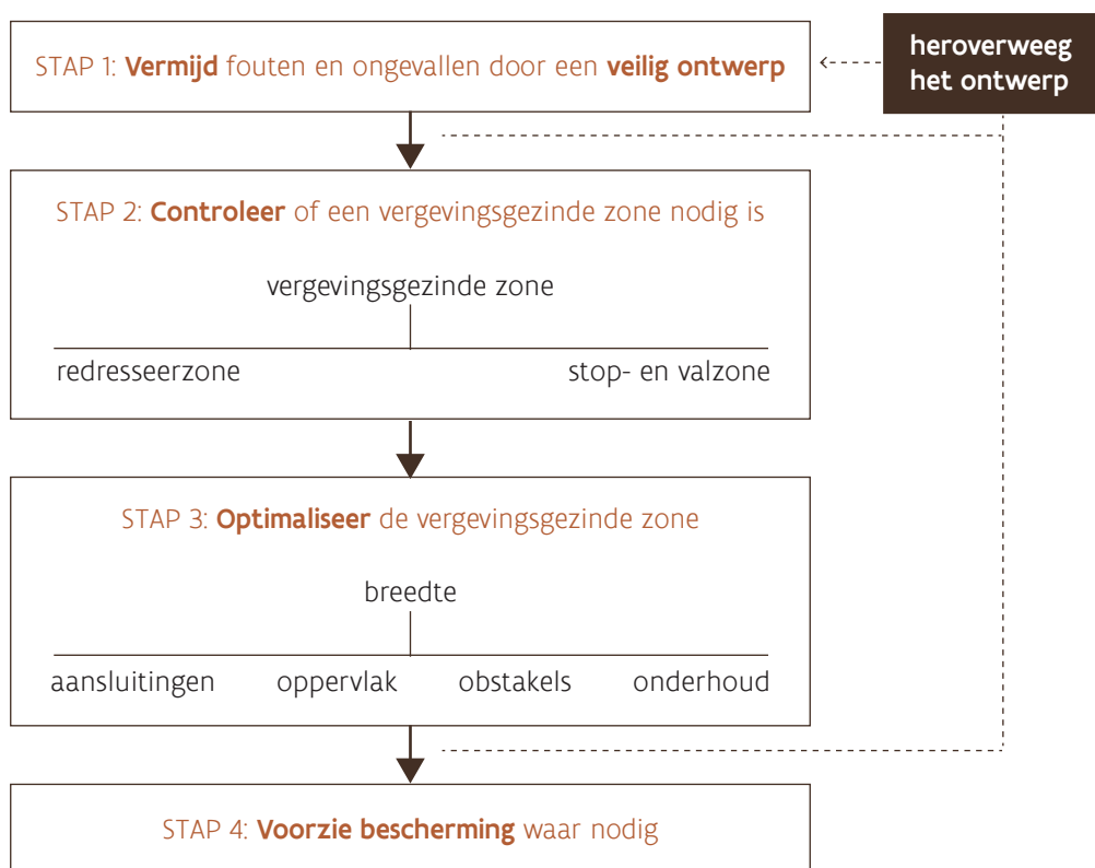
figuur 1: Stappenplan vergevingsgezinde infrastructuur kwetsbare weggebruikers
