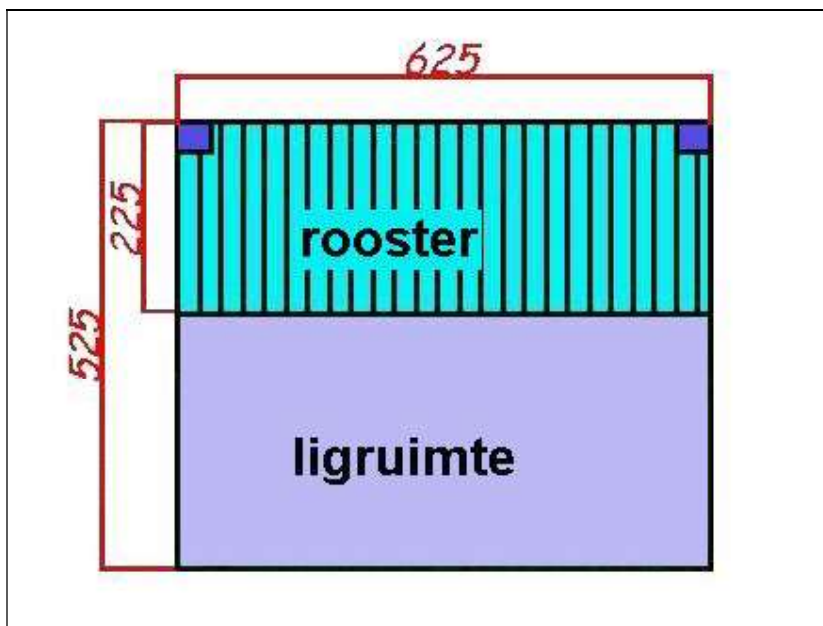
Figuur 30 Voorbeeld 2 stal lay-out voor 14 onbepikt gevoederde zeugen
