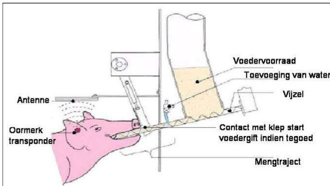
Figuur 35 Schema nippelvoeding
