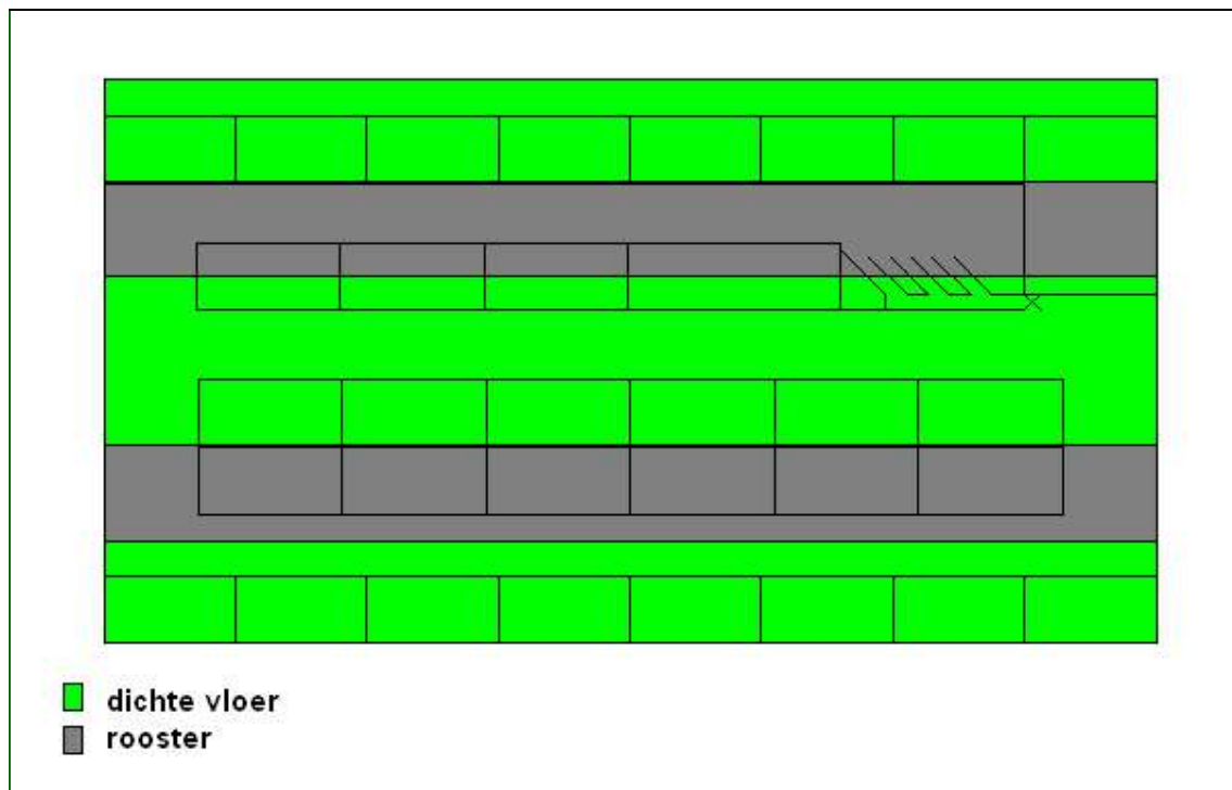
Figuur 56 Mogelijke stallay-out na renovatie naar voederstations (hier met 1 grote groep)
