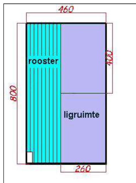
Figuur 37 Voorbeeld van een stal lay-out voor 15 zeugen en een nippelstation
