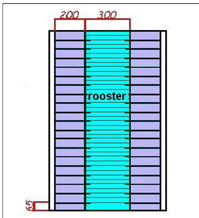
Figuur 22 Voorbeeld stal lay-out voederligboxen met uitloop
