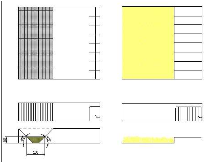
Figuur 13 Mogelijke emissie-arme uitvoering van het dropvoedersysteem (links V-3.5 en rechts V-3.7)
