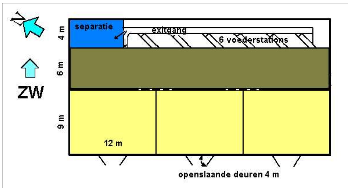
Figuur 19 Door ASG-Praktijkonderzoek aanbevolen stalmodel
