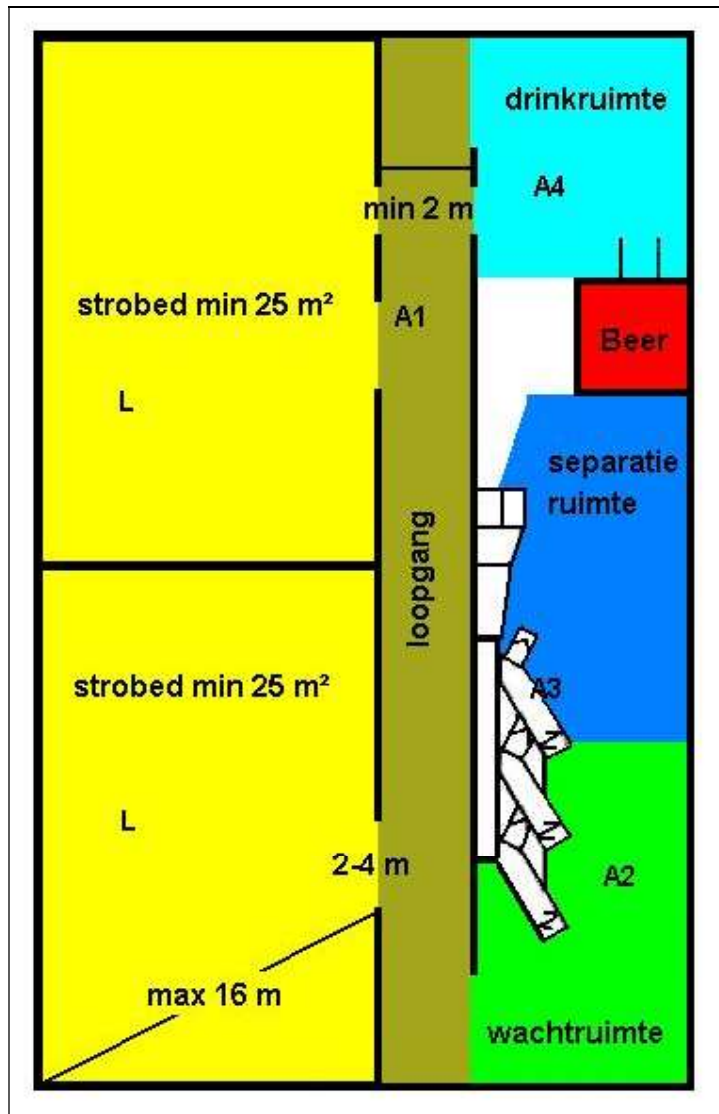
Figuur 18 Emissie-arm systeem voor zeugen V-3.6
