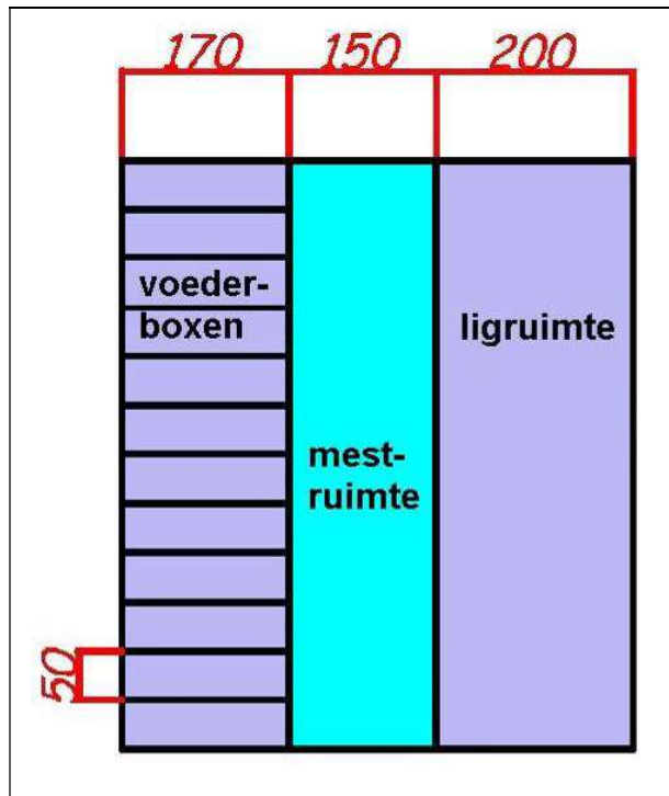
Figuur 24 Voorbeeld stal lay-out met aparte ligruimte
