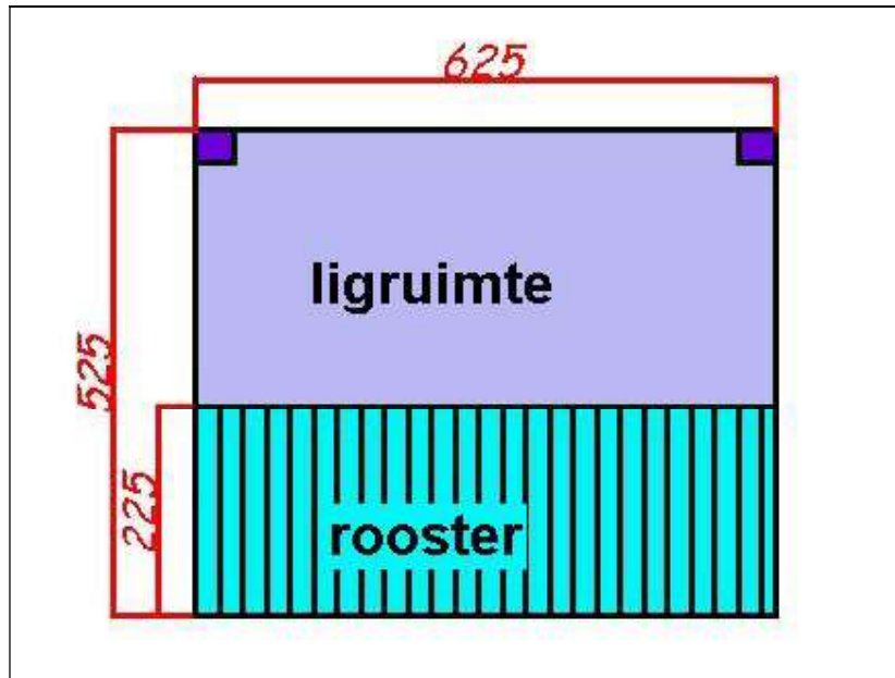
Figuur 29 Voorbeeld 1 stal lay-out voor 14 onbeperkt gevoederde zeugen
