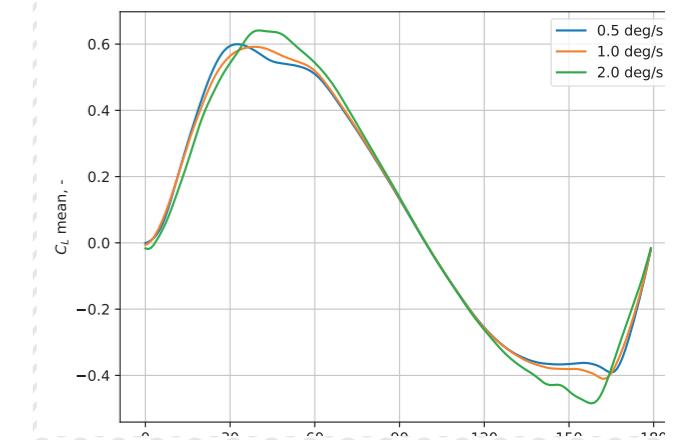
Fig. 1 – Visualisatie van (a) het rekenrooster rond een NACA roer en (b) de stroming rond het roer bij kleine invalshoek. Fig. 2 – Lift coëfficiënt op het roerblad als functie van de invalshoek, (a) invloed van rotatiesnelheid, (b) gemiddelde data per rotatiesnelheid.
