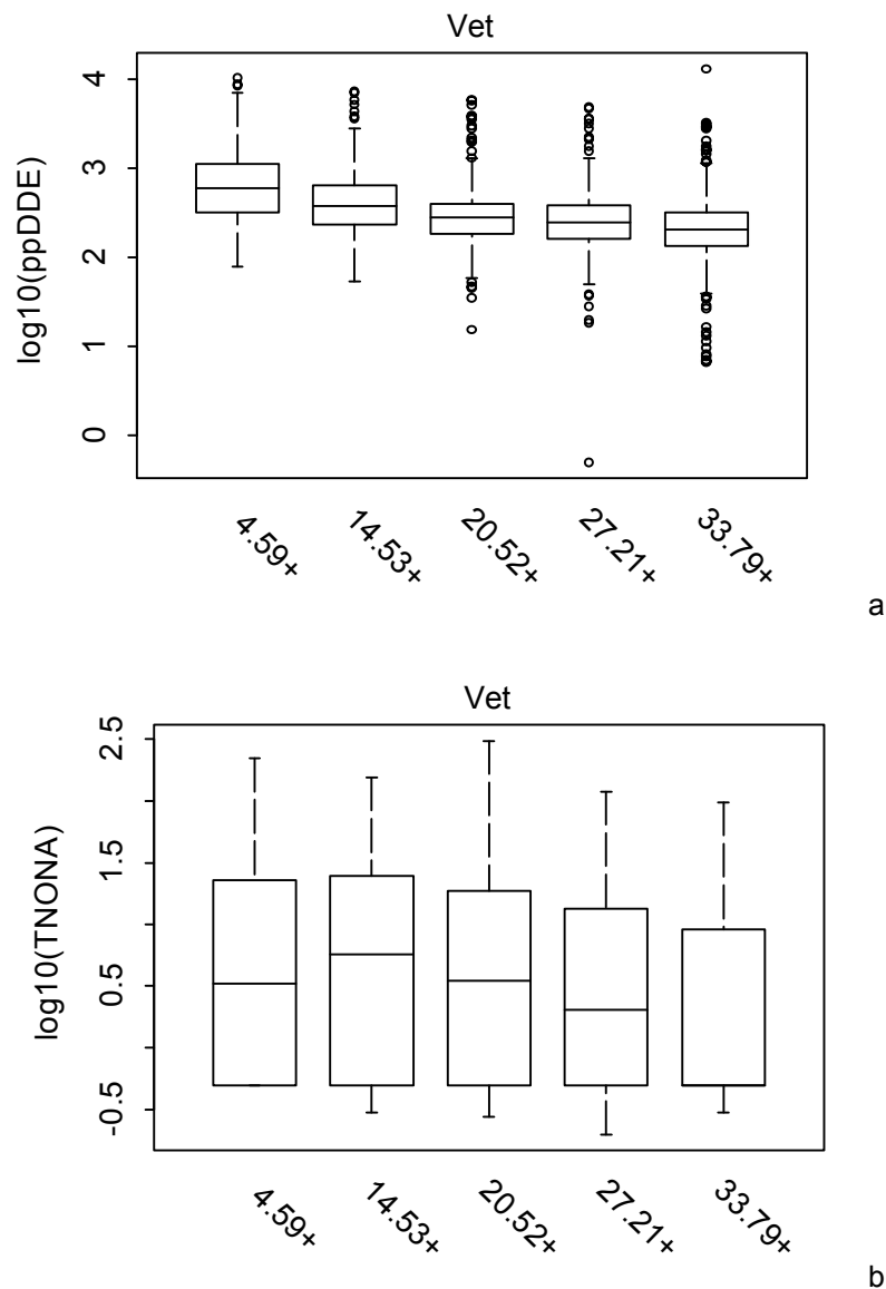
Figuur 6.11: (a) Er is een licht dalende trend voor pp' -DDE; (b) Voor TNONA schommelt het vetpercentage.
