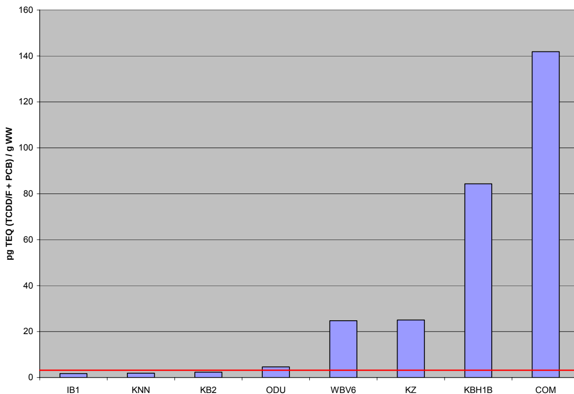
Figuur 6.15: Concentraties aan dioxines, furanen en dioxineachtige PCB's in spierweefsel van paling (Vlaanderen 2001-2005). De rode lijn stelt de grens voor waarboven de embryonale ontwikkeling van paling sterk negatieve gevolgen ondervindt (4 pg TEQ(PCDD's/PCDF's + PCB's)/g ww).
