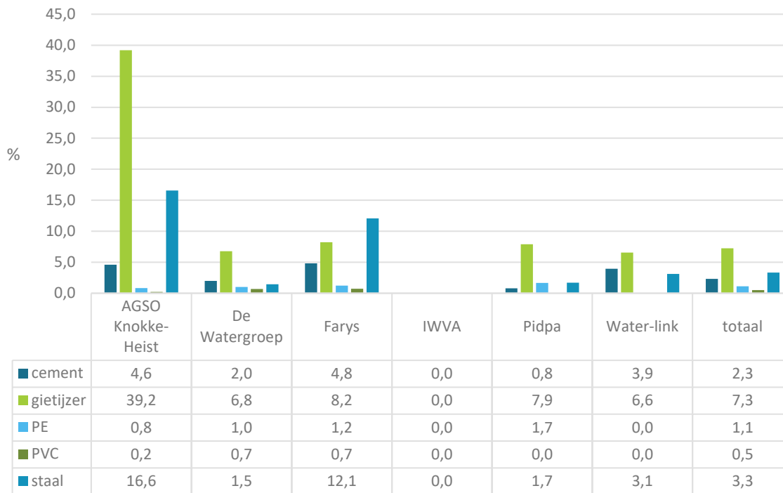
Figuur 13 Aandeel toevoer- en distributieleidingen ouder dan de technische levensduur per materiaal per waterbedrijf (2019)
