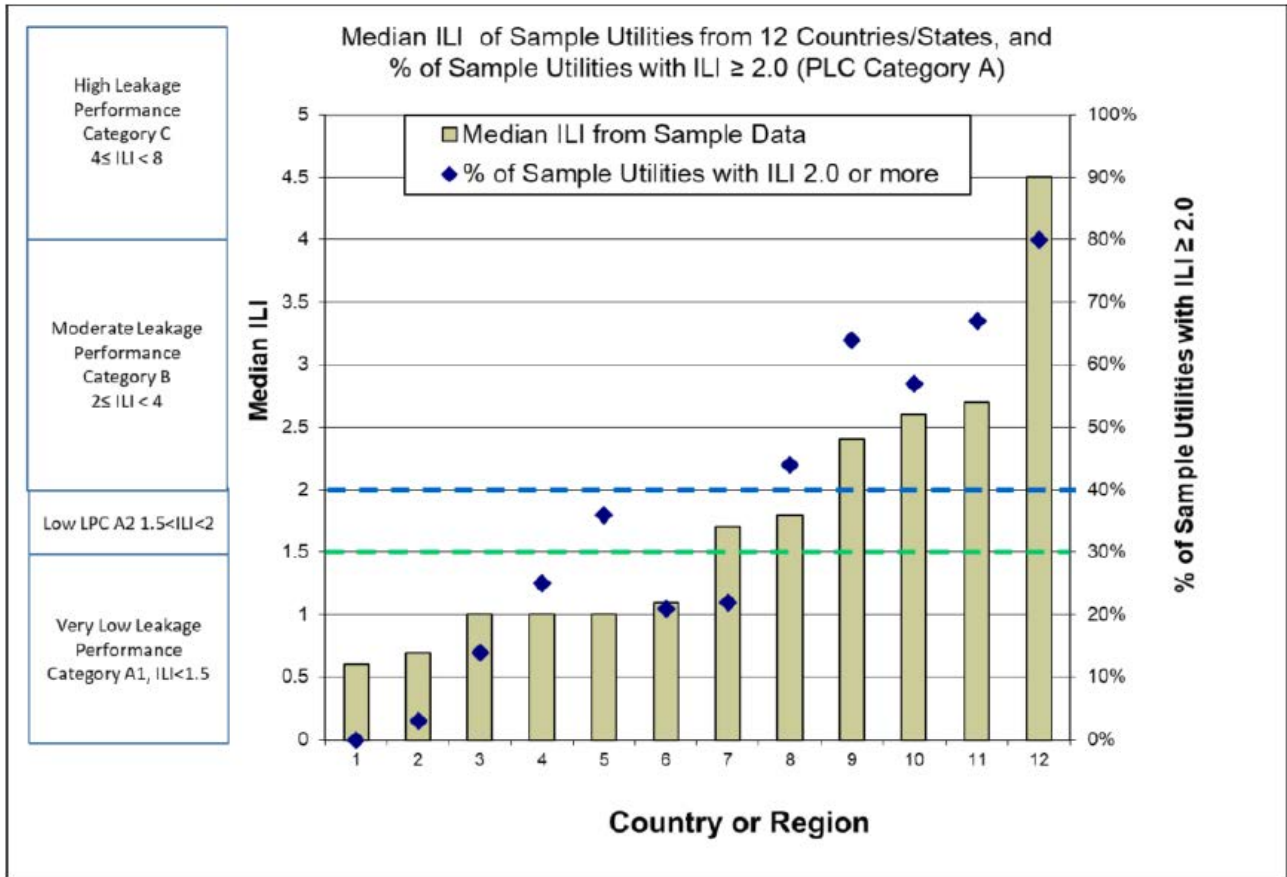
Figuur 8 Internationale vergelijking ILI waterbedrijven 17
