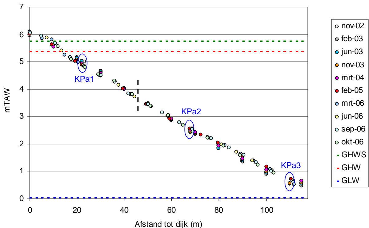
Figuur 5.21: Hoogteprofiel van de a-raai, met gemiddeld hoog (GHW) en laag water (GLW) en gemiddeld hoogwater bij springtij (GHWS). De verticale stippellijn duidt de grens aan tussen hersteld gebied en oorspronkelijk slik.
