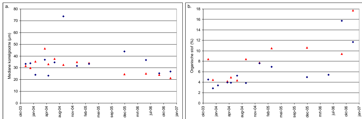
Figuur 6.9: Mediane korrelgrootte (a) en percentage organische stof (b) op locatie PA3 voor de diepte fracties 0-10cm (◇) en 0-1cm (△).
