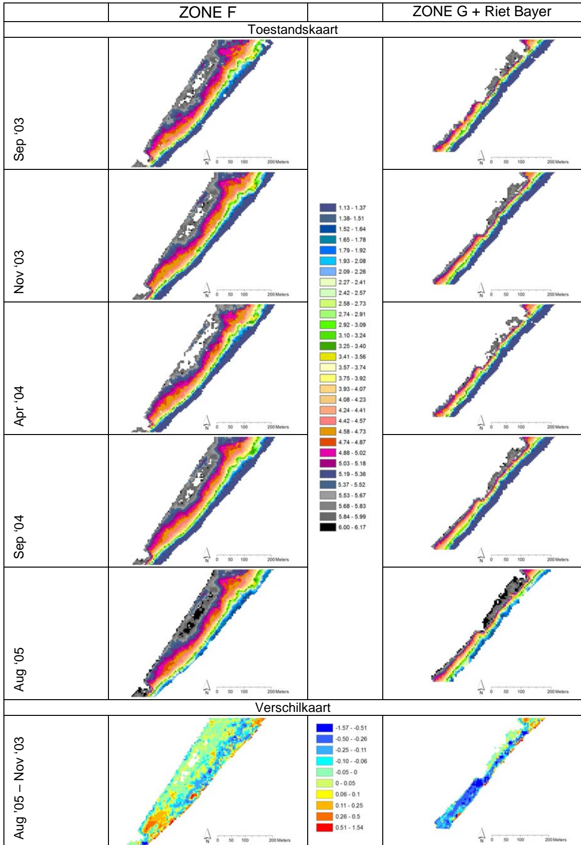
Figuur 5.15: Toestandskaarten en verschilkaarten op basis van DTM's van zones F, G en het rietveld ter hoogte van Bayer op Ketenisse schor.
