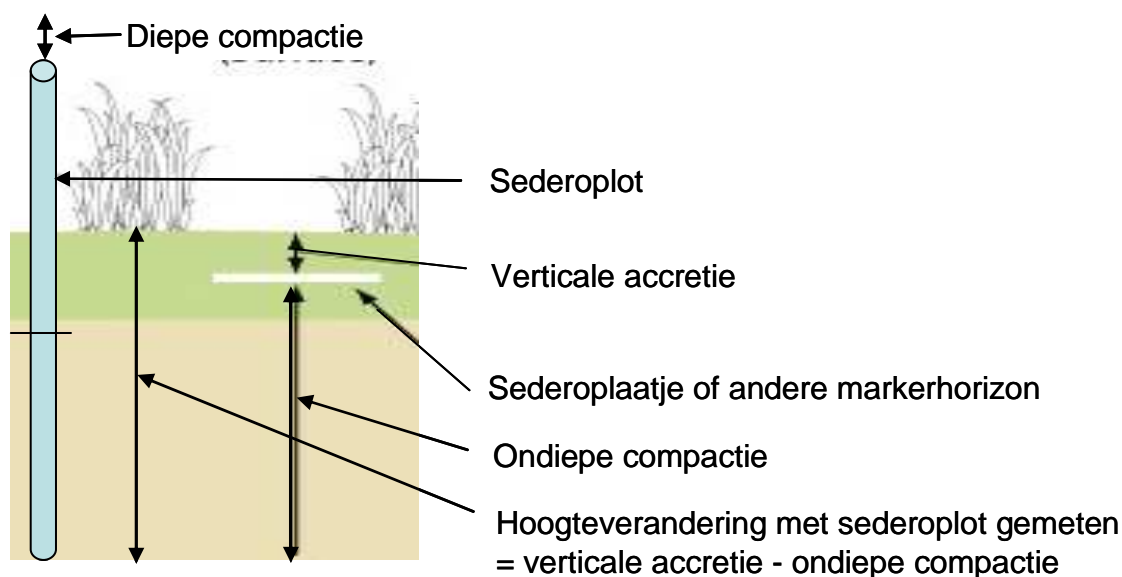
Figuur 12.1: Mogelijke meetmethoden om de verschillende oorzaken van hoogteveranderingen na te gaan bij het gebruik van sederplots en sederplaatjes.
