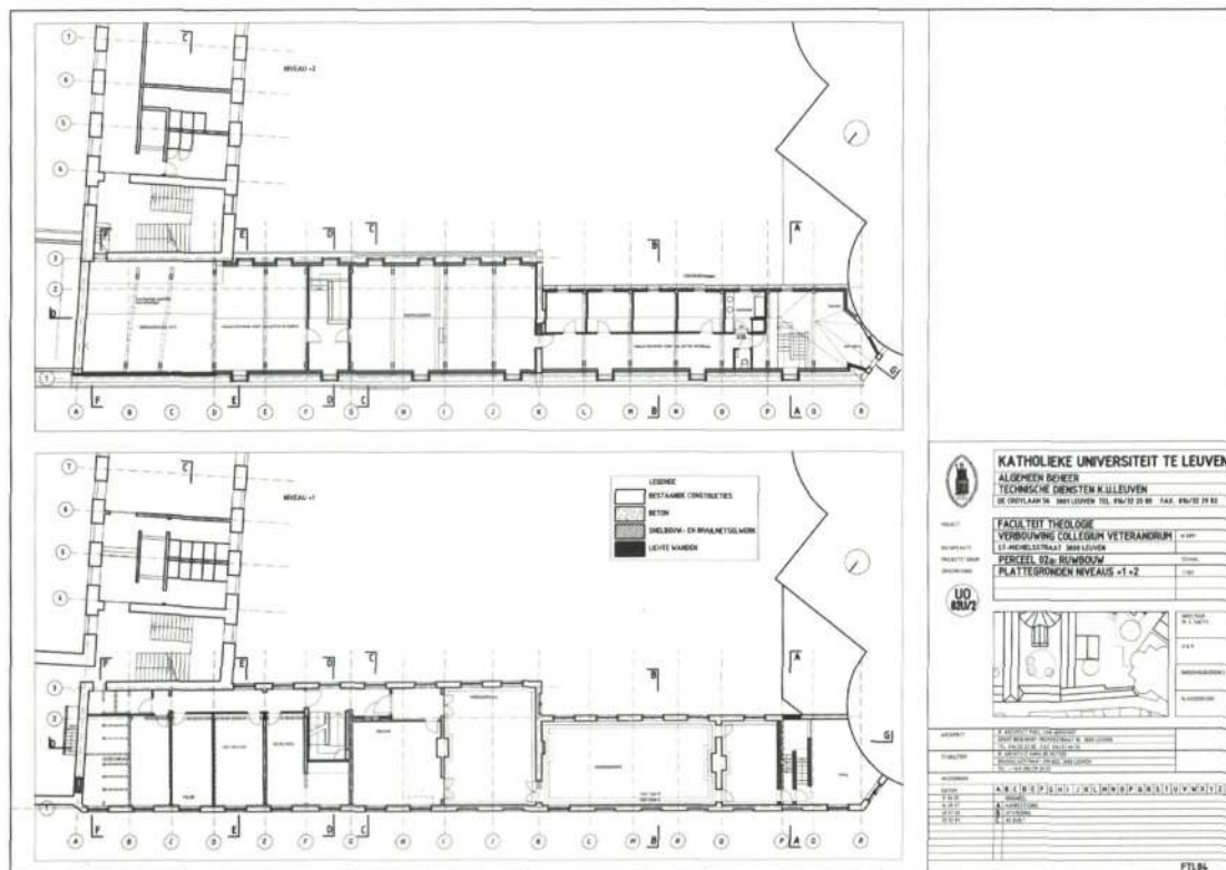
Grondplan der verdiepingen, toestand na de werken (arch. P. Van Aerschot)
