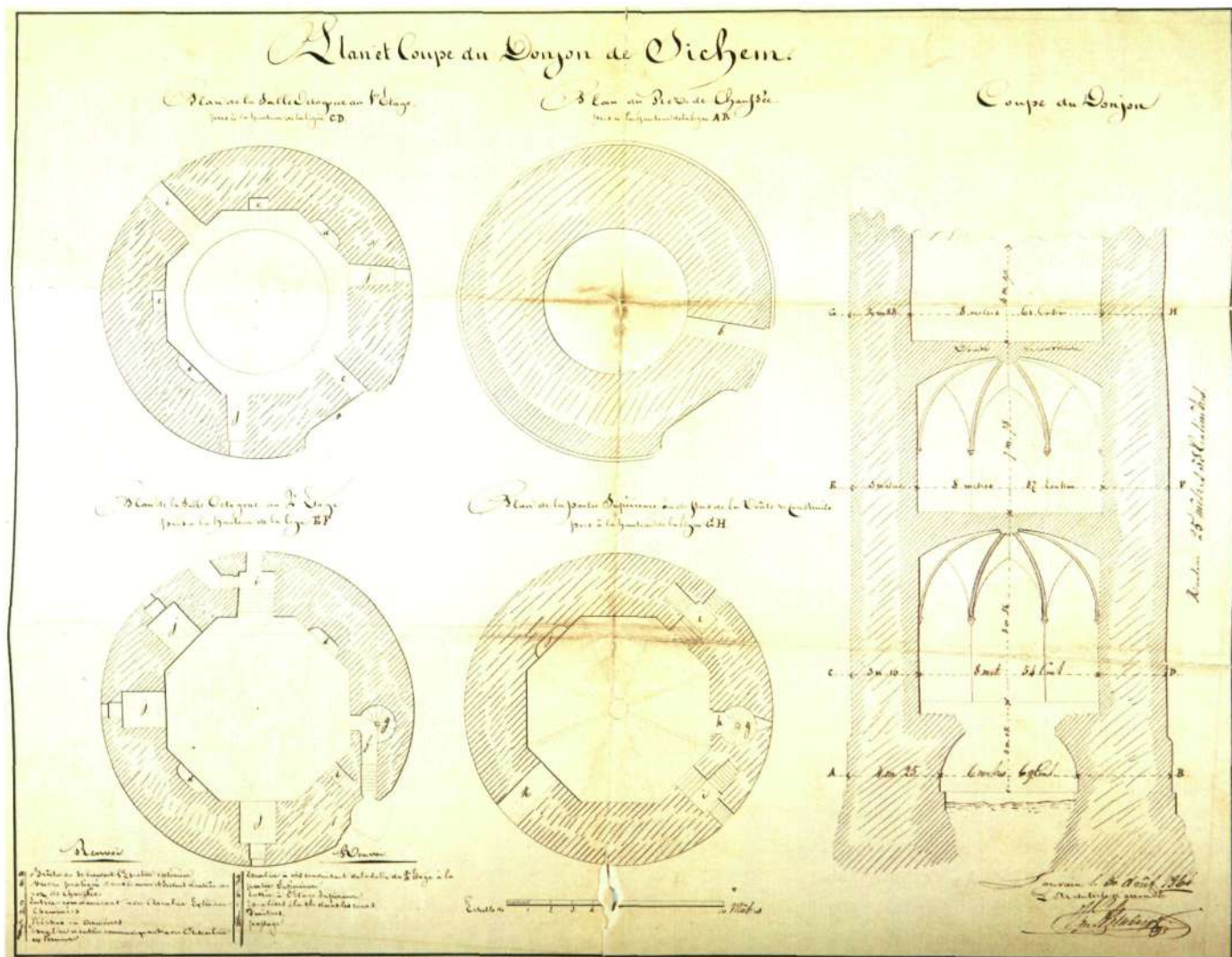
Plan van de Maagdentoren door Alexander Van Arenbergh, 30 augustus 1864. Op de dwarsdoorsnede van de toren zijn de gereconstrueerde gewelven van de tweede verdieping goed te zien ( voûte reconstruite ). De 'muuraanzetten' aan de buitenkant van de toren zijn verdwenen (Archief KCML, dossier Maagdentoren)
