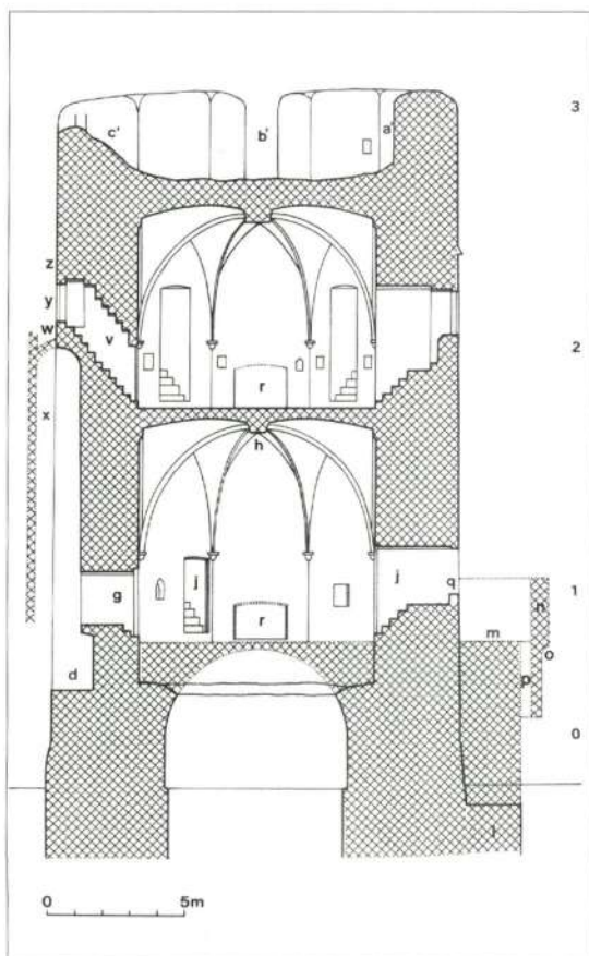
Doorsnede van de toren (uit DOPERE F. en UBREGTS W., 1991, p. 254-255)
