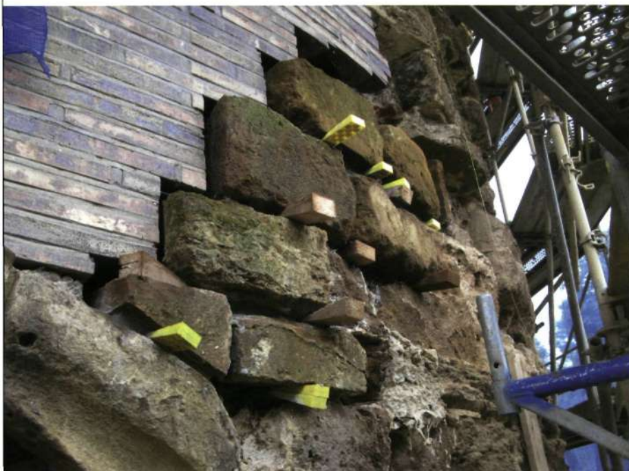
Herstelling met Diestiaan ijzerzandsteen afkomstig van de instorting (foto H. Thibaut)
