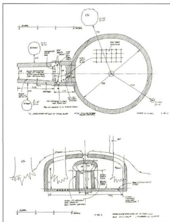
◀ De ijskelder in het Vijverhof (opmeting en tekening J.M. Nolf)
