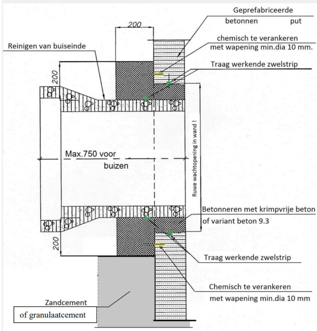
Figuur 7-3-C: aansluiting riolering op toegangs- en verbindingsput met ruwe uitspaaropening
