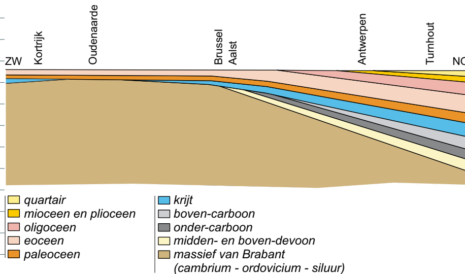
Fig. 14 Geologie van Vlaanderen
