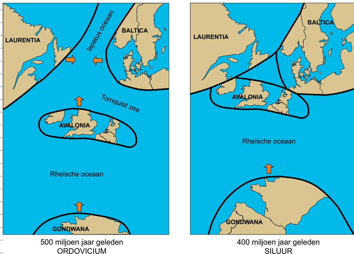
Fig.4 De Caledonische plooingsfase Continentverschuivingen tijdens het Ordovicium en het Siluur
