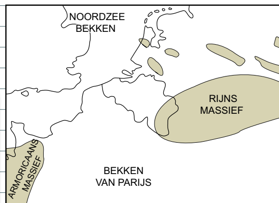
Fig.9 Paleogeografie tijdens het Laat-Krijt
