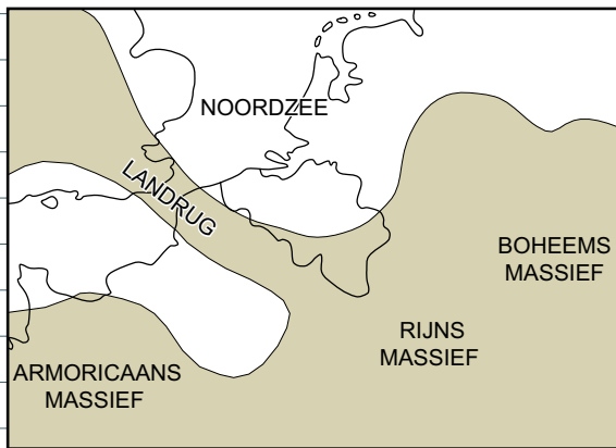
Fig. 11 Paleogeografie tijdens het Midden-Eoceen
