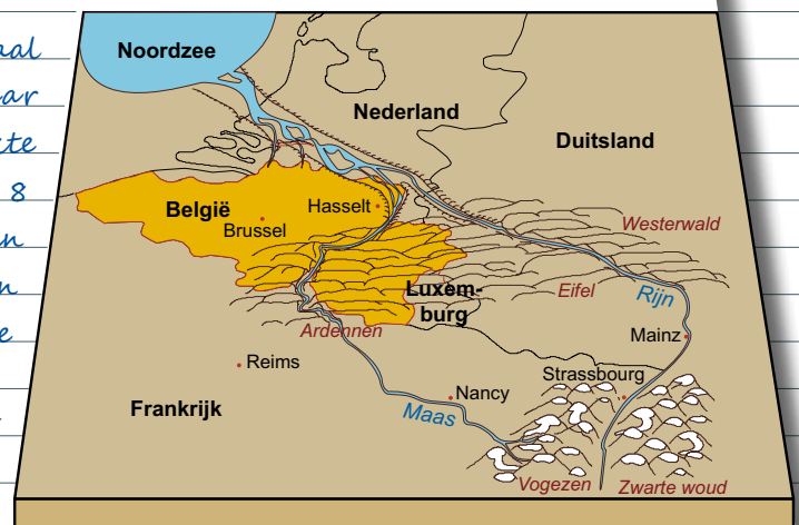
Fig. 15 Maas en Rijn 600.000 jaar geleden
