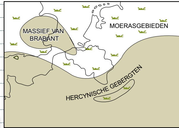
Fig.7 Paleogeografie tijdens het Laat-Carboon
