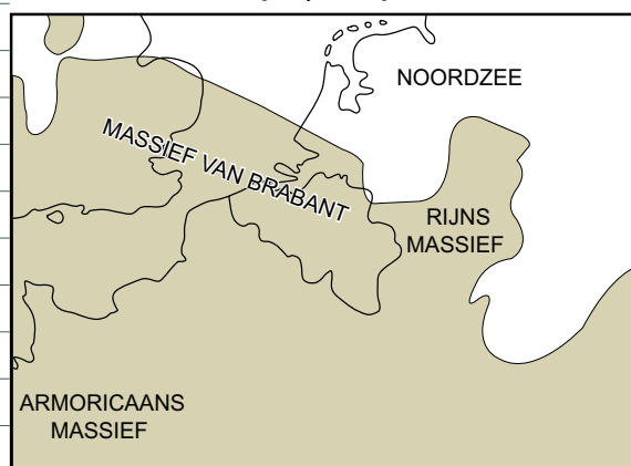
Fig.8 Paleogeografie tijdens het Perm
