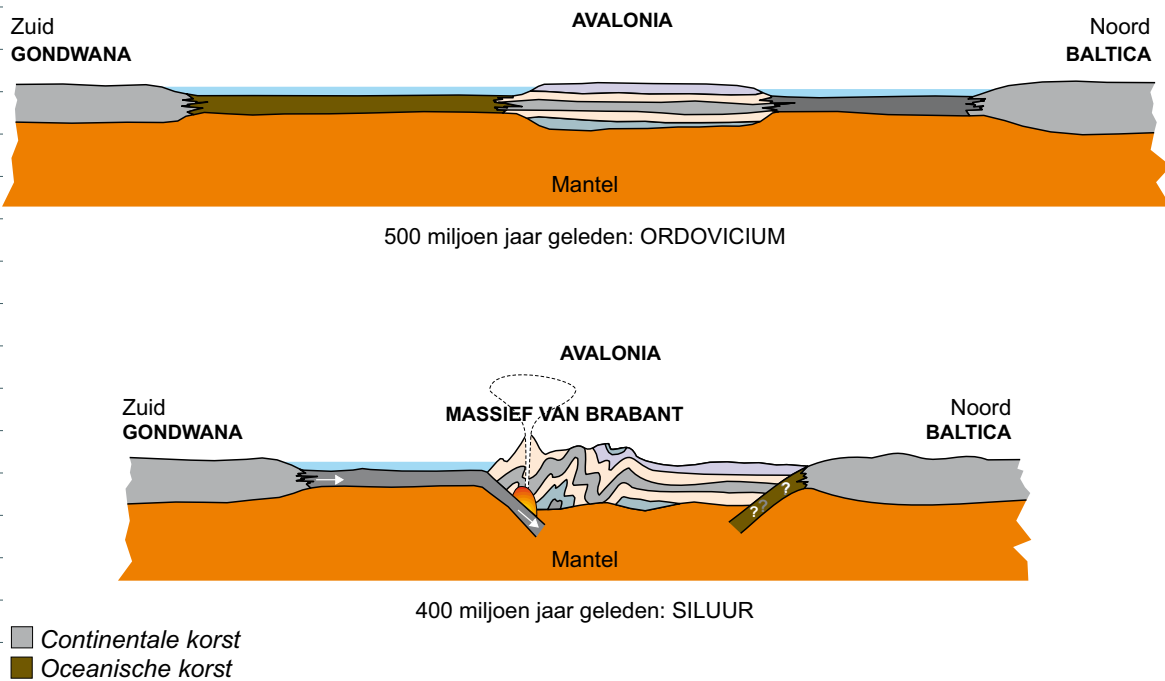
Fig.5 Het massief van Brabant
