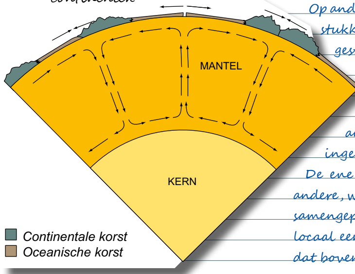
Fig.1 Verschuivingen van de continenten
