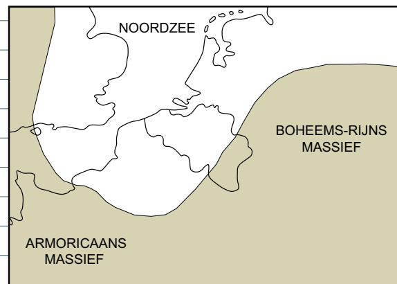
Fig. 10 Paleogeografie tijdens het Vroeg-Eoceen
