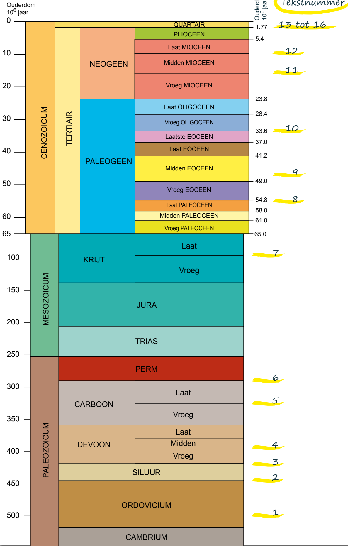
Fig.3 Chronostratigrafie (in miljoenen jaren)
