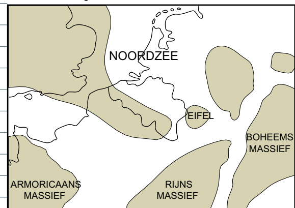
Fig. 12 Paleogeografie tijdens het Vroeg-Oligoceen
