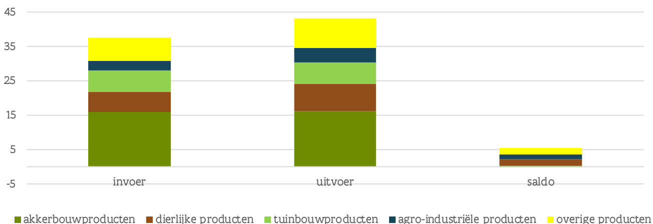
Figuur 2: agrarische invoer, uitvoer en handelssaldo opgesplitst per productgroep, in miljard euro, Vlaanderen, 2021
