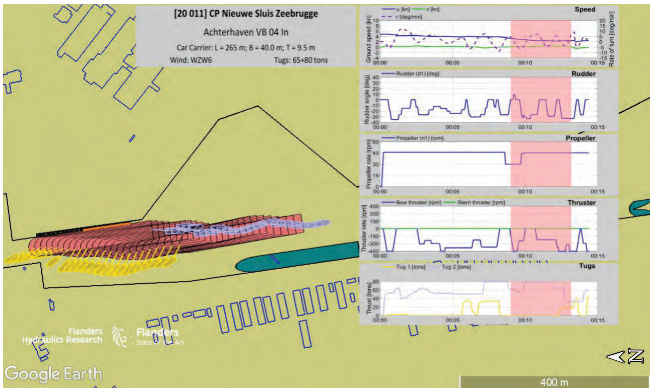
Figuur 15 – Sluiscadering in simulatie VB_04
