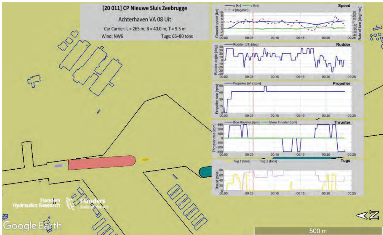
Figuur 13 – Contact tussen achterschip en oostelijke oever voorhaven bij sluisuitvaart in simulatie VA_08
