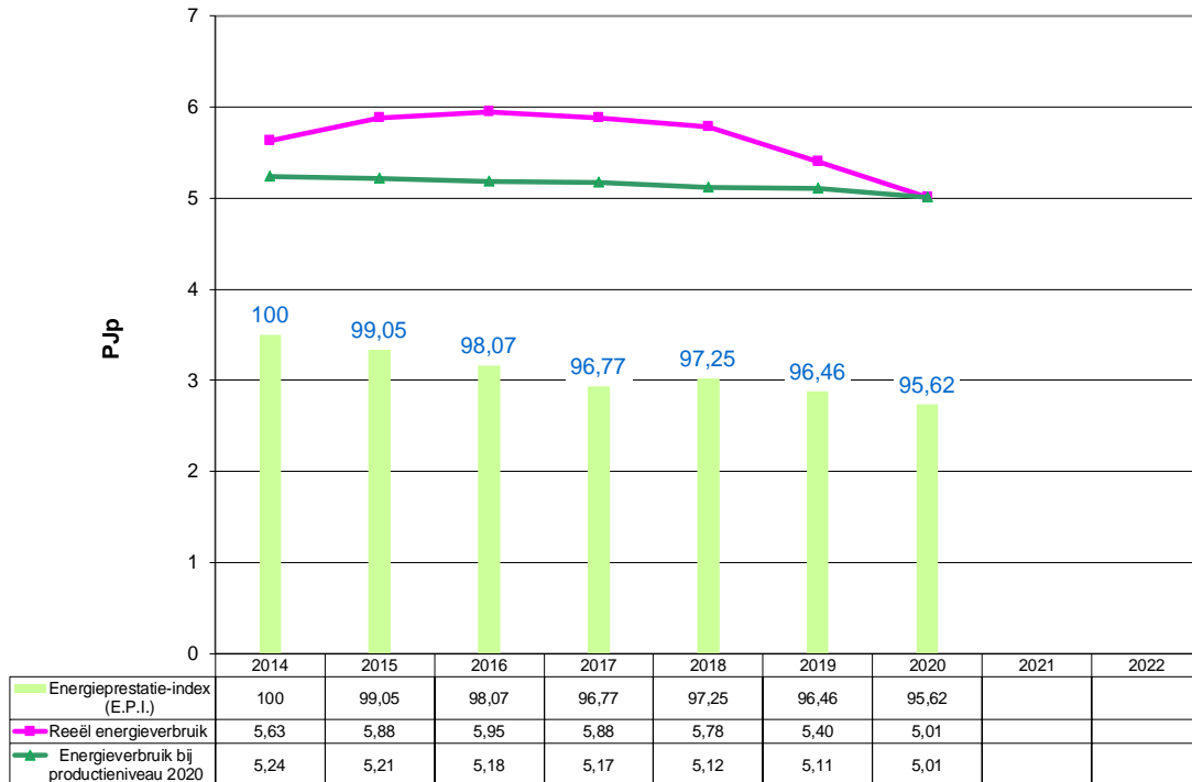
Grafiek 44: Evolutie 2014 – 2020 van het energieverbruik en de E.P.I. voor Textiel & Hout (niet VER-bedrijven)
