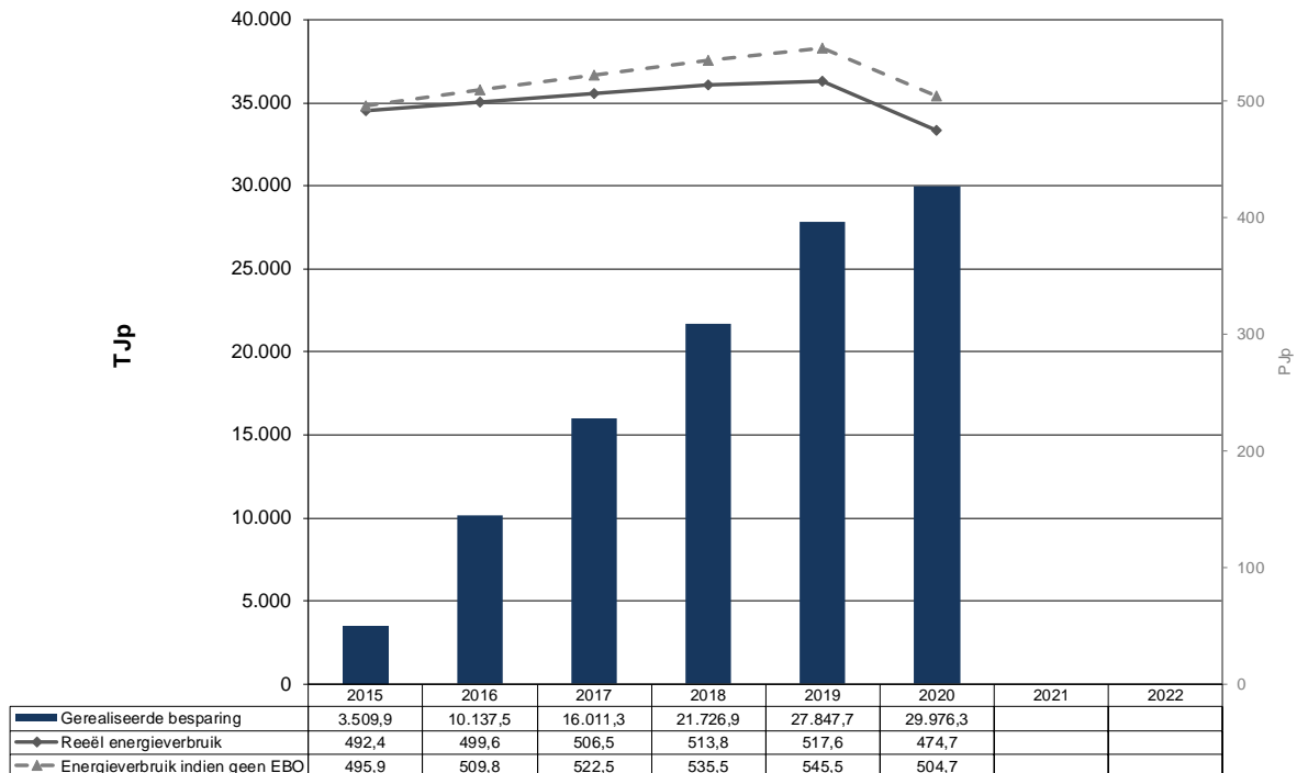
Grafiek 1: Gerealiseerde besparingen (VER en niet VER-bedrijven)
