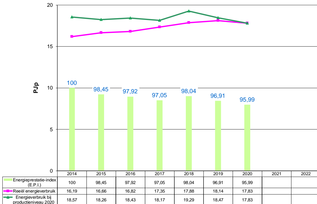
Grafiek 38: Evolutie 2014 – 2020 van het energieverbruik en de E.P.I. voor Voeding & Mengvoeders (niet VER-bedrijven)
