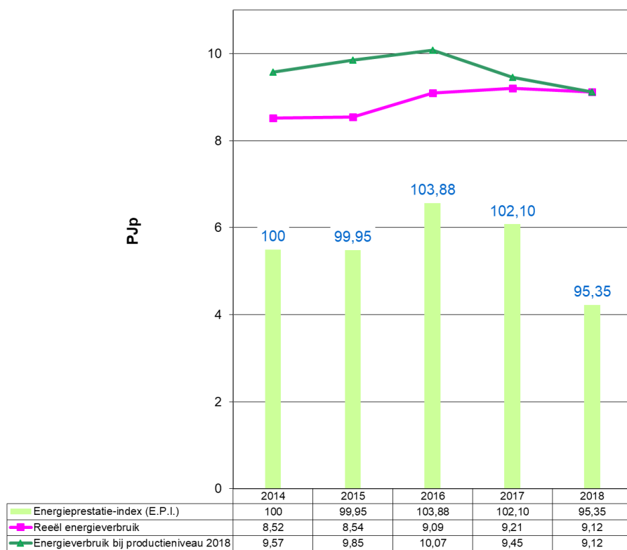
Grafiek 43: Evolutie 2014 – 2018 van het energieverbruik en de E.P.I. voor Textiel & Hout (VER-bedrijven)
