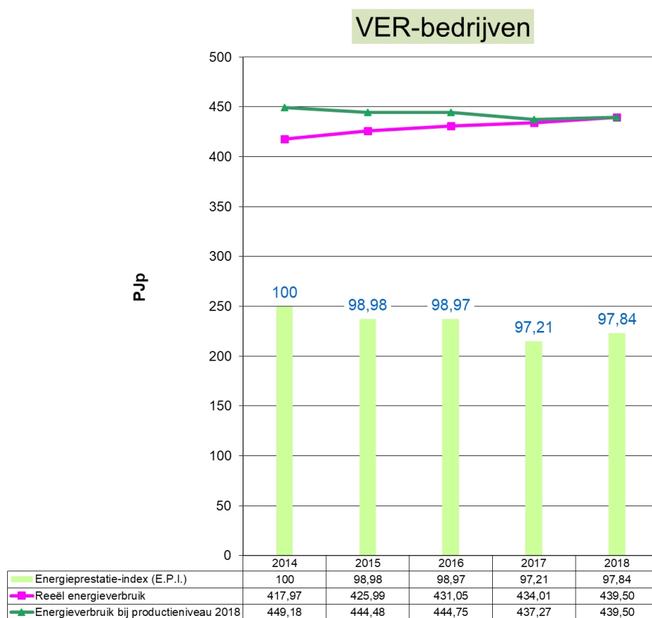
Grafiek 27: Evolutie 2014 – 2018 van het energieverbruik en de E.P.I. voor de VER-bedrijven
