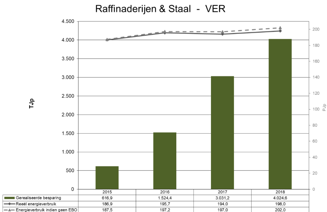
Grafiek 7: Gerealiseerde besparingen Raffinaderijen & Staal (VER-bedrijven)
