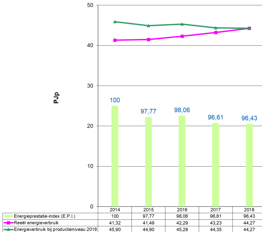
Grafiek 36: Evolutie 2014 – 2018 van het energieverbruik en de E.P.I. voor Voeding & Mengvoeders (VER en niet VER-bedrijven)
