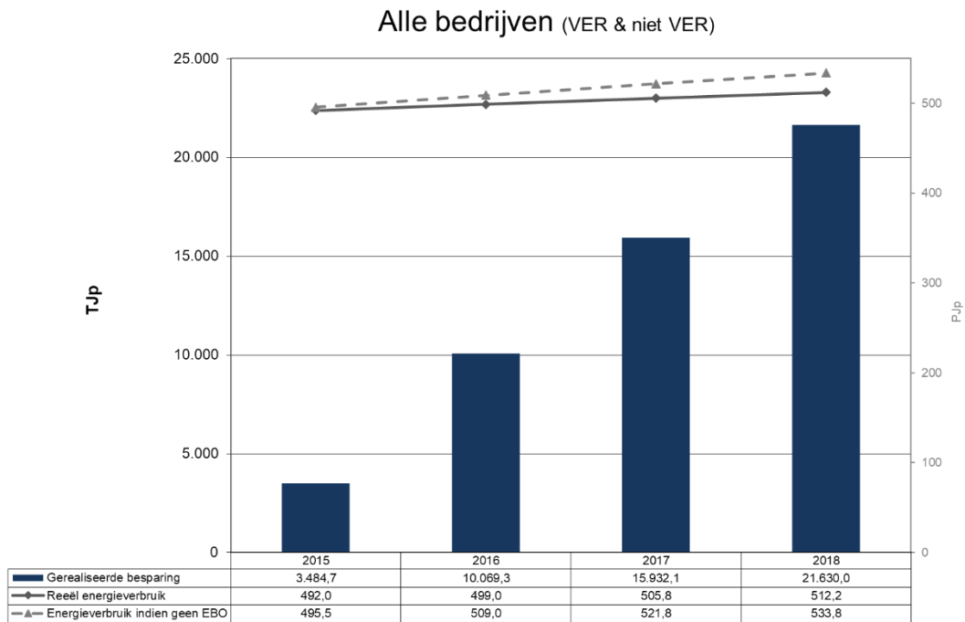
Grafiek 1: Gerealiseerde besparingen (VER en niet VER-bedrijven)
