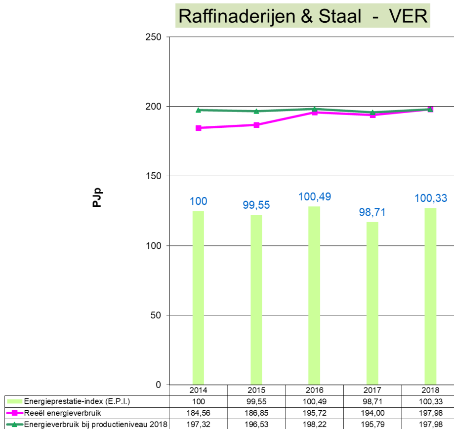
Grafiek 32: Evolutie 2014 – 2018 van het energieverbruik en de E.P.I. voor Raffinaderijen & Staal (VER-bedrijven)
