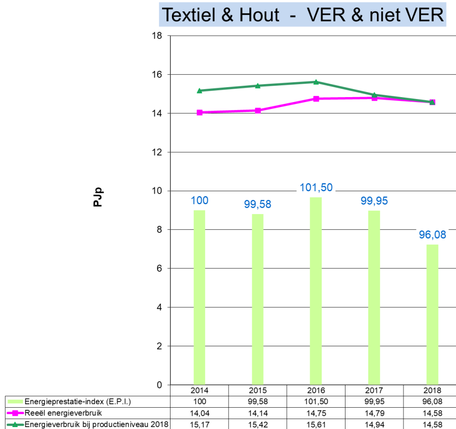
Grafiek 42: Evolutie 2014 – 2018 van het energieverbruik en de E.P.I. voor Textiel & Hout (VER en niet VER-bedrijven)
