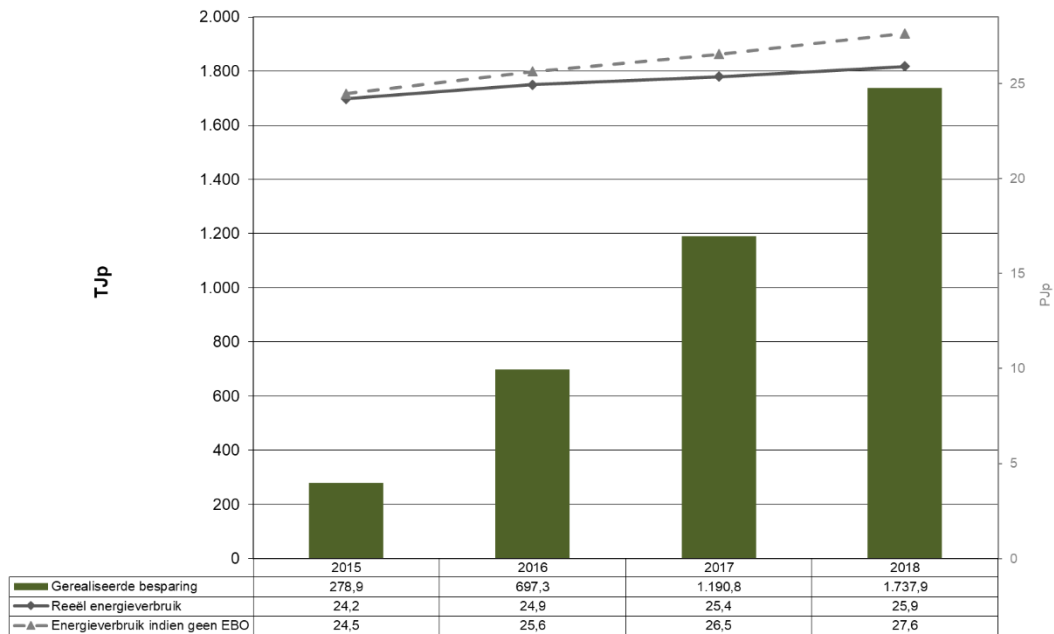
Grafiek 12: Gerealiseerde besparingen Voeding & Mengvoeders (VER-bedrijven)
