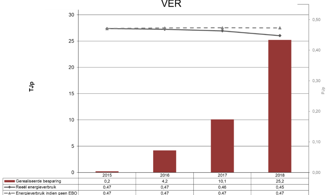
Grafiek 10: Gerealiseerde besparingen Papier, Papier- en kartonverwerking & Drukkerijen (niet VER-bedrijven)
