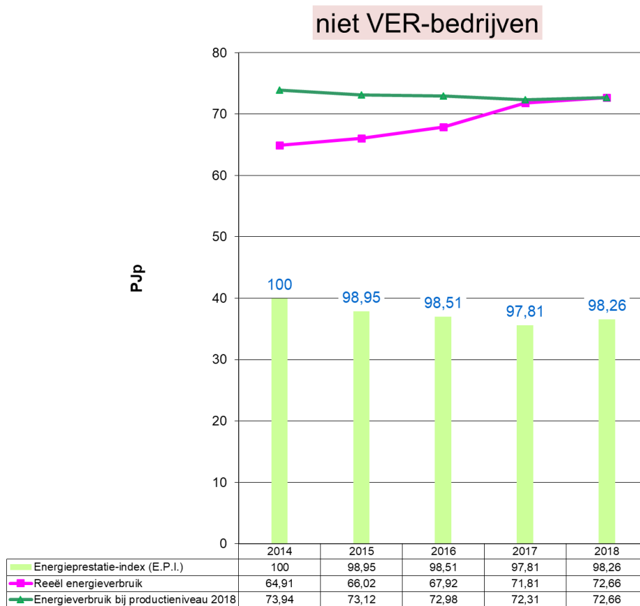
Grafiek 28: Evolutie 2014 – 2018 van het energieverbruik en de E.P.I. voor de niet VER-bedrijven
