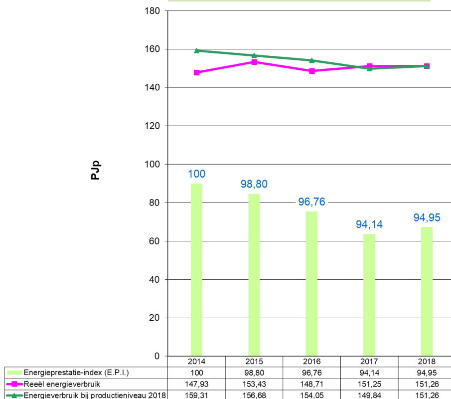
Grafiek 30: Evolutie 2014 – 2018 van het energieverbruik en de E.P.I. voor Chemie & Kunststoffen (VER-bedrijven)
