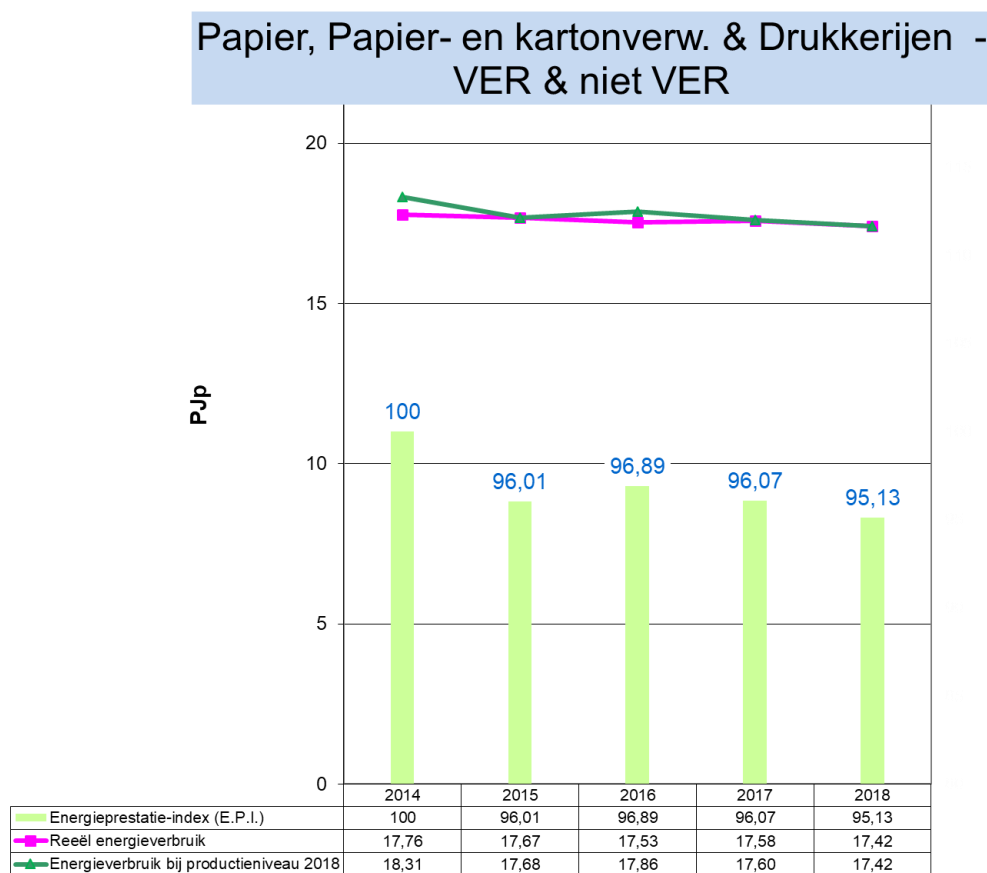
Grafiek 33: Evolutie 2014 – 2018 van het energieverbruik en de E.P.I. voor Papier, Papier- en kartonverwerking & Drukkerijen (VER en niet VER-bedrijven)
