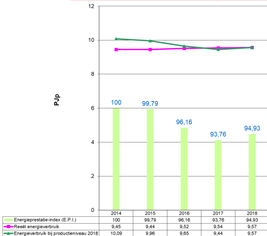
Grafiek 41: Evolutie 2014 – 2018 van het energieverbruik en de E.P.I. voor Non-ferro & Metaalverwerking (niet VER-bedrijven)
