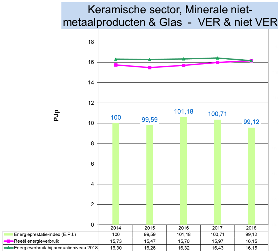
Grafiek 45: Evolutie 2014 – 2018 van het energieverbruik en de E.P.I. voor Keramische sector, Minerale niet-metaalproducten & Glas (VER en niet VER-bedrijven)
