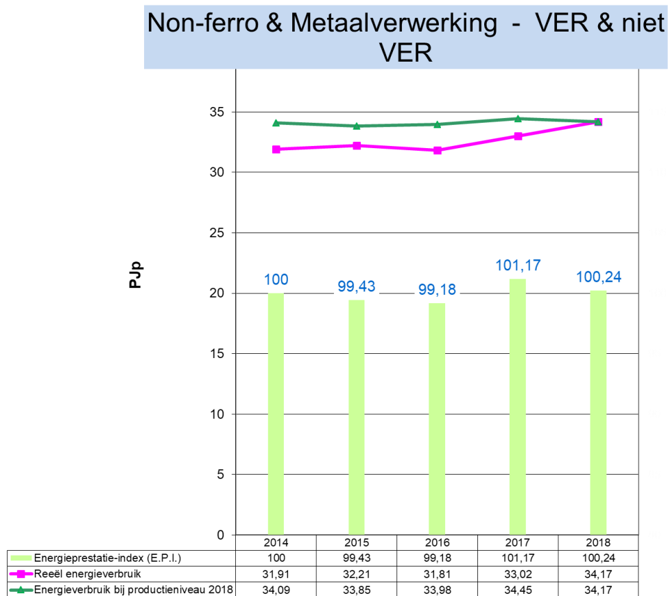
Grafiek 39: Evolutie 2014 – 2018 van het energieverbruik en de E.P.I. voor Non-ferro & Metaalverwerking (VER en niet VER-bedrijven)
