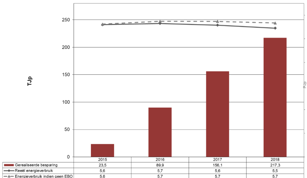
Grafiek 19: Gerealiseerde besparingen Textiel & Hout (VER en niet VER-bedrijven)
