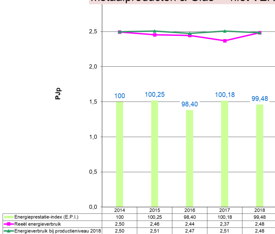
Grafiek 47: Evolutie 2014 – 2018 van het energieverbruik en de E.P.I. voor Keramische sector, Minerale niet-metaalproducten & Glas (niet VER-bedrijven)
