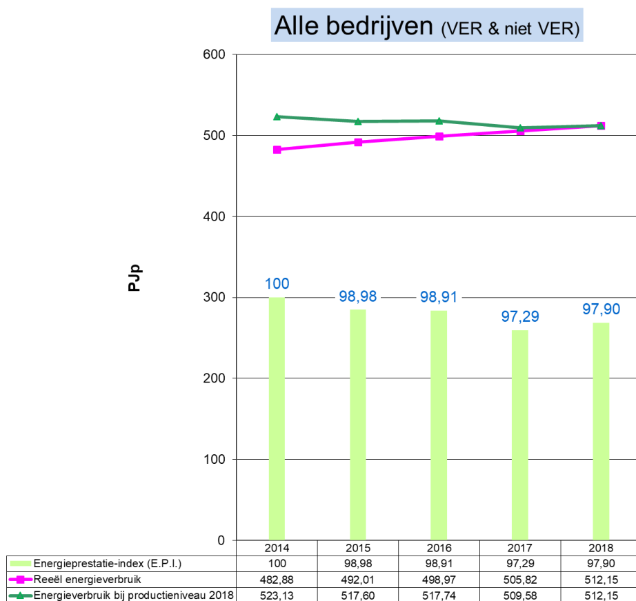
Grafiek 26: Evolutie 2014 – 2018 van het energieverbruik en de E.P.I. voor alle bedrijven
