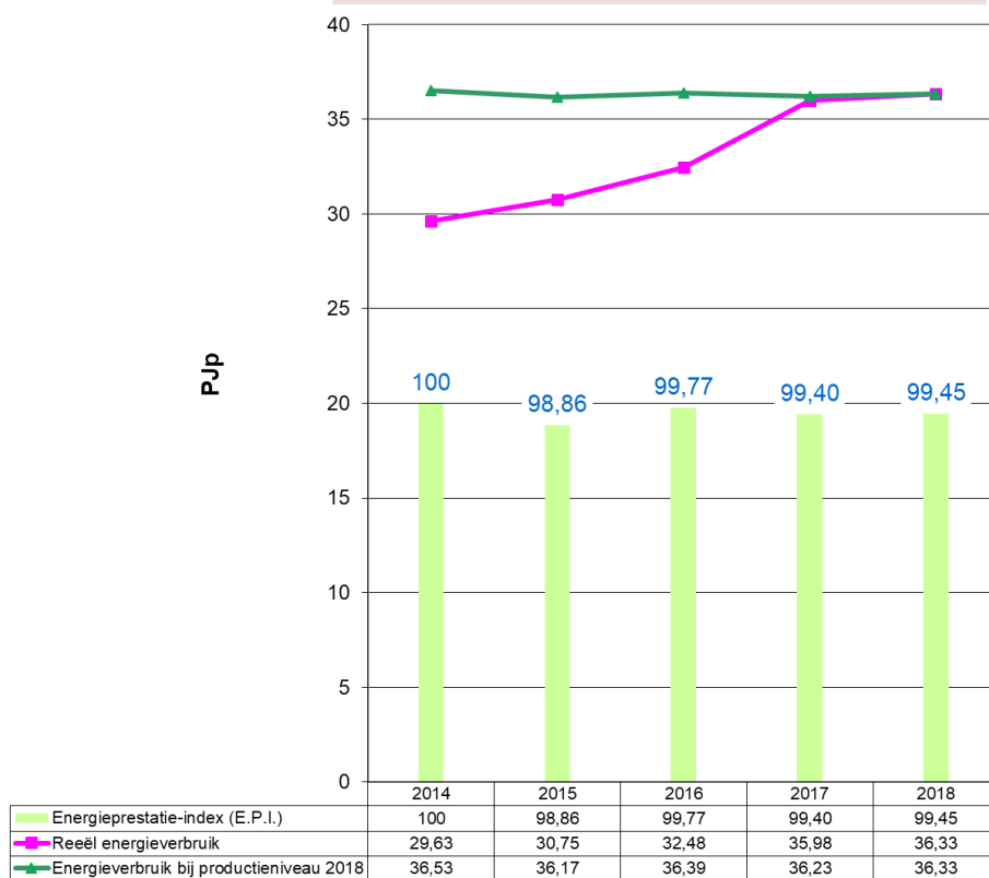
Grafiek 31: Evolutie 2014 – 2018 van het energieverbruik en de E.P.I. voor Chemie & Kunststoffen (niet VER-bedrijven)
