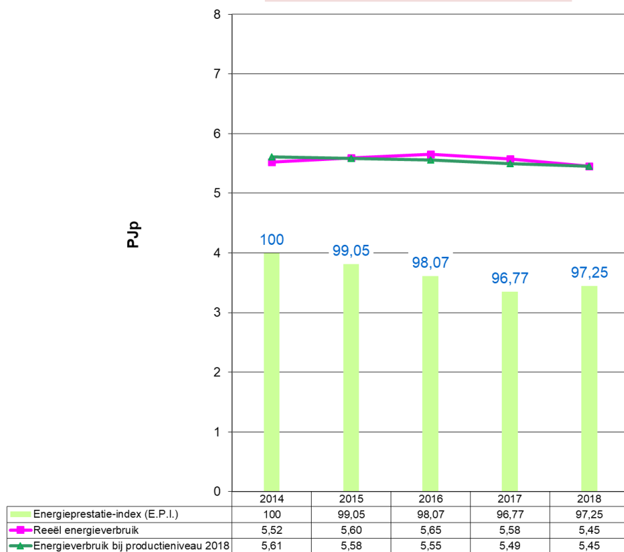
Grafiek 44: Evolutie 2014 – 2018 van het energieverbruik en de E.P.I. voor Textiel & Hout (niet VER-bedrijven)
