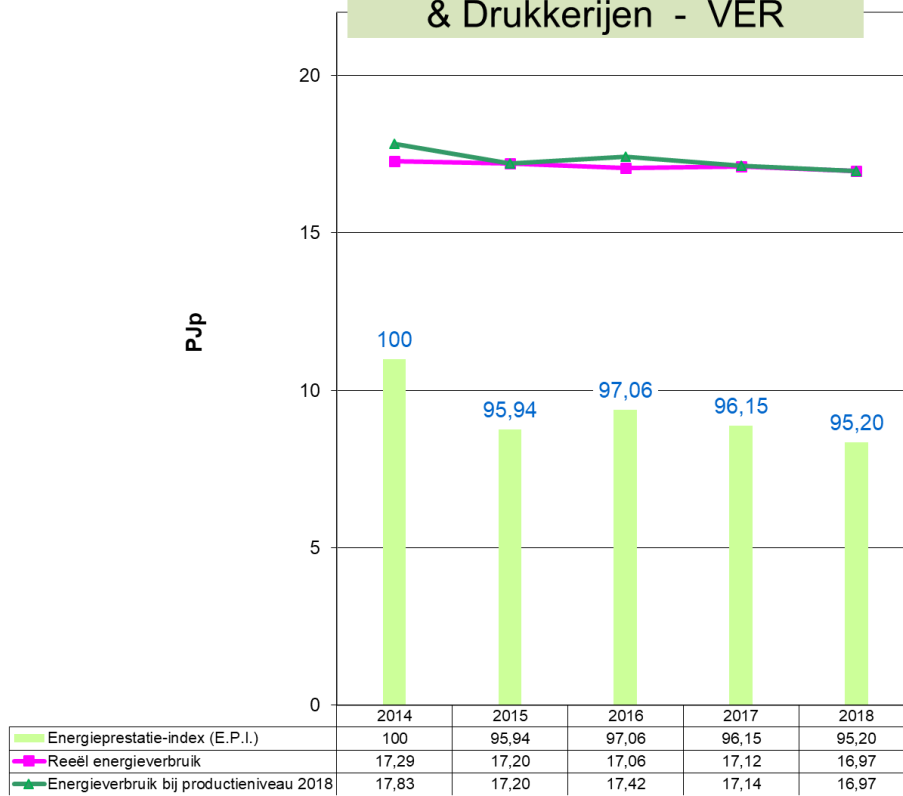
Grafiek 34: Evolutie 2014 – 2018 van het energieverbruik en de E.P.I. voor Papier, Papier- en kartonverwerking & Drukkerijen (VER-bedrijven)
