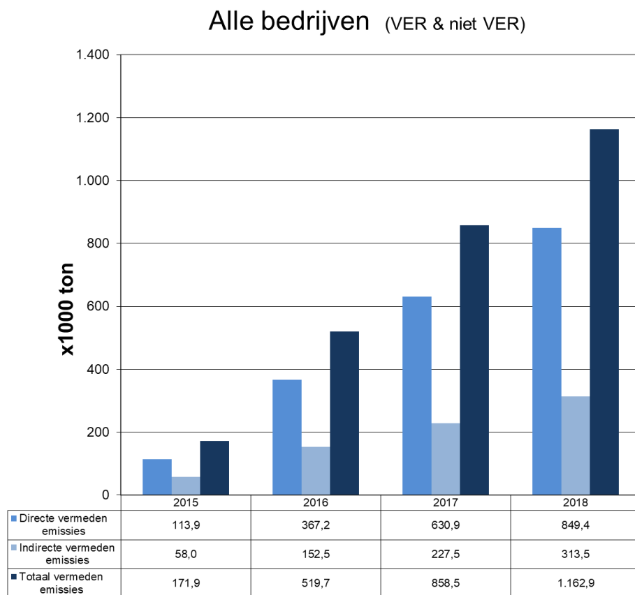
Grafiek 23: Vermeden CO 2 -emissies (VER en niet VER-bedrijven)
