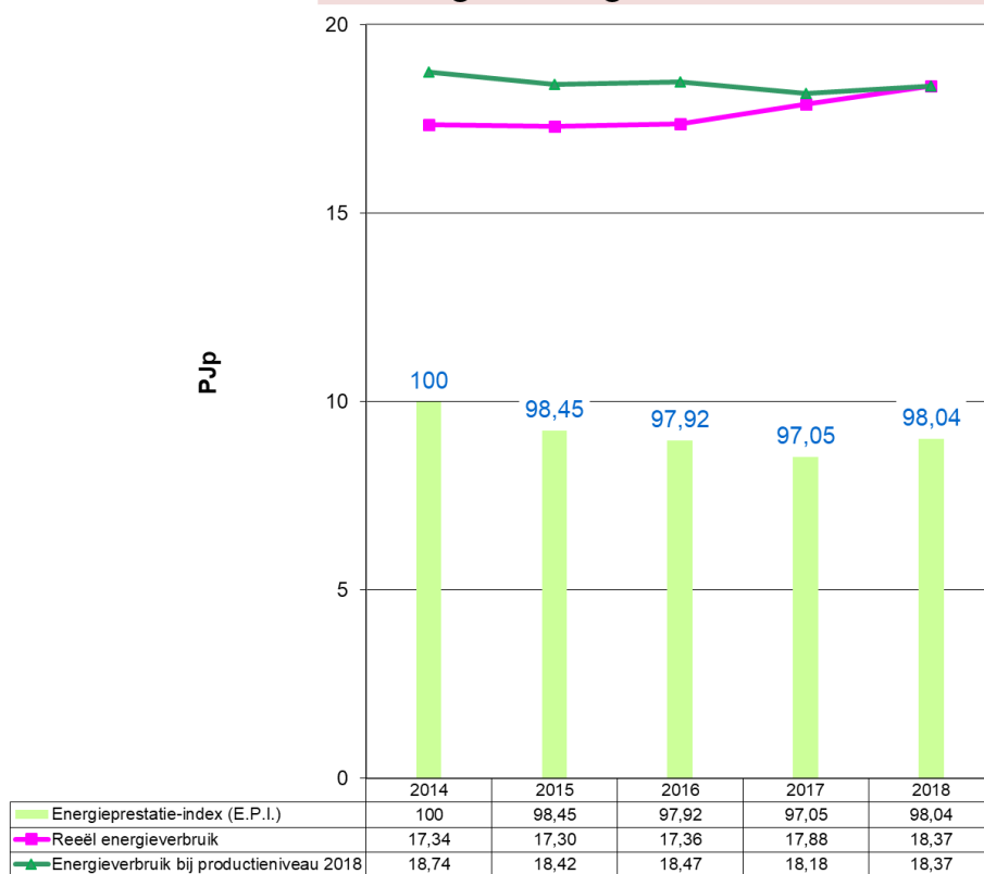
Grafiek 38: Evolutie 2014 – 2018 van het energieverbruik en de E.P.I. voor Voeding & Mengvoeders (niet VER-bedrijven)
