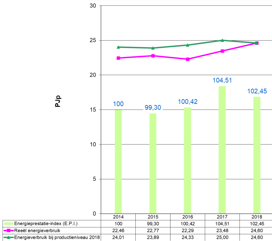
Grafiek 40: Evolutie 2014 – 2018 van het energieverbruik en de E.P.I. voor Non-ferro & Metaalverwerking (VER-bedrijven)
