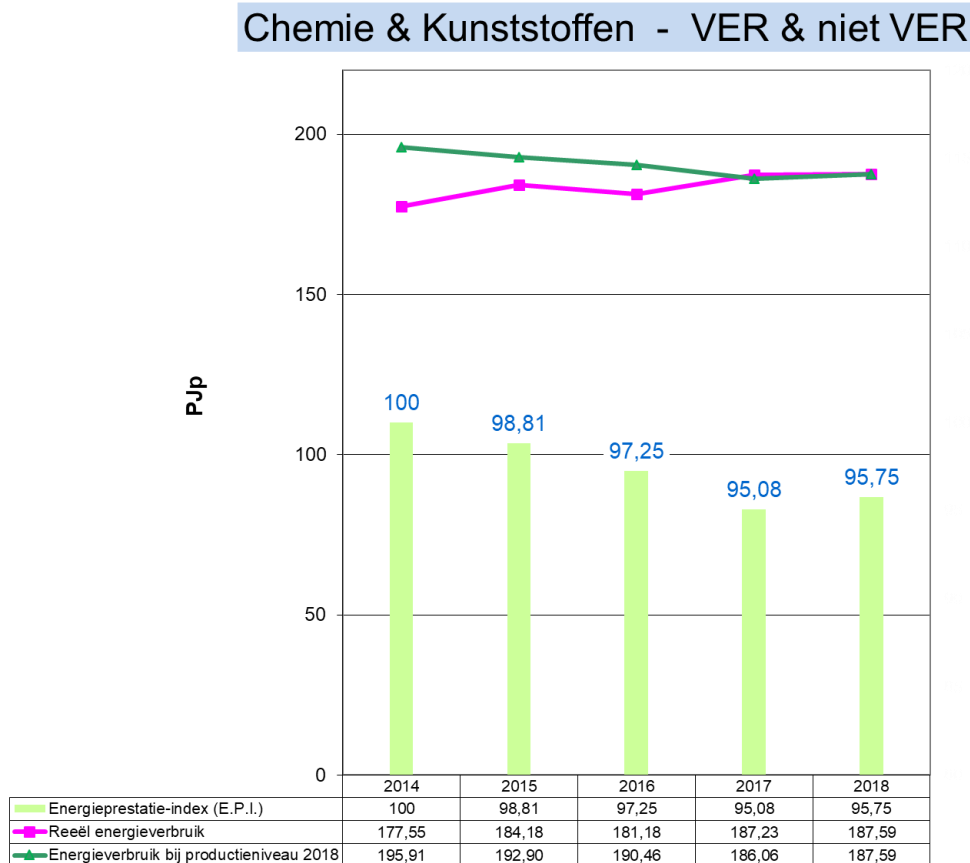
Grafiek 29: Evolutie 2014 – 2018 van het energieverbruik en de E.P.I. voor Chemie & Kunststoffen (VER en niet VER-bedrijven)
