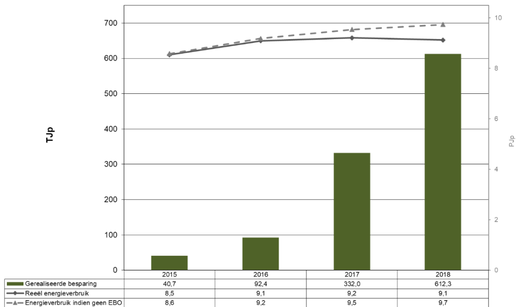
Grafiek 18: Gerealiseerde besparingen Textiel & Hout (VER en niet VER-bedrijven)
