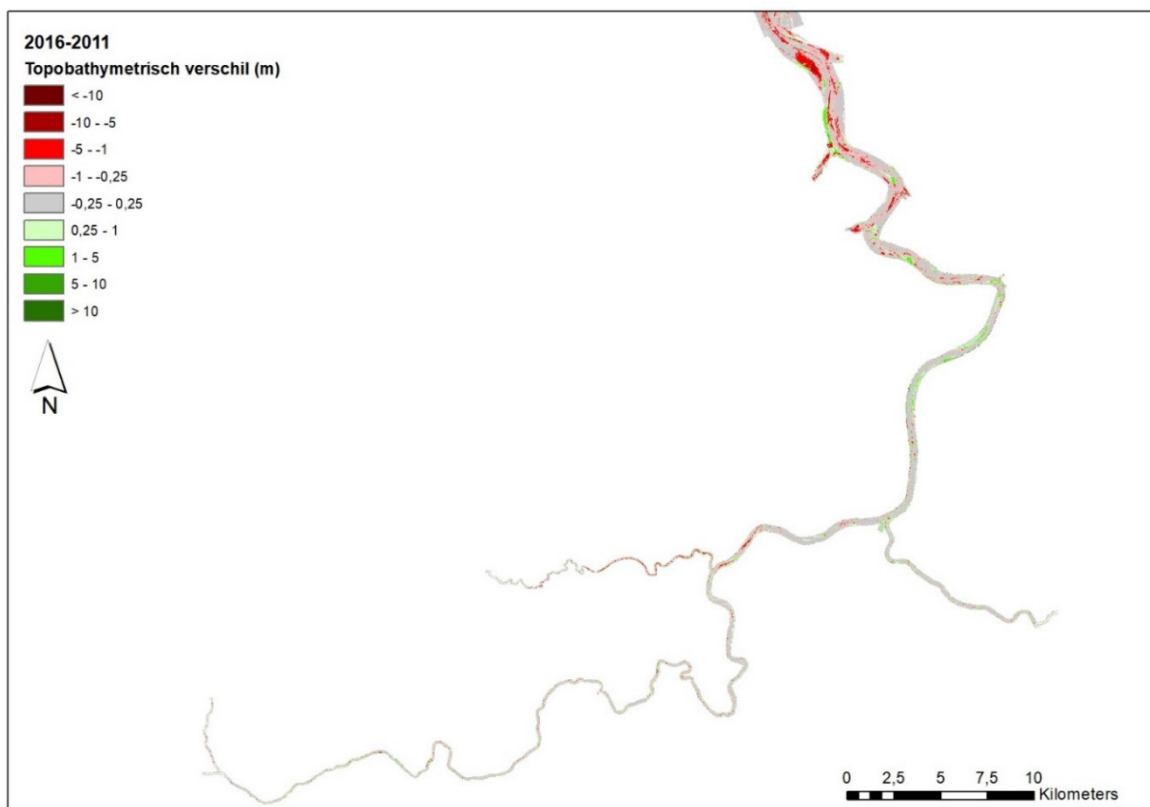
Figuur 11 – Verschilkaart op basis van de bathymetrieën van 2016 en 2011.
