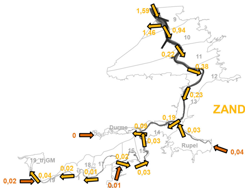
Figuur 16 – Schematische voorstelling van het zandtransport [MTDS/jaar] over de periode 2011-2016 (referentiescenario)
