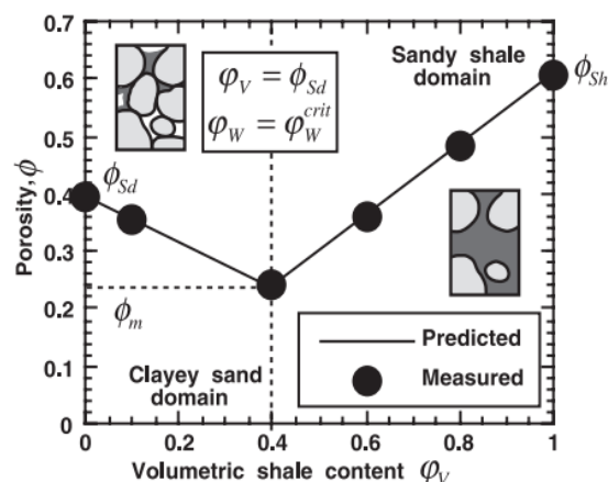
Figuur 6 – "Ideal packing model": voorspelde porositeit als een functie van het volumetrisch slibpercentage. Een porositeitsminimum treedt op wanneer het volumetrisch slibpercentage gelijk is aan de porositeit van de zandcomponent (Koltermann et al., 1995).
