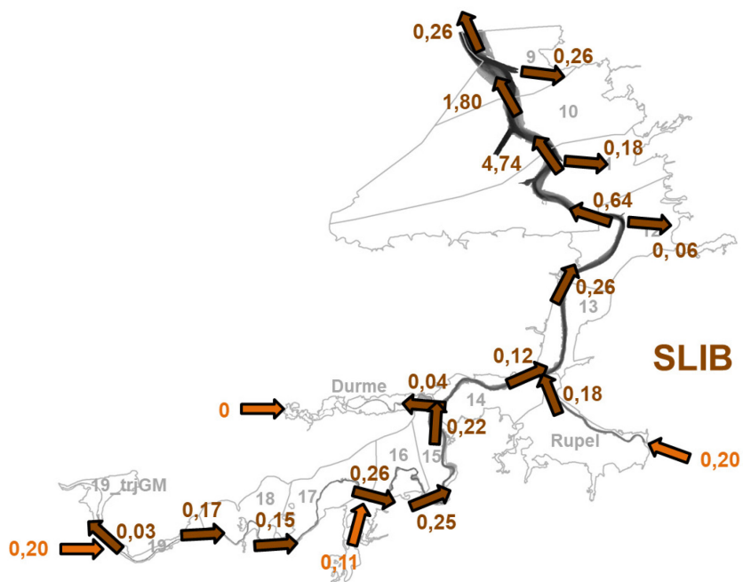
Figuur 17 – Schematische voorstelling van het slibtransport [MTDS/jaar] over de periode 2011-2016 (referentiescenario).
