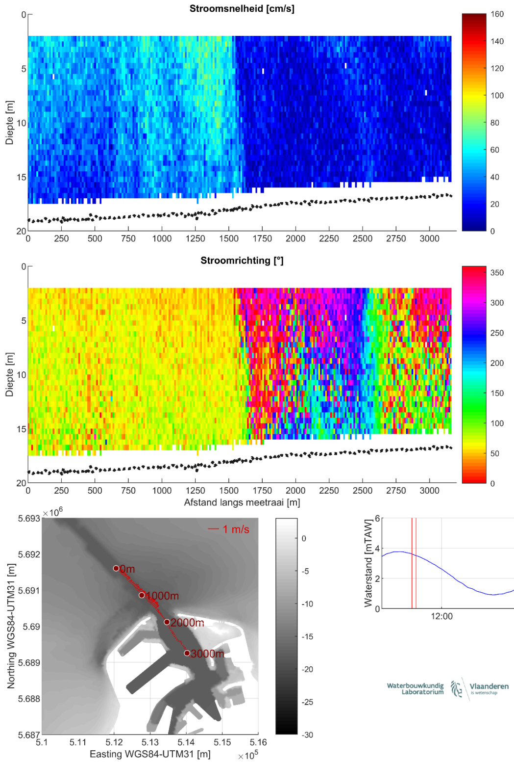
Figuur 11 – Stroomgegevens 10/08/2023 raai 6: snelheids grootte (top), -richting (midden) en diepte-gemiddelde vectoren (onder)
