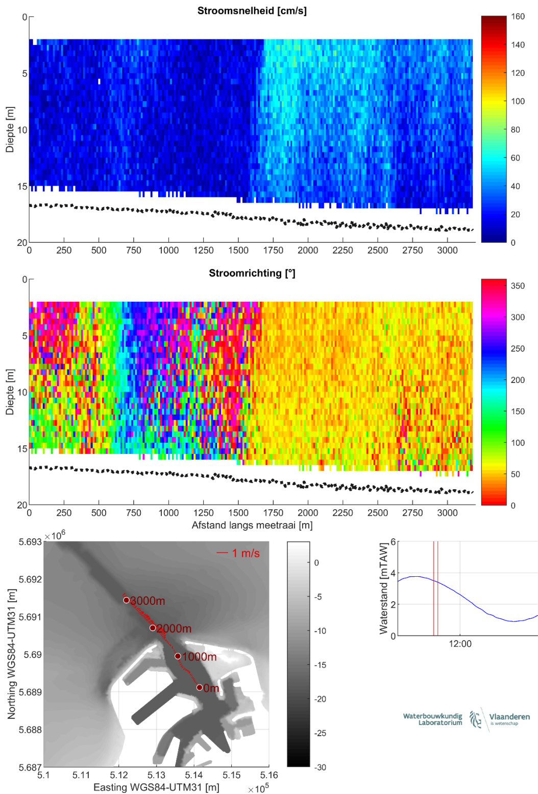
Figuur 12 – Stroomgegevens 10/08/2023 raai 7: snelheids grootte (top), -richting (midden) en diepte-gemiddelde vectoren (onder)
