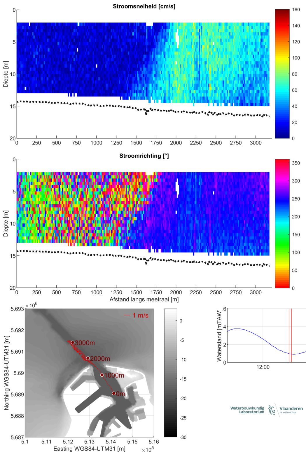
Figuur 28 – Stroomgegevens 10/08/2023 raai 23: snelheids grootte (top), -richting (midden) en diepte-gemiddelde vectoren (onder)
