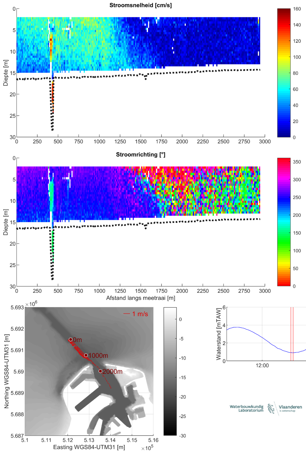
Figuur 29 – Stroomgegevens 10/08/2023 raai 24: snelheids grootte (top), -richting (midden) en diepte-gemiddelde vectoren (onder)
