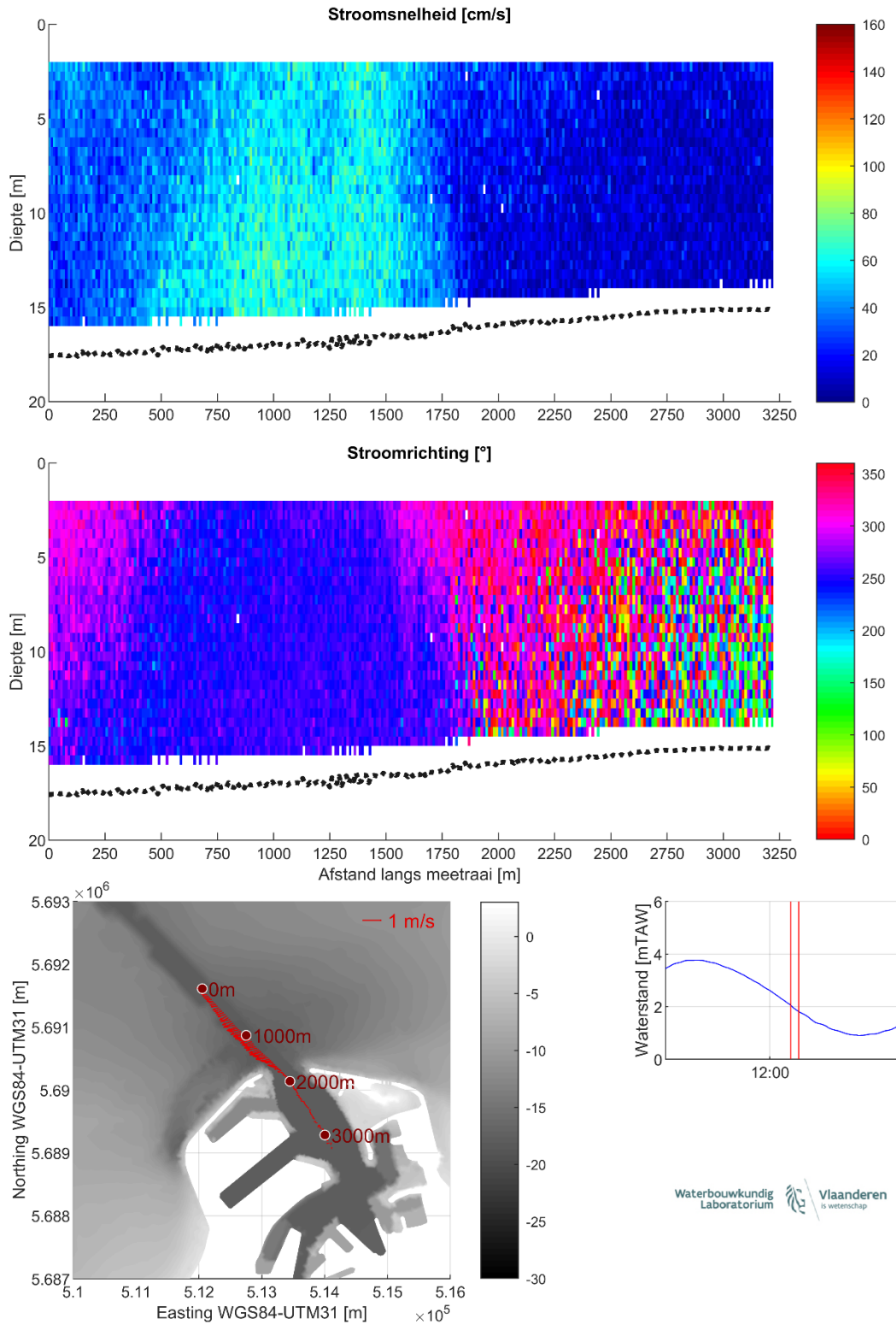
Figuur 21 – Stroomgegevens 10/08/2023 raai 16: snelheids grootte (top), -richting (midden) en diepte-gemiddelde vectoren (onder)
