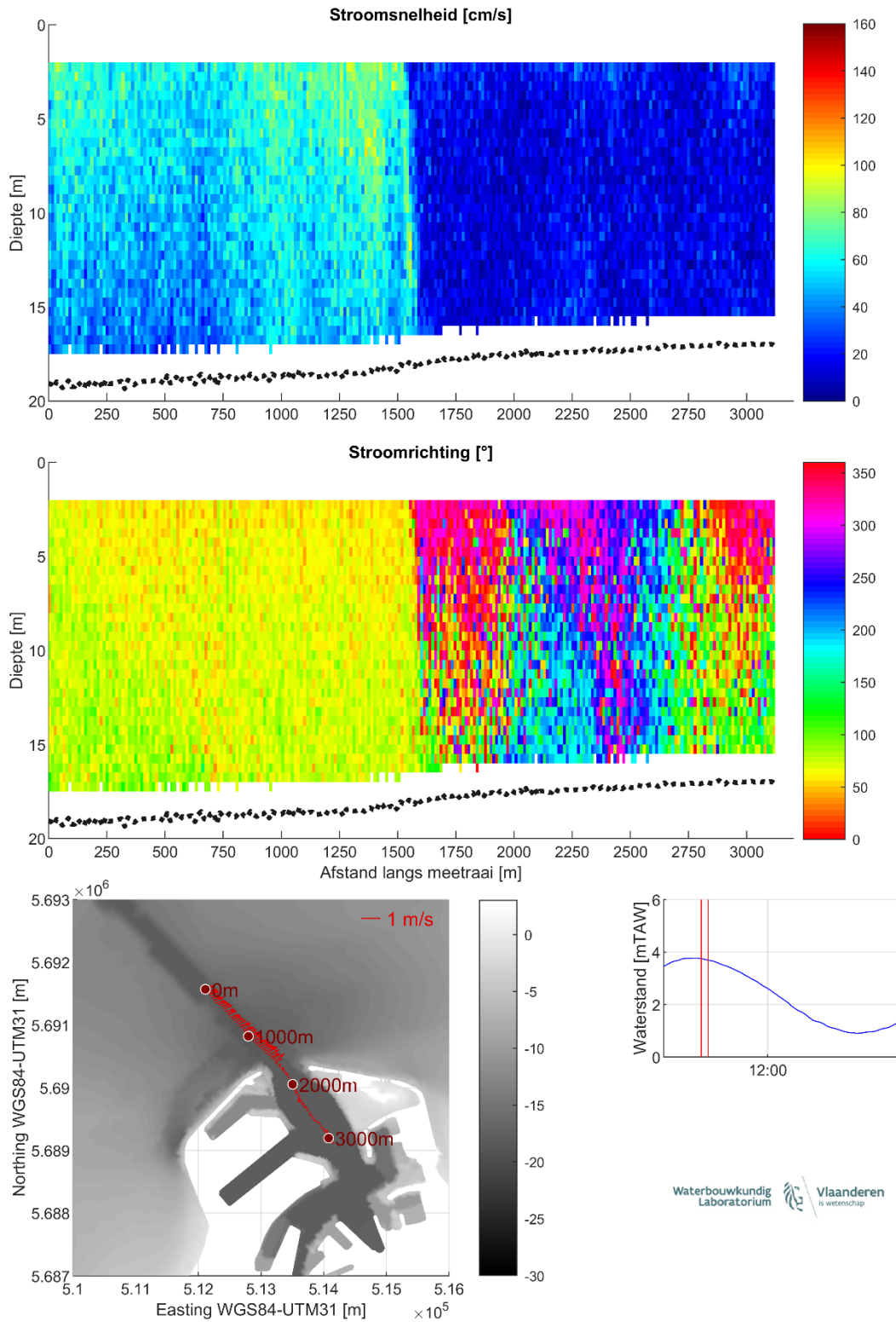
Figuur 9 – Stroomgegevens 10/08/2023 raai 4: snelheidsgrootte (top), -richting (midden) en diepte-gemiddelde vectoren (onder)
