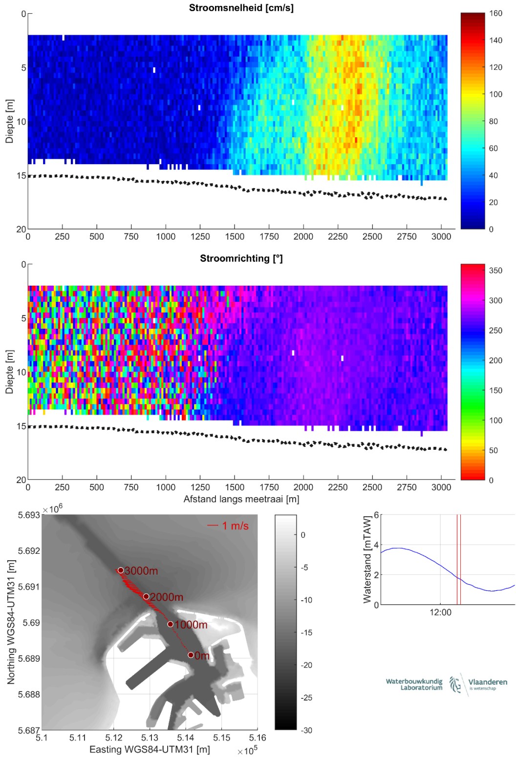
Figuur 22 – Stroomgegevens 10/08/2023 raai 17: snelheids grootte (top), -richting (midden) en diepte-gemiddelde vectoren (onder)
