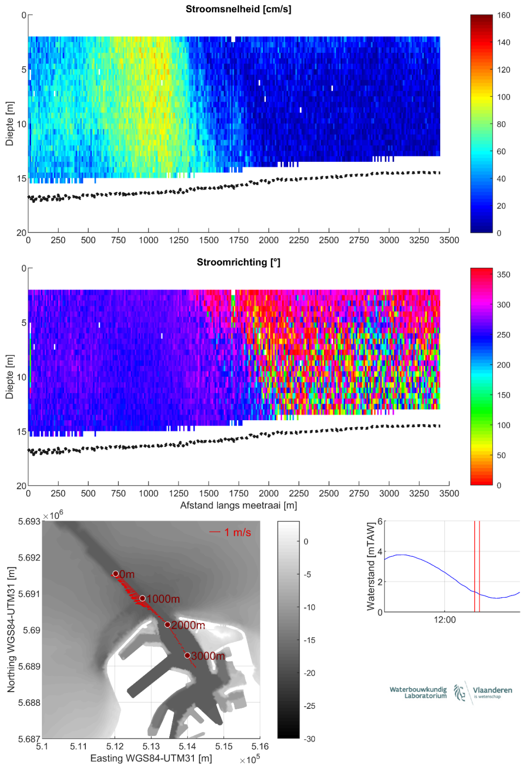
Figuur 25 – Stroomgegevens 10/08/2023 raai 20: snelheids grootte (top), -richting (midden) en diepte-gemiddelde vectoren (onder)
