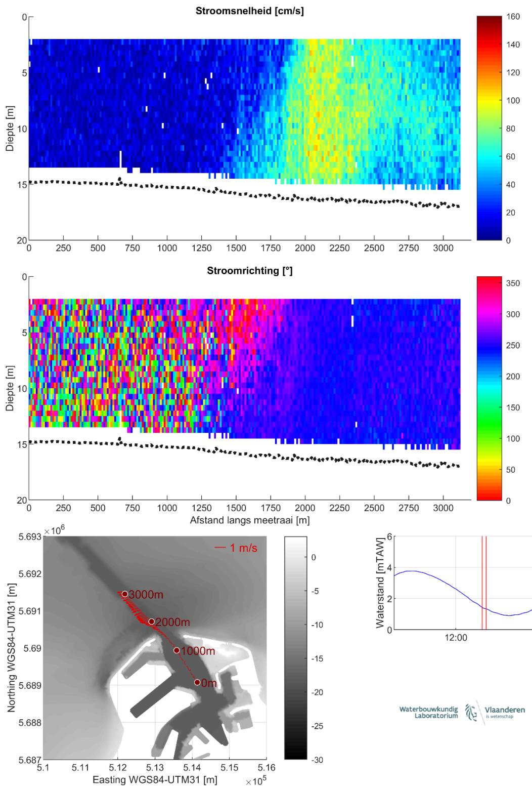
Figuur 24 – Stroomgegevens 10/08/2023 raai 19: snelheids grootte (top), -richting (midden) en diepte-gemiddelde vectoren (onder)
