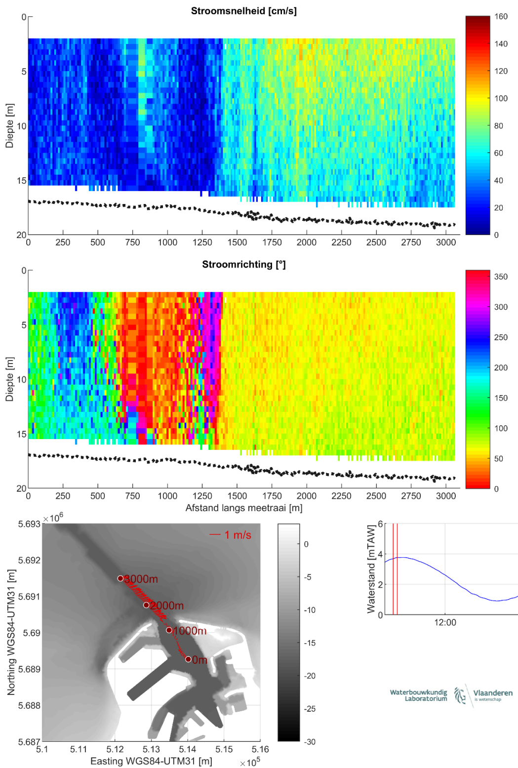
Figuur 6 – Stroomgegevens 10/08/2023 raai 1: snelheids grootte (top), -richting (midden) en diepte-gemiddelde vectoren (onder)
