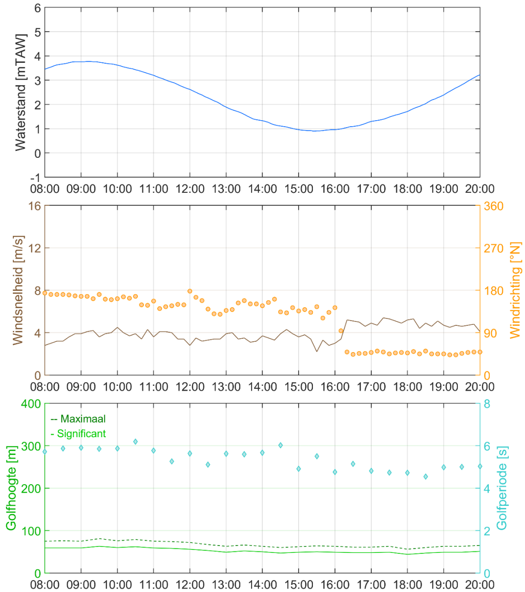
Figuur 5 – Verloop van de omgevingscondities tijdens meetcampagne
