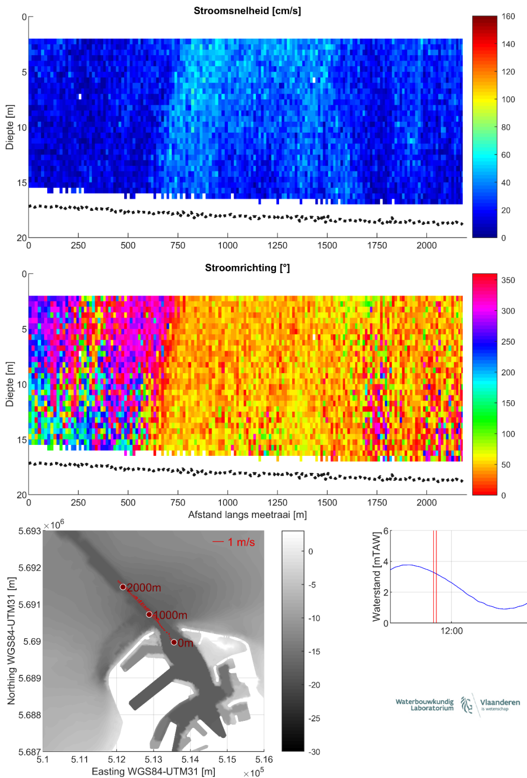
Figuur 14 – Stroomgegevens 10/08/2023 raai 9: snelheids grootte (top), -richting (midden) en diepte-gemiddelde vectoren (onder)
