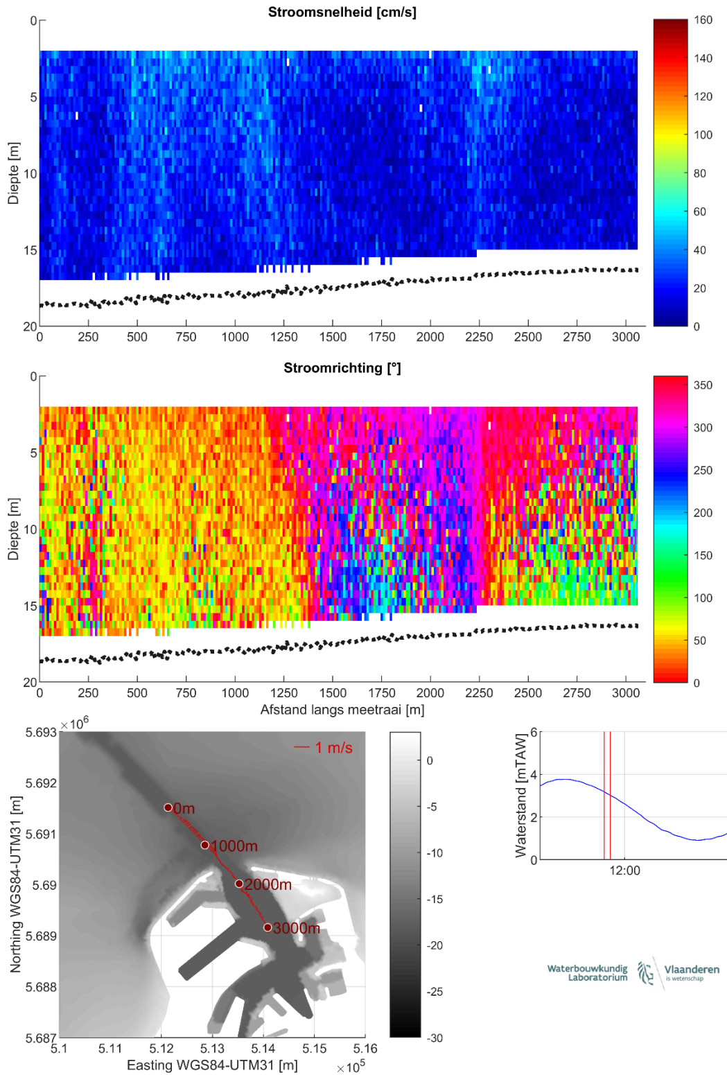
Figuur 15 – Stroomgegevens 10/08/2023 raai 10: snelheids grootte (top), -richting (midden) en diepte-gemiddelde vectoren (onder)
