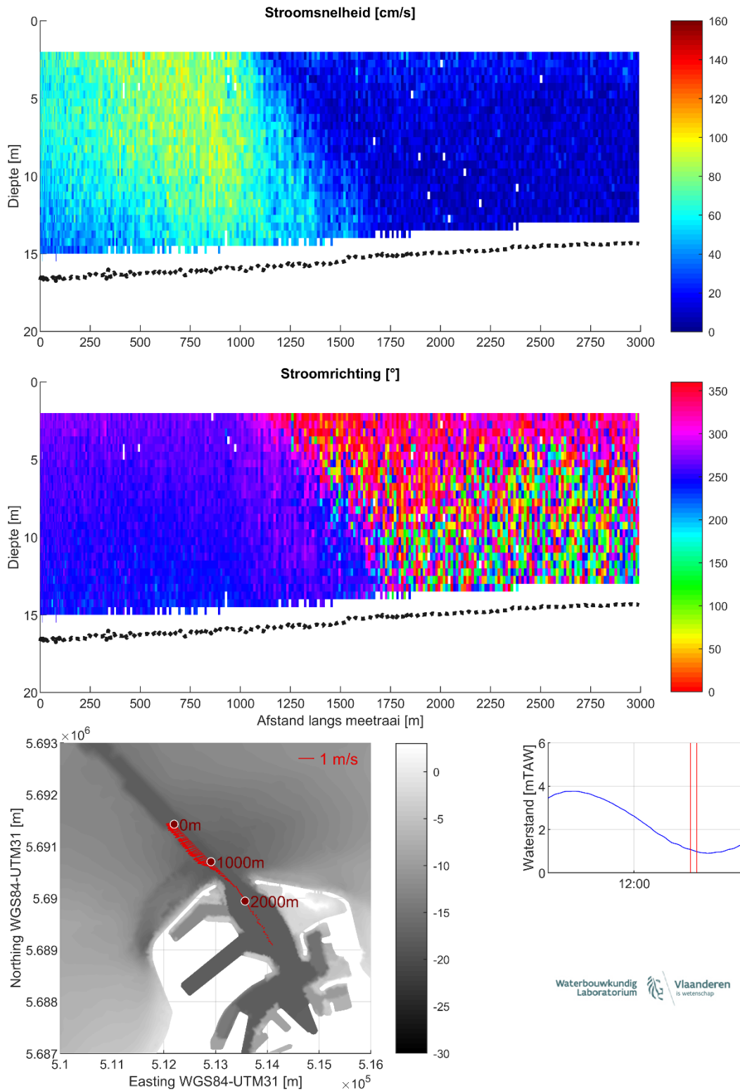
Figuur 27 – Stroomgegevens 10/08/2023 raai 22: snelheids grootte (top), -richting (midden) en diepte-gemiddelde vectoren (onder)
