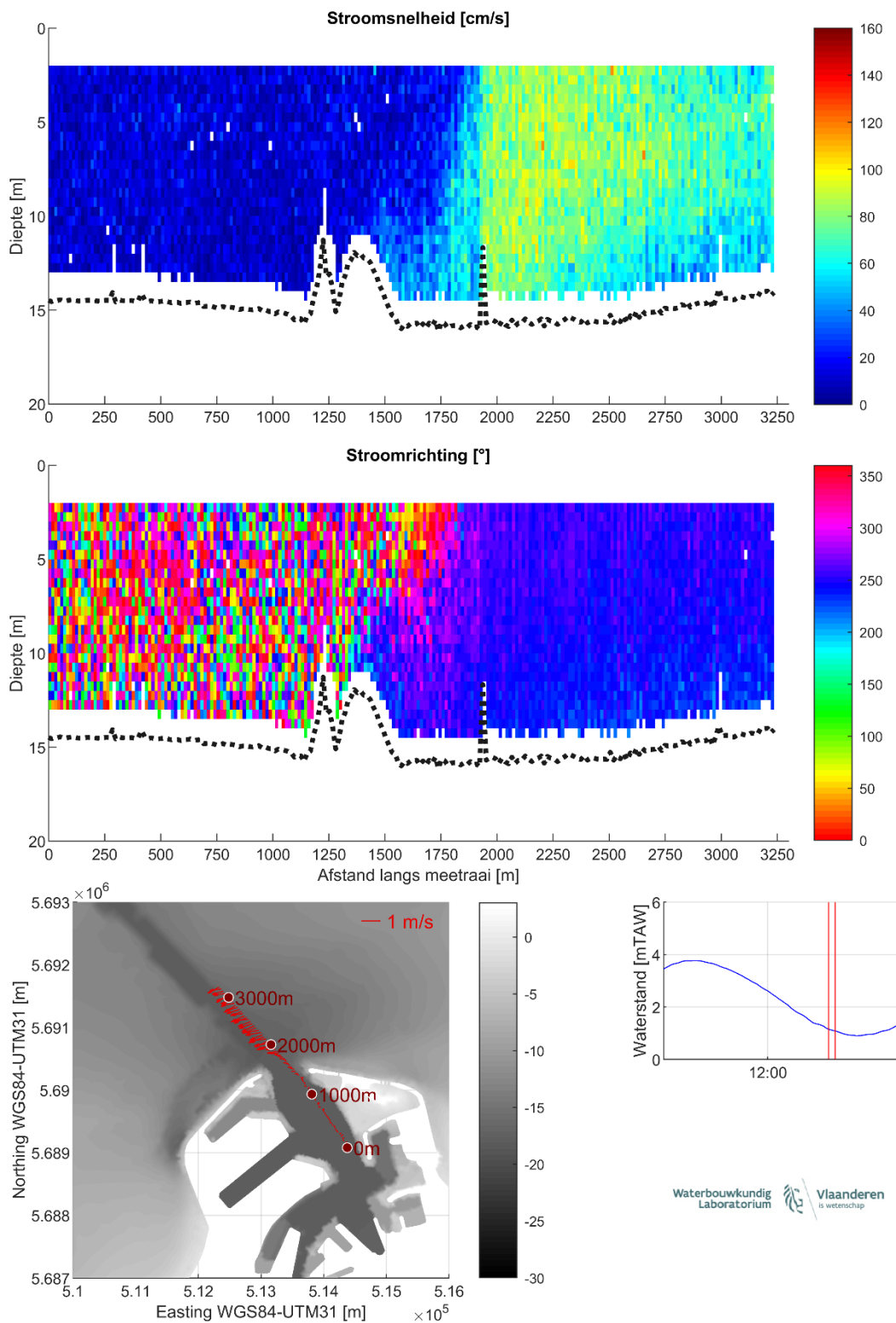
Figuur 26 – Stroomgegevens 10/08/2023 raai 21: snelheids grootte (top), -richting (midden) en diepte-gemiddelde vectoren (onder)
