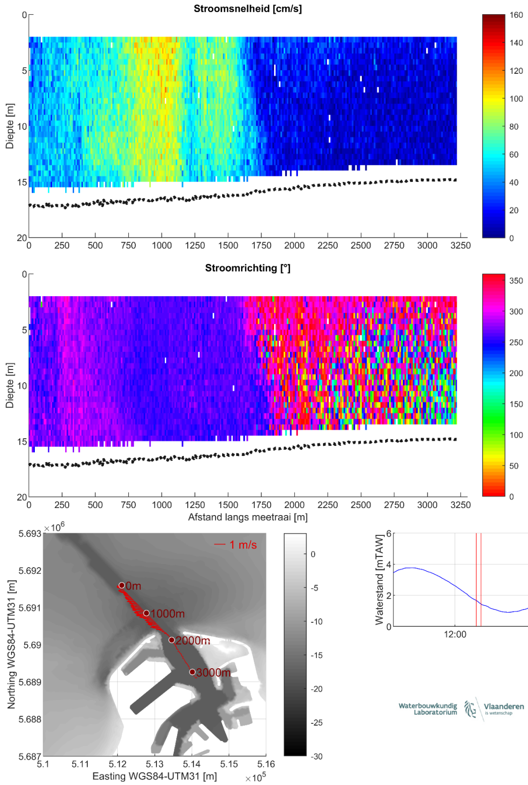
Figuur 23 – Stroomgegevens 10/08/2023 raai 18: snelheids grootte (top), -richting (midden) en diepte-gemiddelde vectoren (onder)
