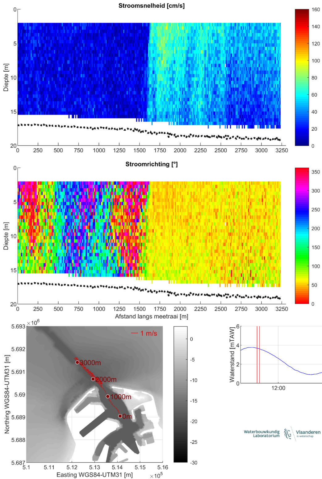
Figuur 10 – Stroomgegevens 10/08/2023 raai 5: snelheids grootte (top), -richting (midden) en diepte-gemiddelde vectoren (onder)
