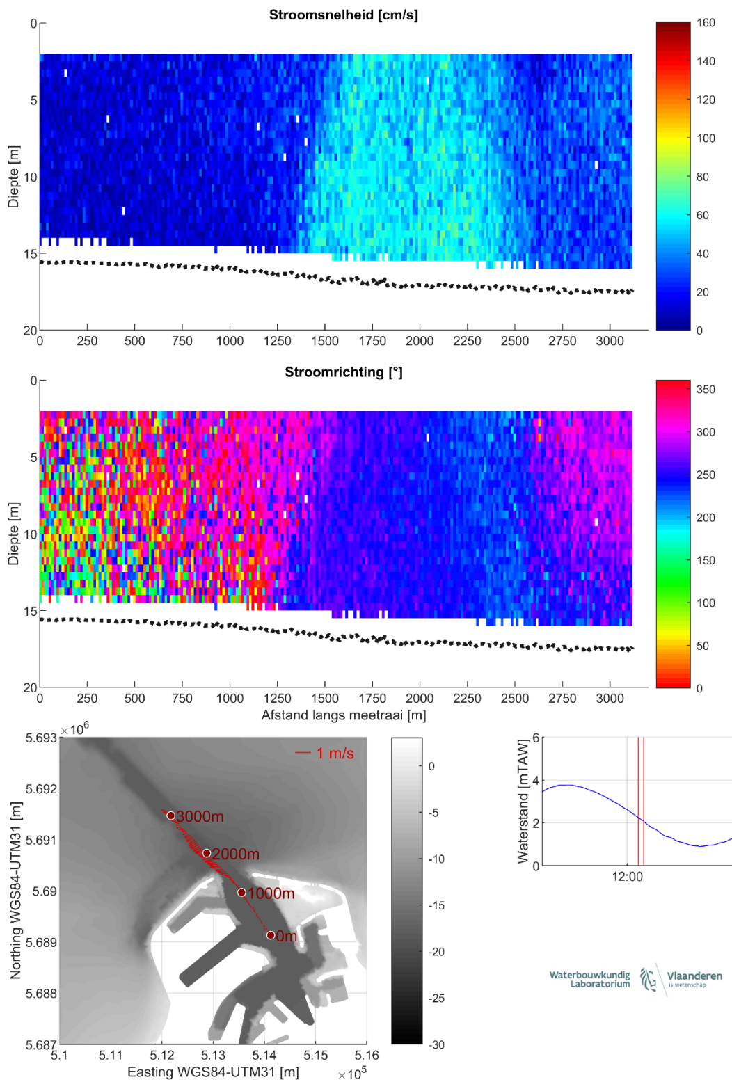
Figuur 20 – Stroomgegevens 10/08/2023 raai 15: snelheids grootte (top), -richting (midden) en diepte-gemiddelde vectoren (onder)
