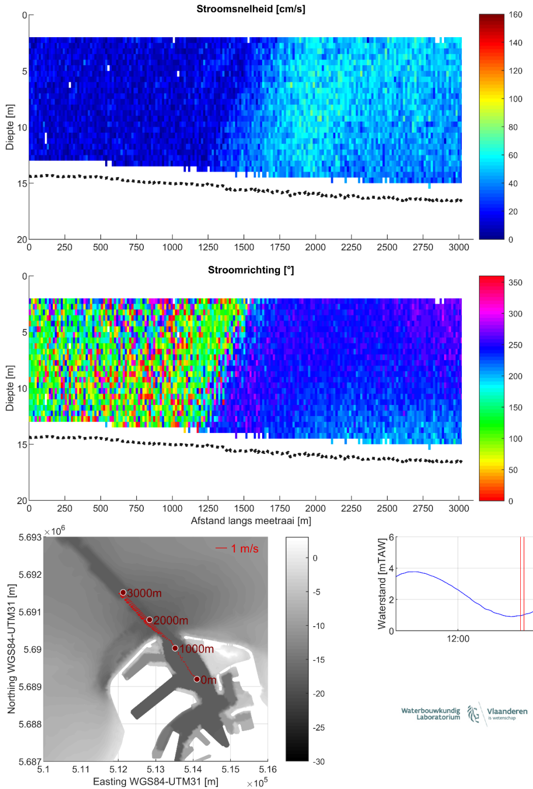
Figuur 32 – Stroomgegevens 10/08/2023 raai 27: snelheids grootte (top), -richting (midden) en diepte-gemiddelde vectoren (onder)
