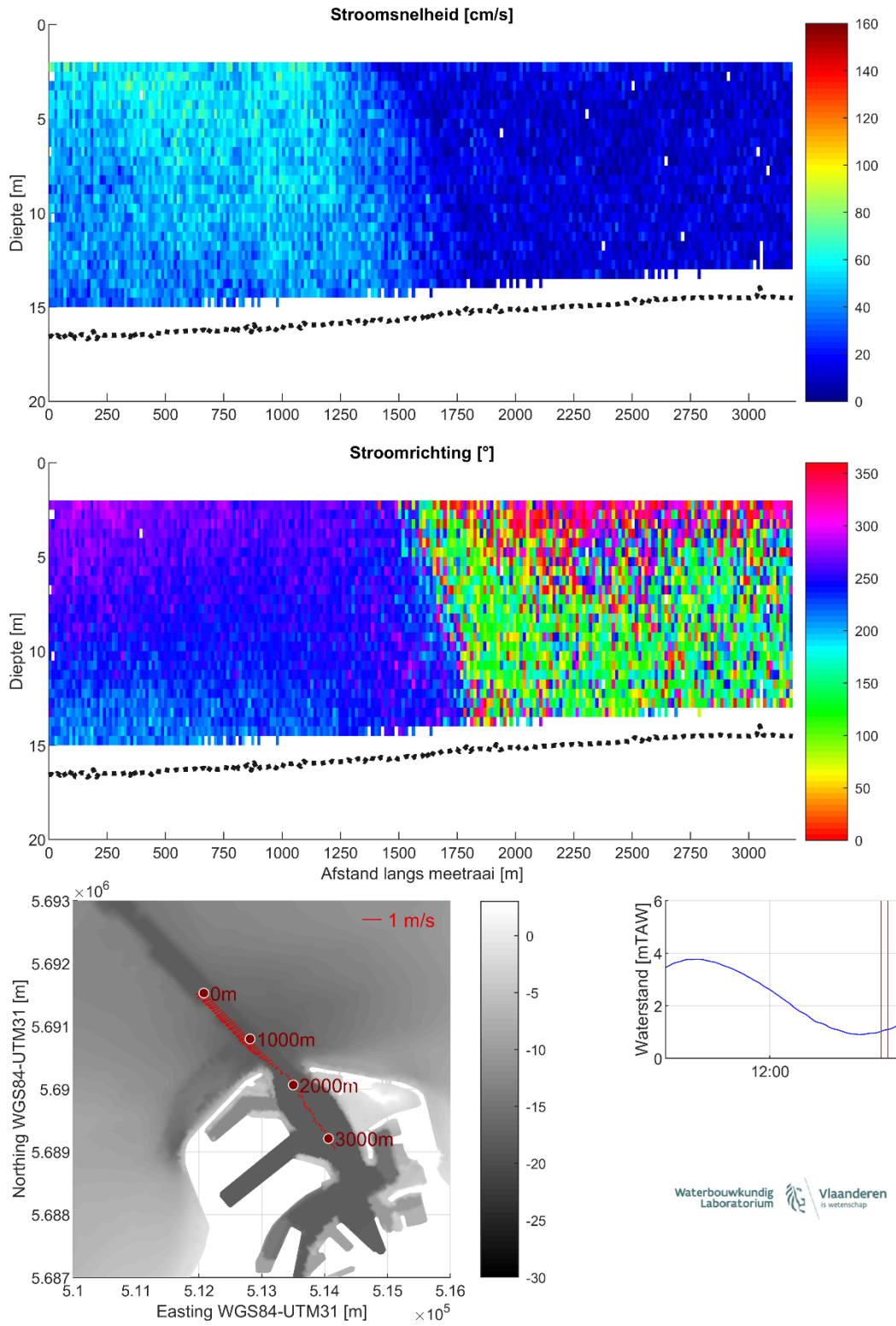
Figuur 33 – Stroomgegevens 10/08/2023 raai 28: snelheids grootte (top), -richting (midden) en diepte-gemiddelde vectoren (onder)
