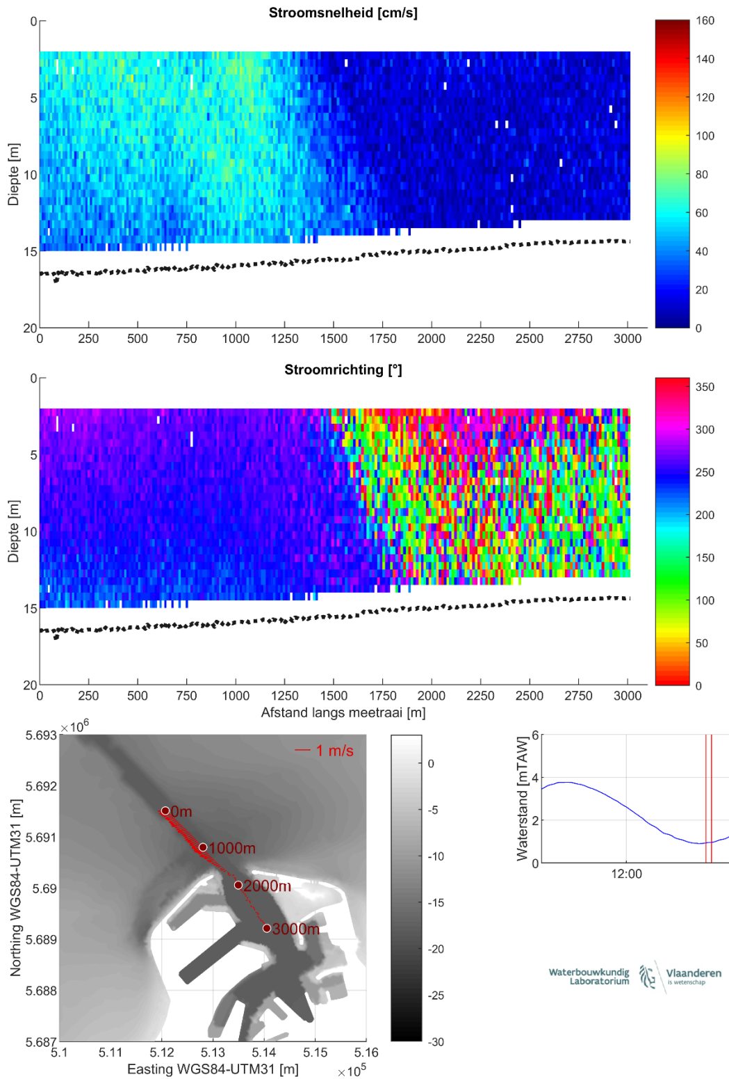
Figuur 31 – Stroomgegevens 10/08/2023 raai 26: snelheids grootte (top), -richting (midden) en diepte-gemiddelde vectoren (onder)
