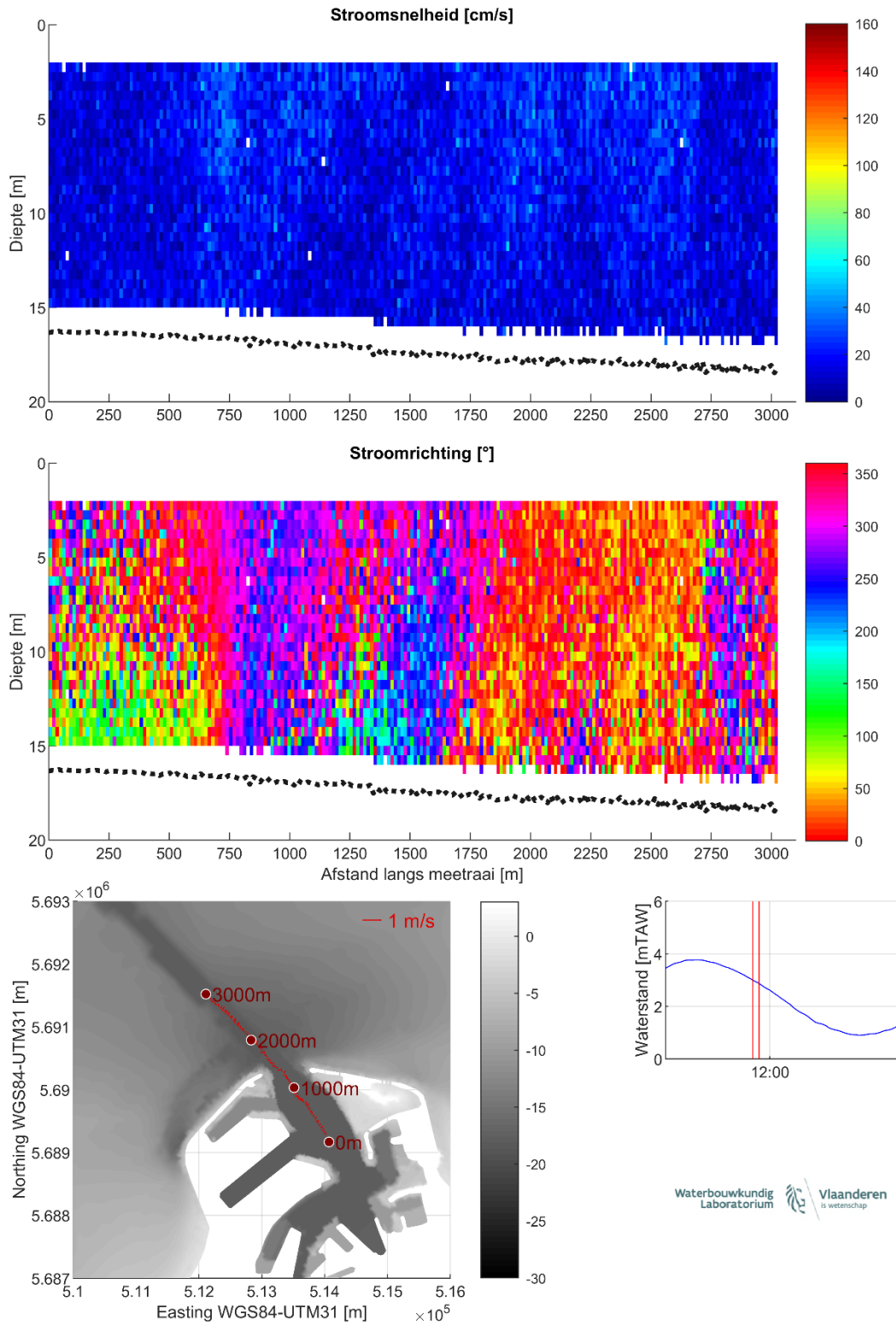
Figuur 16 – Stroomgegevens 10/08/2023 raai 11: snelheids grootte (top), -richting (midden) en diepte-gemiddelde vectoren (onder)
