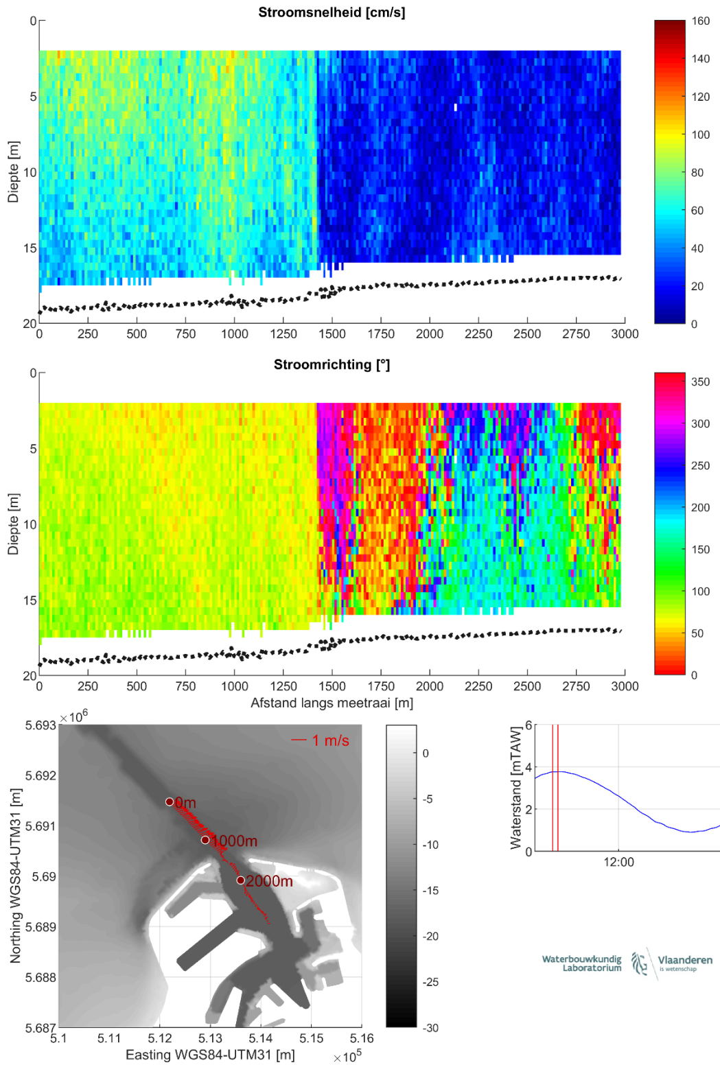
Figuur 7 – Stroomgegevens 10/08/2023 raai 2: snelheidsgrootte (top), -richting (midden) en diepte-gemiddelde vectoren (onder)
