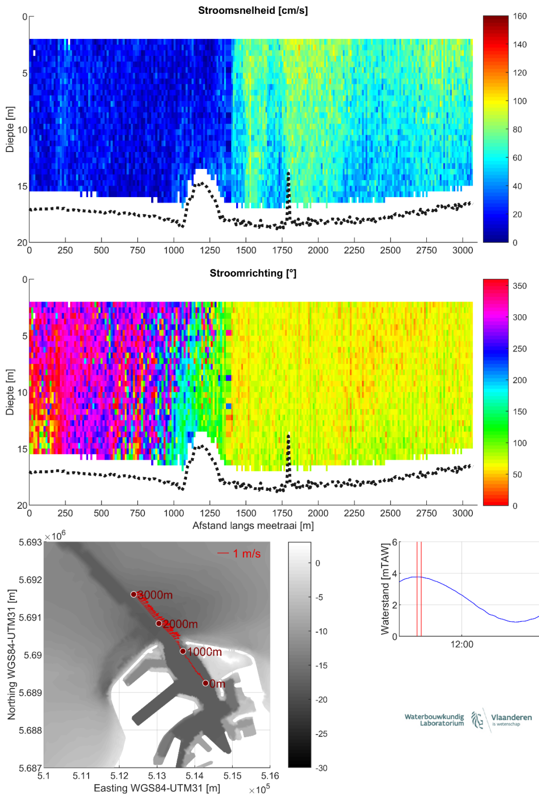
Figuur 8 – Stroomgegevens 10/08/2023 raai 3: snelheidsgrootte (top), -richting (midden) en diepte-gemiddelde vectoren (onder)
