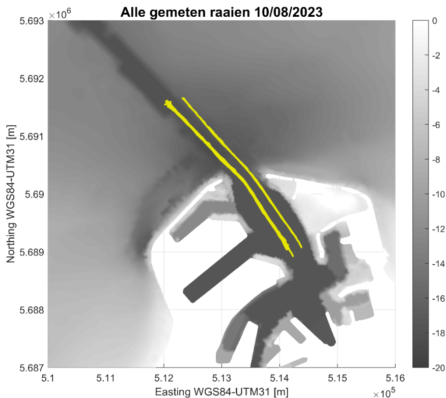
Figuur 3 – Ligging gemeten raaien op de meetdag 10/08/2023
