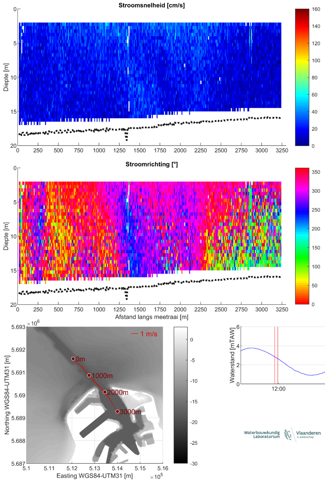
Figuur 17 – Stroomgegevens 10/08/2023 raai 12: snelheids grootte (top), -richting (midden) en diepte-gemiddelde vectoren (onder)
