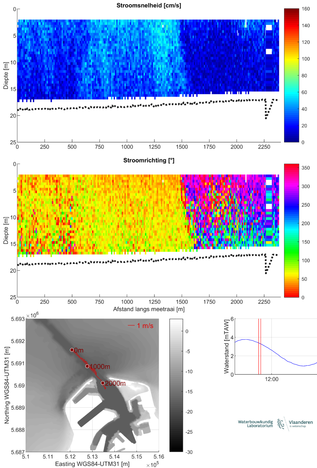
Figuur 13 – Stroomgegevens 10/08/2023 raai 8: snelheids grootte (top), -richting (midden) en diepte-gemiddelde vectoren (onder)
