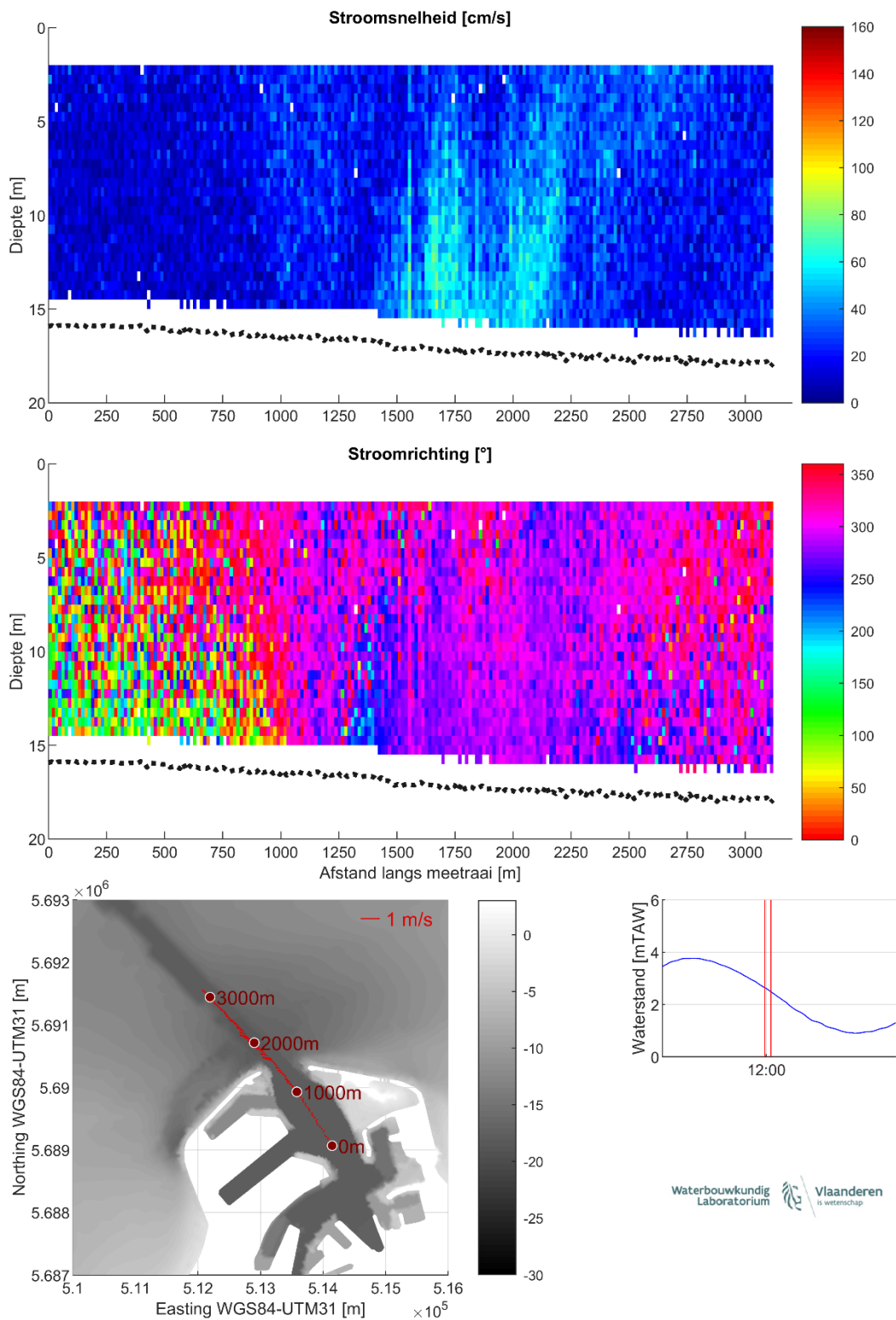
Figuur 18 – Stroomgegevens 10/08/2023 raai 13: snelheids grootte (top), -richting (midden) en diepte-gemiddelde vectoren (onder)
