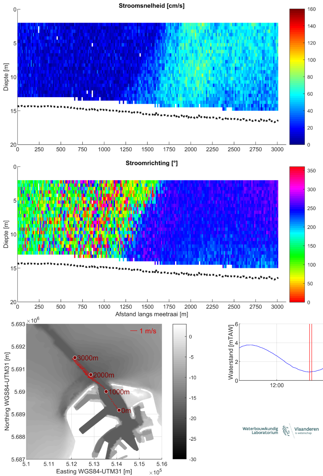
Figuur 30 – Stroomgegevens 10/08/2023 raai 25: snelheids grootte (top), -richting (midden) en diepte-gemiddelde vectoren (onder)
