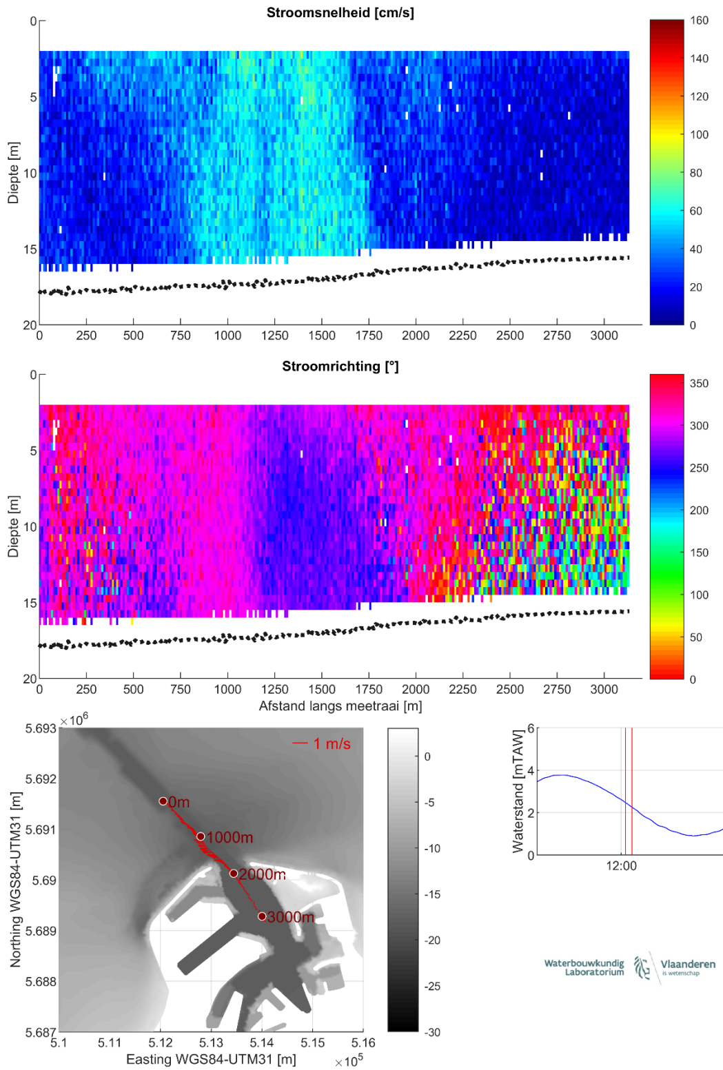
Figuur 19 – Stroomgegevens 10/08/2023 raai 14: snelheids grootte (top), -richting (midden) en diepte-gemiddelde vectoren (onder)
