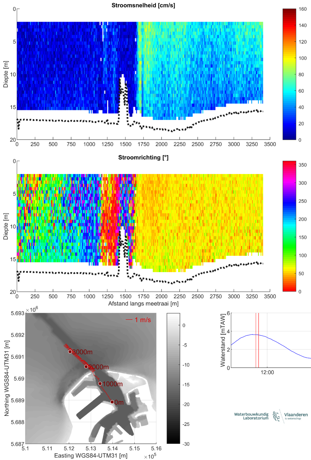
Figuur 12 – Stroomgegevens 11/08/2023 raai 7: snelheids grootte (top), -richting (midden) en diepte-gemiddelde vectoren (onder)
