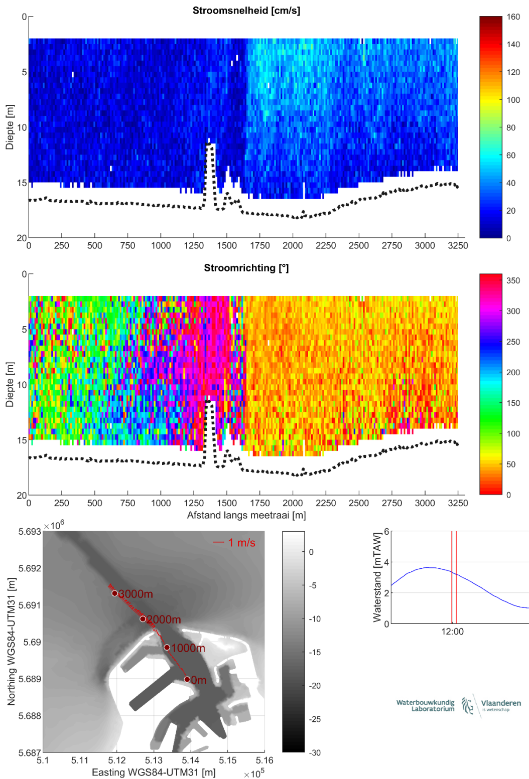
Figuur 16 – Stroomgegevens 11/08/2023 raai 11: snelheids grootte (top), -richting (midden) en diepte-gemiddelde vectoren (onder)
