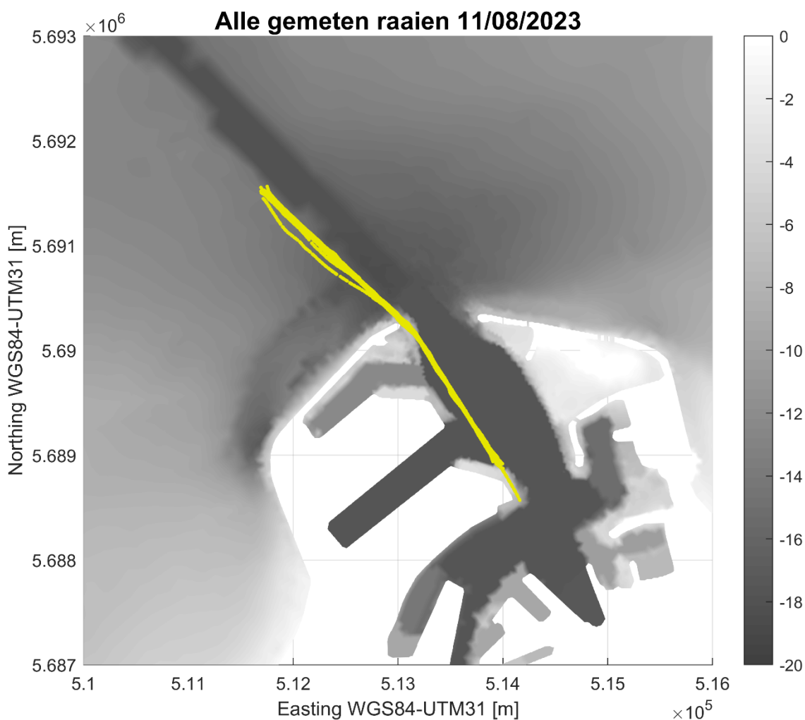
Figuur 3 – Ligging gemeten raaien op de meetdag 11/08/2023
