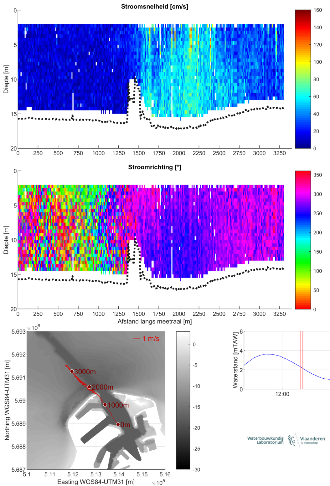
Figuur 22 – Stroomgegevens 11/08/2023 raai 17: snelheids grootte (top), -richting (midden) en diepte-gemiddelde vectoren (onder)
