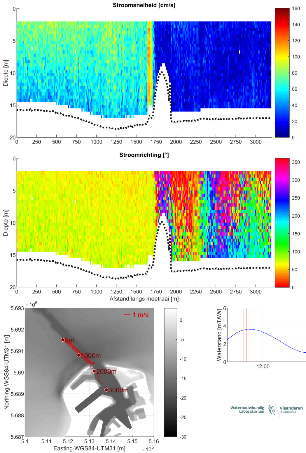
Figuur 9 – Stroomgegevens 11/08/2023 raai 4: snelheidsgrootte (top), -richting (midden) en diepte-gemiddelde vectoren (onder)
