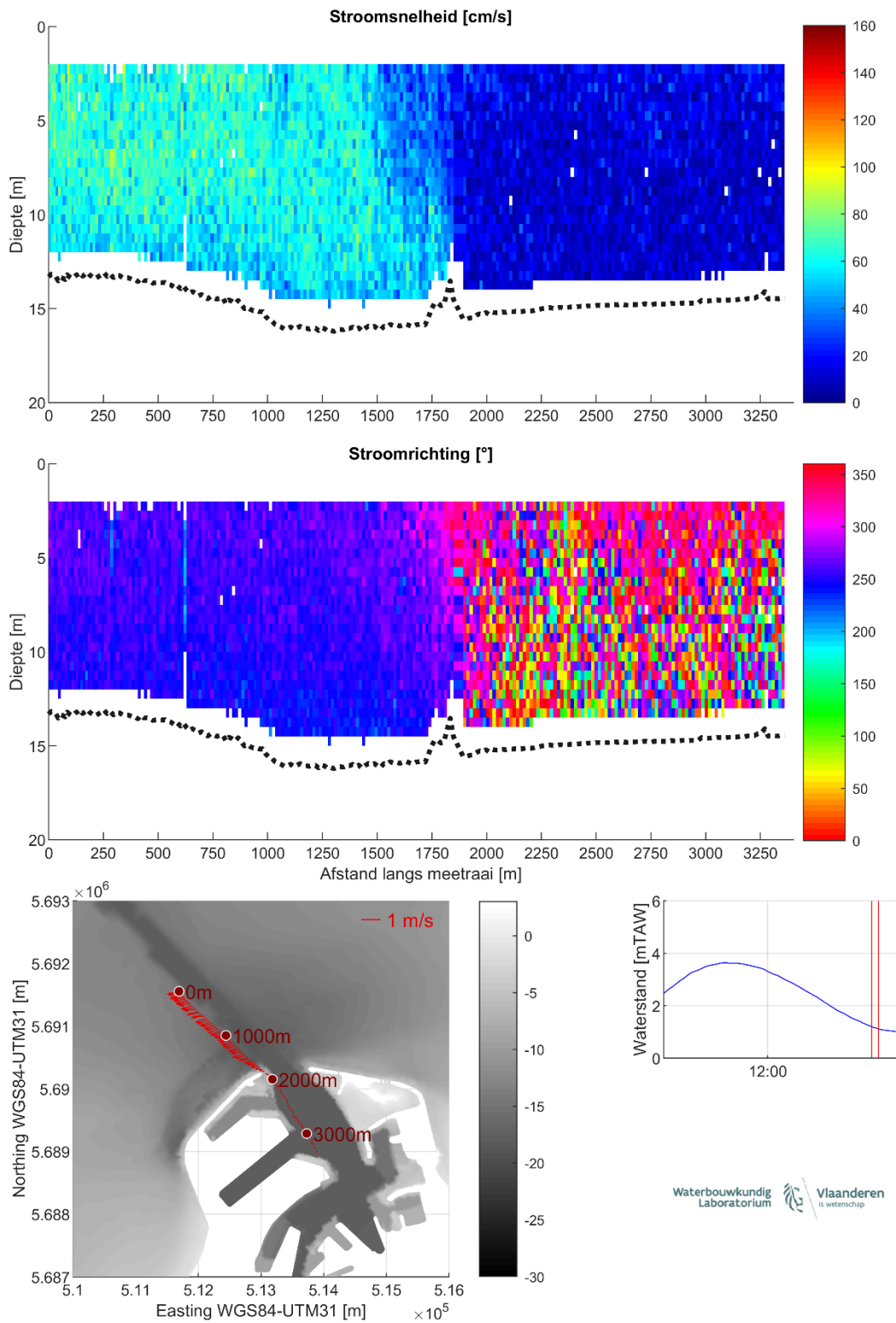
Figuur 29 – Stroomgegevens 11/08/2023 raai 24: snelheids grootte (top), -richting (midden) en diepte-gemiddelde vectoren (onder)
