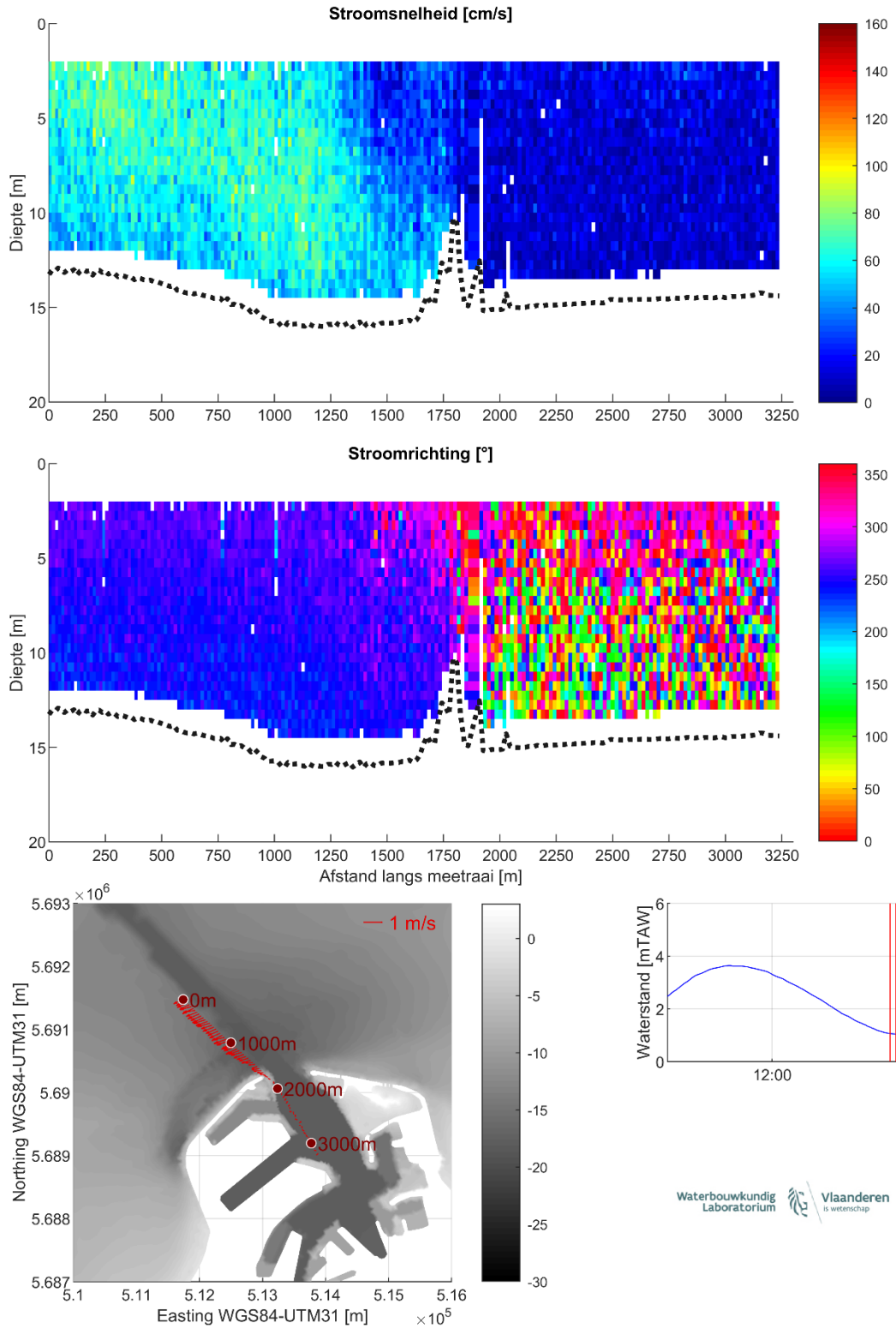
Figuur 31 – Stroomgegevens 11/08/2023 raai 26: snelheids grootte (top), -richting (midden) en diepte-gemiddelde vectoren (onder)
