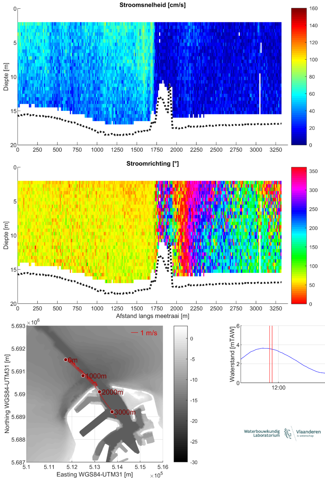
Figuur 13 – Stroomgegevens 11/08/2023 raai 8: snelheids grootte (top), -richting (midden) en diepte-gemiddelde vectoren (onder)
