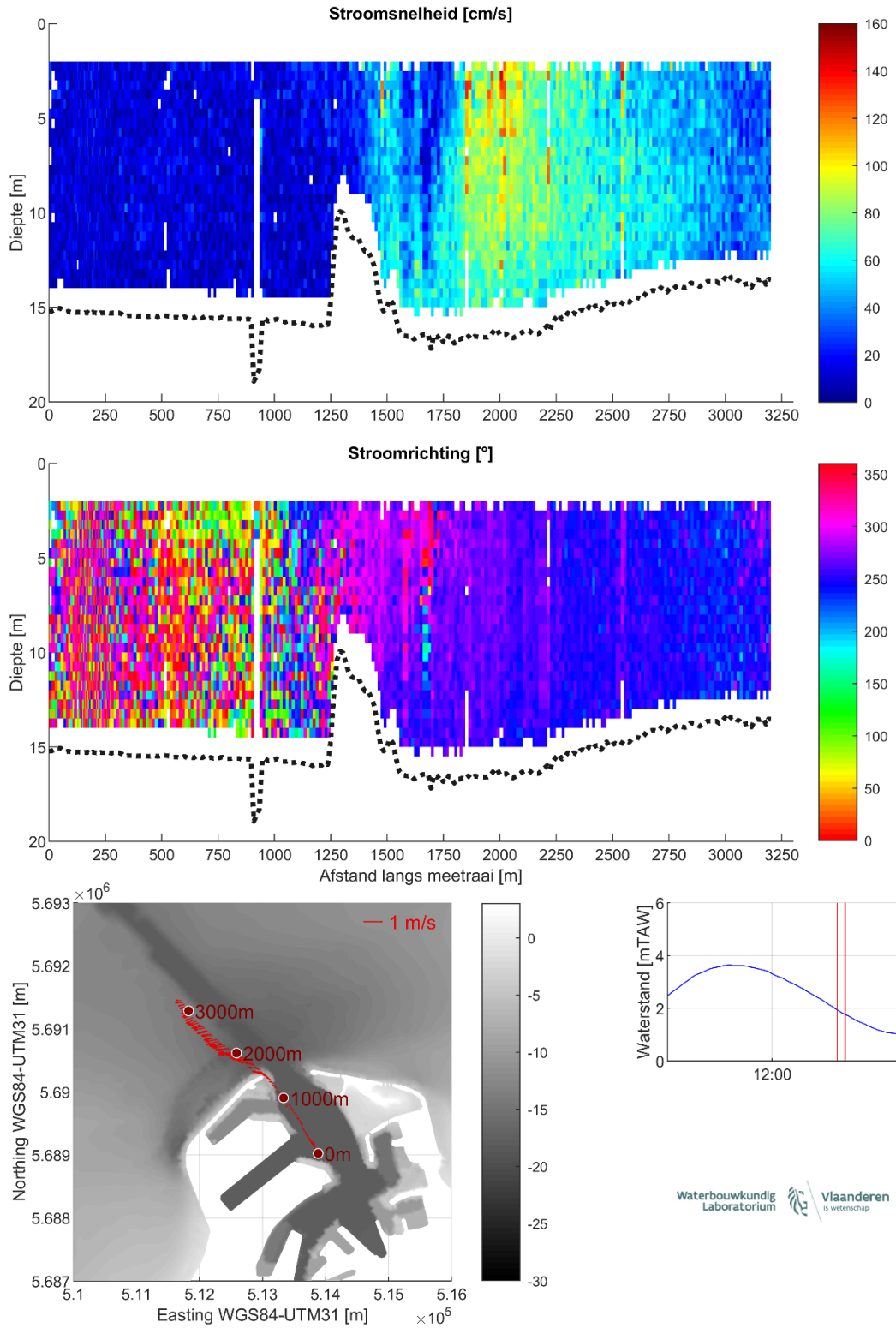
Figuur 24 – Stroomgegevens 11/08/2023 raai 19: snelheids grootte (top), -richting (midden) en diepte-gemiddelde vectoren (onder)
