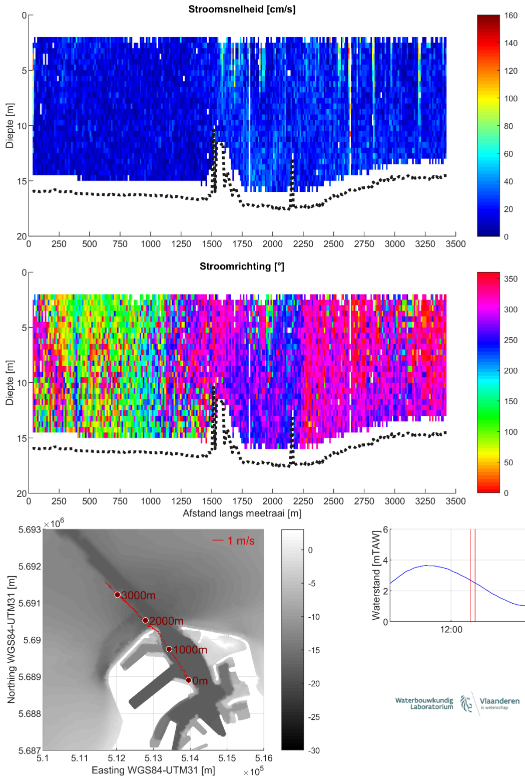
Figuur 20 – Stroomgegevens 11/08/2023 raai 15: snelheids grootte (top), -richting (midden) en diepte-gemiddelde vectoren (onder)
