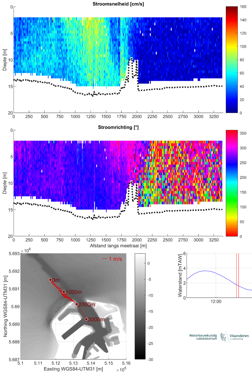
Figuur 25 – Stroomgegevens 11/08/2023 raai 20: snelheids grootte (top), -richting (midden) en diepte-gemiddelde vectoren (onder)
