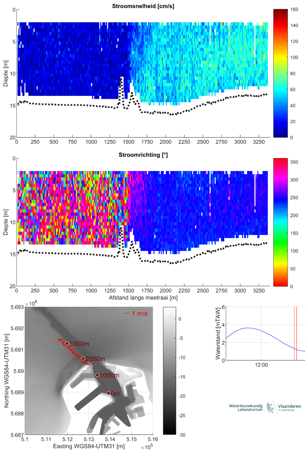
Figuur 28 – Stroomgegevens 11/08/2023 raai 23: snelheids grootte (top), -richting (midden) en diepte-gemiddelde vectoren (onder)
