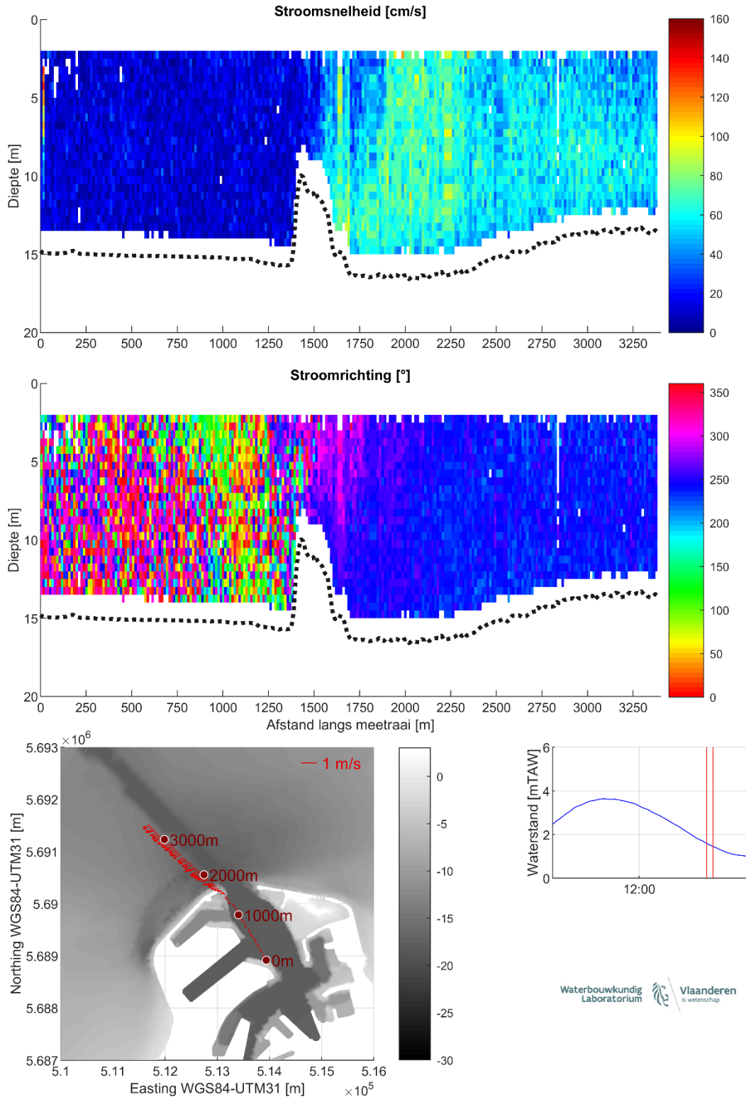
Figuur 26 – Stroomgegevens 11/08/2023 raai 21: snelheidsgrootte (top), -richting (midden) en diepte-gemiddelde vectoren (onder)
