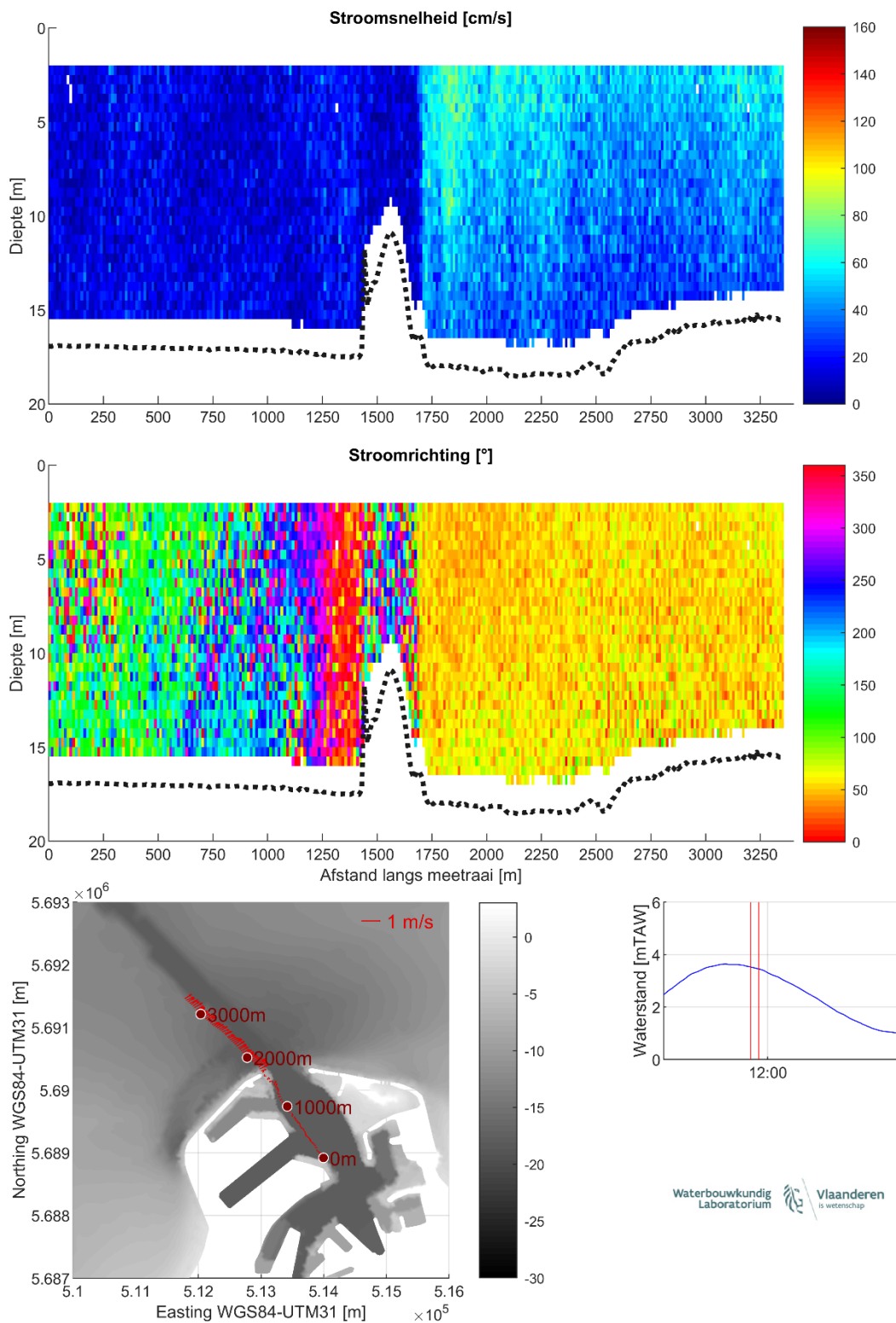
Figuur 14 – Stroomgegevens 11/08/2023 raai 9: snelheidsgrötte (top), -richting (midden) en diepte-gemiddelde vectoren (onder)
