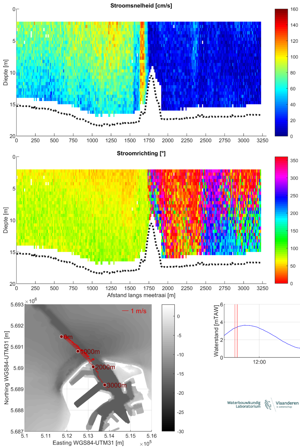
Figuur 7 – Stroomgegevens 11/08/2023 raai 2: snelheids grootte (top), -richting (midden) en diepte-gemiddelde vectoren (onder)
