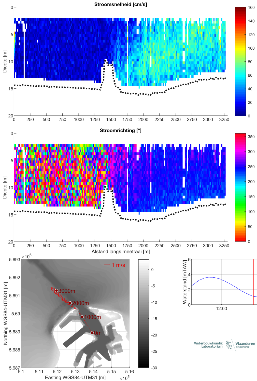
Figuur 30 – Stroomgegevens 11/08/2023 raai 25: snelheids grootte (top), -richting (midden) en diepte-gemiddelde vectoren (onder)
