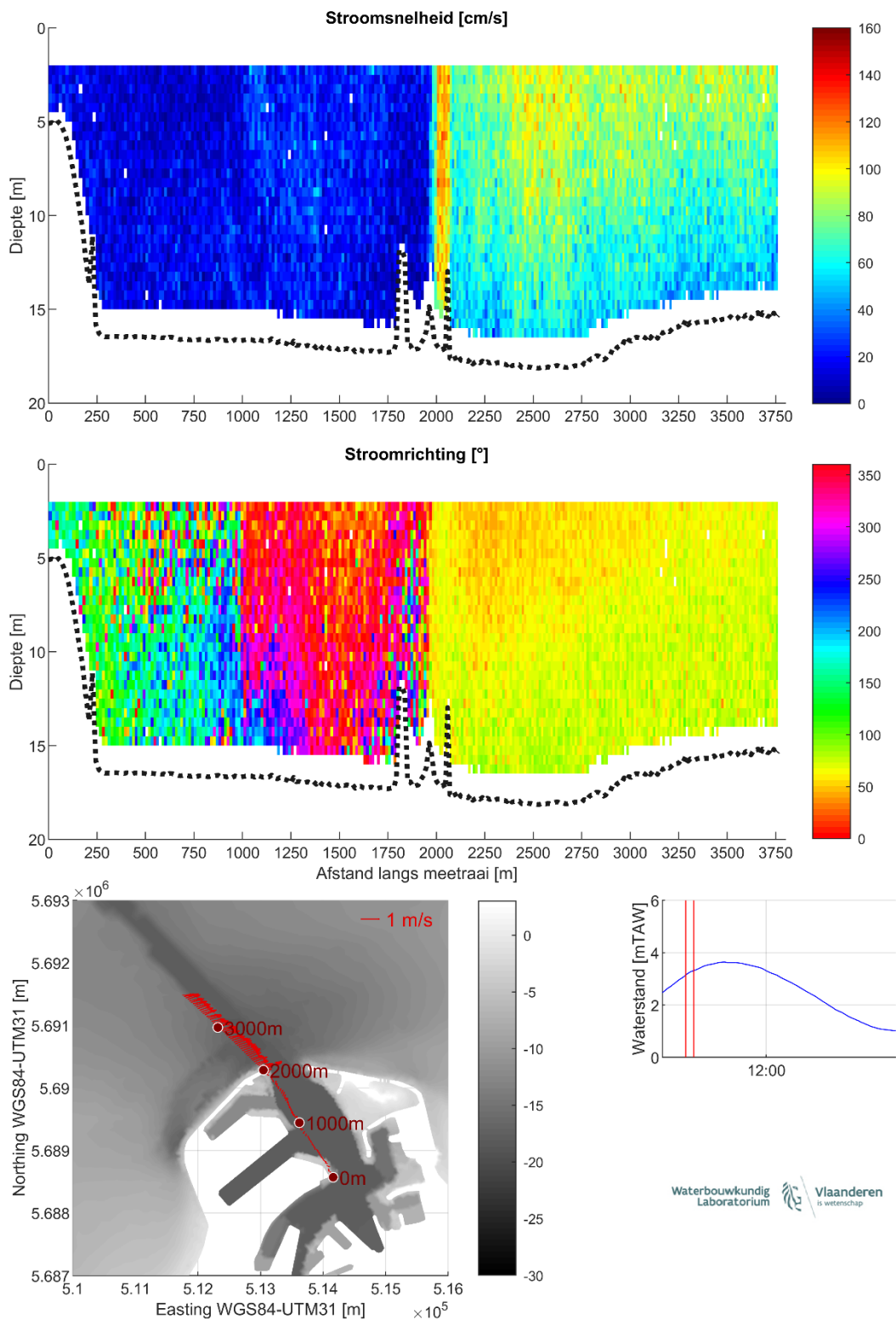
Figuur 6 – Stroomgegevens 11/08/2023 raai 1: snelheids-grootte (top), -richting (midden) en diepte-gemiddelde vectoren (onder)
