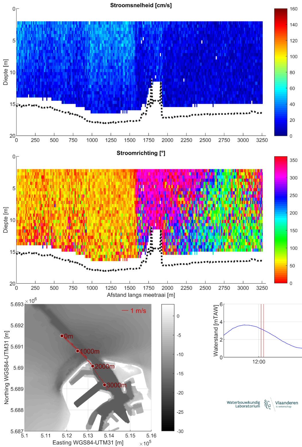
Figuur 17 – Stroomgegevens 11/08/2023 raai 12: snelheids grootte (top), -richting (midden) en diepte-gemiddelde vectoren (onder)
