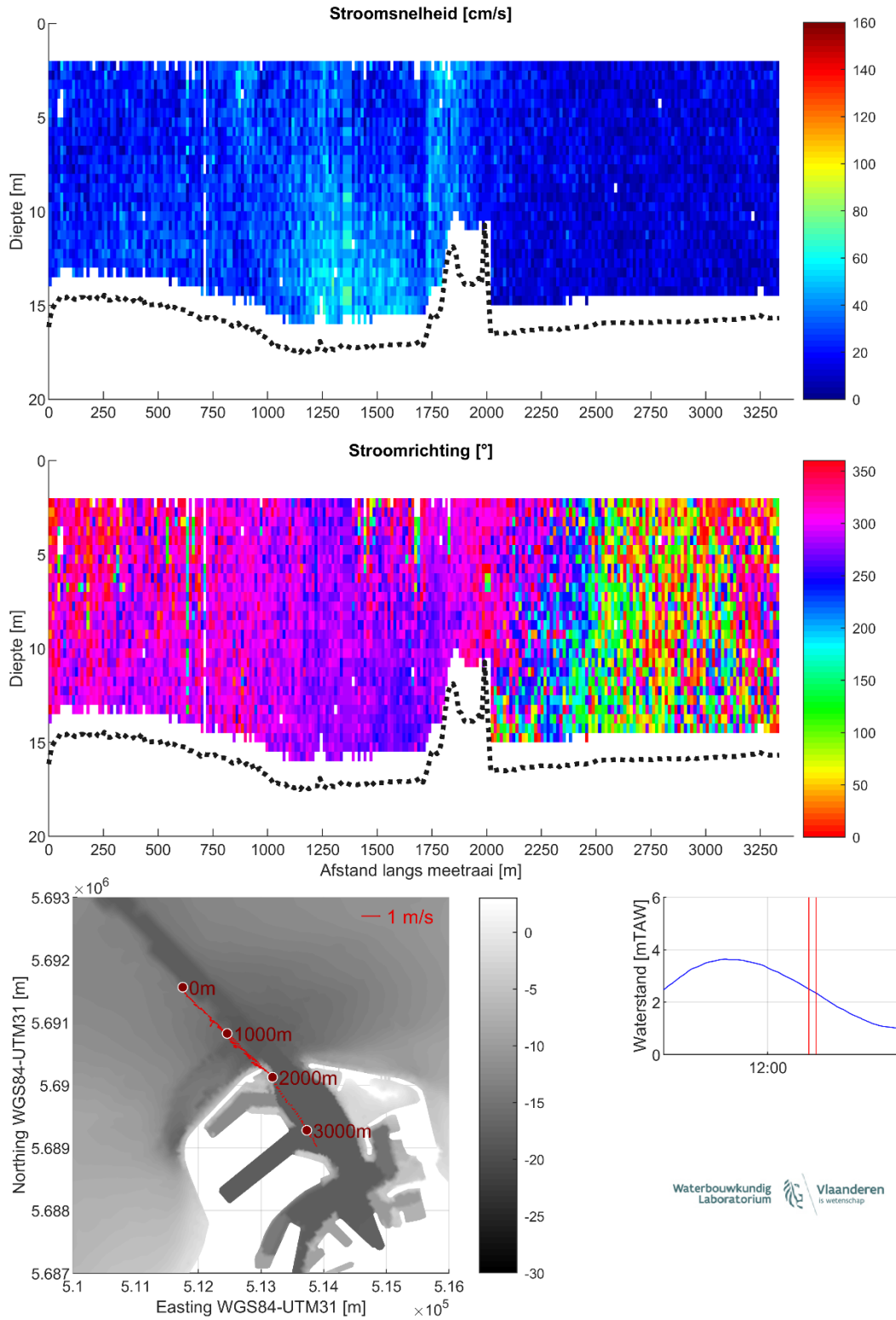
Figuur 21 – Stroomgegevens 11/08/2023 raai 16: snelheids grootte (top), -richting (midden) en diepte-gemiddelde vectoren (onder)
