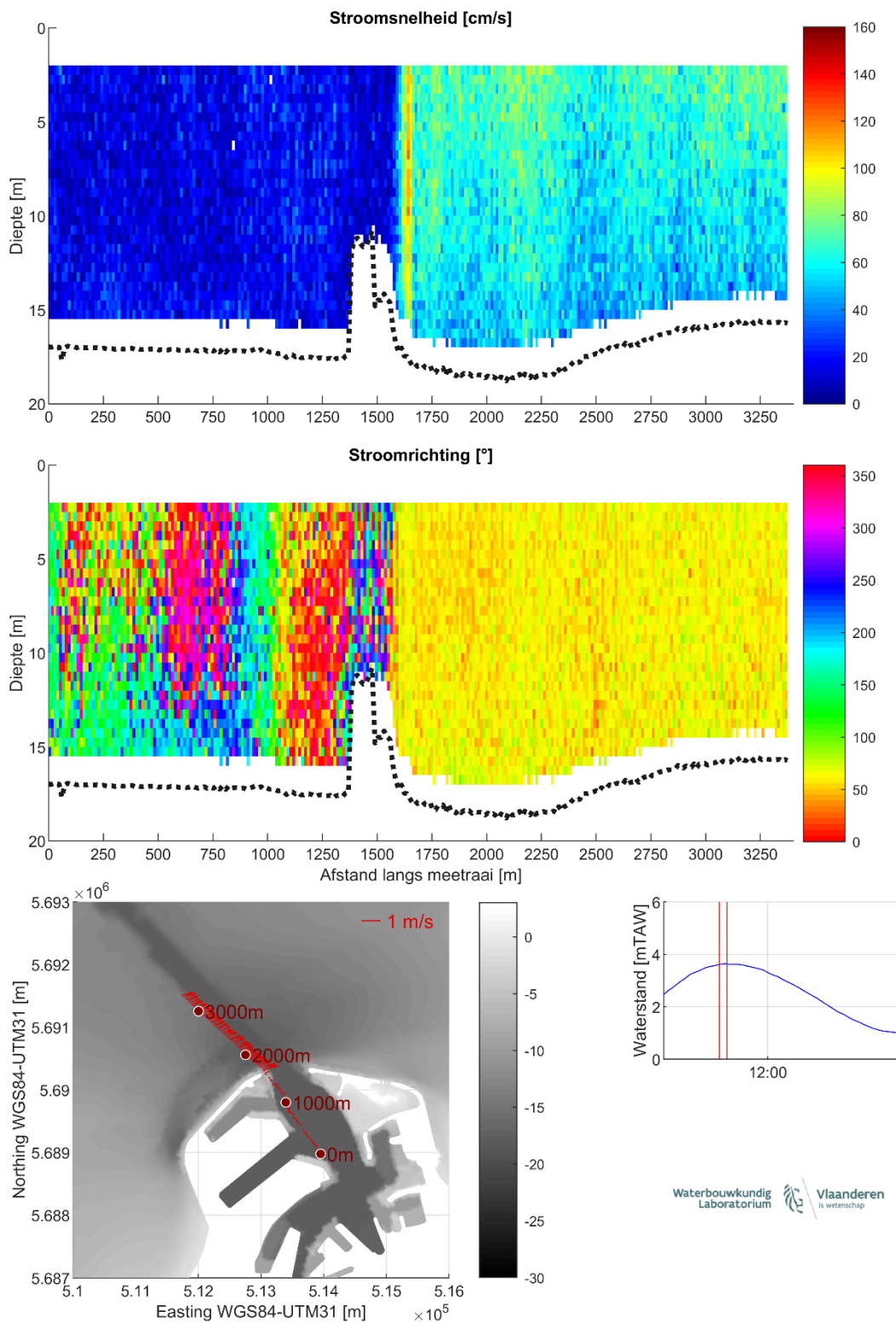
Figuur 10 – Stroomgegevens 11/08/2023 raai 5: snelheids grootte (top), -richting (midden) en diepte-gemiddelde vectoren (onder)
