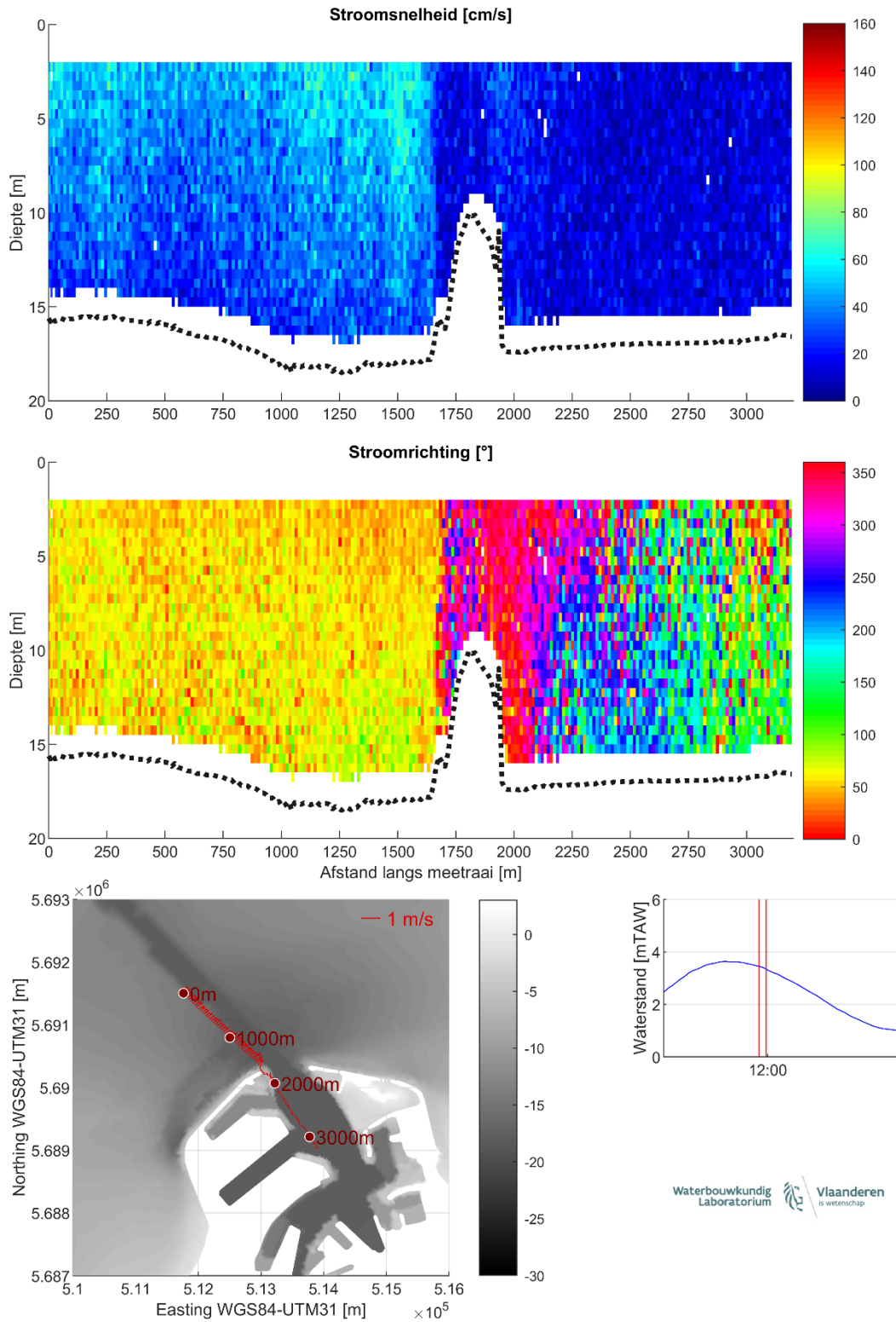
Figuur 15 – Stroomgegevens 11/08/2023 raai 10: snelheids grootte (top), -richting (midden) en diepte-gemiddelde vectoren (onder)
