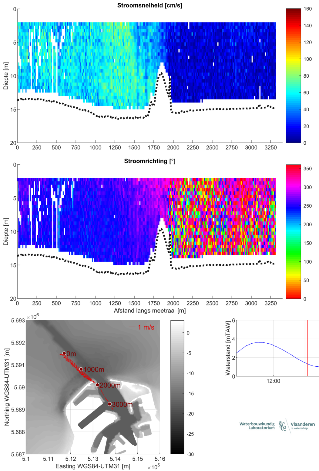
Figuur 27 – Stroomgegevens 11/08/2023 raai 22: snelheids grootte (top), -richting (midden) en diepte-gemiddelde vectoren (onder)
