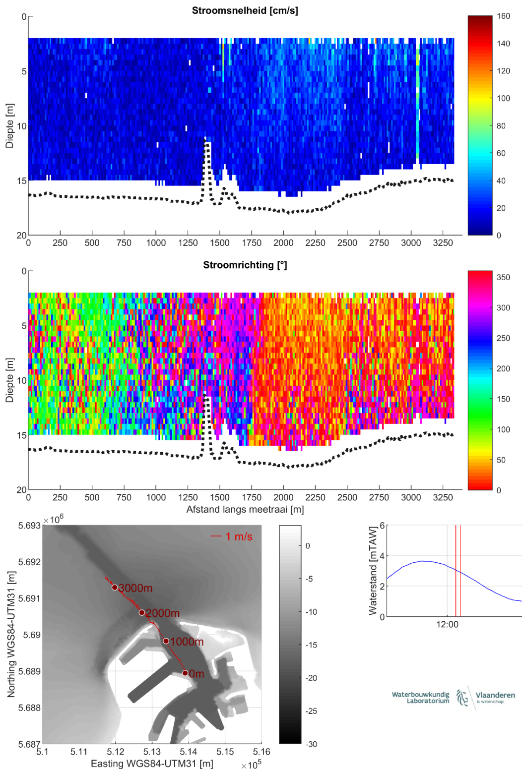
Figuur 18 – Stroomgegevens 11/08/2023 raai 13: snelheids grootte (top), -richting (midden) en diepte-gemiddelde vectoren (onder)
