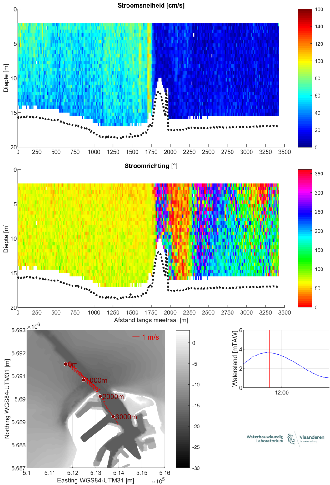
Figuur 11 – Stroomgegevens 11/08/2023 raai 6: snelheids grootte (top), -richting (midden) en diepte-gemiddelde vectoren (onder)
