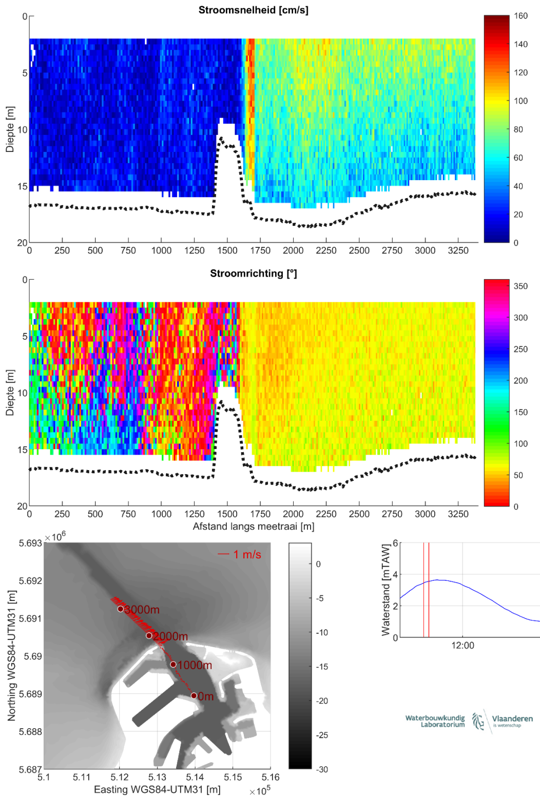
Figuur 8 – Stroomgegevens 11/08/2023 raai 3: snelheids grootte (top), -richting (midden) en diepte-gemiddelde vectoren (onder)
