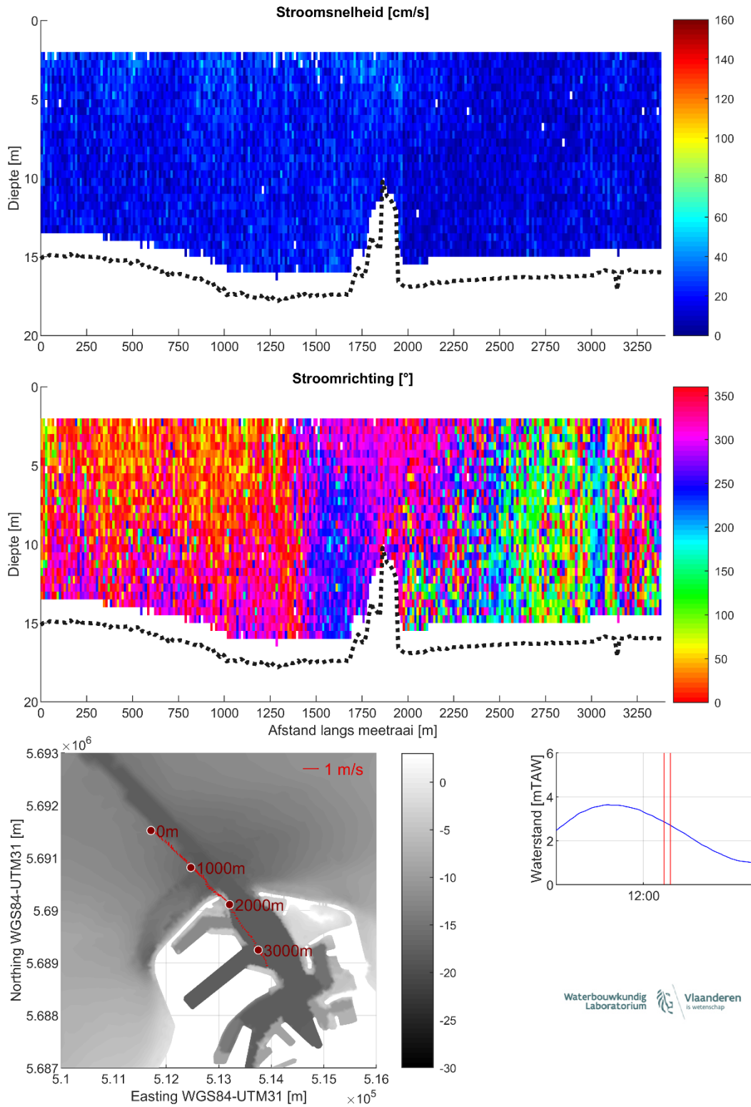
Figuur 19 – Stroomgegevens 11/08/2023 raai 14: snelheids grootte (top), -richting (midden) en diepte-gemiddelde vectoren (onder)
