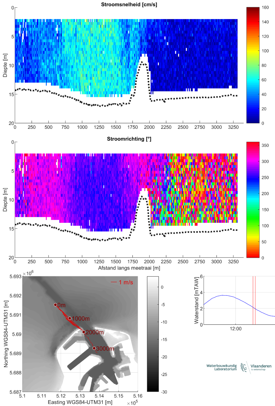
Figuur 23 – Stroomgegevens 11/08/2023 raai 18: snelheids grootte (top), -richting (midden) en diepte-gemiddelde vectoren (onder)
