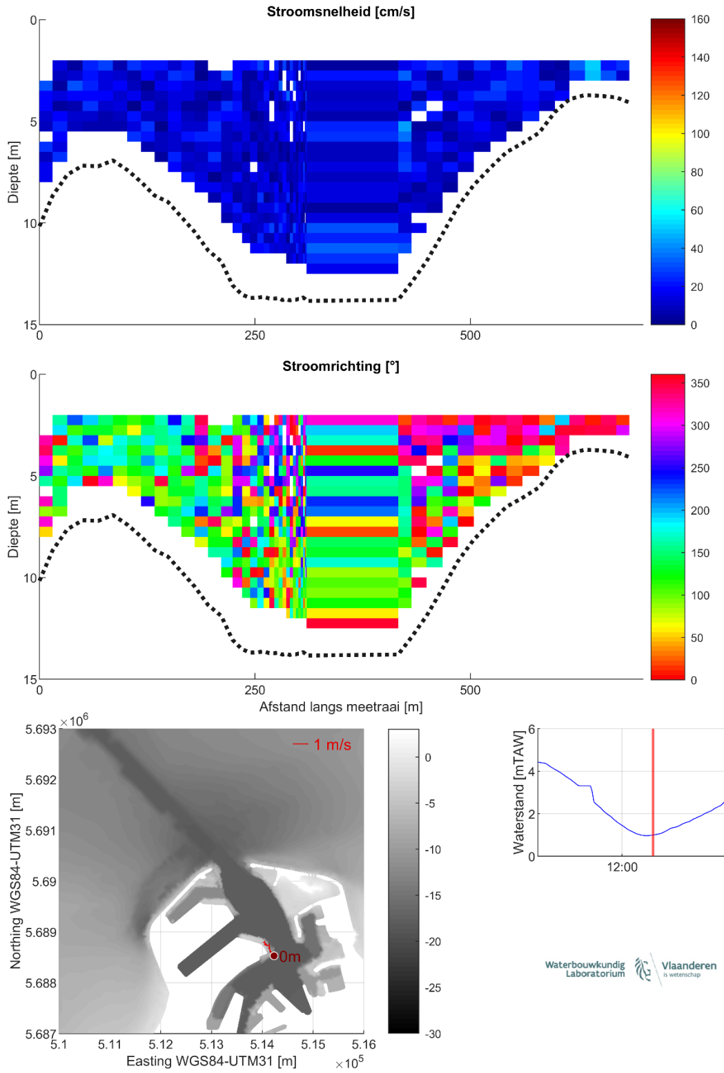
Figuur 26 – Stroomgegevens 08/08/2023 raai 21: snelheids grootte (top), -richting (midden) en diepte-gemiddelde vectoren (onder)
