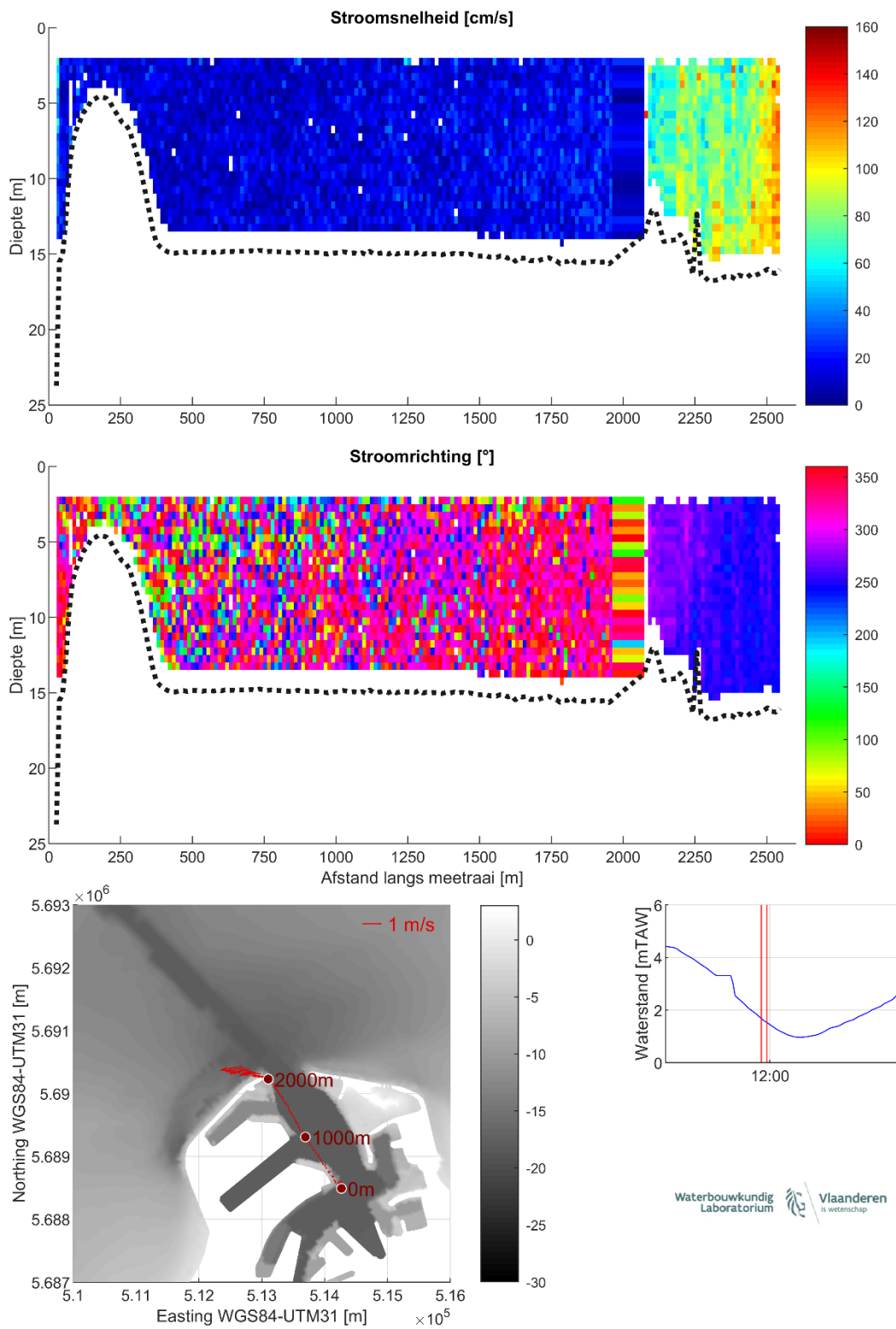
Figuur 19 – Stroomgegevens 08/08/2023 raai 14: snelheids grootte (top), -richting (midden) en diepte-gemiddelde vectoren (onder)
