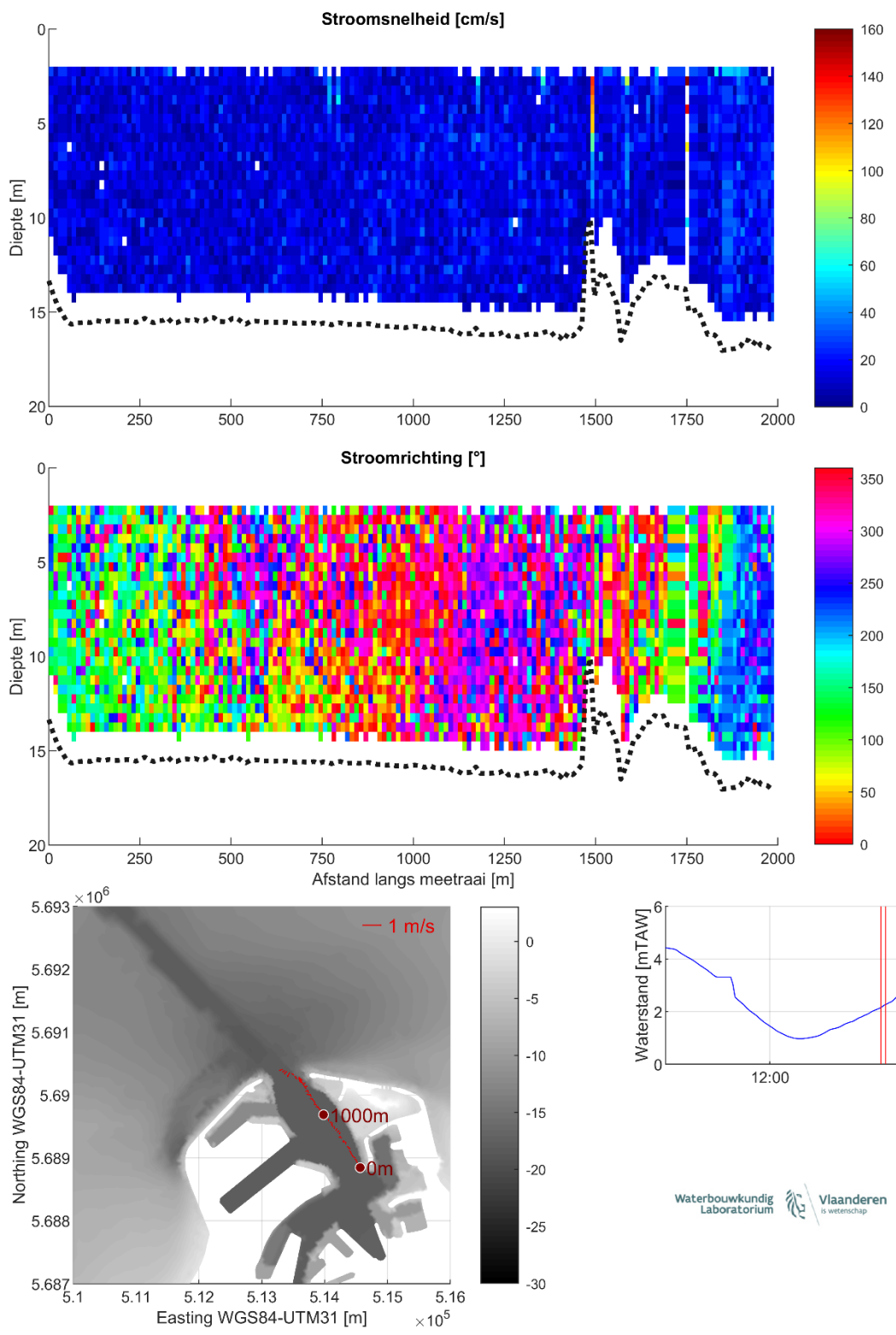
Figuur 39 – Stroomgegevens 08/08/2023 raai 34: snelheids grootte (top), -richting (midden) en diepte-gemiddelde vectoren (onder)
