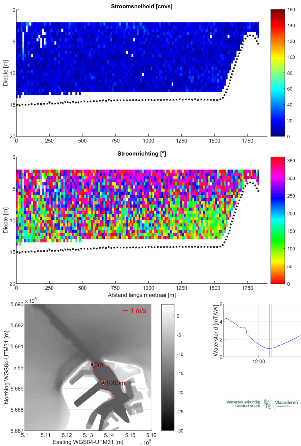
Figuur 25 – Stroomgegevens 08/08/2023 raai 20: snelheids grootte (top), -richting (midden) en diepte-gemiddelde vectoren (onder)
