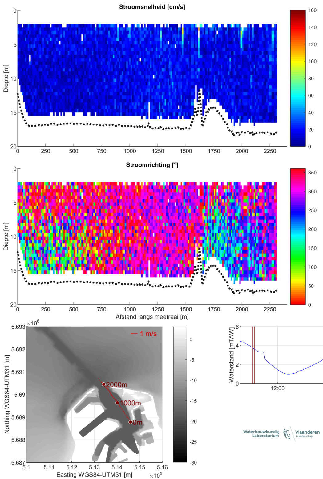
Figuur 9 – Stroomgegevens 08/08/2023 raai 4: snelheidsgruotte (top), -richting (midden) en diepte-gemiddelde vectoren (onder)
