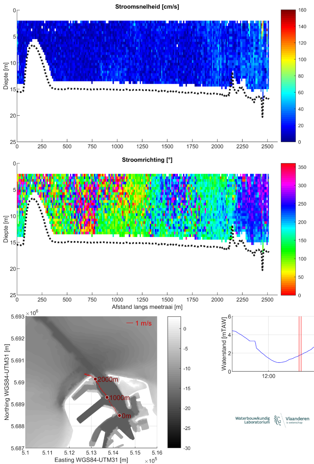
Figuur 35 – Stroomgegevens 08/08/2023 raai 30: snelheids grootte (top), -richting (midden) en diepte-gemiddelde vectoren (onder)
