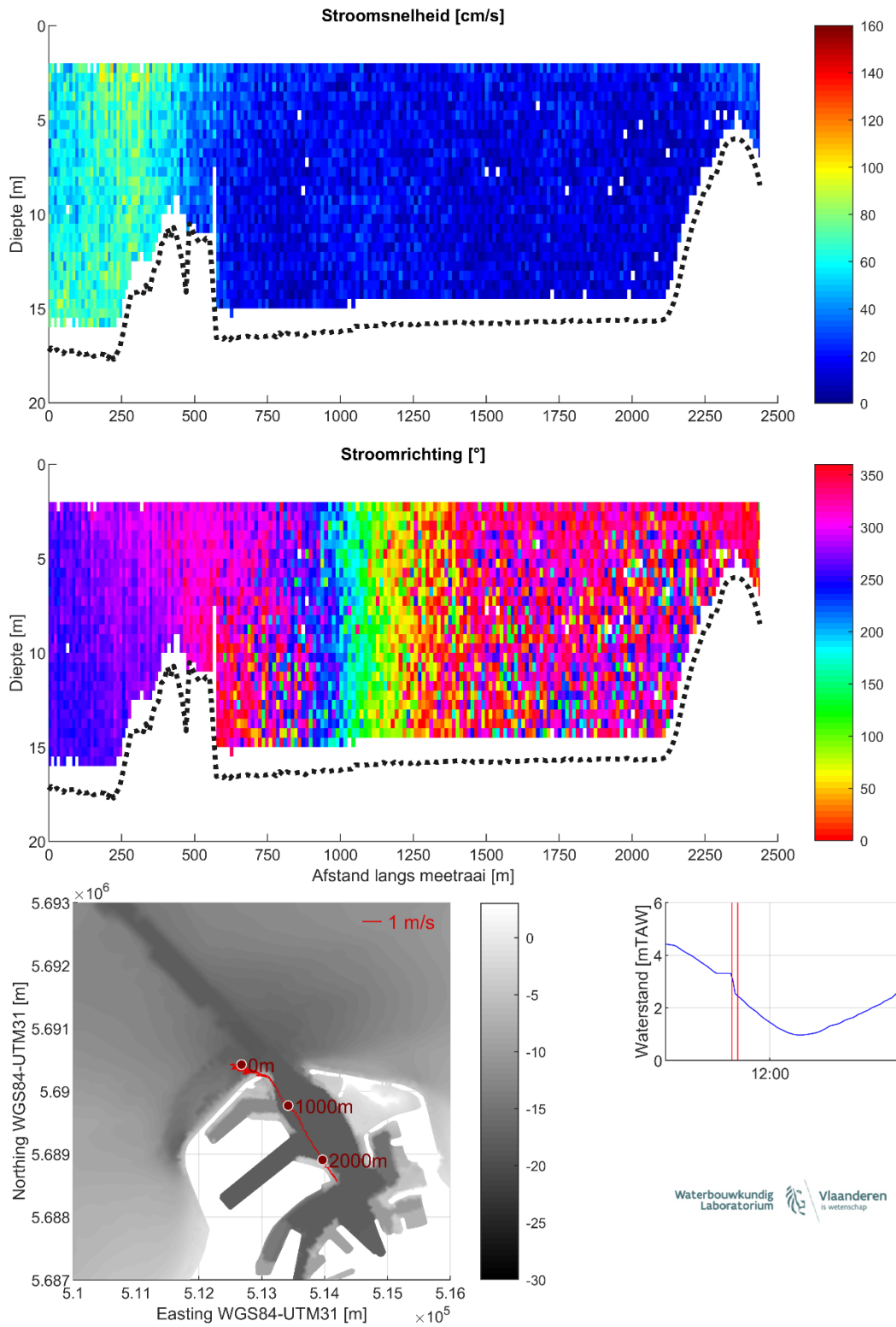
Figuur 14 – Stroomgegevens 08/08/2023 raai 9: snelheids grootte (top), -richting (midden) en diepte-gemiddelde vectoren (onder)
