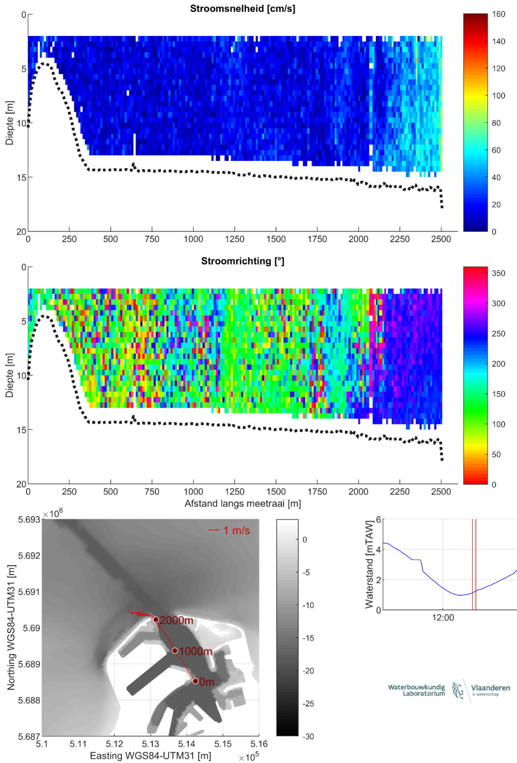
Figuur 29 – Stroomgegevens 08/08/2023 raai 24: snelheids grootte (top), -richting (midden) en diepte-gemiddelde vectoren (onder)
