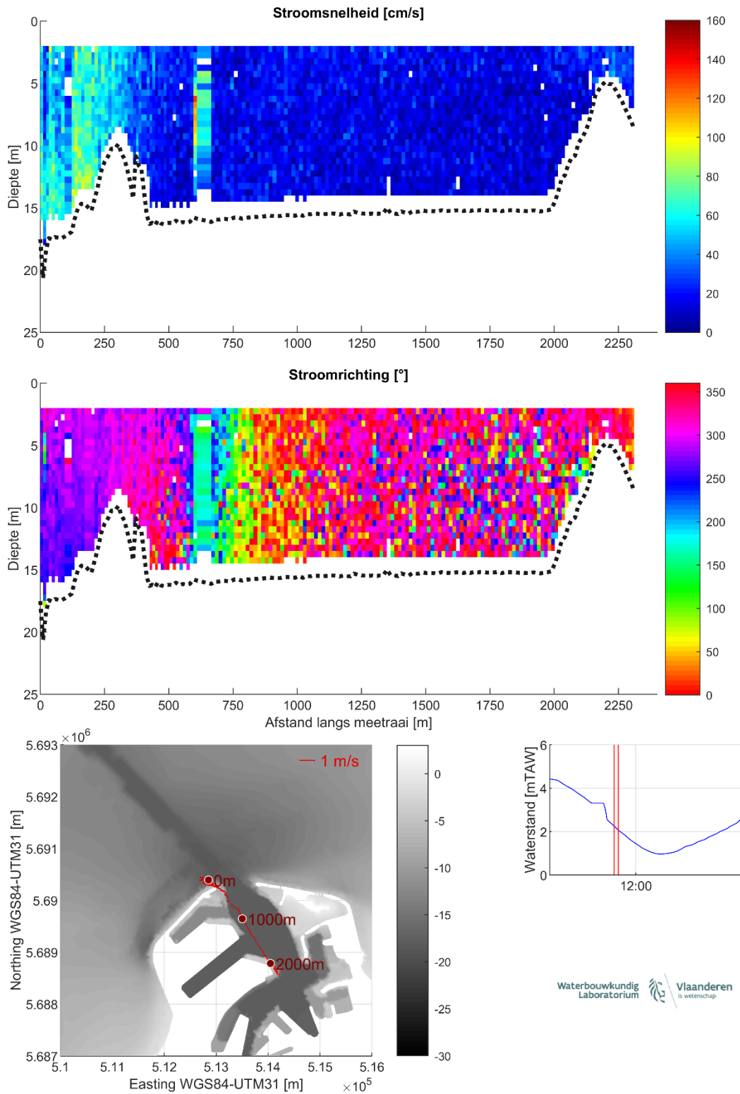
Figuur 16 – Stroomgegevens 08/08/2023 raai 11: snelheids grootte (top), -richting (midden) en diepte-gemiddelde vectoren (onder)
