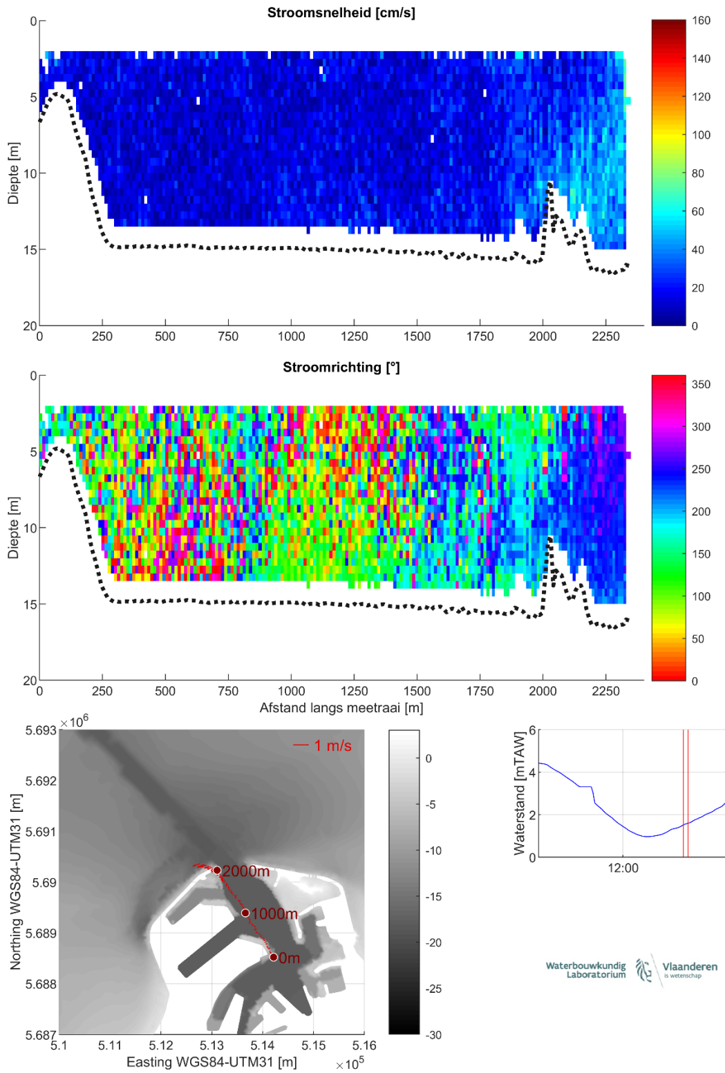
Figuur 33 – Stroomgegevens 08/08/2023 raai 28: snelheids grootte (top), -richting (midden) en diepte-gemiddelde vectoren (onder)
