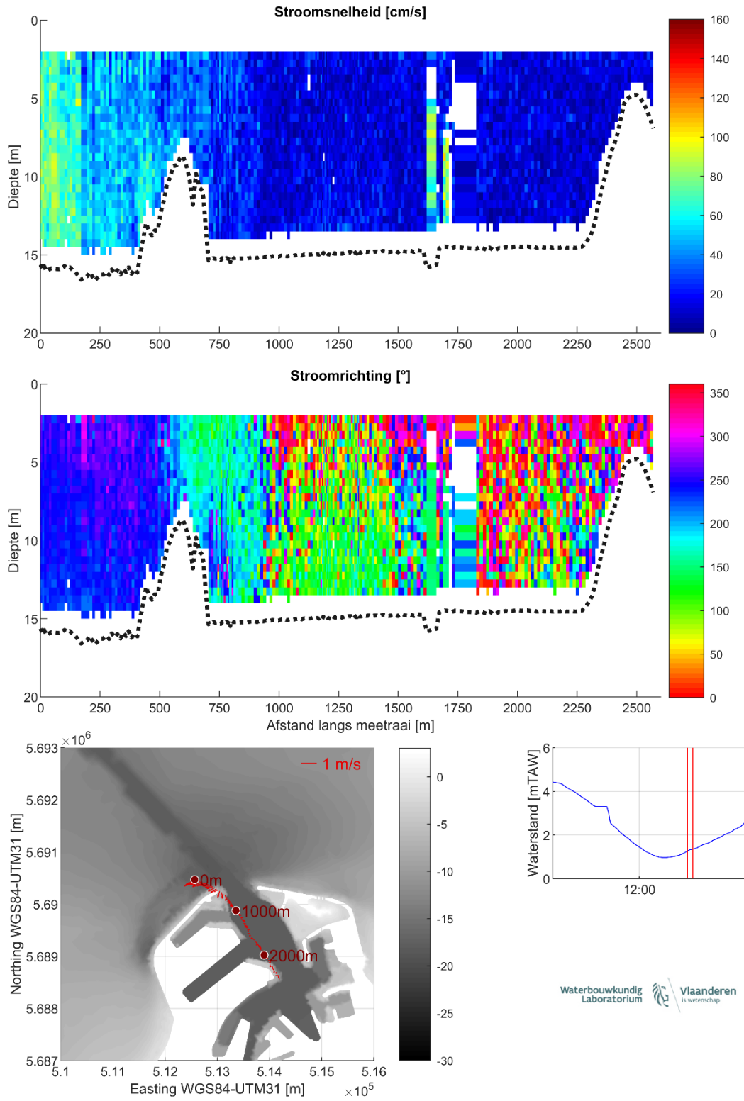
Figuur 30 – Stroomgegevens 08/08/2023 raai 25: snelheids grootte (top), -richting (midden) en diepte-gemiddelde vectoren (onder)
