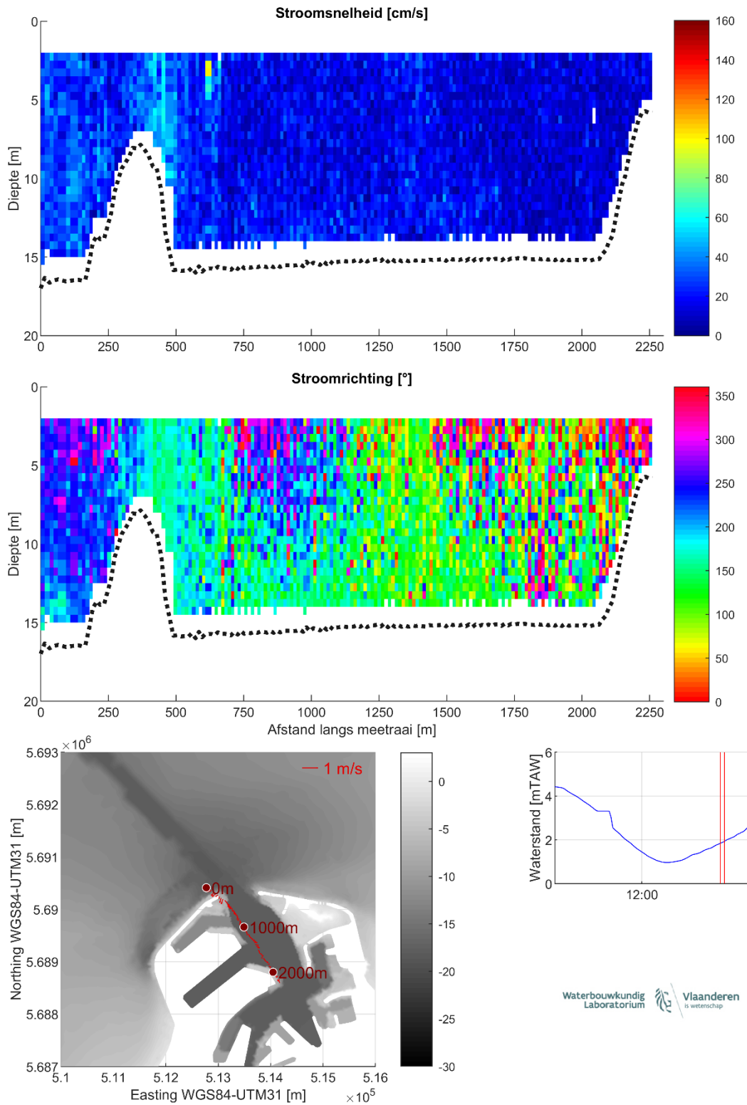
Figuur 36 – Stroomgegevens 08/08/2023 raai 31: snelheids grootte (top), -richting (midden) en diepte-gemiddelde vectoren (onder)
