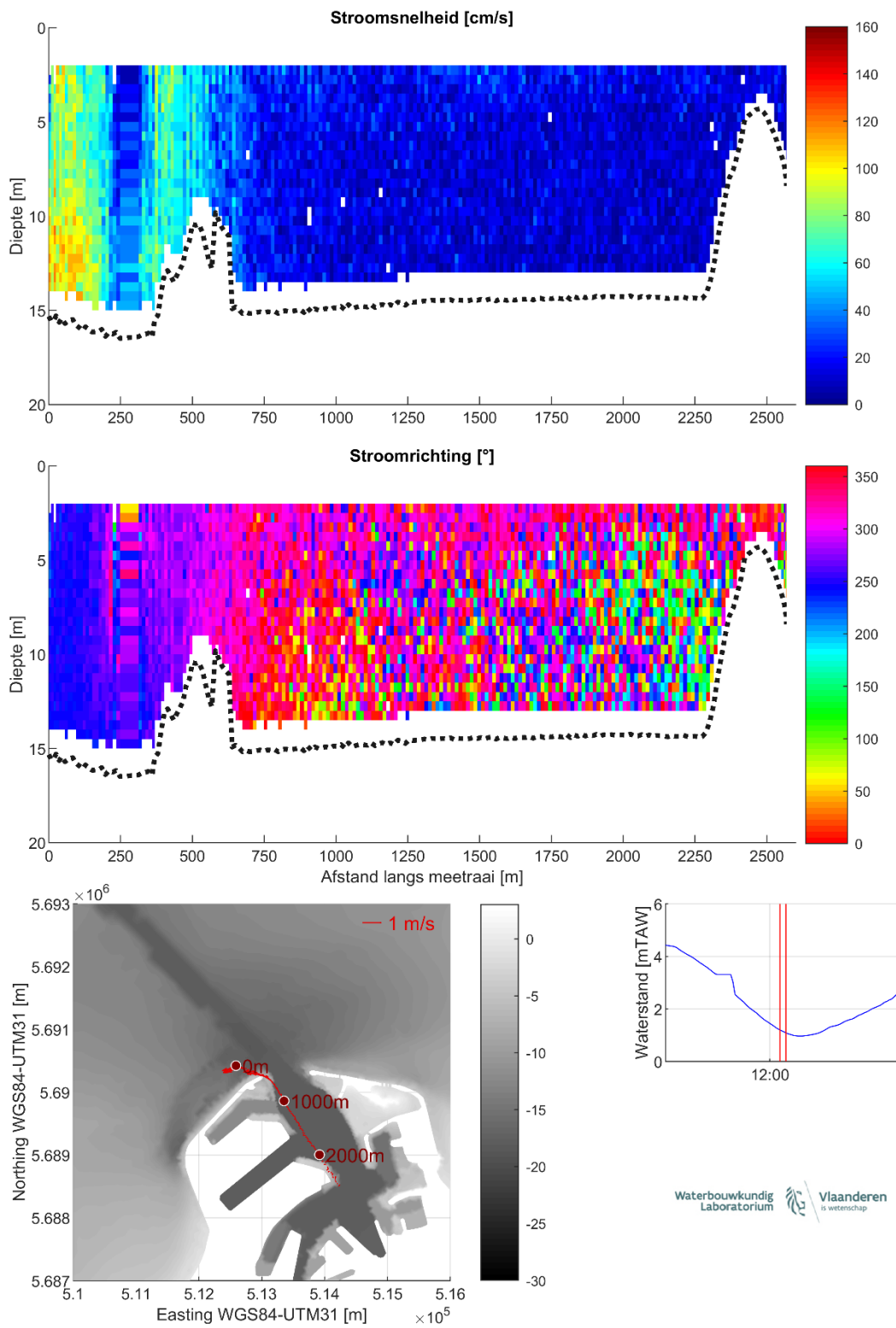
Figuur 21 – Stroomgegevens 08/08/2023 raai 16: snelheids grootte (top), -richting (midden) en diepte-gemiddelde vectoren (onder)
