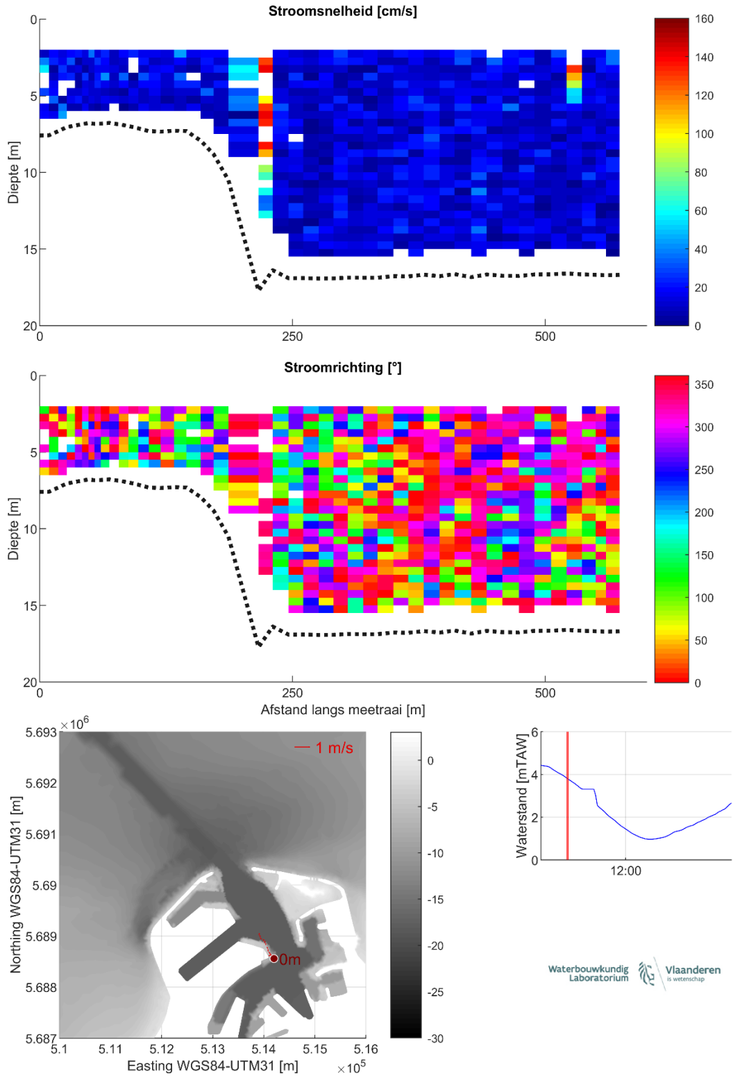
Figuur 8 – Stroomgegevens 08/08/2023 raai 3: snelheids grootte (top), -richting (midden) en diepte-gemiddelde vectoren (onder)
