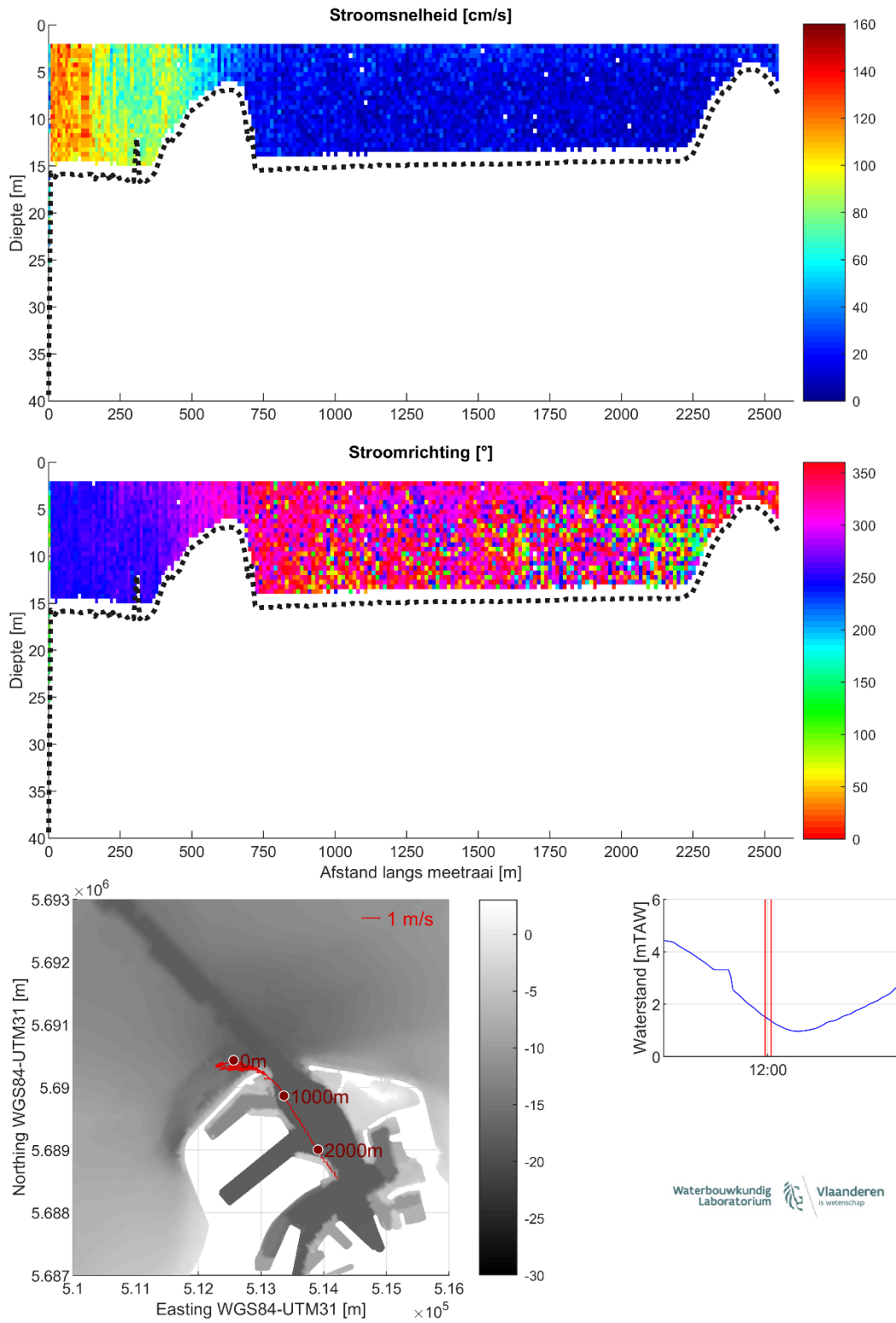
Figuur 20 – Stroomgegevens 08/08/2023 raai 15: snelheids grootte (top), -richting (midden) en diepte-gemiddelde vectoren (onder)
