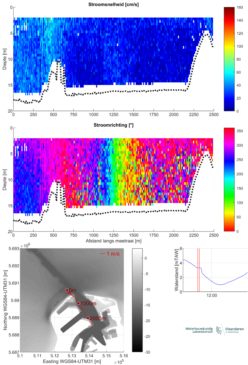
Figuur 12 – Stroomgegevens 08/08/2023 raai 7: snelheids grootte (top), -richting (midden) en diepte-gemiddelde vectoren (onder)
