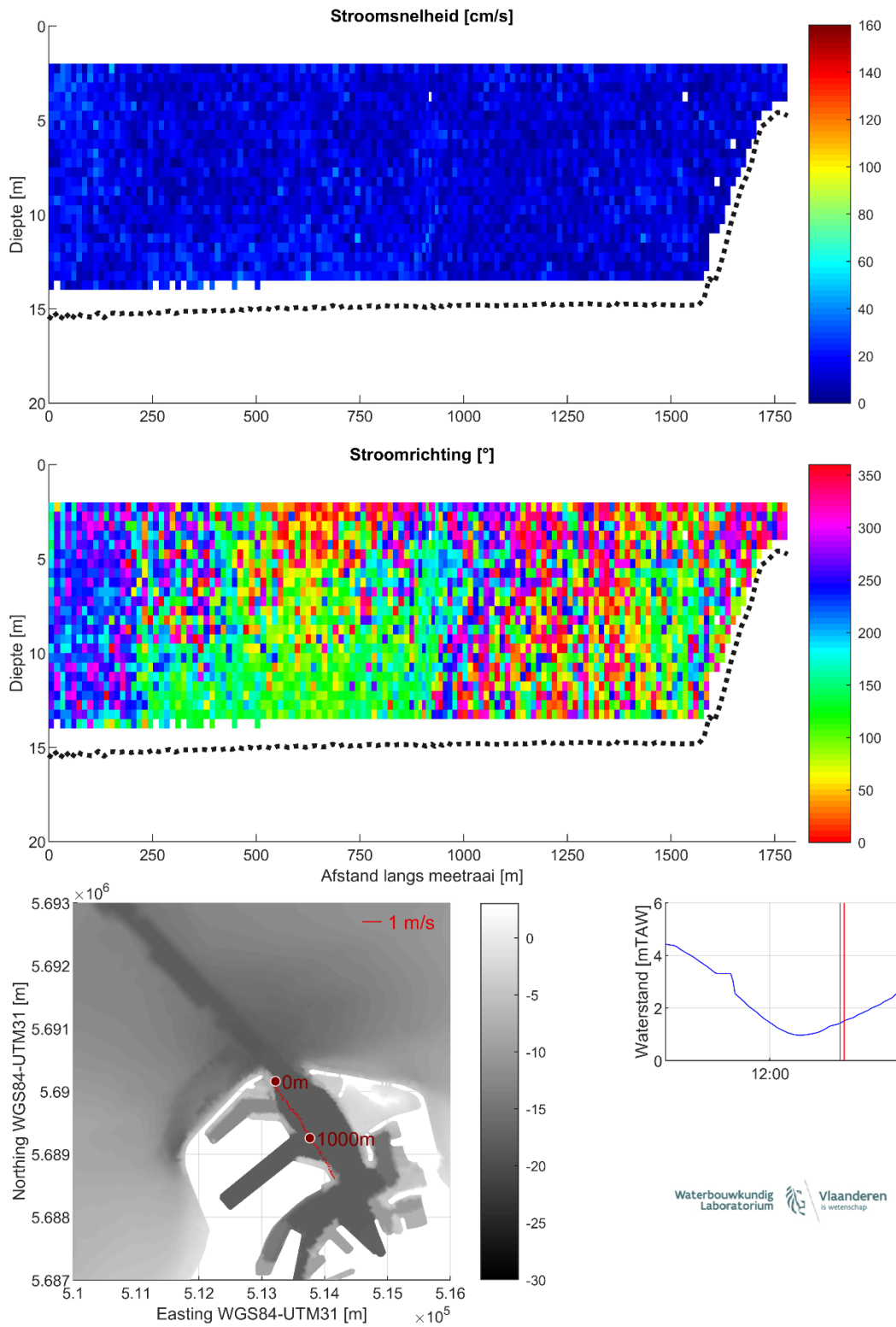
Figuur 32 – Stroomgegevens 08/08/2023 raai 27: snelheids grootte (top), -richting (midden) en diepte-gemiddelde vectoren (onder)
