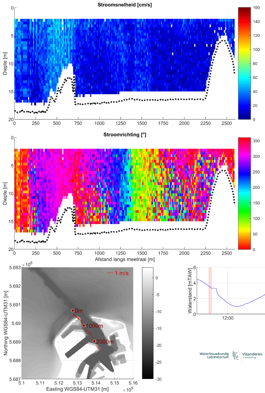
Figuur 10 – Stroomgegevens 08/08/2023 raai 5: snelheids grootte (top), -richting (midden) en diepte-gemiddelde vectoren (onder)
