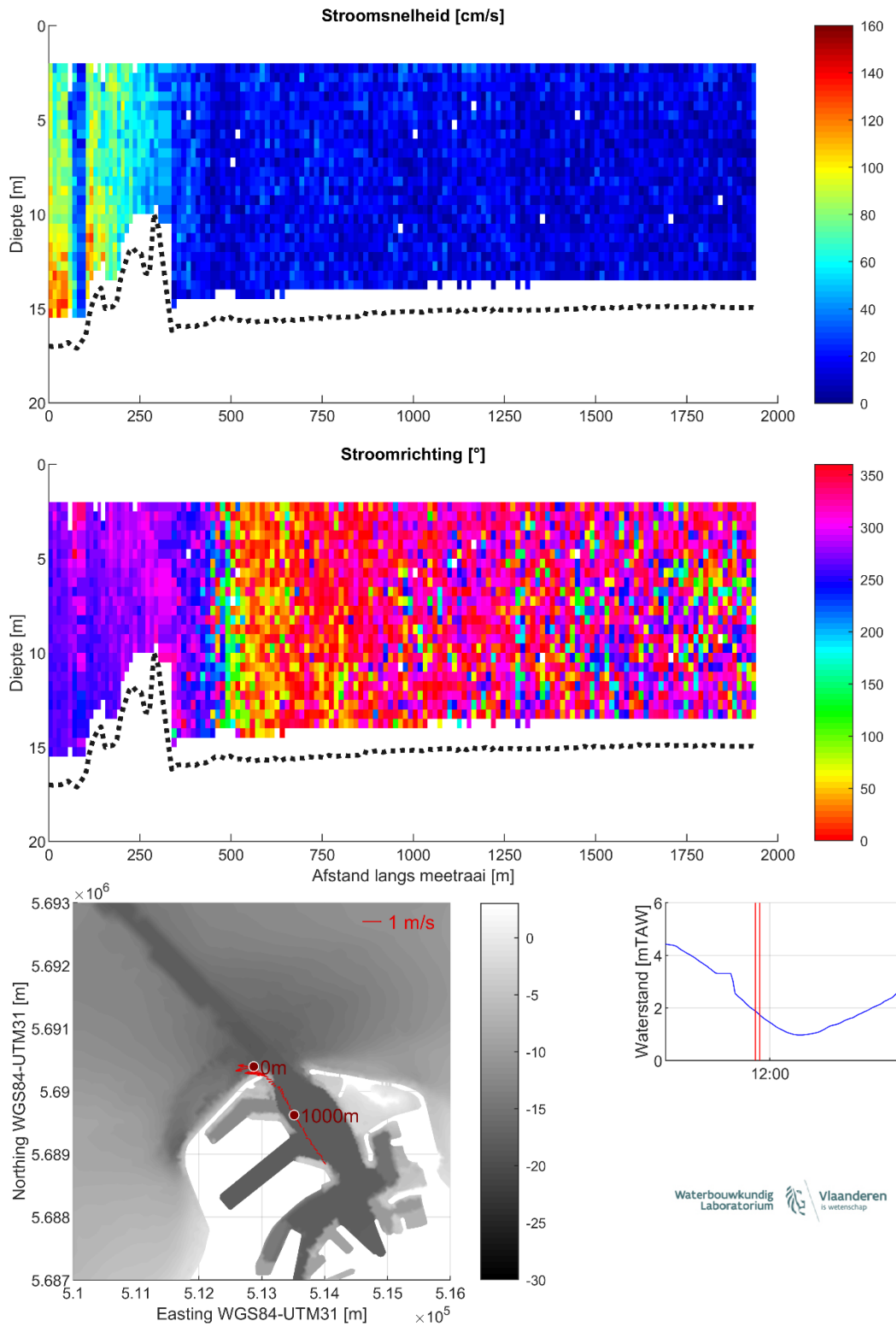
Figuur 18 – Stroomgegevens 08/08/2023 raai 13: snelheids grootte (top), -richting (midden) en diepte-gemiddelde vectoren (onder)
