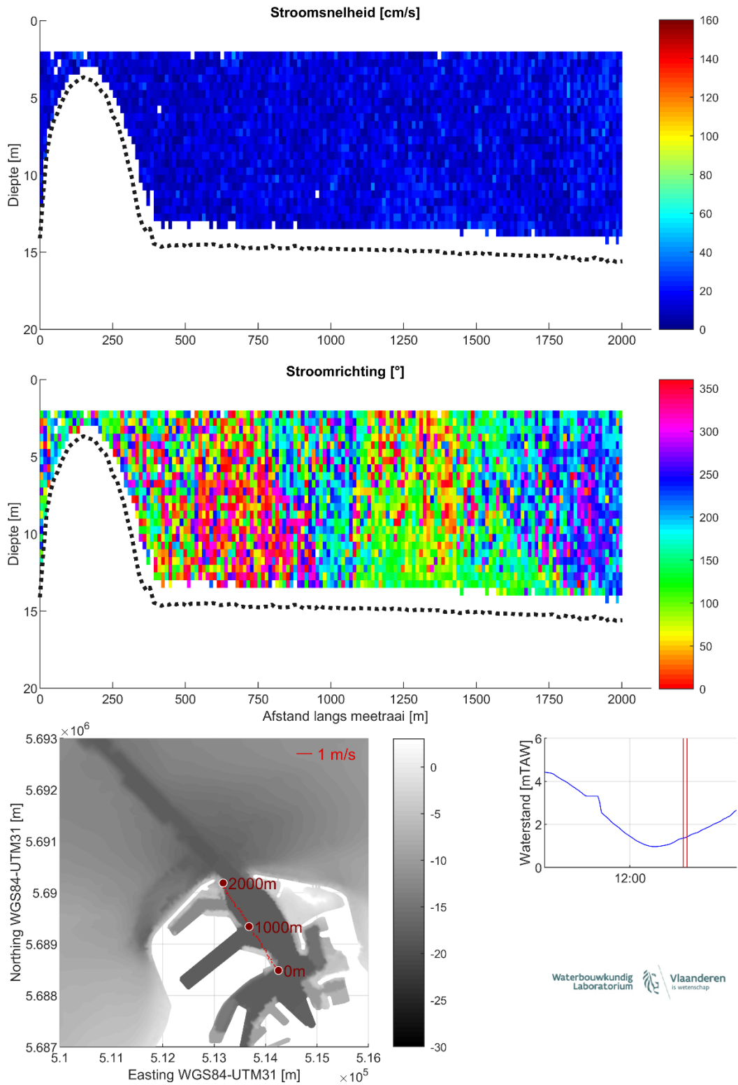
Figuur 31 – Stroomgegevens 08/08/2023 raai 26: snelheids grootte (top), -richting (midden) en diepte-gemiddelde vectoren (onder)
