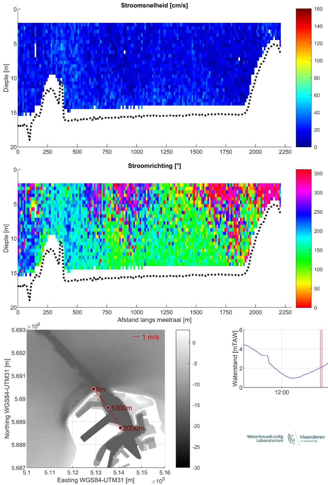
Figuur 38 – Stroomgegevens 08/08/2023 raai 33: snelheids grootte (top), -richting (midden) en diepte-gemiddelde vectoren (onder)
