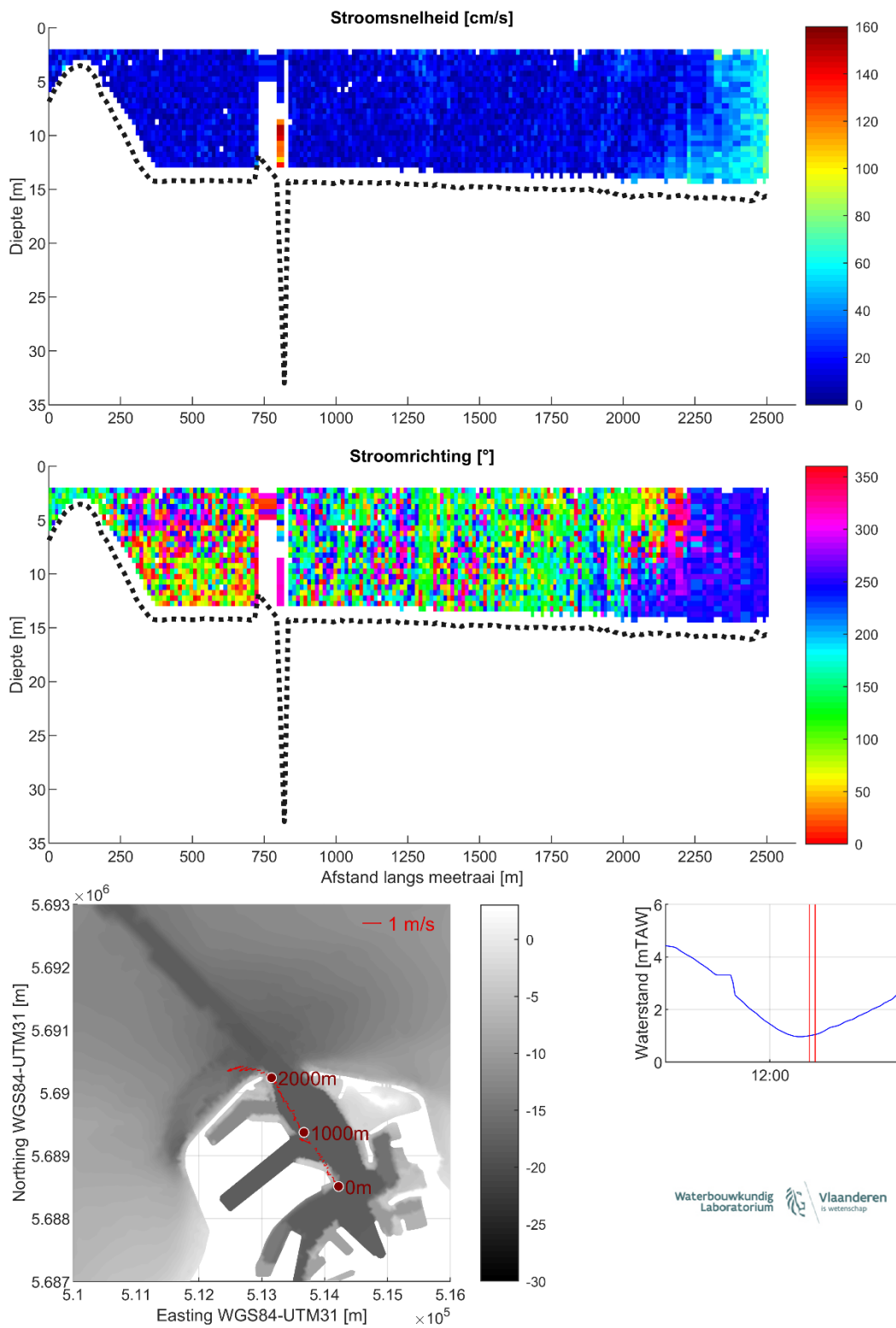
Figuur 27 – Stroomgegevens 08/08/2023 raai 22: snelheids grootte (top), -richting (midden) en diepte-gemiddelde vectoren (onder)
