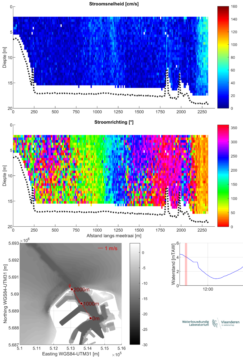
Figuur 6 – Stroomgegevens 08/08/2023 raai 1: snelheids grootte (top), -richting (midden) en diepte-gemiddelde vectoren (onder)
