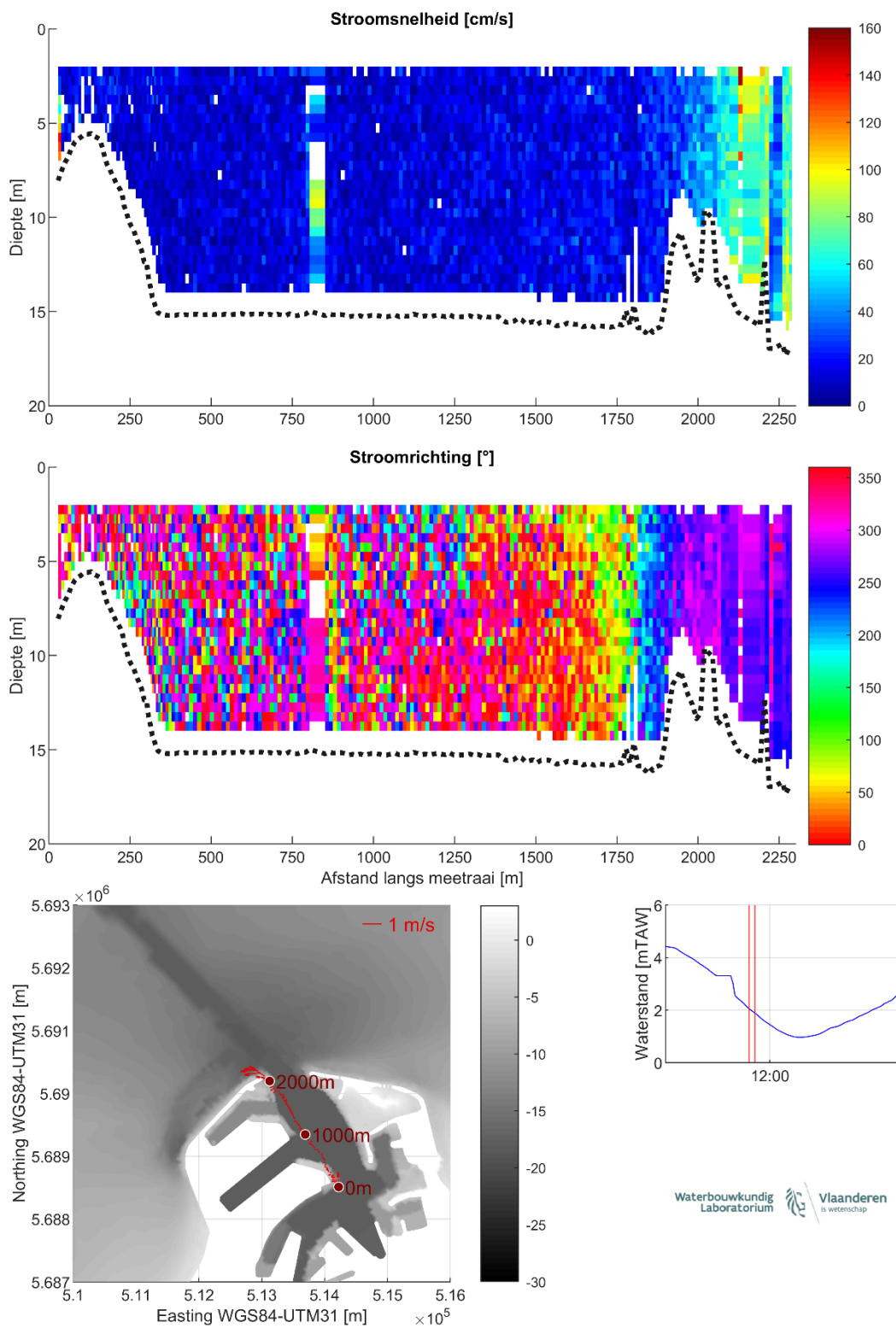
Figuur 17 – Stroomgegevens 08/08/2023 raai 12: snelheids grootte (top), -richting (midden) en diepte-gemiddelde vectoren (onder)
