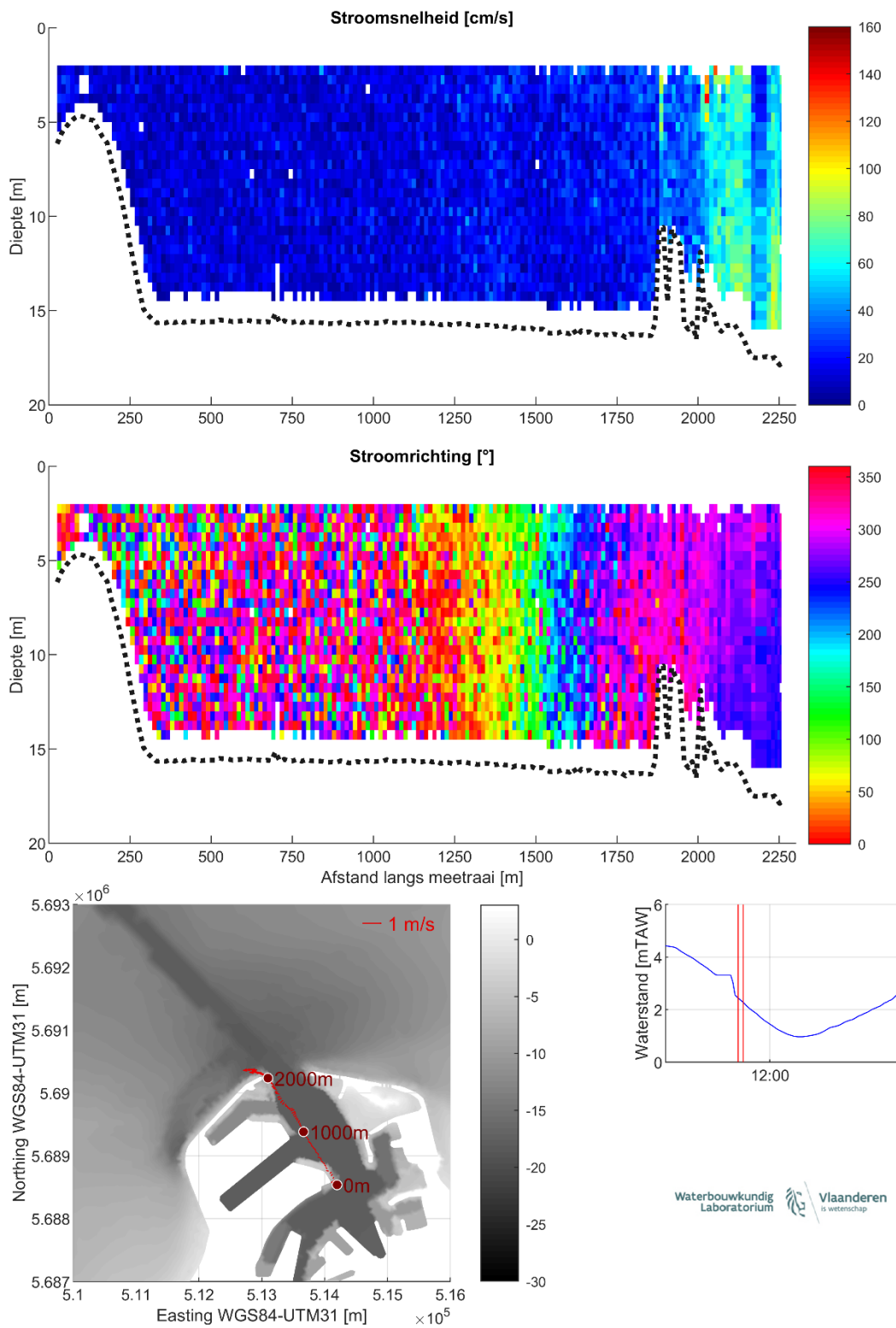
Figuur 15 – Stroomgegevens 08/08/2023 raai 10: snelheids grootte (top), -richting (midden) en diepte-gemiddelde vectoren (onder)
