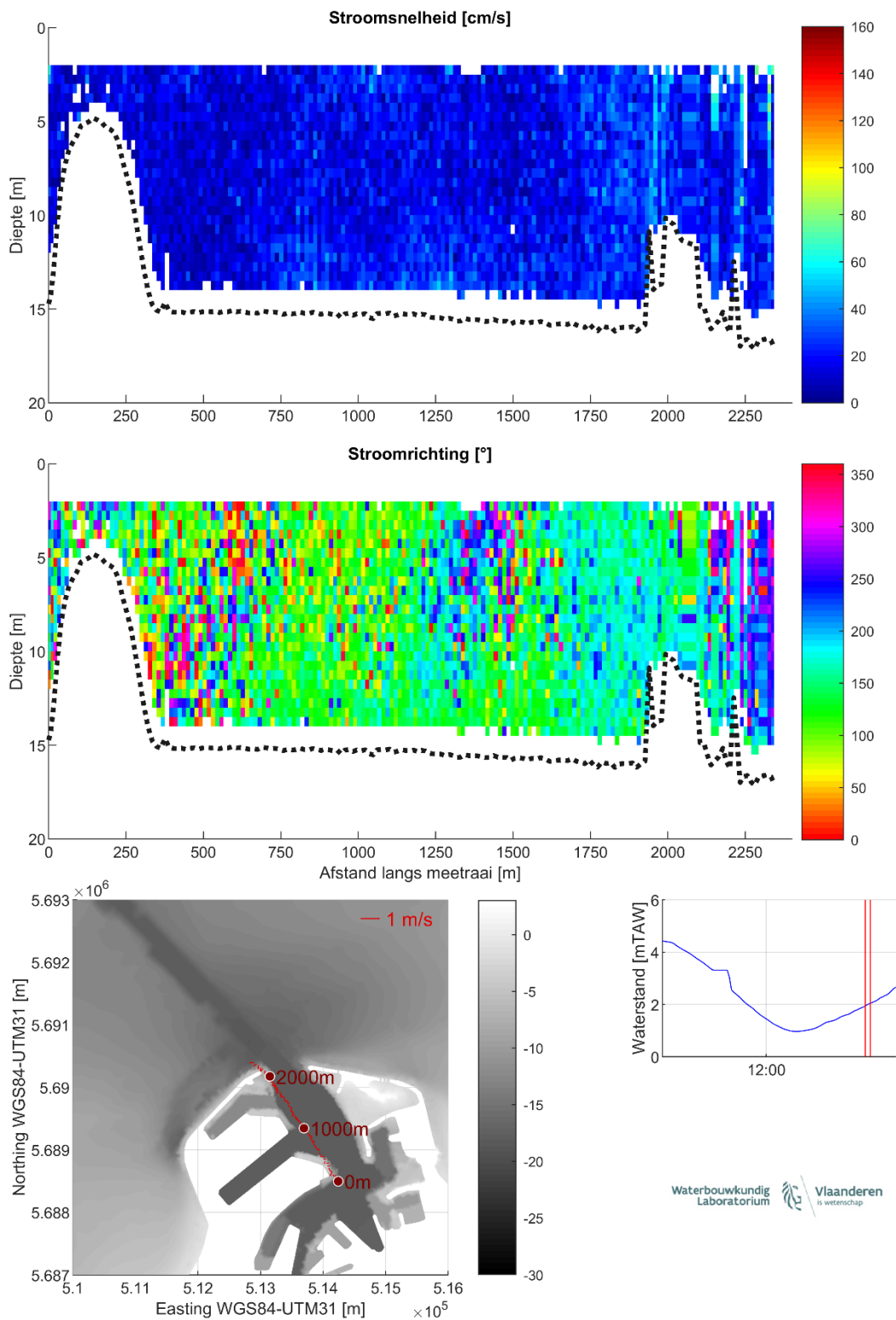
Figuur 37 – Stroomgegevens 08/08/2023 raai 32: snelheids grootte (top), -richting (midden) en diepte-gemiddelde vectoren (onder)
