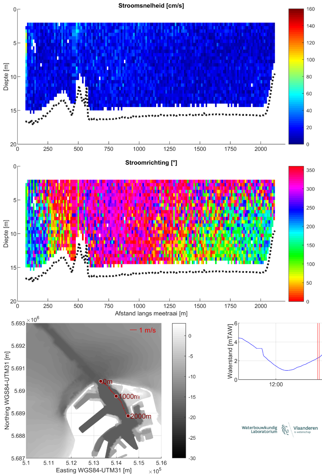
Figuur 40 – Stroomgegevens 08/08/2023 raai 35: snelheids grootte (top), -richting (midden) en diepte-gemiddelde vectoren (onder)
