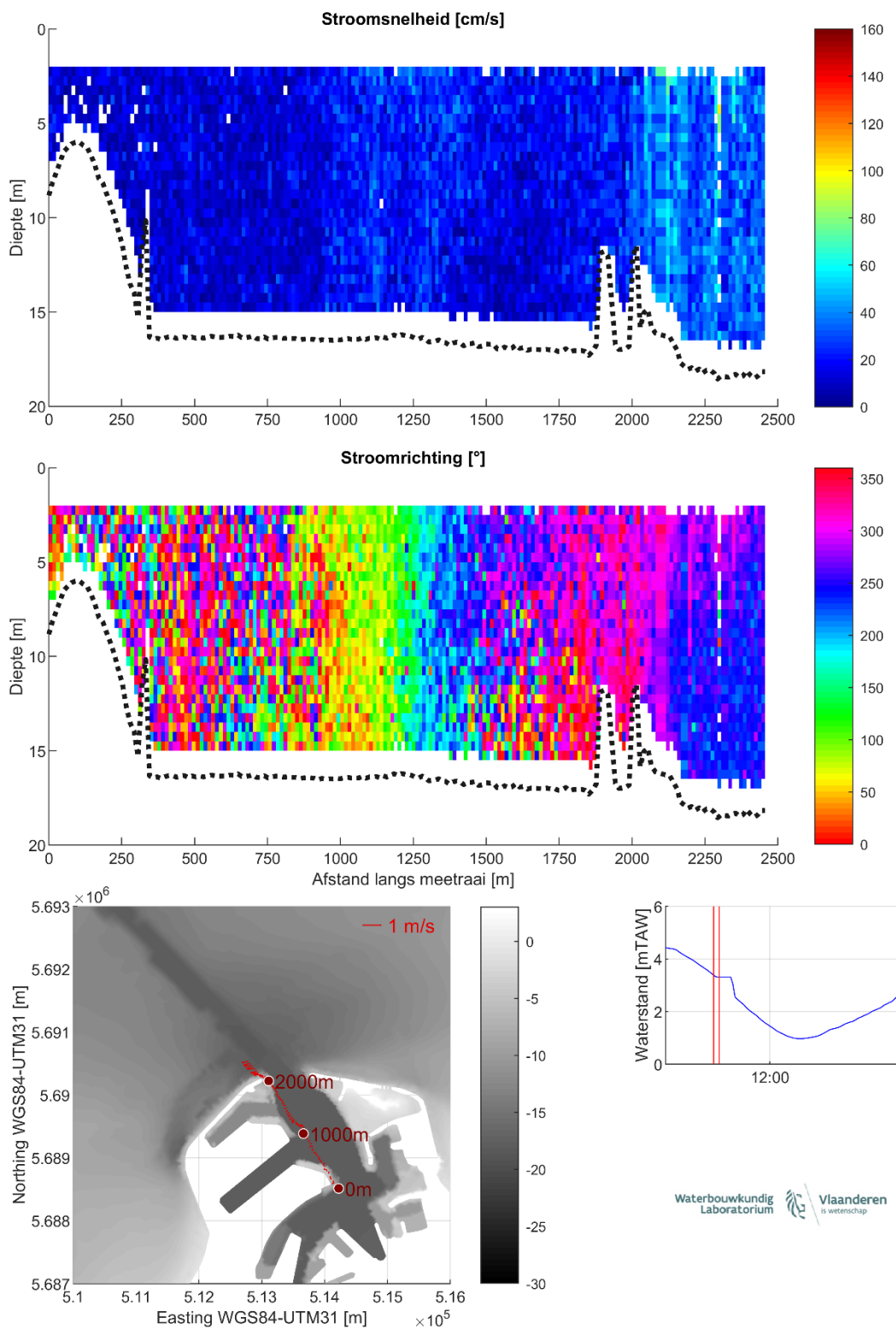
Figuur 11 – Stroomgegevens 08/08/2023 raai 6: snelheids grootte (top), -richting (midden) en diepte-gemiddelde vectoren (onder)
