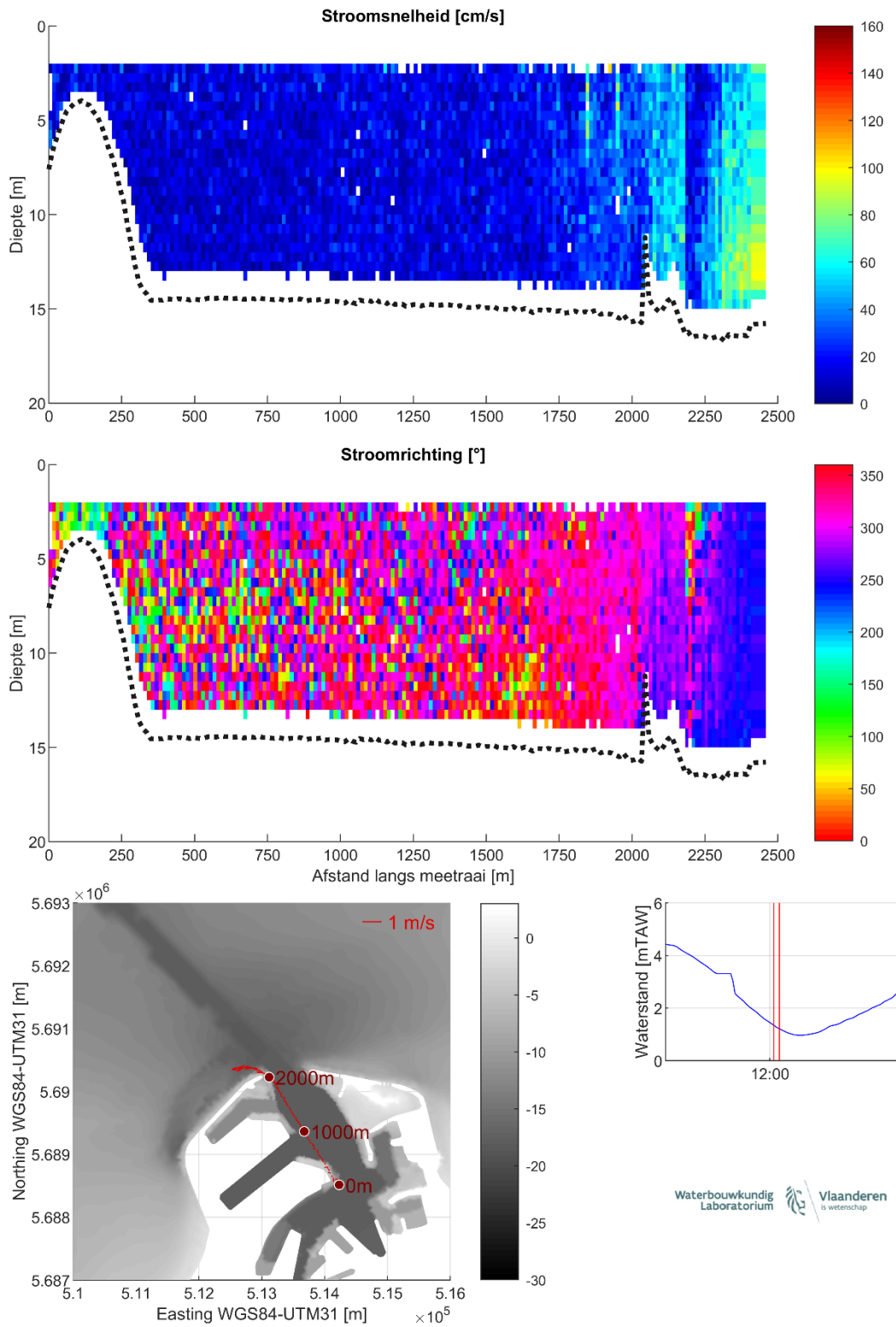
Figuur 23 – Stroomgegevens 08/08/2023 raai 18: snelheids grootte (top), -richting (midden) en diepte-gemiddelde vectoren (onder)
