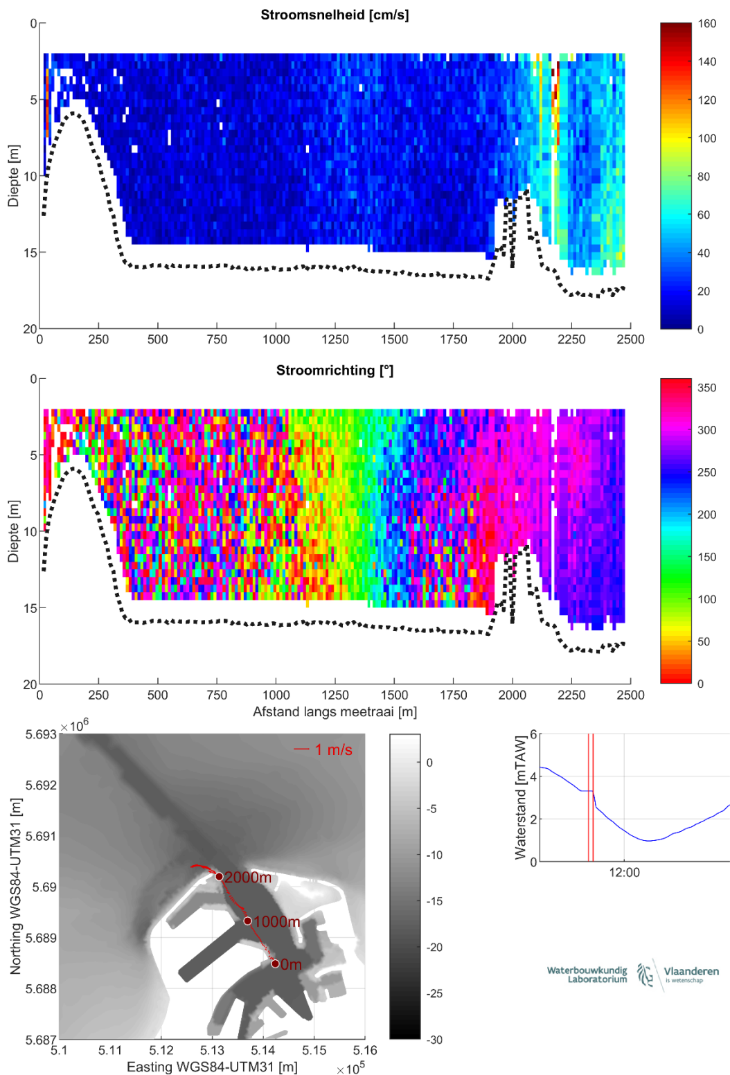
Figuur 13 – Stroomgegevens 08/08/2023 raai 8: snelheids grootte (top), -richting (midden) en diepte-gemiddelde vectoren (onder)
