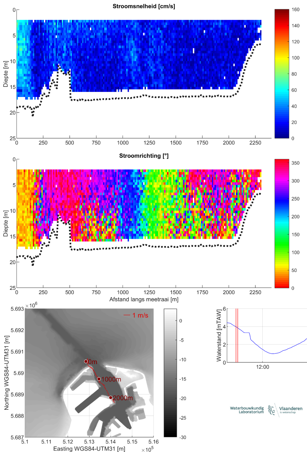
Figuur 7 – Stroomgegevens 08/08/2023 raai 2: snelheids grootte (top), -richting (midden) en diepte-gemiddelde vectoren (onder)
