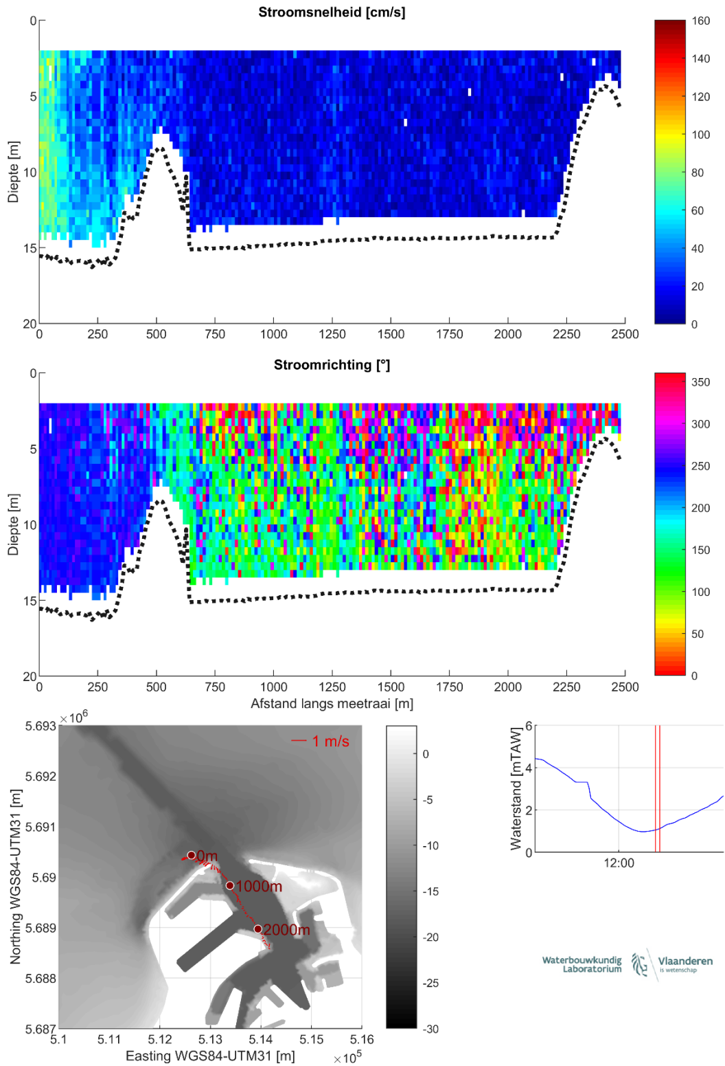
Figuur 28 – Stroomgegevens 08/08/2023 raai 23: snelheids grootte (top), -richting (midden) en diepte-gemiddelde vectoren (onder)
