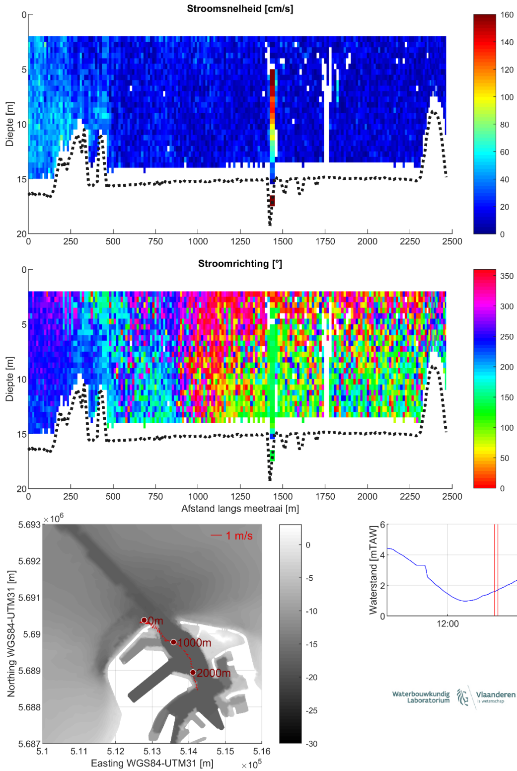
Figuur 34 – Stroomgegevens 08/08/2023 raai 29: snelheids grootte (top), -richting (midden) en diepte-gemiddelde vectoren (onder)
