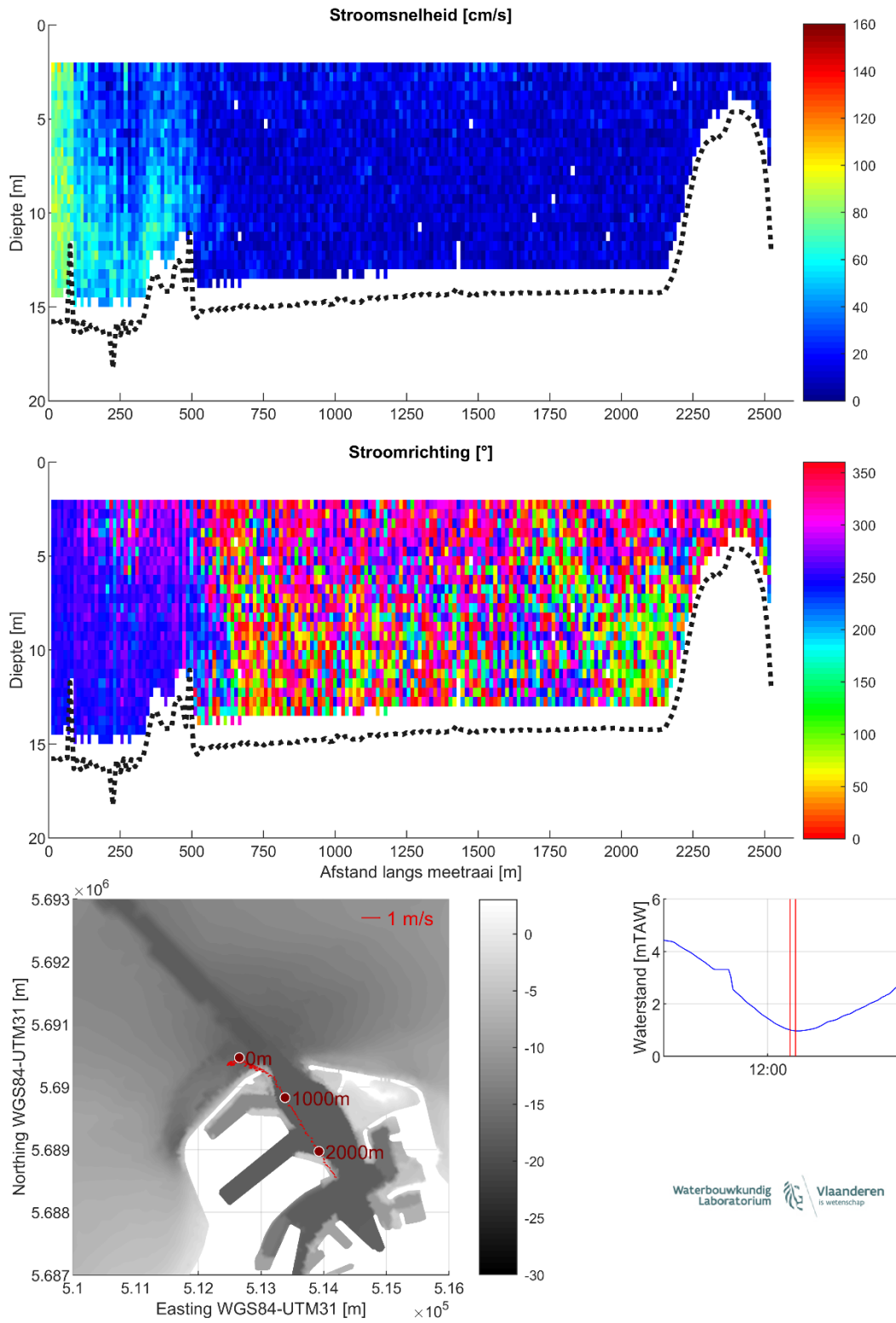
Figuur 24 – Stroomgegevens 08/08/2023 raai 19: snelheids grootte (top), -richting (midden) en diepte-gemiddelde vectoren (onder)
