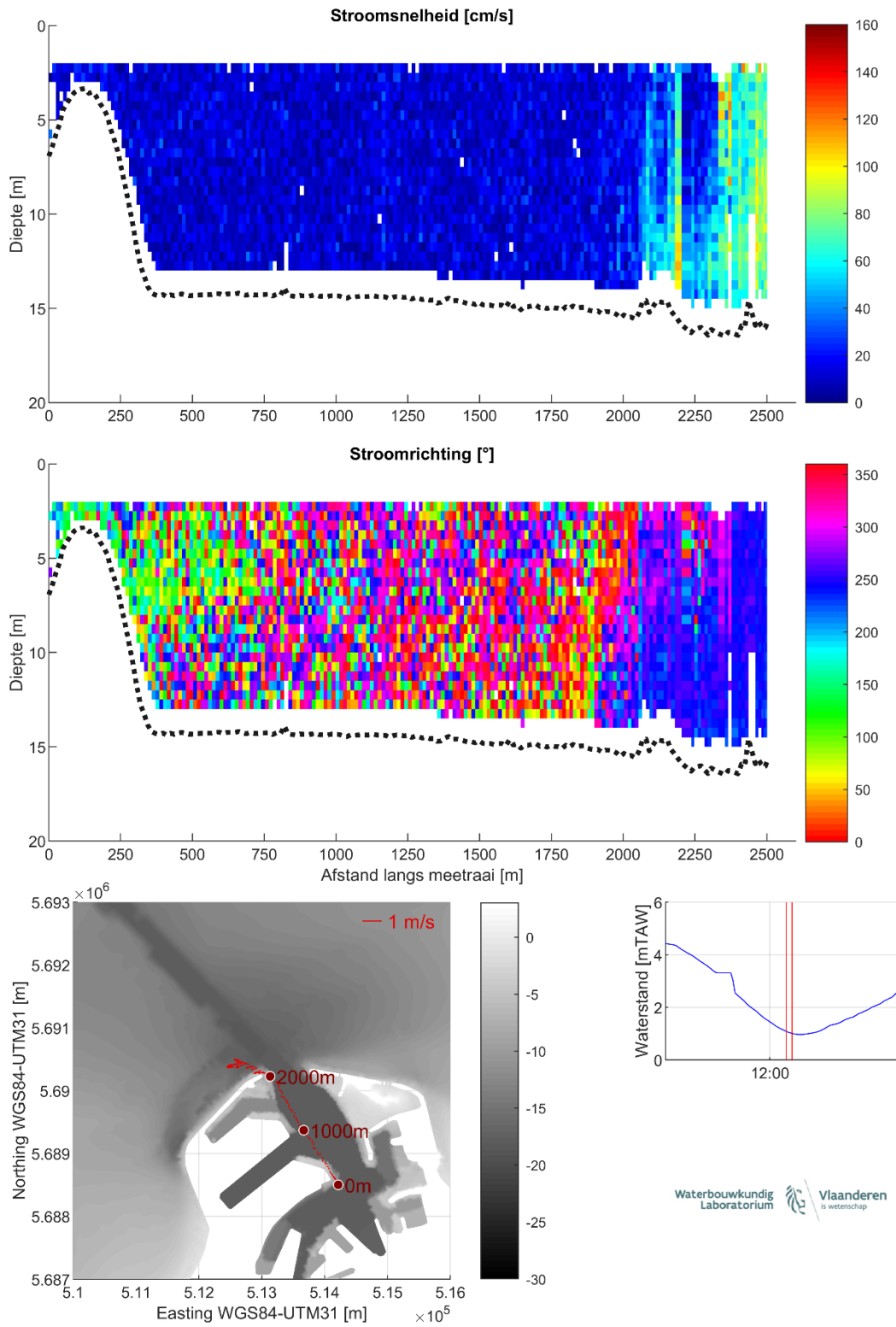
Figuur 22 – Stroomgegevens 08/08/2023 raai 17: snelheids grootte (top), -richting (midden) en diepte-gemiddelde vectoren (onder)
