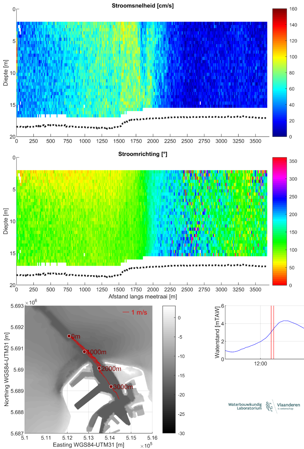
Figuur 23 – Stroomgegevens 16/08/2023 raai 18: snelheids grootte (top), -richting (midden) en diepte-gemiddelde vectoren (onder)
