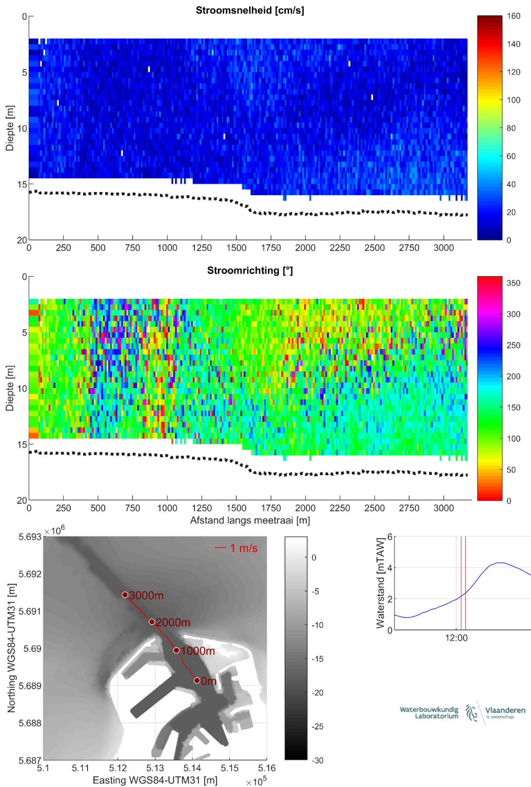
Figuur 20 – Stroomgegevens 16/08/2023 raai 15: snelheids grootte (top), -richting (midden) en diepte-gemiddelde vectoren (onder)
