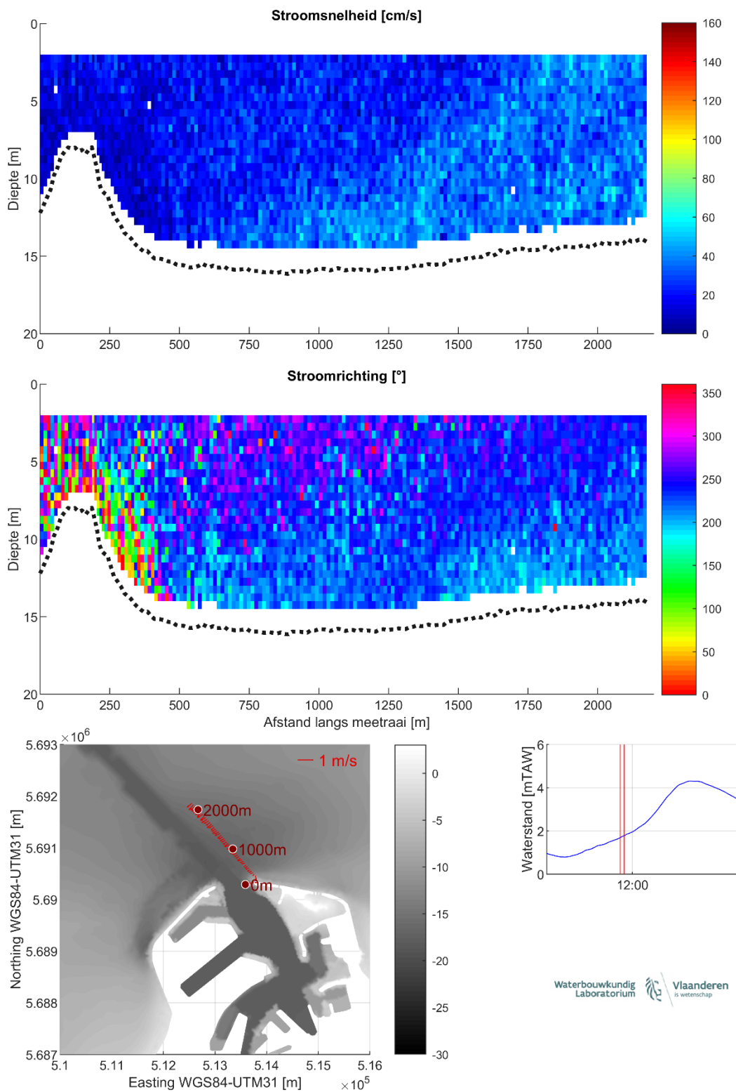
Figuur 16 – Stroomgegevens 16/08/2023 raai 11: snelheids grootte (top), -richting (midden) en diepte-gemiddelde vectoren (onder)
