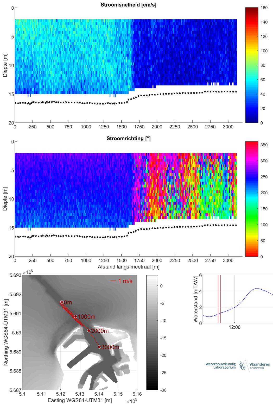
Figuur 11 – Stroomgegevens 16/08/2023 raai 6: snelheids grootte (top), -richting (midden) en diepte-gemiddelde vectoren (onder)
