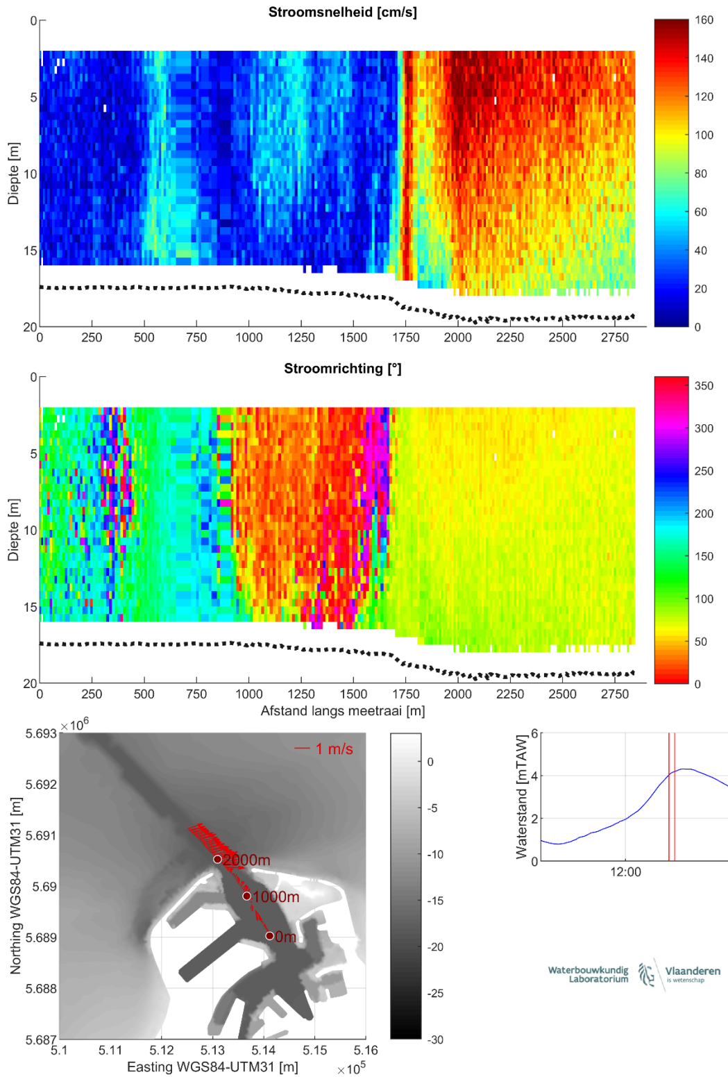
Figuur 26 – Stroomgegevens 16/08/2023 raai 21: snelheids grootte (top), -richting (midden) en diepte-gemiddelde vectoren (onder)
