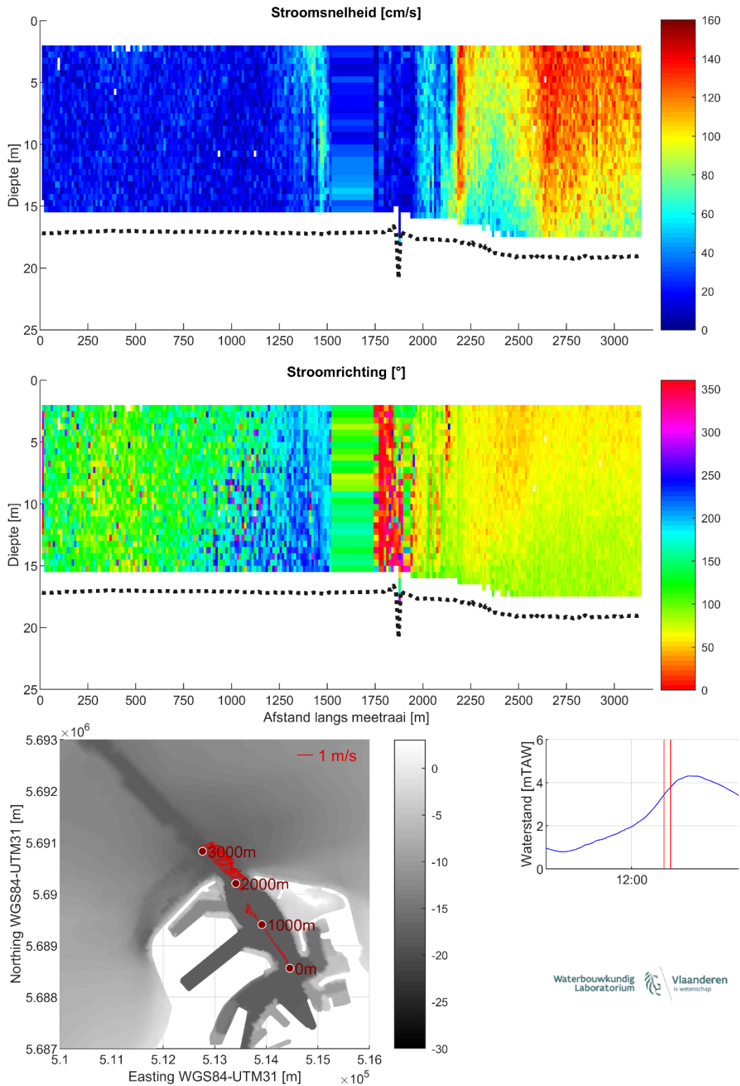
Figuur 24 – Stroomgegevens 16/08/2023 raai 19: snelheids grootte (top), -richting (midden) en diepte-gemiddelde vectoren (onder)
