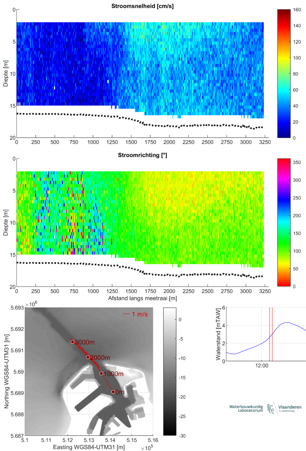
Figuur 22 – Stroomgegevens 16/08/2023 raai 17: snelheids grootte (top), -richting (midden) en diepte-gemiddelde vectoren (onder)
