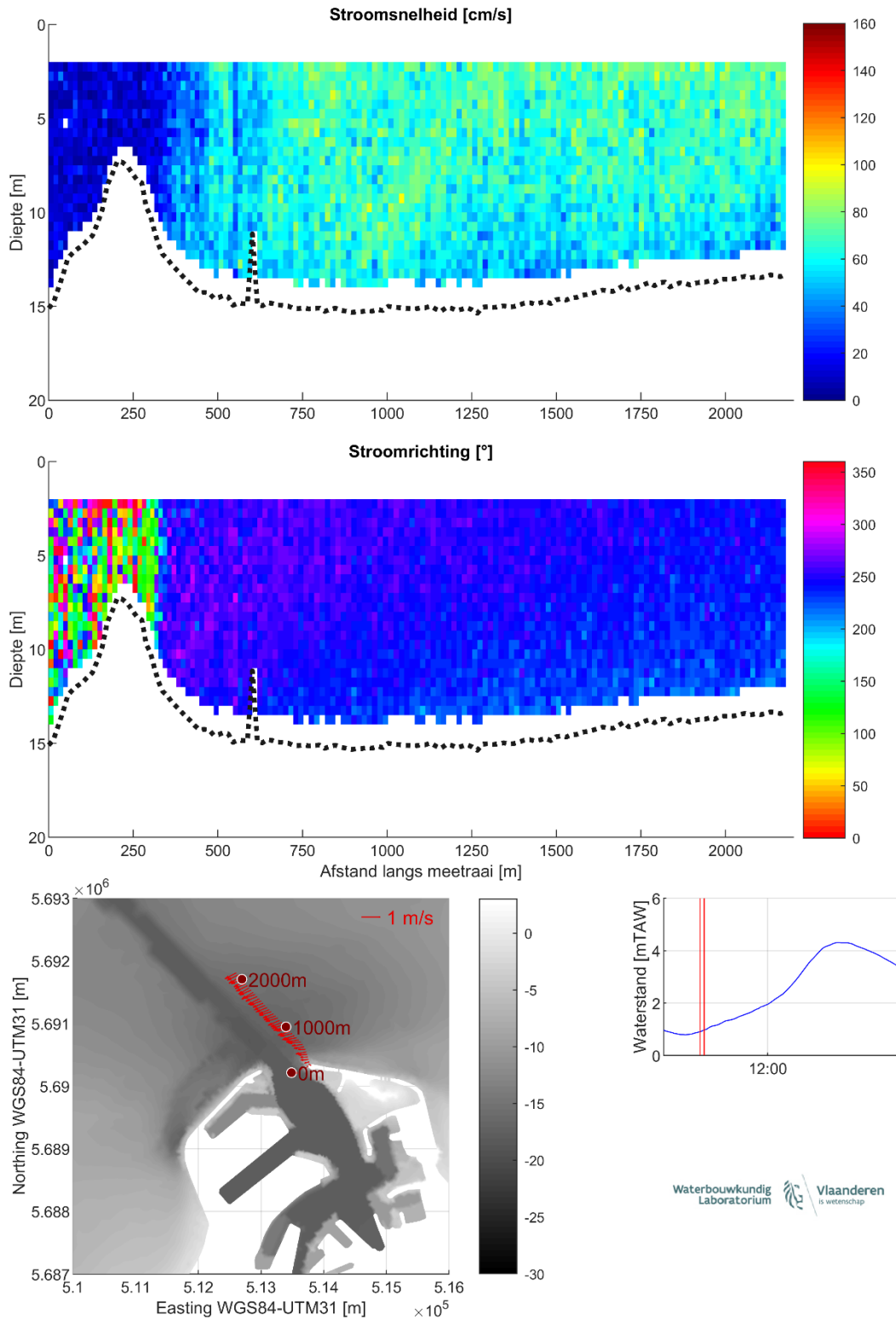
Figuur 8 – Stroomgegevens 16/08/2023 raai 3: snelheidsgrootte (top), -richting (midden) en diepte-gemiddelde vectoren (onder)
