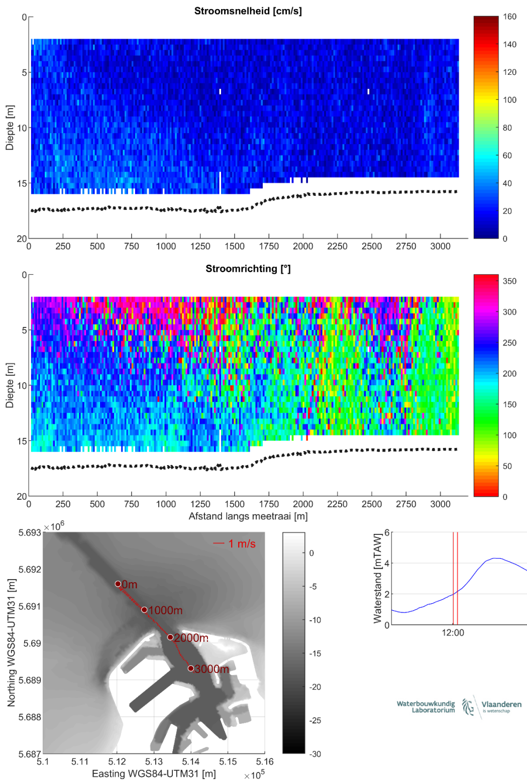
Figuur 19 – Stroomgegevens 16/08/2023 raai 14: snelheids grootte (top), -richting (midden) en diepte-gemiddelde vectoren (onder)
