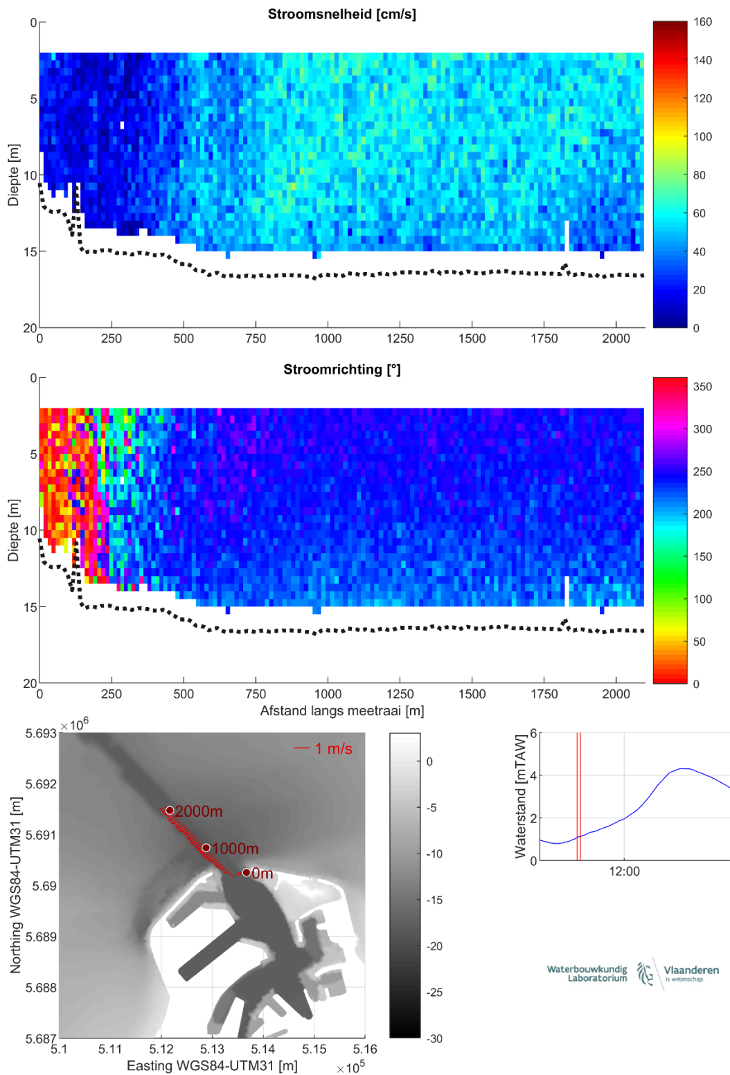
Figuur 10 – Stroomgegevens 16/08/2023 raai 5: snelheids grootte (top), -richting (midden) en diepte-gemiddelde vectoren (onder)
