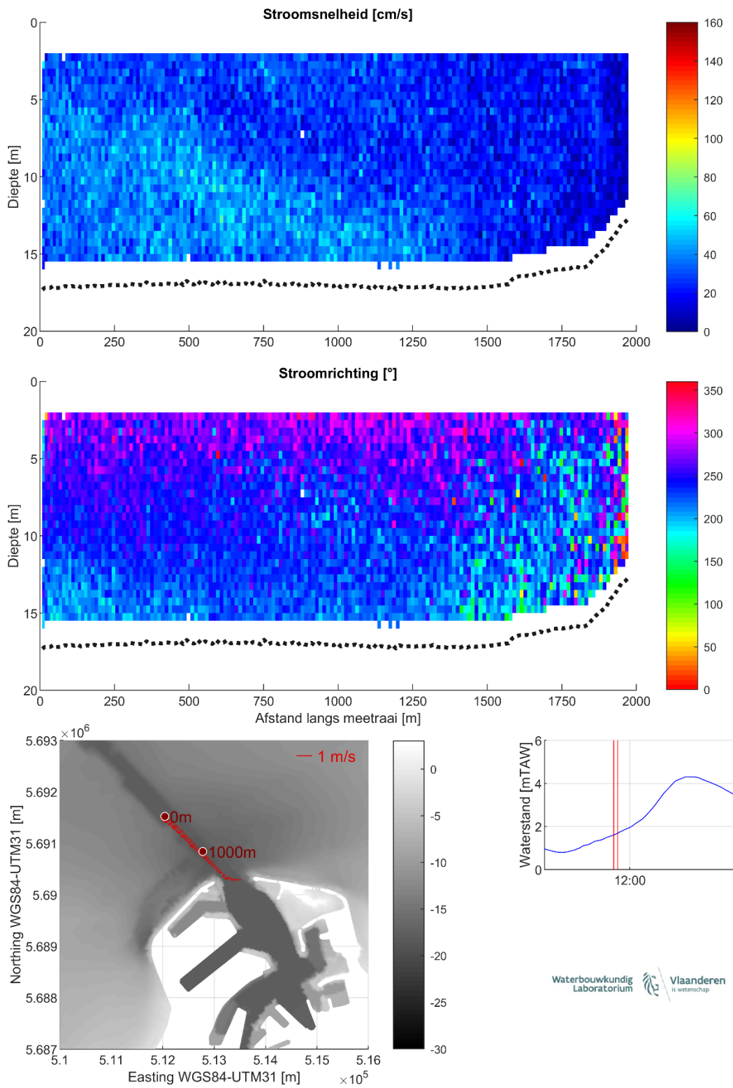
Figuur 15 – Stroomgegevens 16/08/2023 raai 10: snelheids grootte (top), -richting (midden) en diepte-gemiddelde vectoren (onder)
