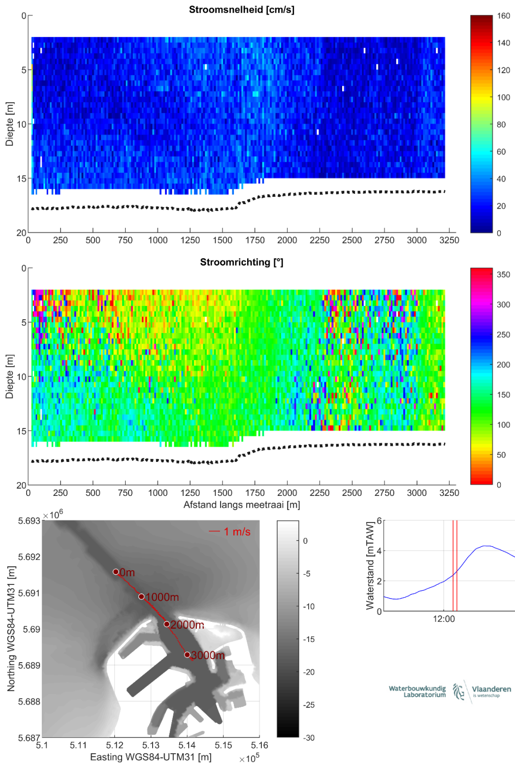
Figuur 21 – Stroomgegevens 16/08/2023 raai 16: snelheids grootte (top), -richting (midden) en diepte-gemiddelde vectoren (onder)
