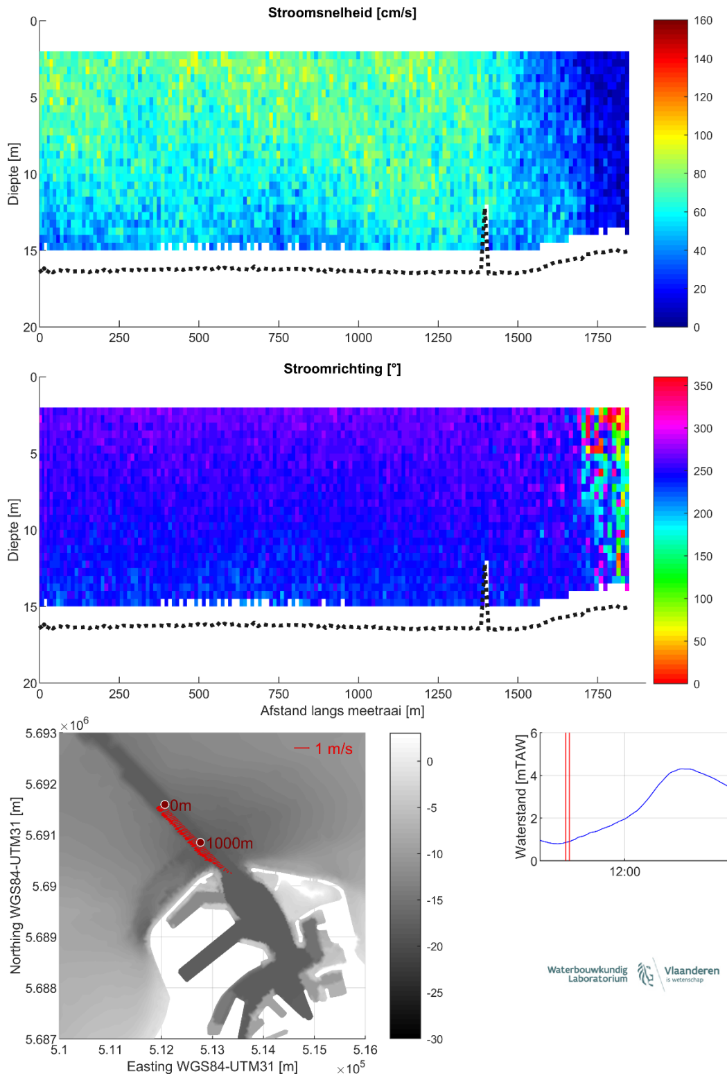
Figuur 7 – Stroomgegevens 16/08/2023 raai 2: snelheids grootte (top), -richting (midden) en diepte-gemiddelde vectoren (onder)
