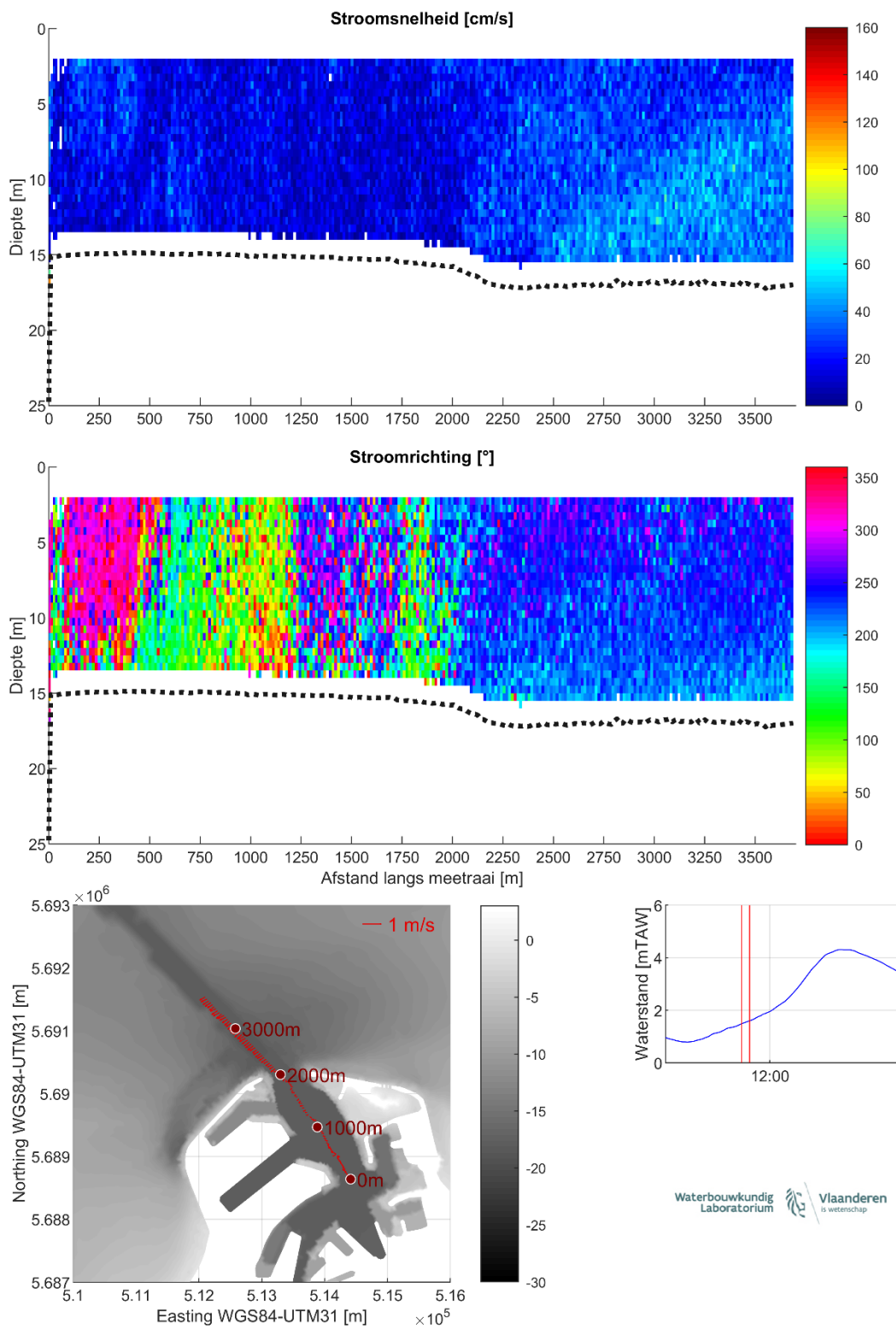
Figuur 14 – Stroomgegevens 16/08/2023 raai 9: snelheids grootte (top), -richting (midden) en diepte-gemiddelde vectoren (onder)
