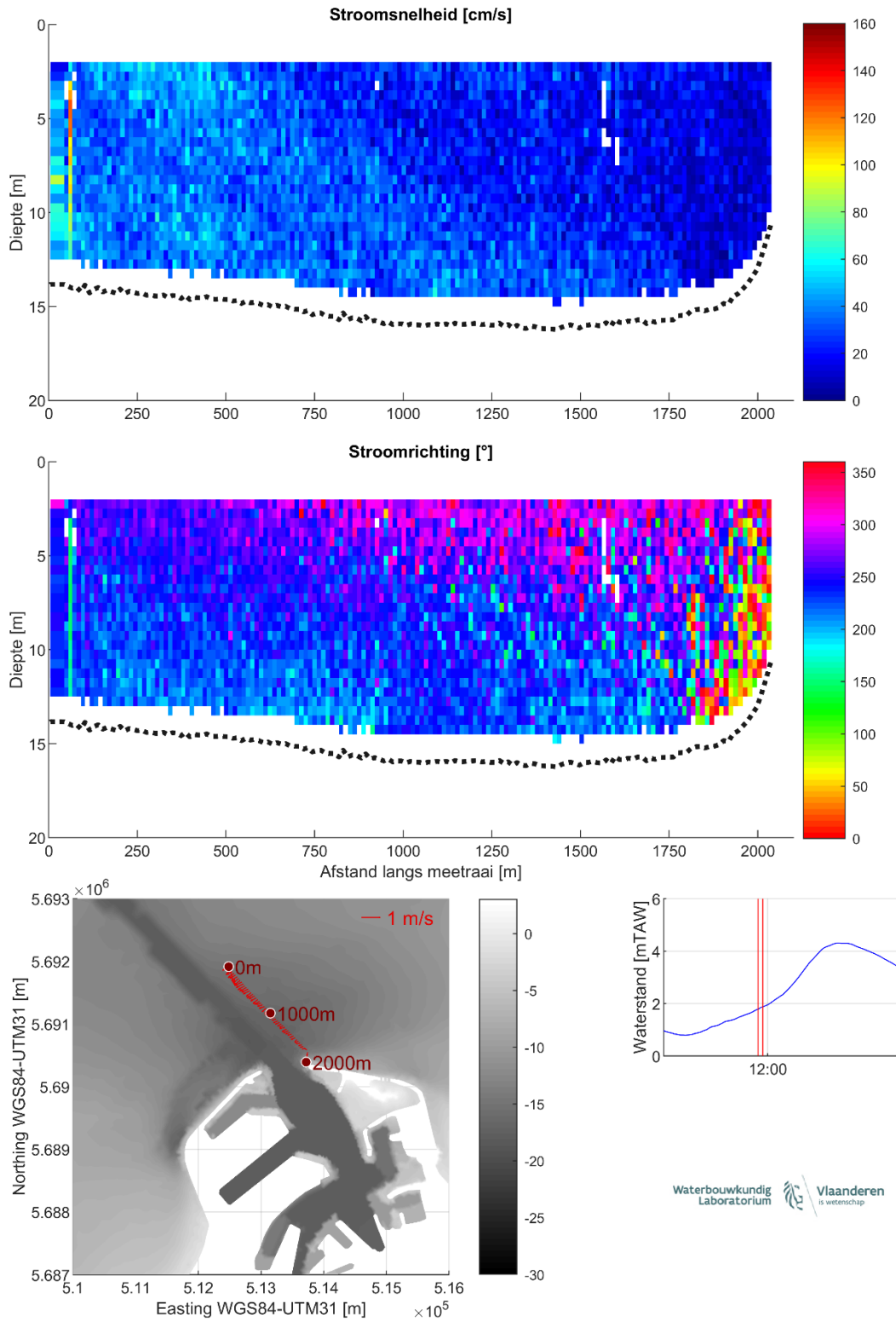
Figuur 17 – Stroomgegevens 16/08/2023 raai 12: snelheids grootte (top), -richting (midden) en diepte-gemiddelde vectoren (onder)
