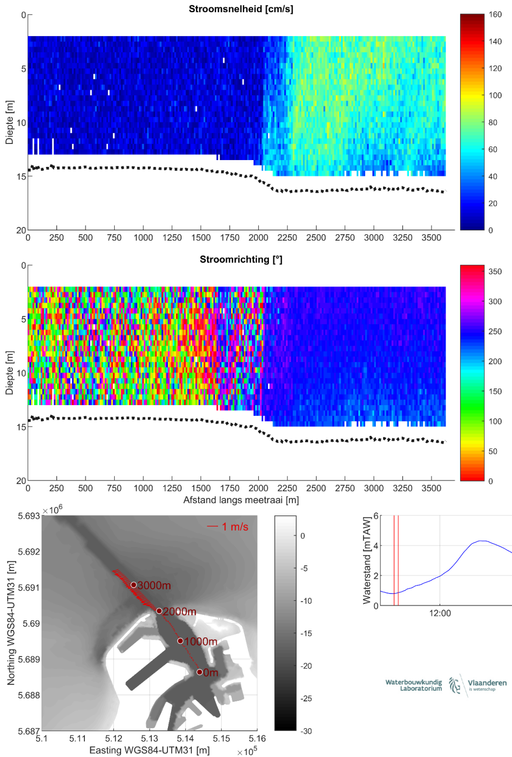
Figuur 6 – Stroomgegevens 16/08/2023 raai 1: snelheidsgrootte (top), -richting (midden) en diepte-gemiddelde vectoren (onder)
