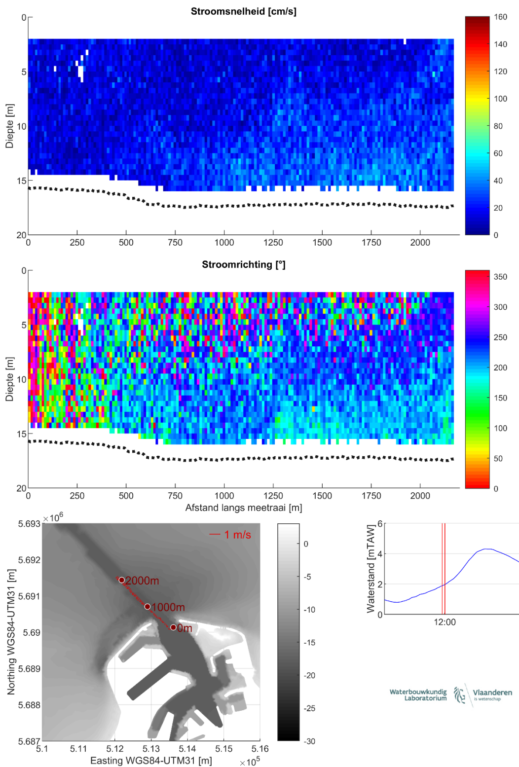
Figuur 18 – Stroomgegevens 16/08/2023 raai 13: snelheids grootte (top), -richting (midden) en diepte-gemiddelde vectoren (onder)
