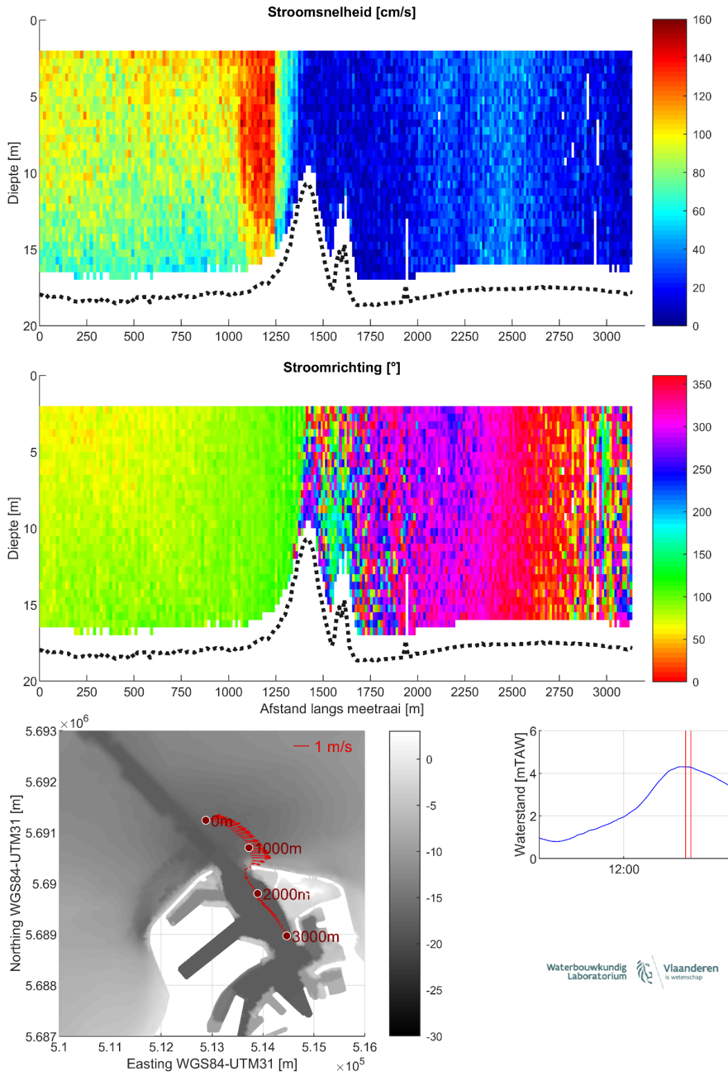
Figuur 29 – Stroomgegevens 16/08/2023 raai 24: snelheids grootte (top), -richting (midden) en diepte-gemiddelde vectoren (onder)
