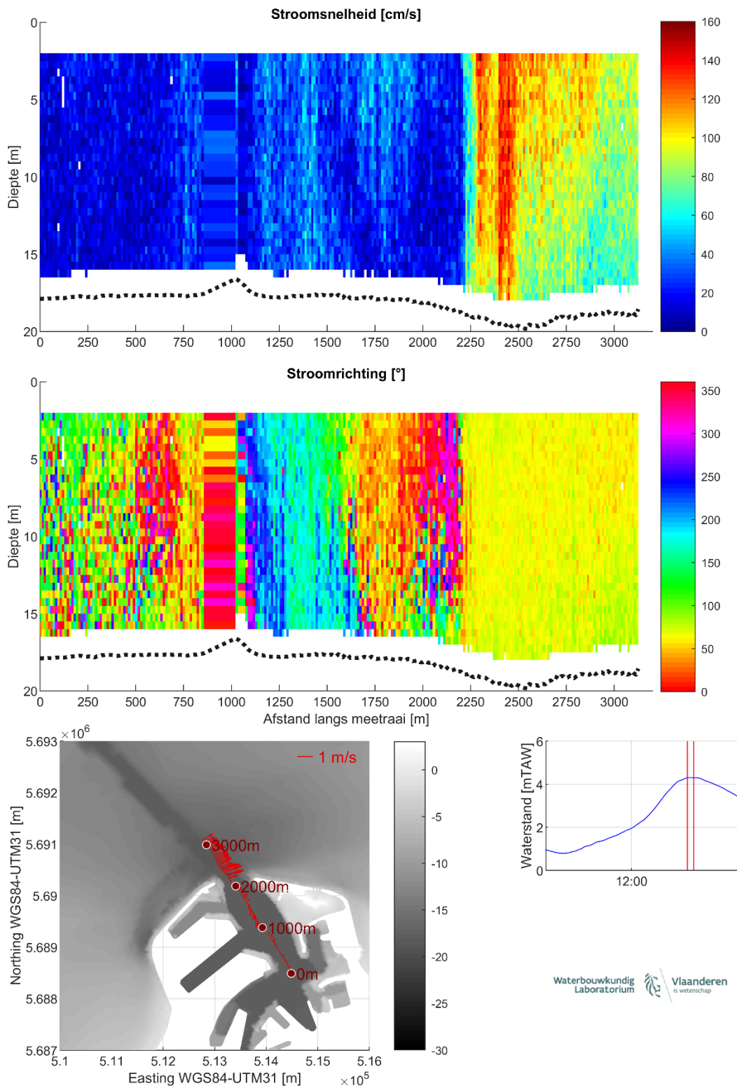
Figuur 28 – Stroomgegevens 16/08/2023 raai 23: snelheids grootte (top), -richting (midden) en diepte-gemiddelde vectoren (onder)
