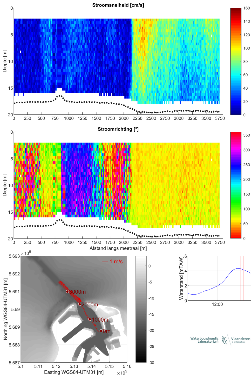
Figuur 30 – Stroomgegevens 16/08/2023 raai 25: snelheids grootte (top), -richting (midden) en diepte-gemiddelde vectoren (onder)
