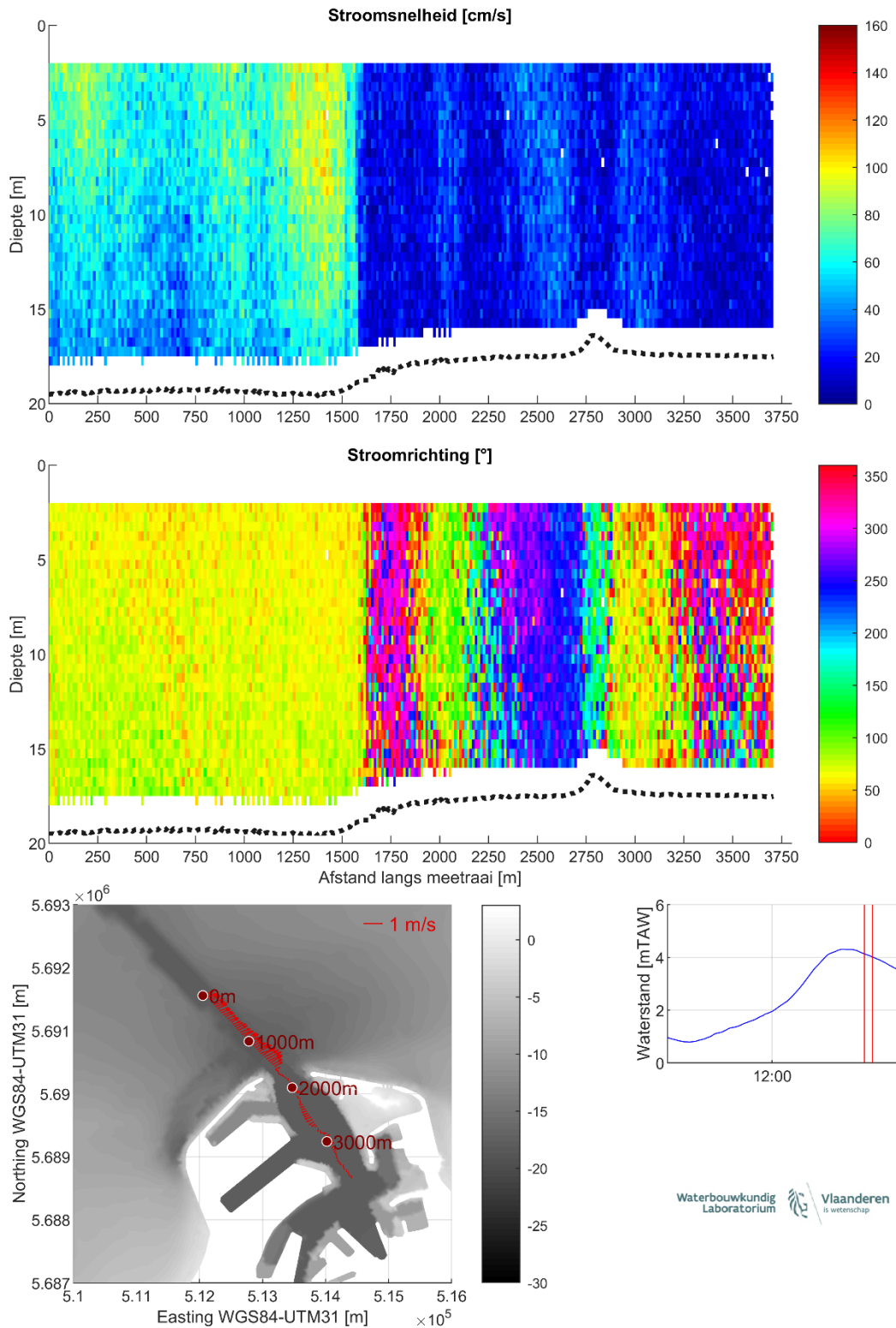
Figuur 31 – Stroomgegevens 16/08/2023 raai 26: snelheids grootte (top), -richting (midden) en diepte-gemiddelde vectoren (onder)
