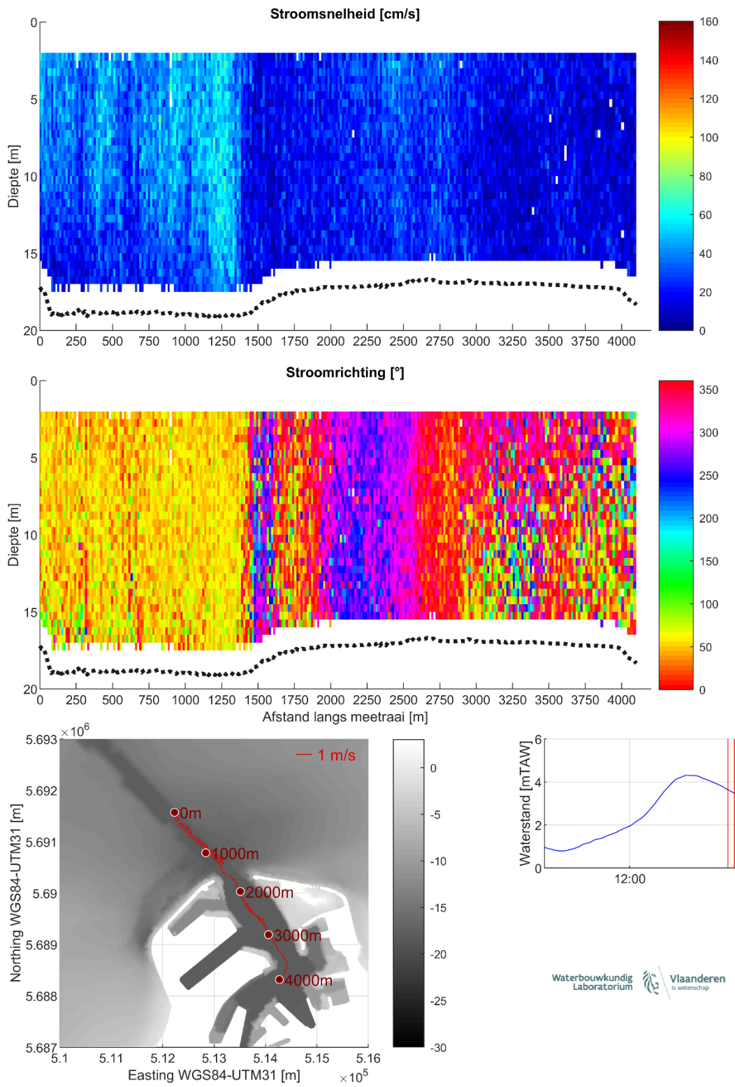
Figuur 35 – Stroomgegevens 16/08/2023 raai 30: snelheids grootte (top), -richting (midden) en diepte-gemiddelde vectoren (onder)
