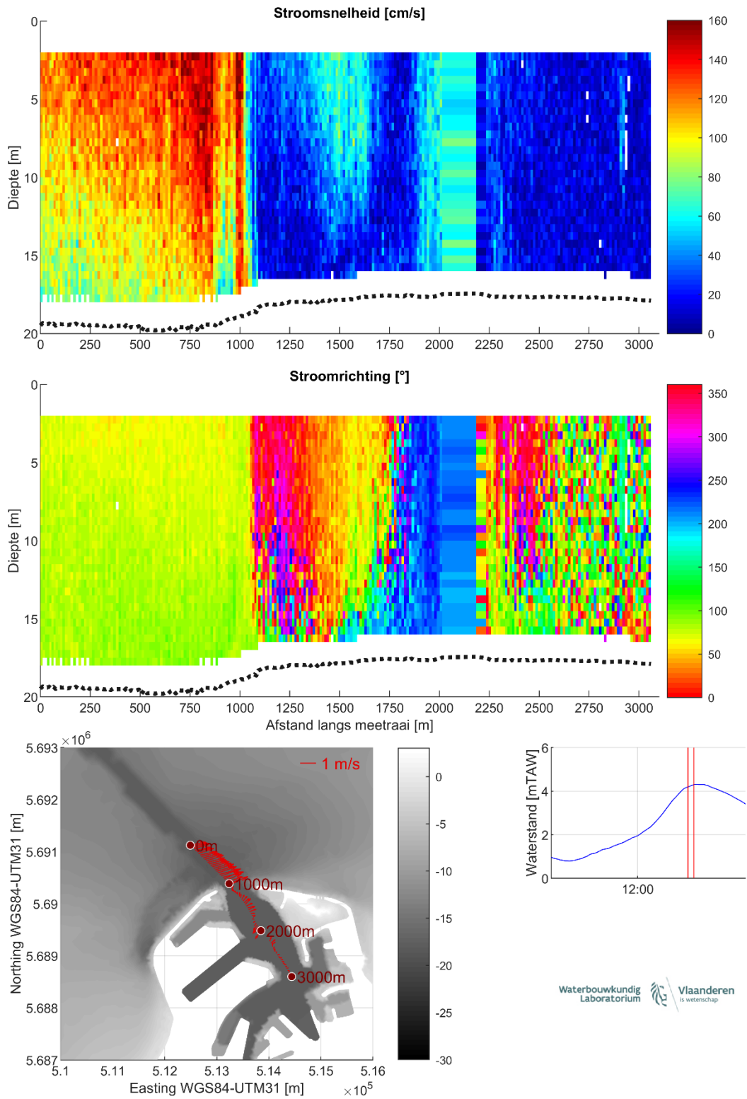
Figuur 27 – Stroomgegevens 16/08/2023 raai 22: snelheids grootte (top), -richting (midden) en diepte-gemiddelde vectoren (onder)
