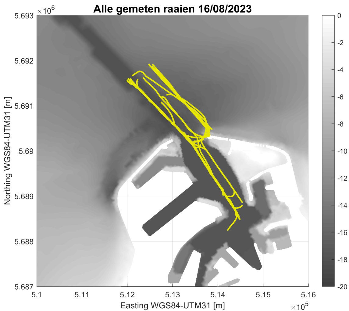
Figuur 3 – Ligging gemeten raaien op de meetdag 16/08/2023
