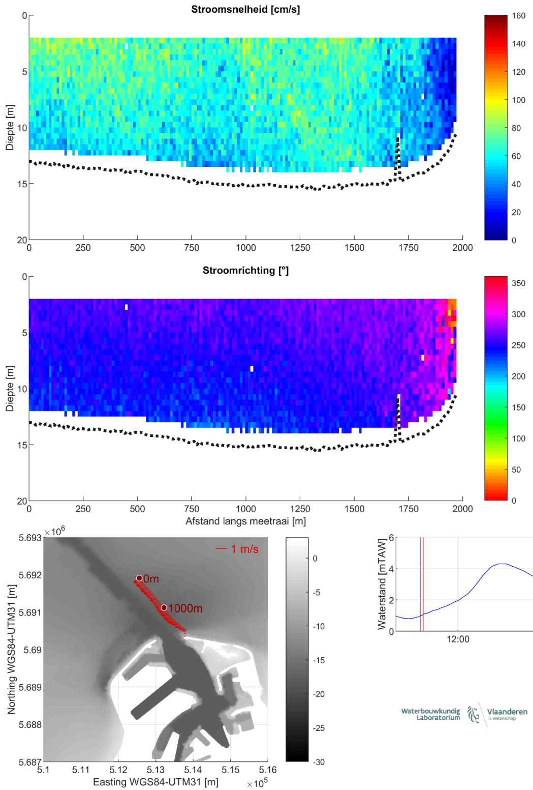
Figuur 9 – Stroomgegevens 16/08/2023 raai 4: snelheids grootte (top), -richting (midden) en diepte-gemiddelde vectoren (onder)
