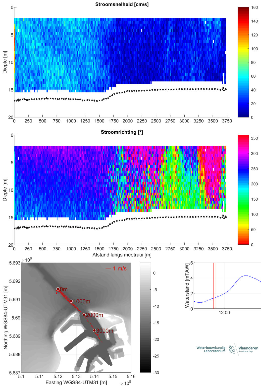
Figuur 13 – Stroomgegevens 16/08/2023 raai 8: snelheids grootte (top), -richting (midden) en diepte-gemiddelde vectoren (onder)
