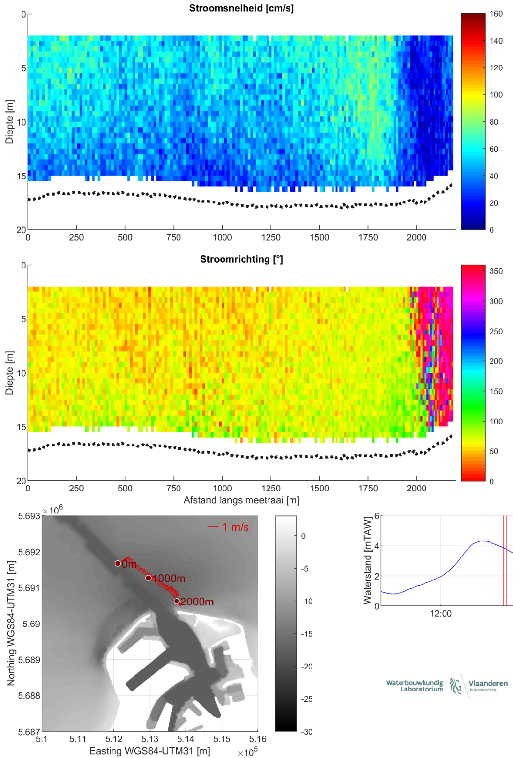
Figuur 33 – Stroomgegevens 16/08/2023 raai 28: snelheids grootte (top), -richting (midden) en diepte-gemiddelde vectoren (onder)
