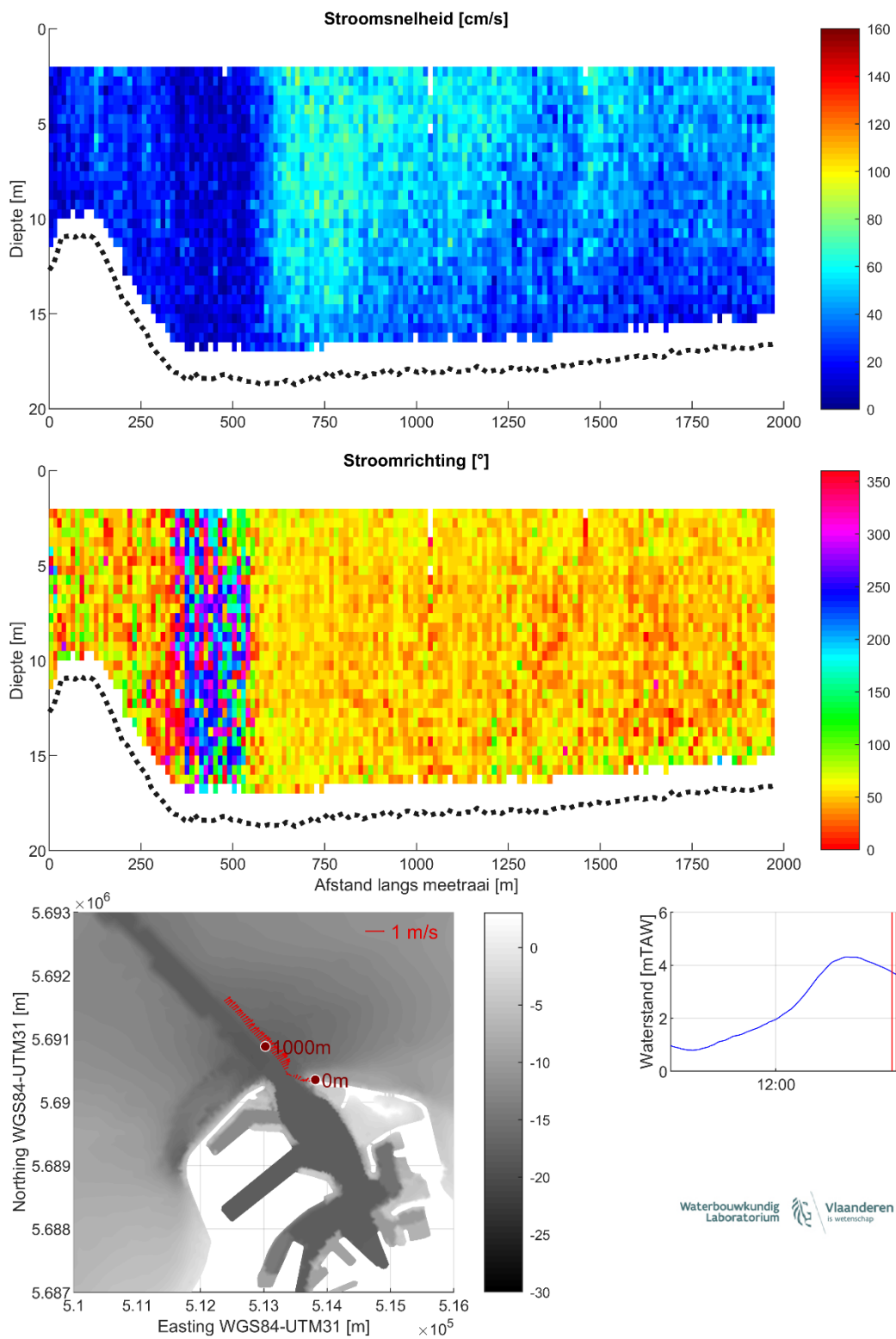
Figuur 34 – Stroomgegevens 16/08/2023 raai 29: snelheids grootte (top), -richting (midden) en diepte-gemiddelde vectoren (onder)
