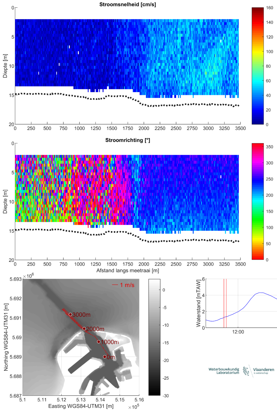
Figuur 12 – Stroomgegevens 16/08/2023 raai 7: snelheidsgruotte (top), -richting (midden) en diepte-gemiddelde vectoren (onder)
