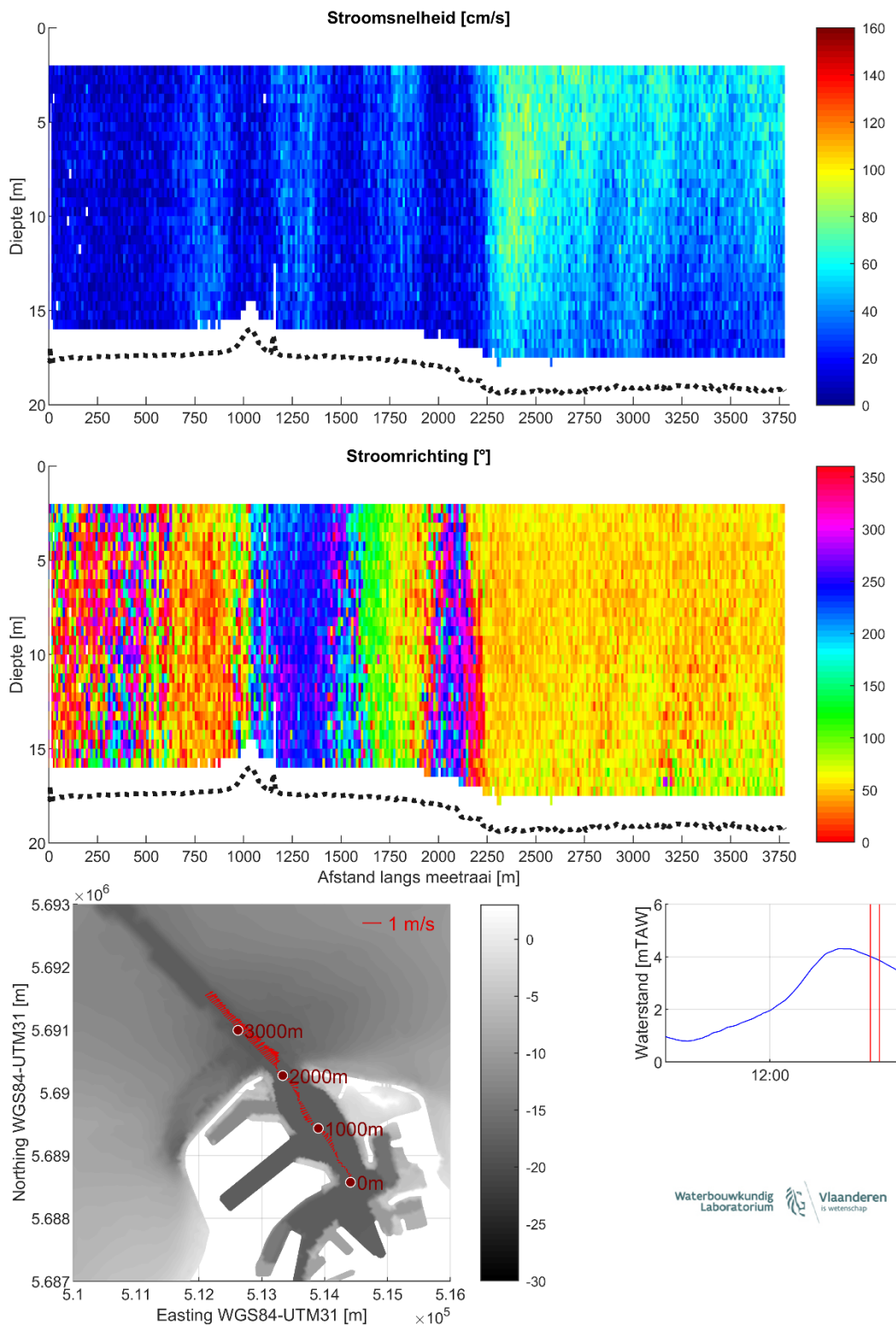
Figuur 32 – Stroomgegevens 16/08/2023 raai 27: snelheids grootte (top), -richting (midden) en diepte-gemiddelde vectoren (onder)
