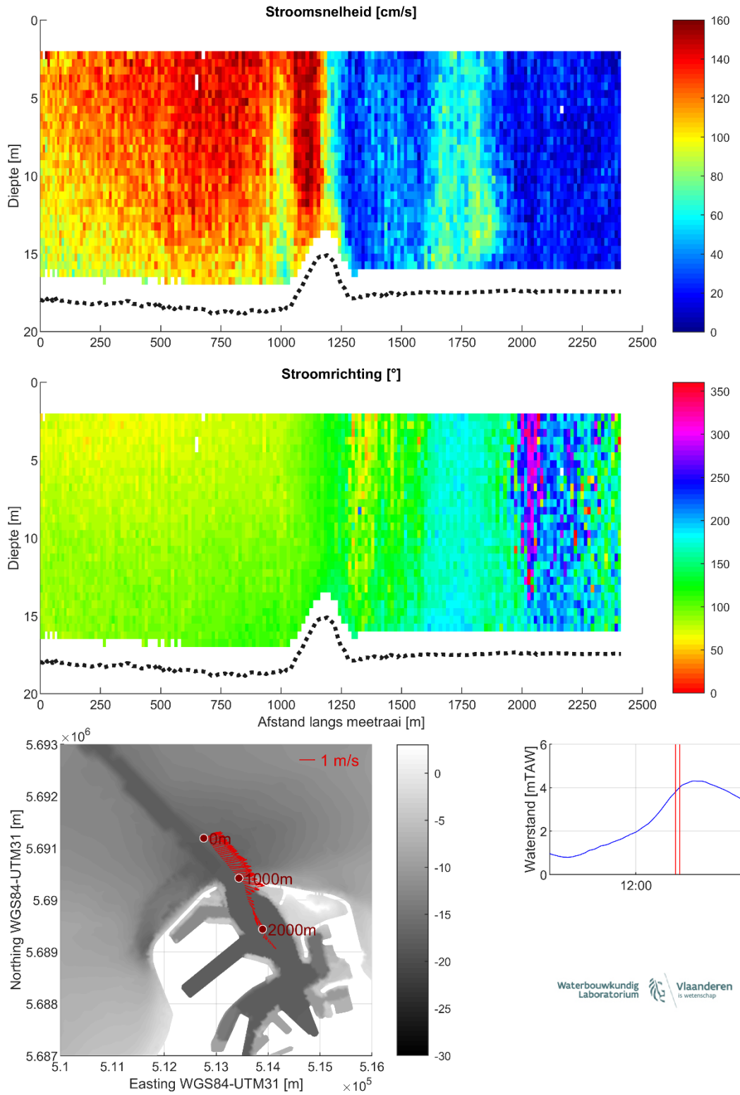
Figuur 25 – Stroomgegevens 16/08/2023 raai 20: snelheids grootte (top), -richting (midden) en diepte-gemiddelde vectoren (onder)
