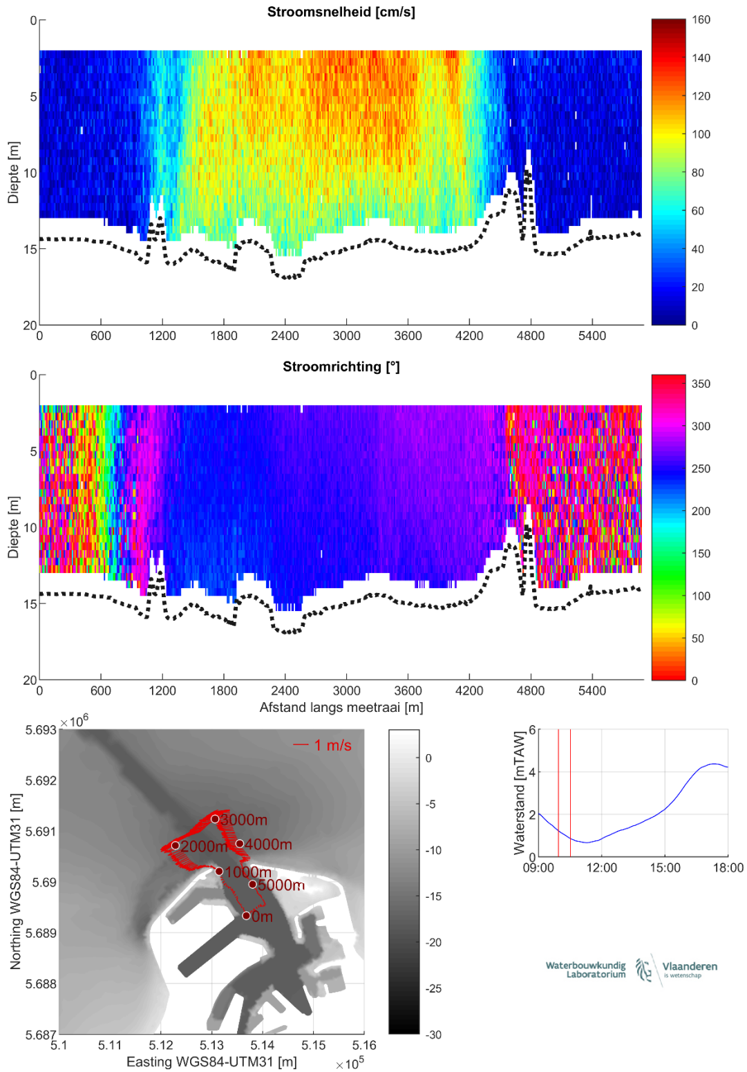
Figuur 7 – Stroomgegevens 21/08/2023 raai 2: snelheids grootte (top), -richting (midden) en diepte-gemiddelde vectoren (onder)
