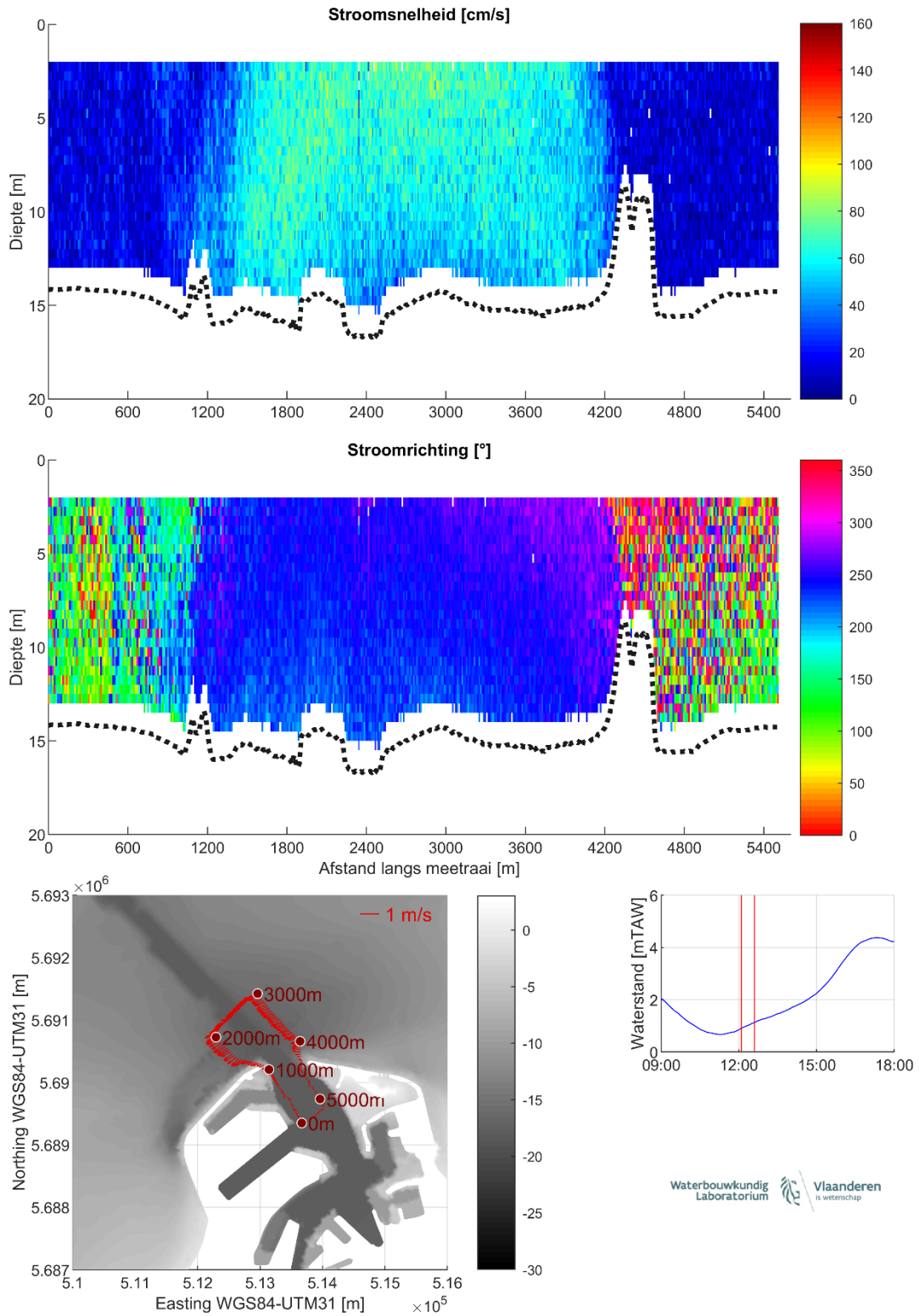
Figuur 11 – Stroomgegevens 21/08/2023 raai 6: snelheids grootte (top), -richting (midden) en diepte-gemiddelde vectoren (onder)
