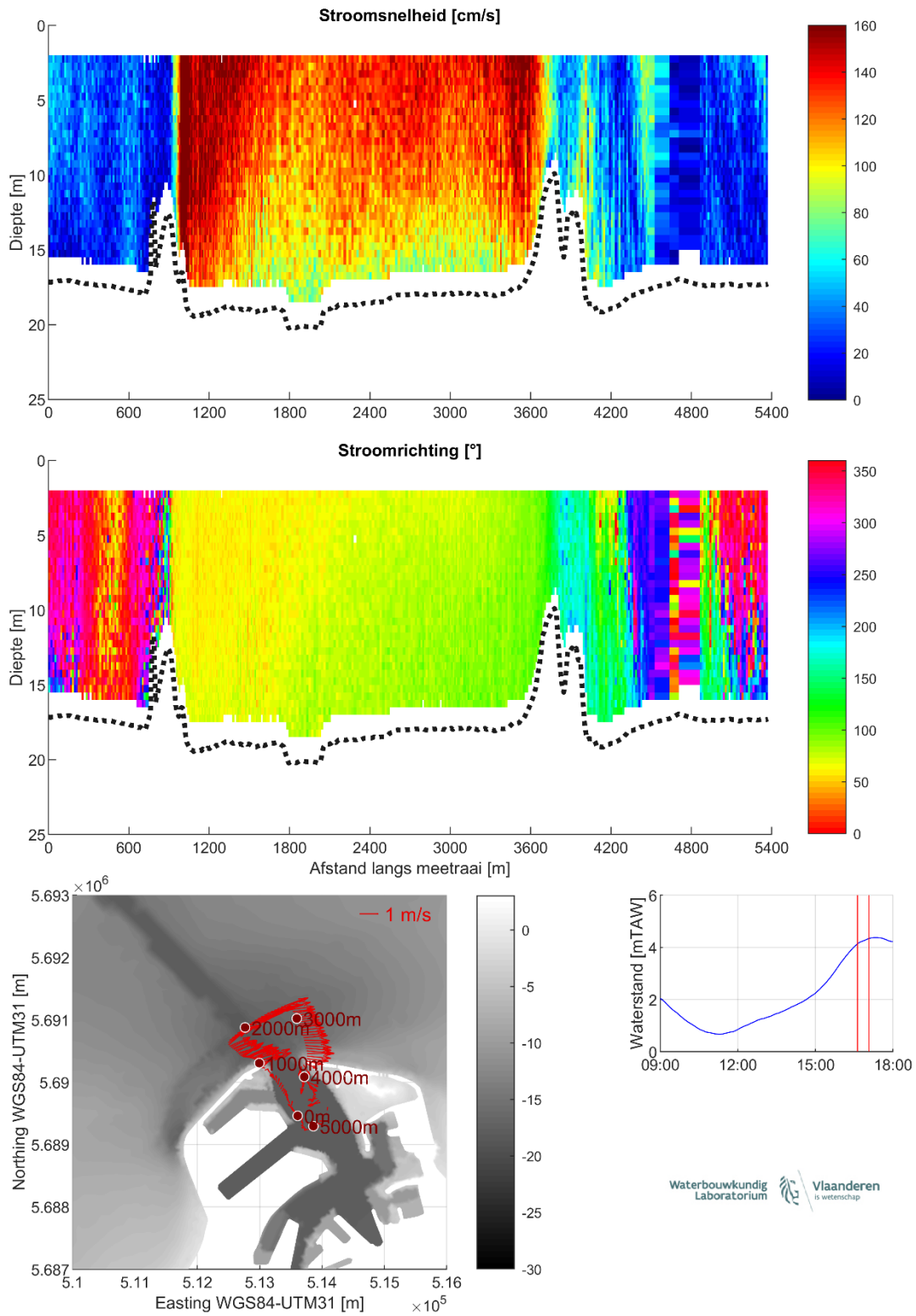
Figuur 20 – Stroomgegevens 21/08/2023 raai 15: snelheids grootte (top), -richting (midden) en diepte-gemiddelde vectoren (onder)
