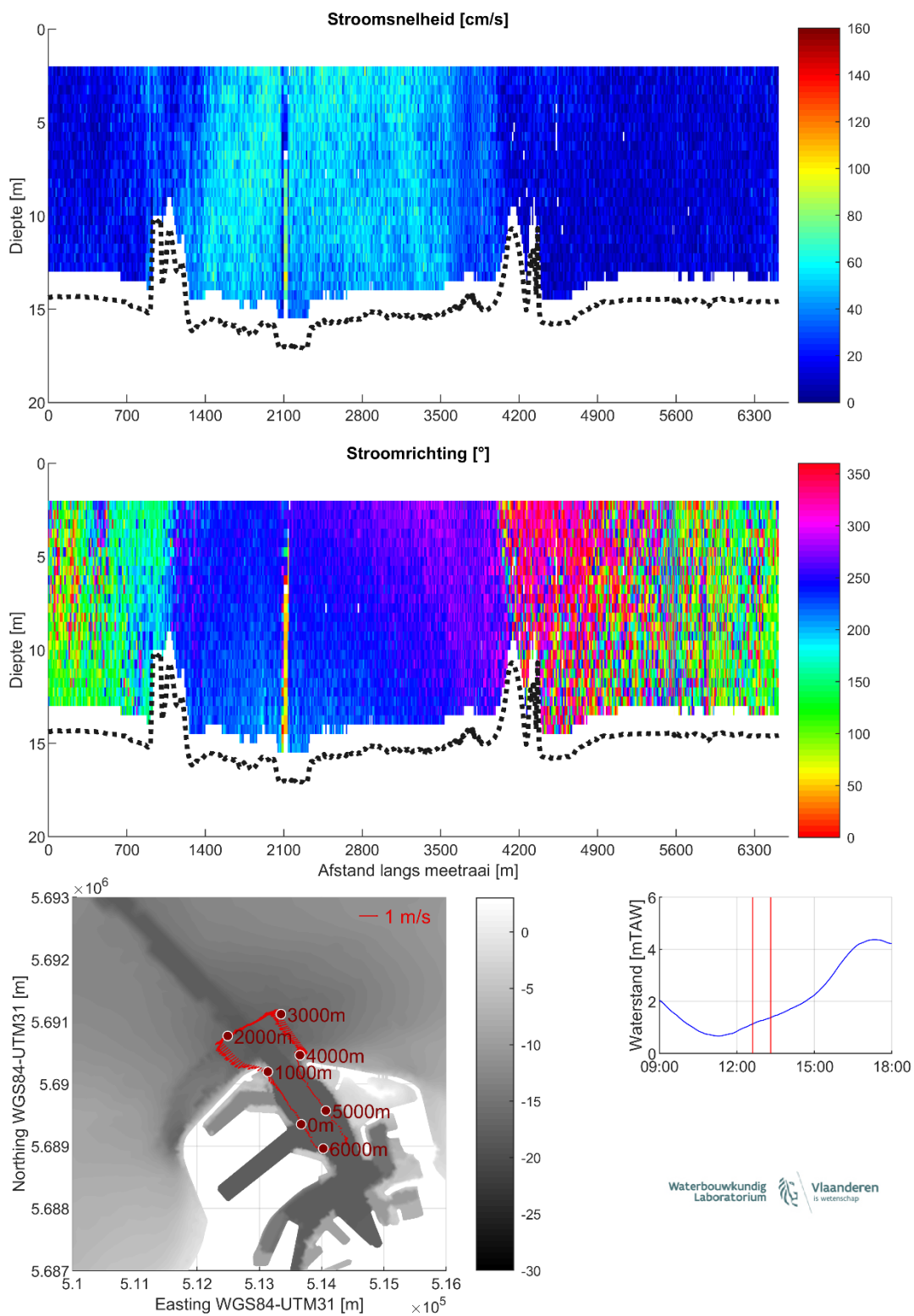
Figuur 12 – Stroomgegevens 21/08/2023 raai 7: snelheids grootte (top), -richting (midden) en diepte-gemiddelde vectoren (onder)
