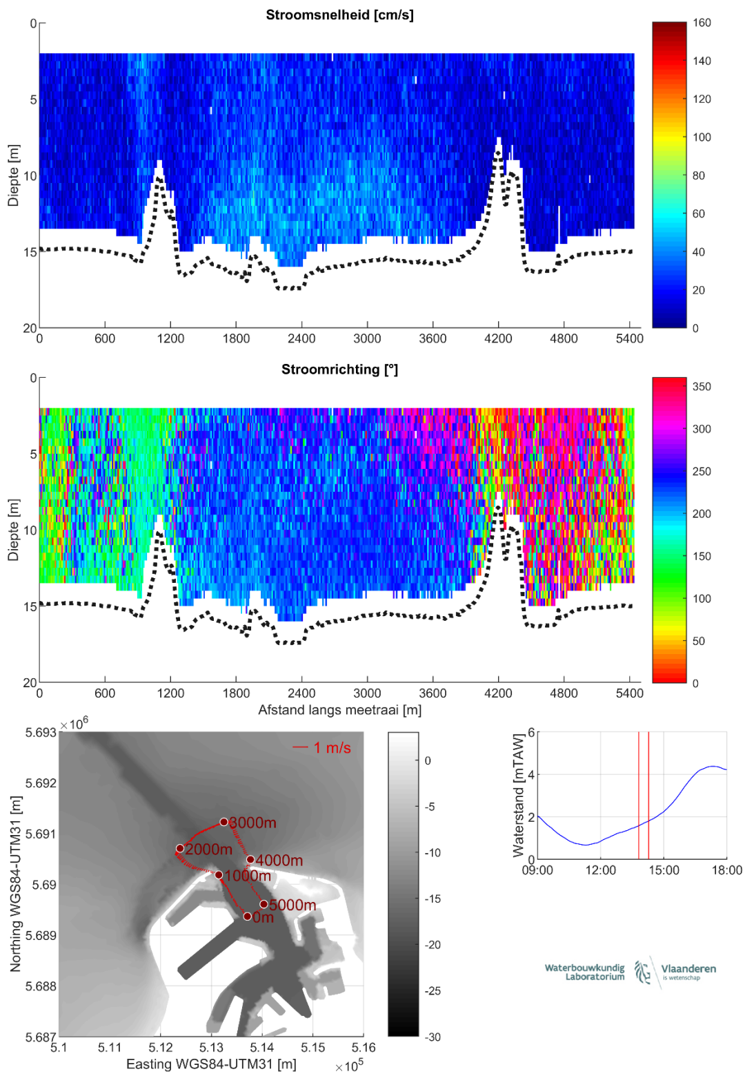
Figuur 14 – Stroomgegevens 21/08/2023 raai 9: snelheids grootte (top), -richting (midden) en diepte-gemiddelde vectoren (onder)
