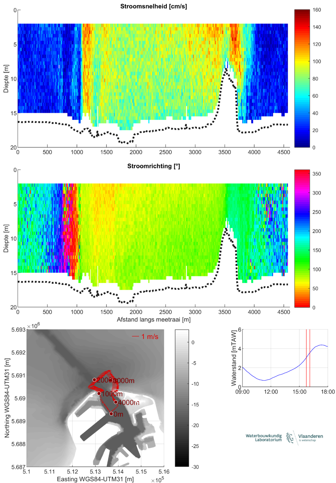
Figuur 18 – Stroomgegevens 21/08/2023 raai 13: snelheids grootte (top), -richting (midden) en diepte-gemiddelde vectoren (onder)
