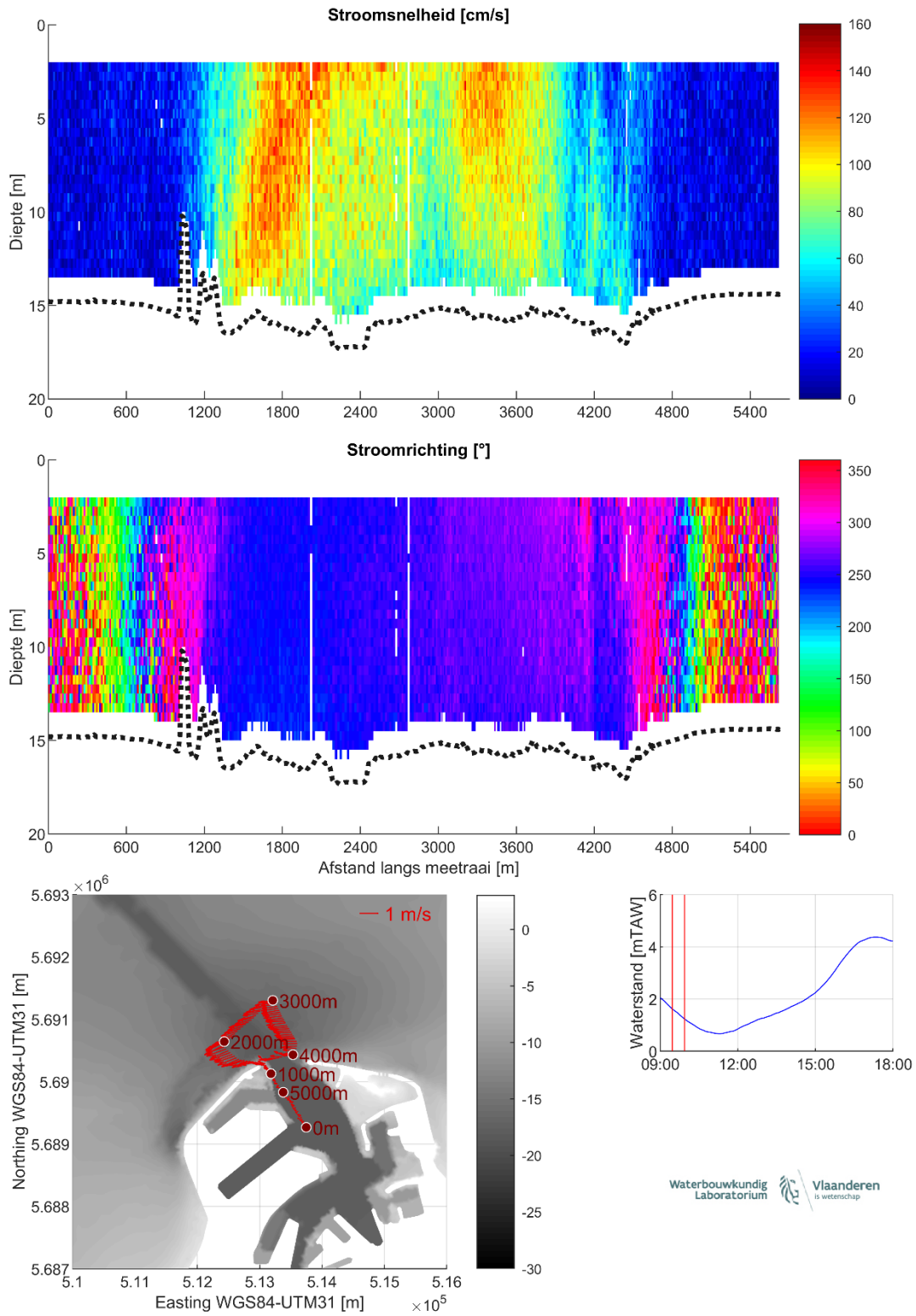
Figuur 6 – Stroomgegevens 21/08/2023 raai 1: snelheids grootte (top), -richting (midden) en diepte-gemiddelde vectoren (onder)
