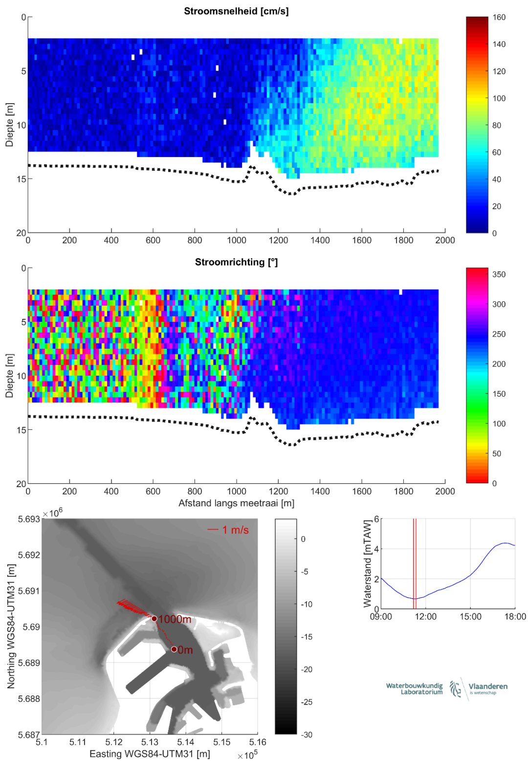
Figuur 9 – Stroomgegevens 21/08/2023 raai 4: snelheidsgrootte (top), -richting (midden) en diepte-gemiddelde vectoren (onder)
