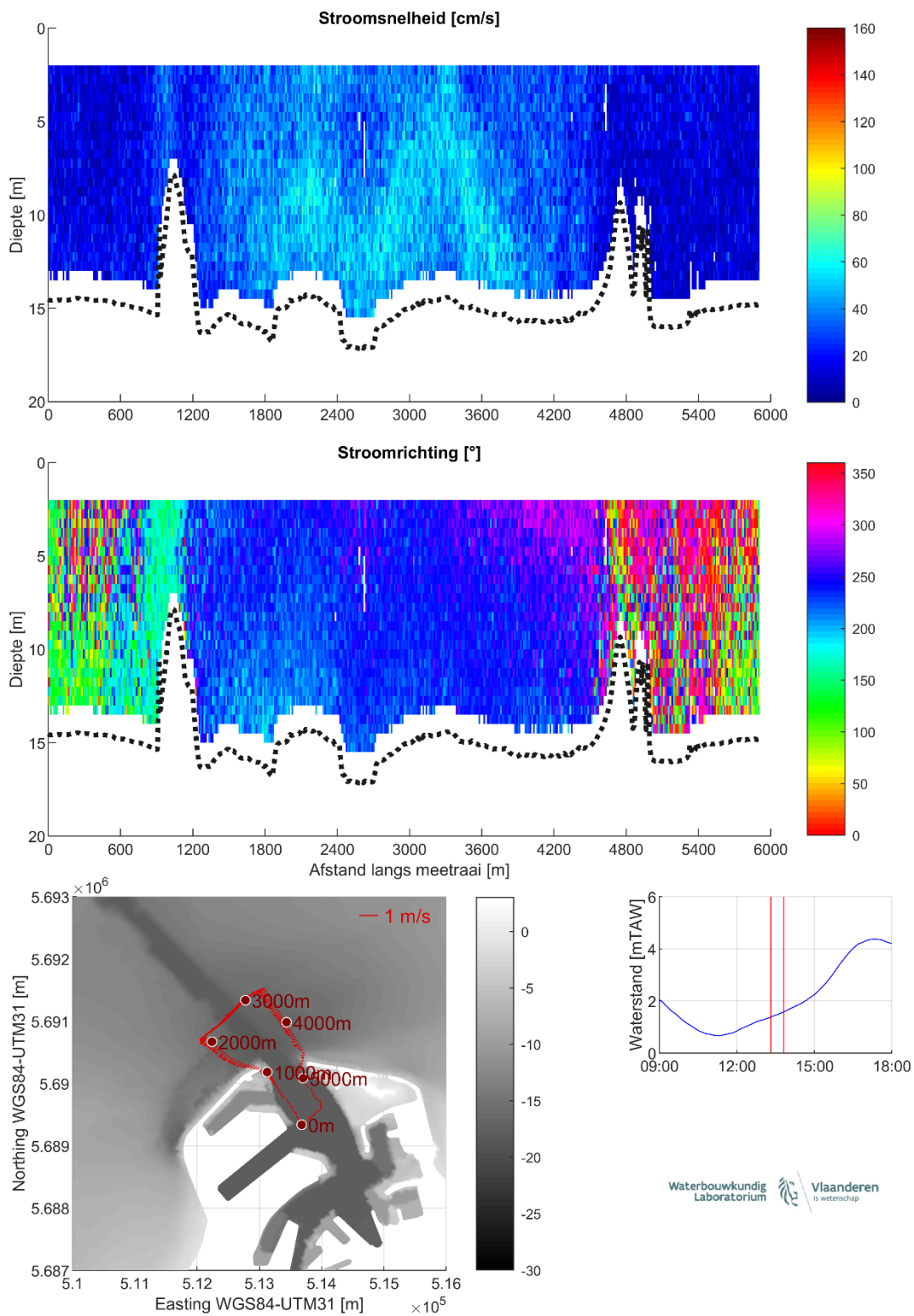
Figuur 13 – Stroomgegevens 21/08/2023 raai 8: snelheids grootte (top), -richting (midden) en diepte-gemiddelde vectoren (onder)
