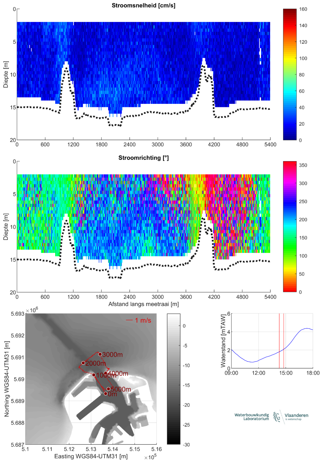
Figuur 15 – Stroomgegevens 21/08/2023 raai 10: snelheids grootte (top), -richting (midden) en diepte-gemiddelde vectoren (onder)
