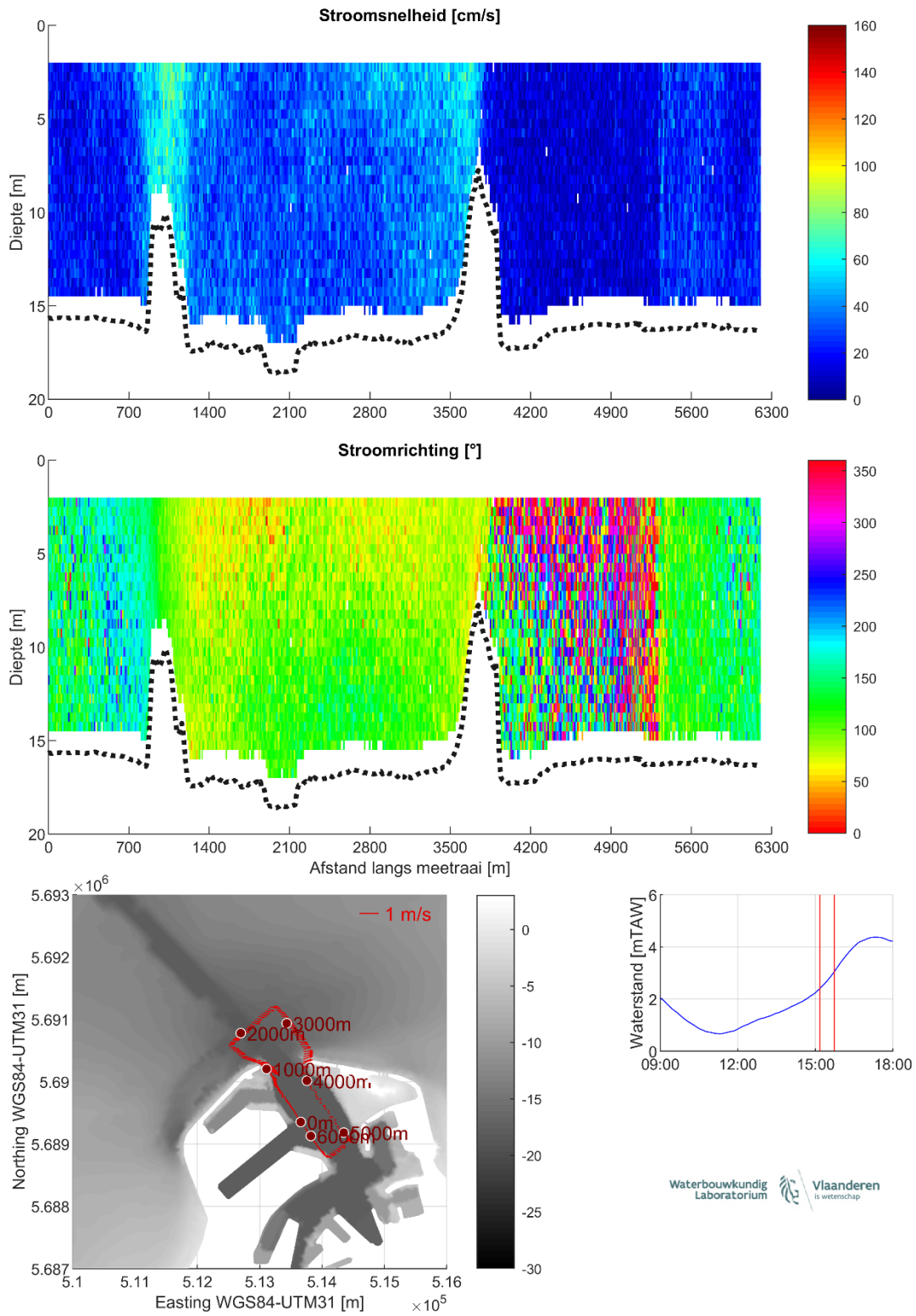
Figuur 17 – Stroomgegevens 21/08/2023 raai 12: snelheids grootte (top), -richting (midden) en diepte-gemiddelde vectoren (onder)
