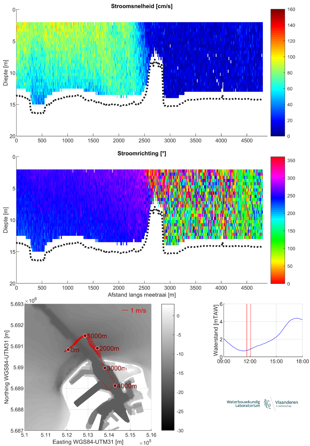
Figuur 10 – Stroomgegevens 21/08/2023 raai 5: snelheids grootte (top), -richting (midden) en diepte-gemiddelde vectoren (onder)
