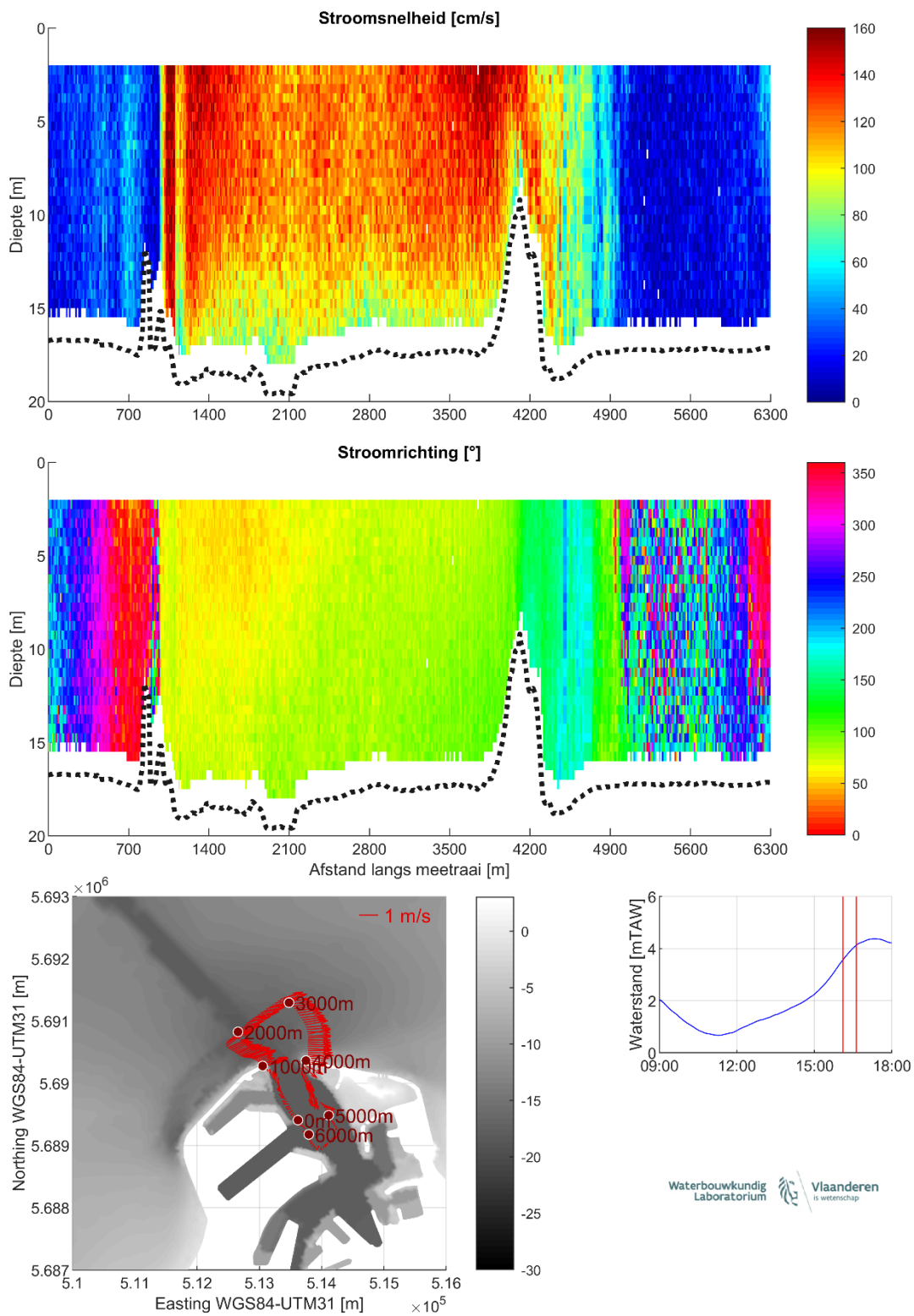
Figuur 19 – Stroomgegevens 21/08/2023 raai 14: snelheids grootte (top), -richting (midden) en diepte-gemiddelde vectoren (onder)
