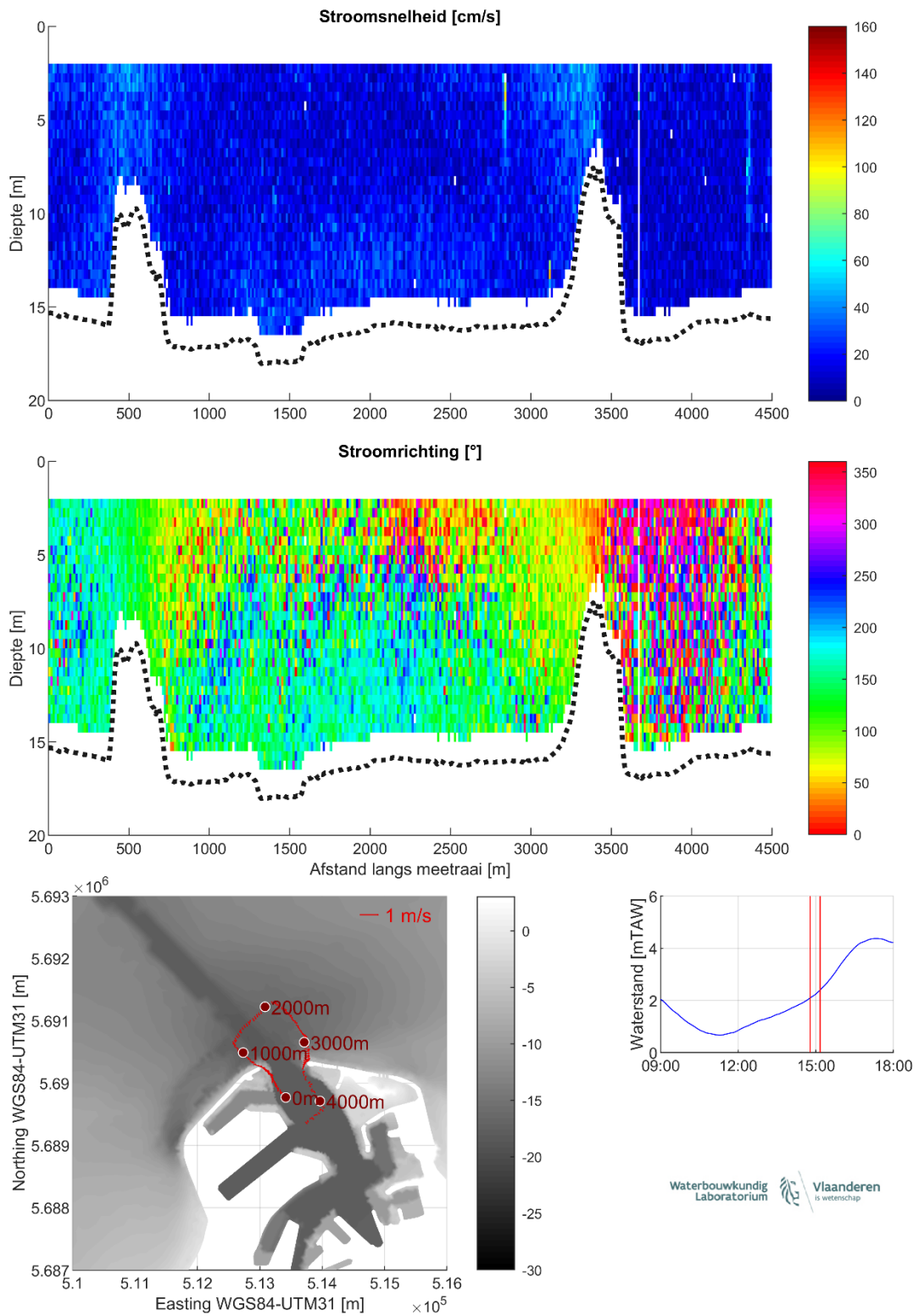
Figuur 16 – Stroomgegevens 21/08/2023 raai 11: snelheids grootte (top), -richting (midden) en diepte-gemiddelde vectoren (onder)
