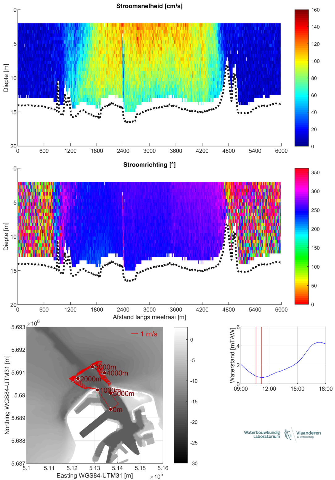
Figuur 8 – Stroomgegevens 21/08/2023 raai 3: snelheids grootte (top), -richting (midden) en diepte-gemiddelde vectoren (onder)
