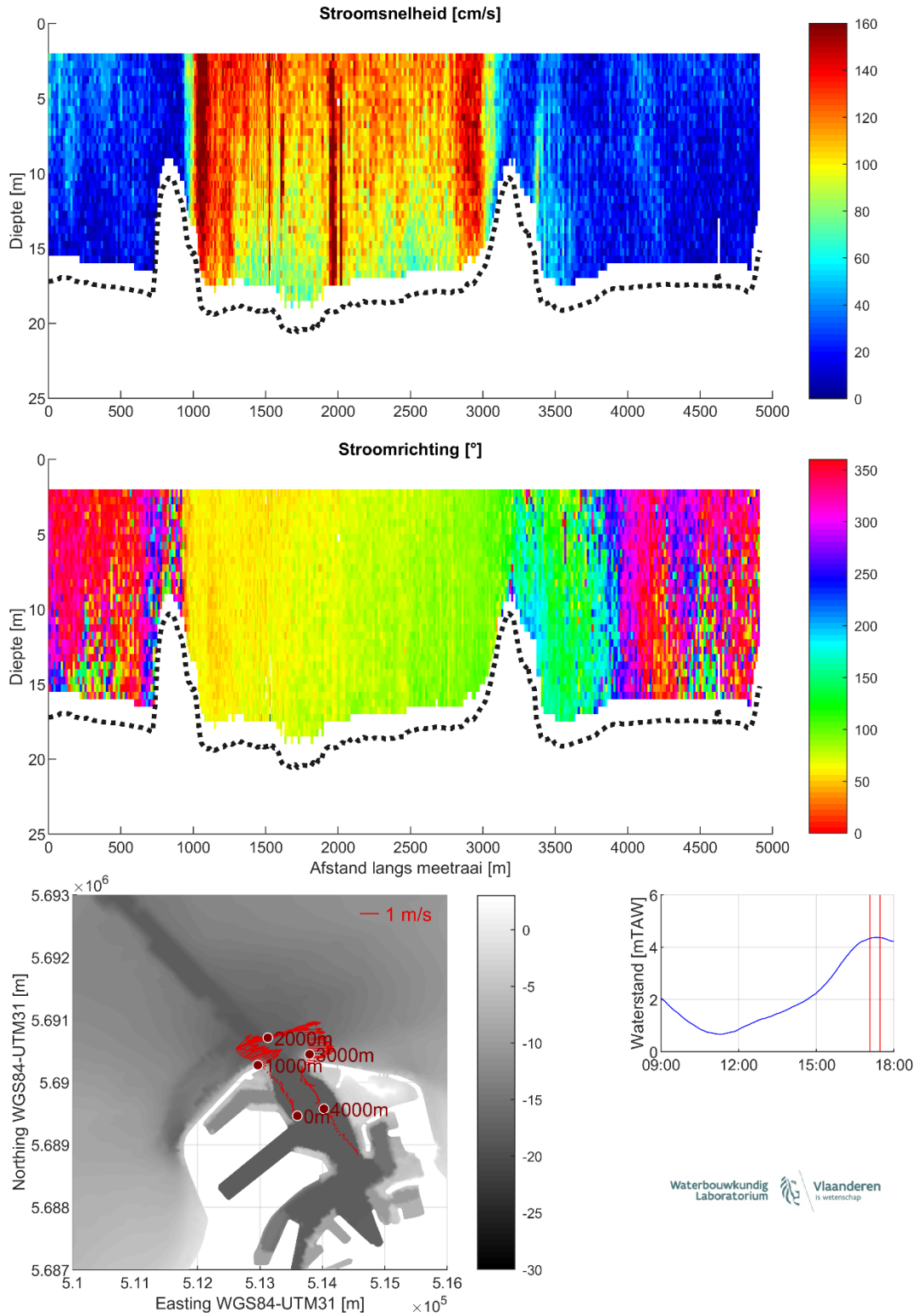
Figuur 21 – Stroomgegevens 21/08/2023 raai 16: snelheids grootte (top), -richting (midden) en diepte-gemiddelde vectoren (onder)
