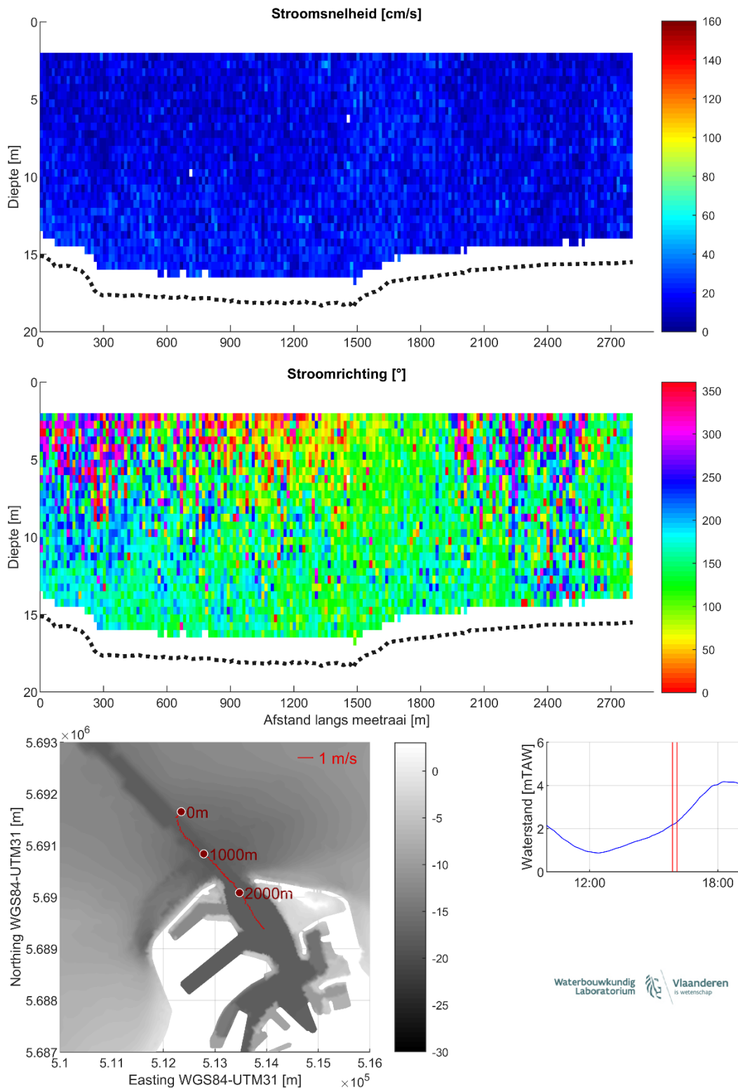
Figuur 27 – Stroomgegevens 23/08/2023 raai 22: snelheids grootte (top), -richting (midden) en diepte-gemiddelde vectoren (onder)
