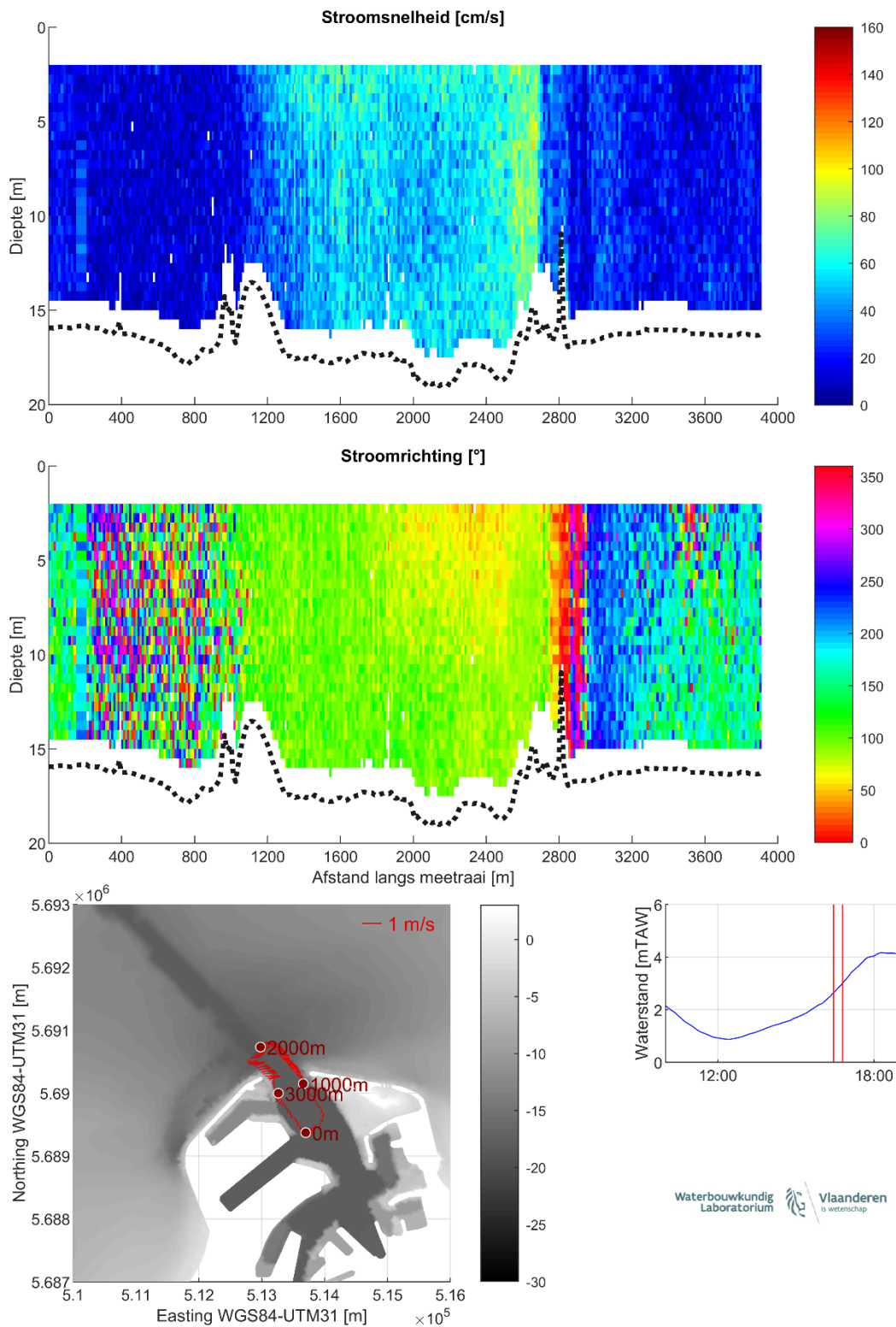
Figuur 30 – Stroomgegevens 23/08/2023 raai 25: snelheids grootte (top), -richting (midden) en diepte-gemiddelde vectoren (onder)
