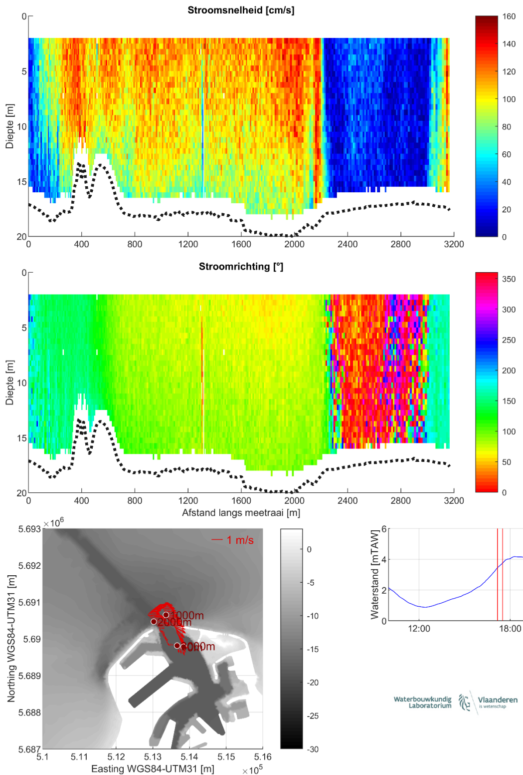
Figuur 32 – Stroomgegevens 23/08/2023 raai 27: snelheids grootte (top), -richting (midden) en diepte-gemiddelde vectoren (onder)
