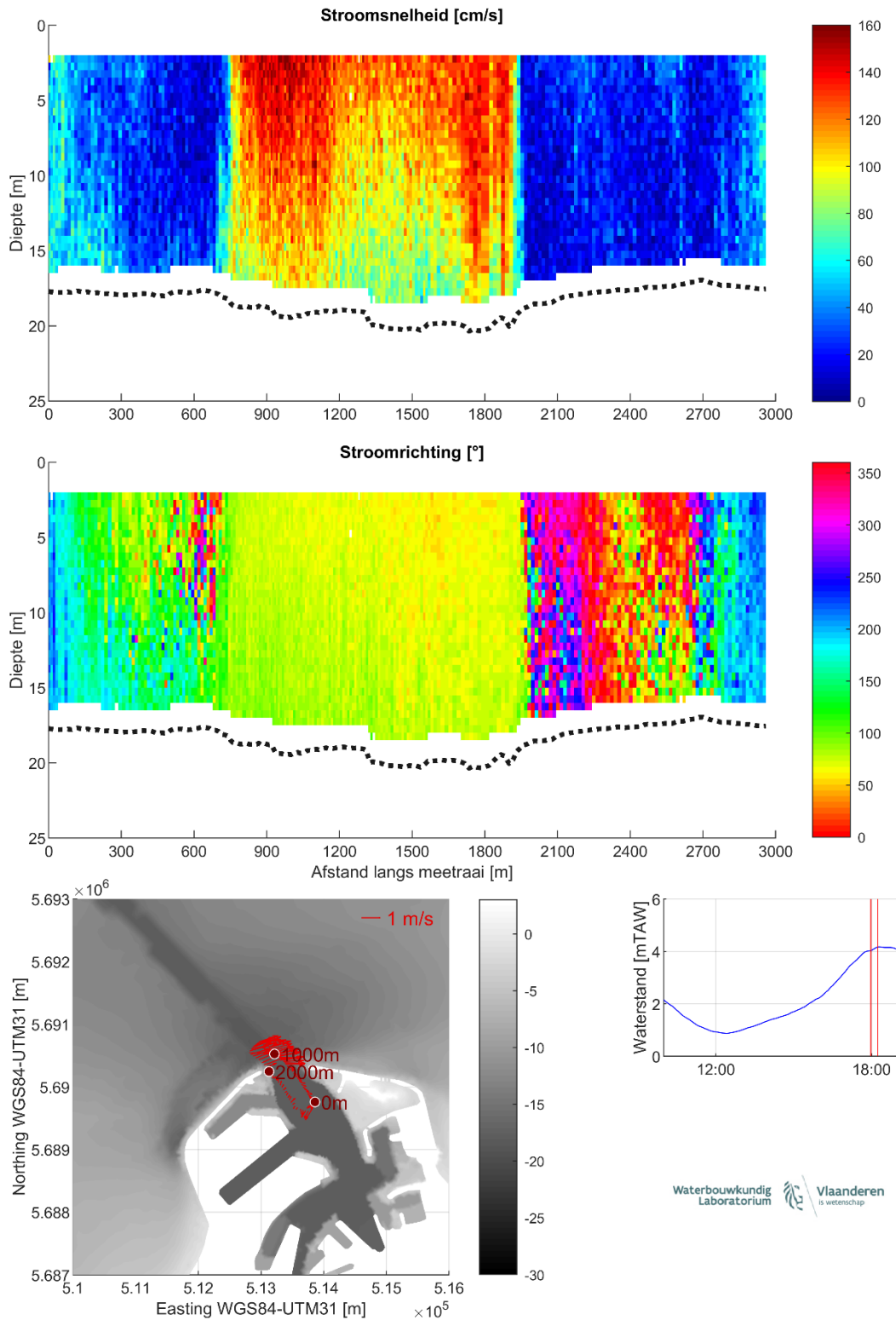
Figuur 35 – Stroomgegevens 23/08/2023 raai 30: snelheids grootte (top), -richting (midden) en diepte-gemiddelde vectoren (onder)
