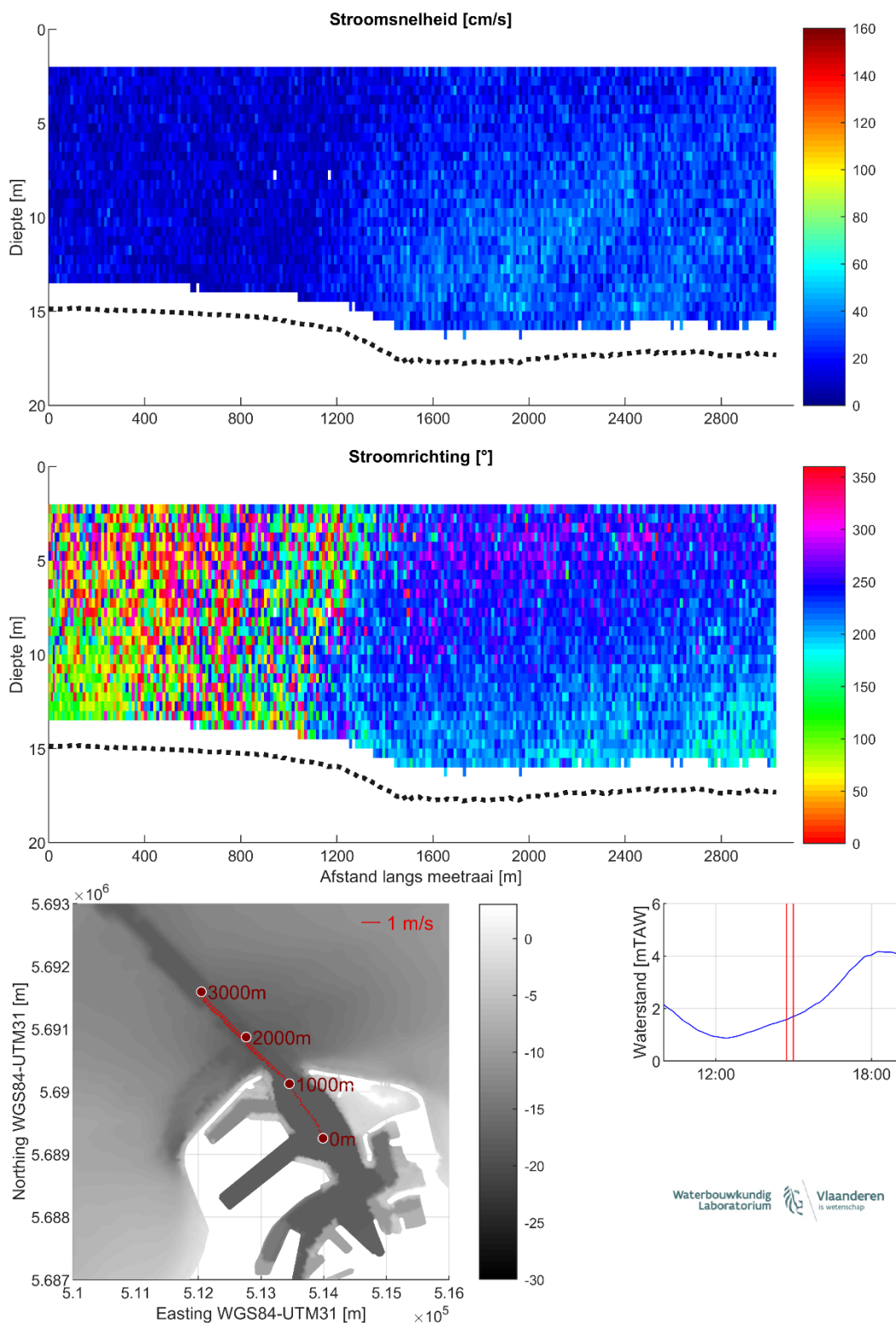
Figuur 22 – Stroomgegevens 23/08/2023 raai 17: snelheids grootte (top), -richting (midden) en diepte-gemiddelde vectoren (onder)
