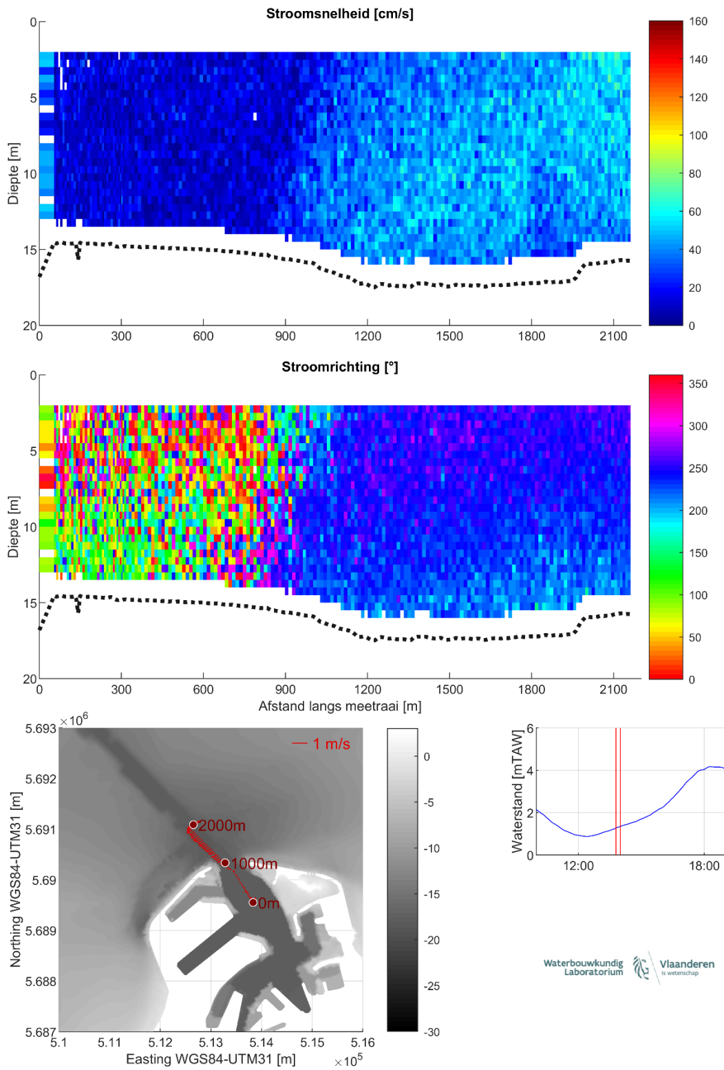
Figuur 18 – Stroomgegevens 23/08/2023 raai 13: snelheids grootte (top), -richting (midden) en diepte-gemiddelde vectoren (onder)
