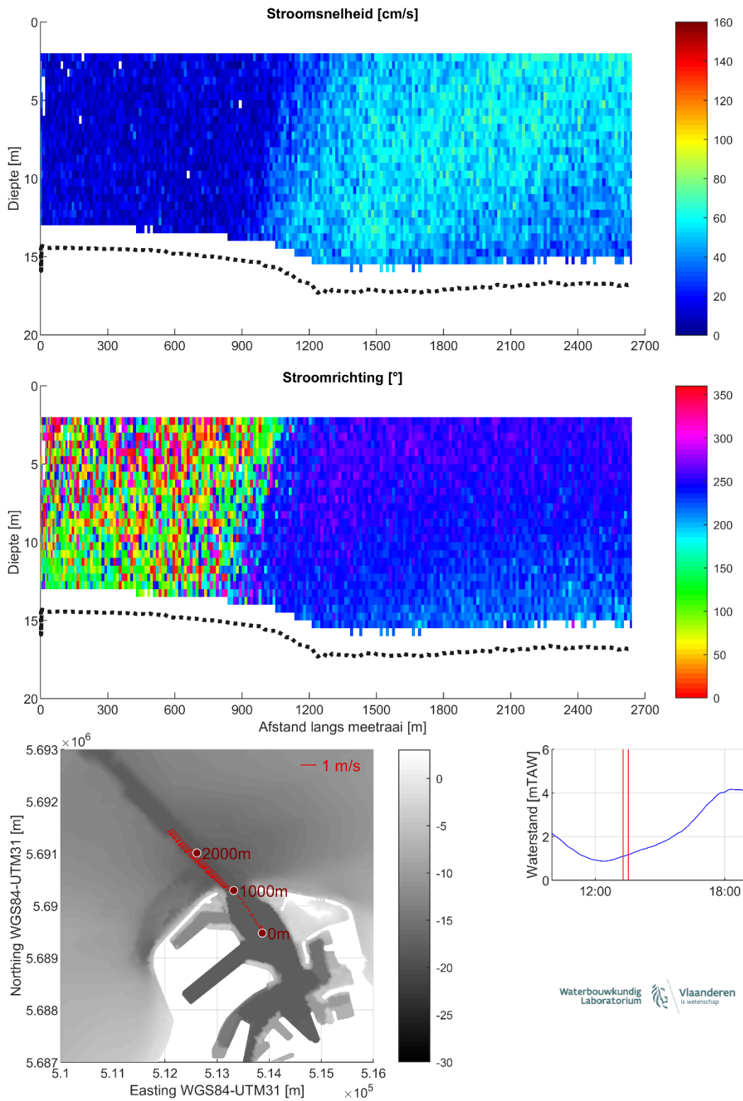
Figuur 16 – Stroomgegevens 23/08/2023 raai 11: snelheids grootte (top), -richting (midden) en diepte-gemiddelde vectoren (onder)
