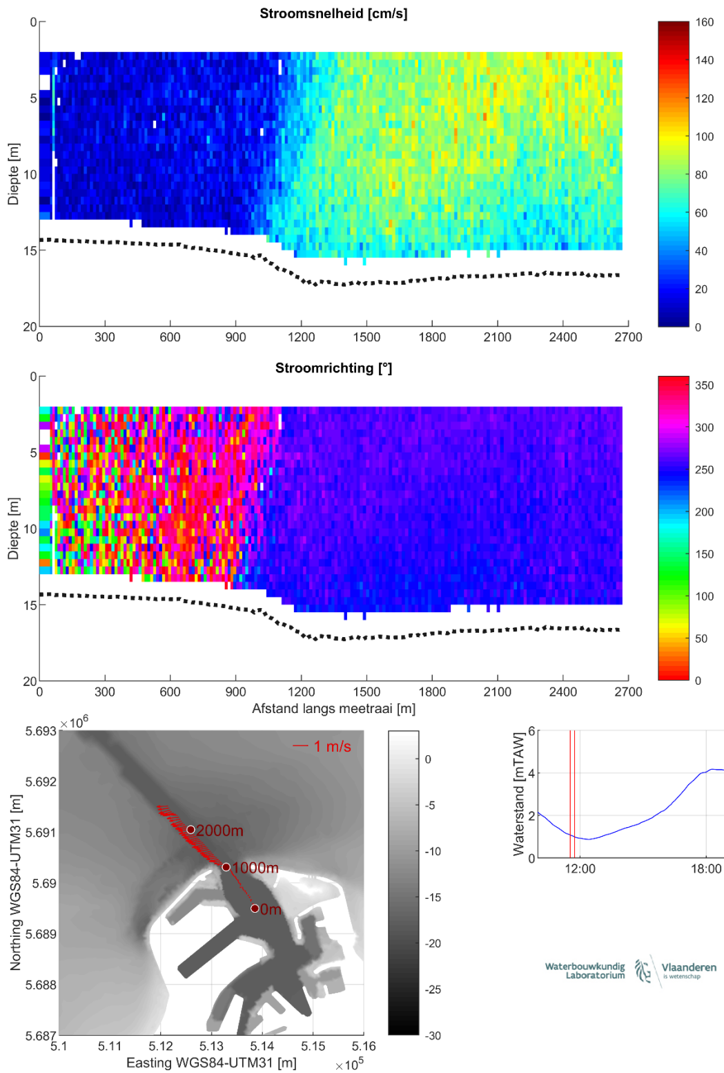
Figuur 8 – Stroomgegevens 23/08/2023 raai 3: snelheids grootte (top), -richting (midden) en diepte-gemiddelde vectoren (onder)
