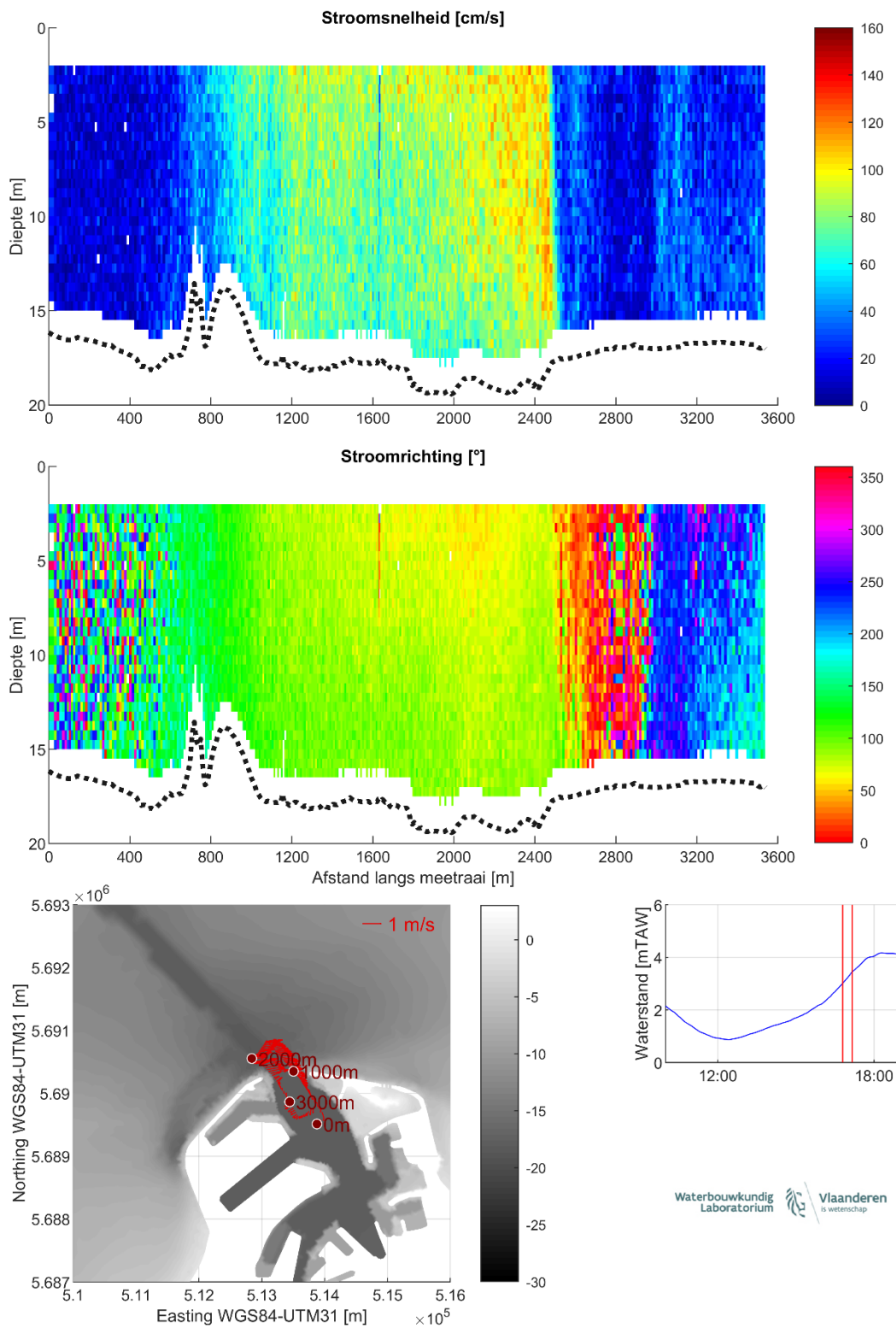
Figuur 31 – Stroomgegevens 23/08/2023 raai 26: snelheids grootte (top), -richting (midden) en diepte-gemiddelde vectoren (onder)
