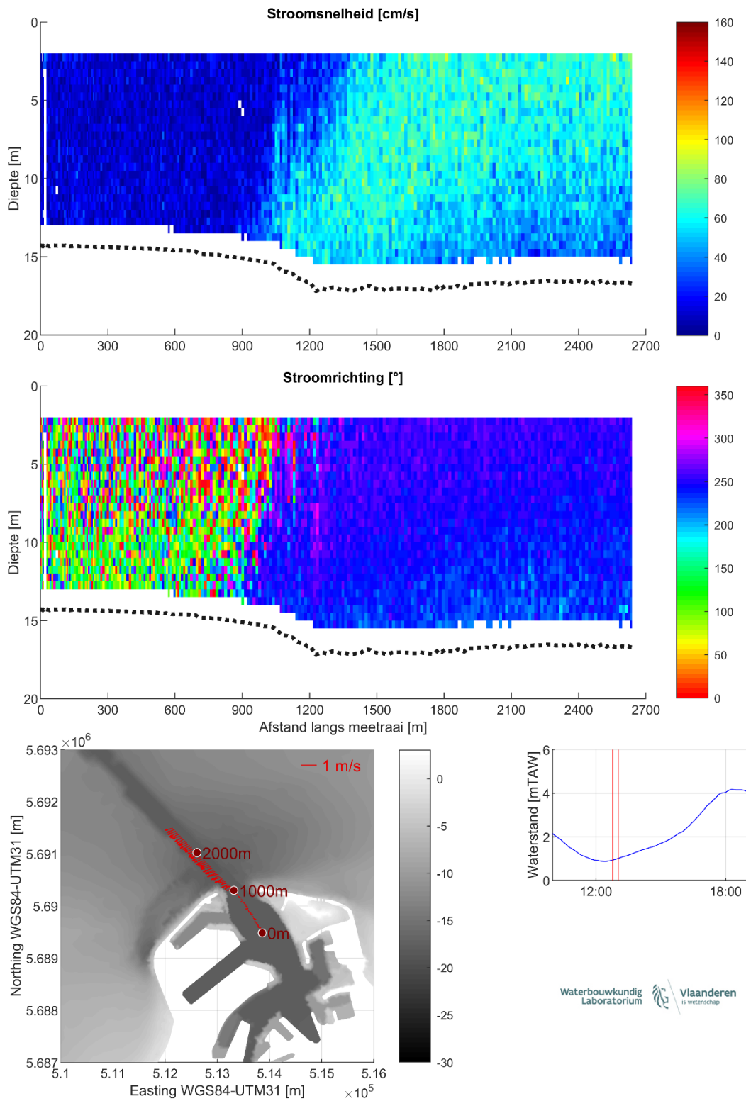
Figuur 14 – Stroomgegevens 23/08/2023 raai 9: snelheids grootte (top), -richting (midden) en diepte-gemiddelde vectoren (onder)
