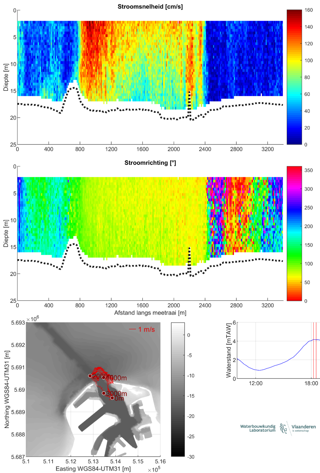
Figuur 36 – Stroomgegevens 23/08/2023 raai 31: snelheids grootte (top), -richting (midden) en diepte-gemiddelde vectoren (onder)
