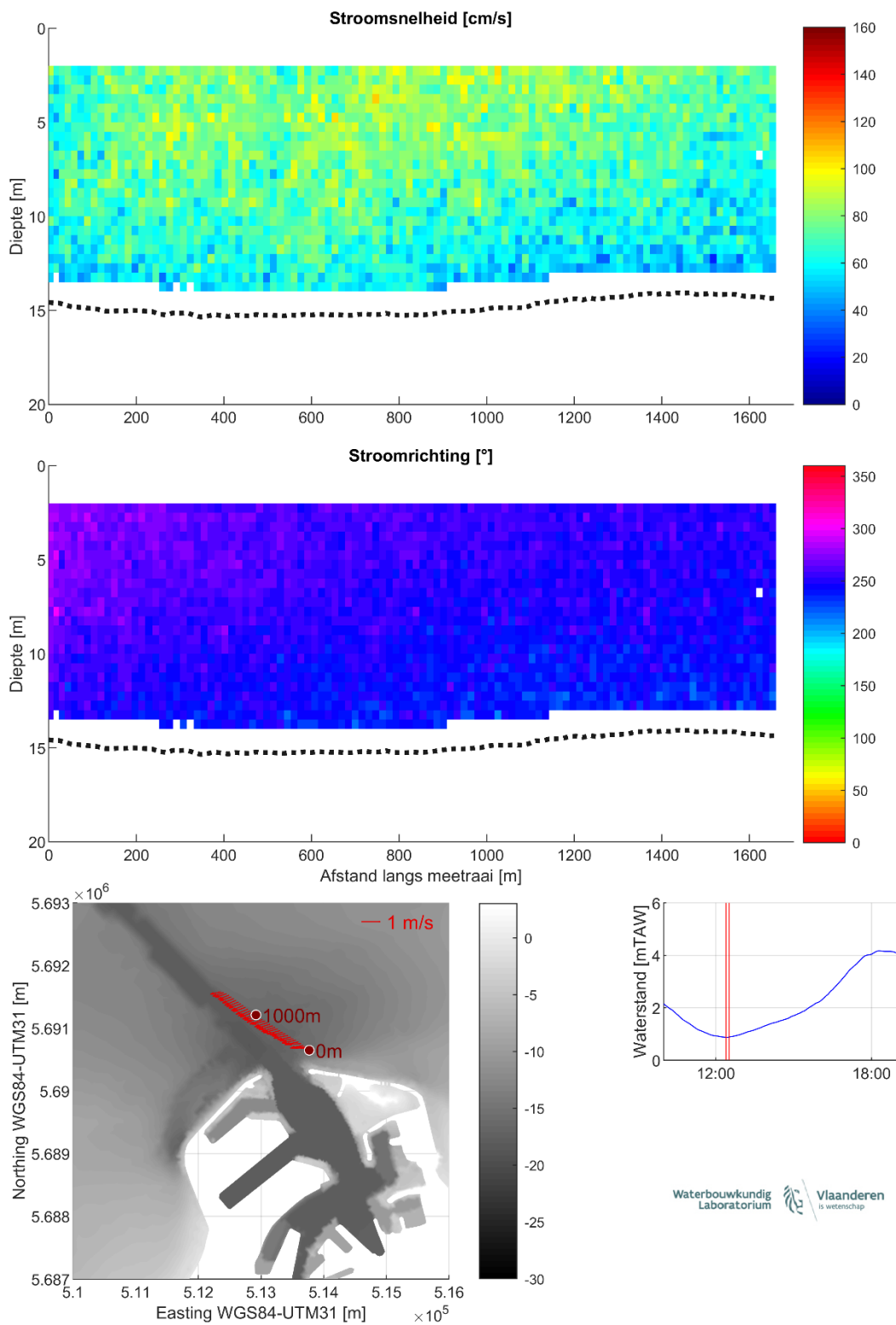
Figuur 12 – Stroomgegevens 23/08/2023 raai 7: snelheids grootte (top), -richting (midden) en diepte-gemiddelde vectoren (onder)
