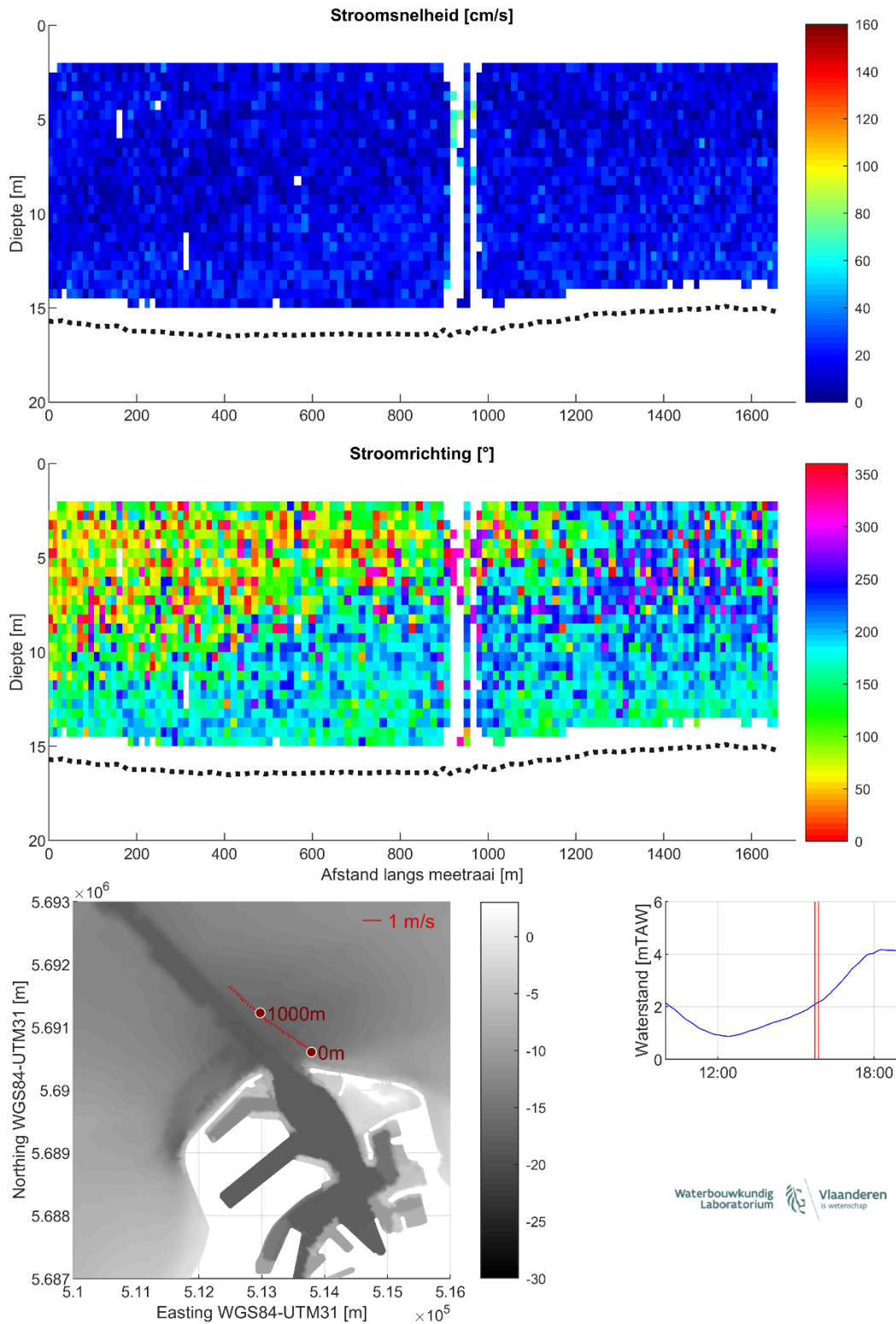
Figuur 26 – Stroomgegevens 23/08/2023 raai 21: snelheids grootte (top), -richting (midden) en diepte-gemiddelde vectoren (onder)
