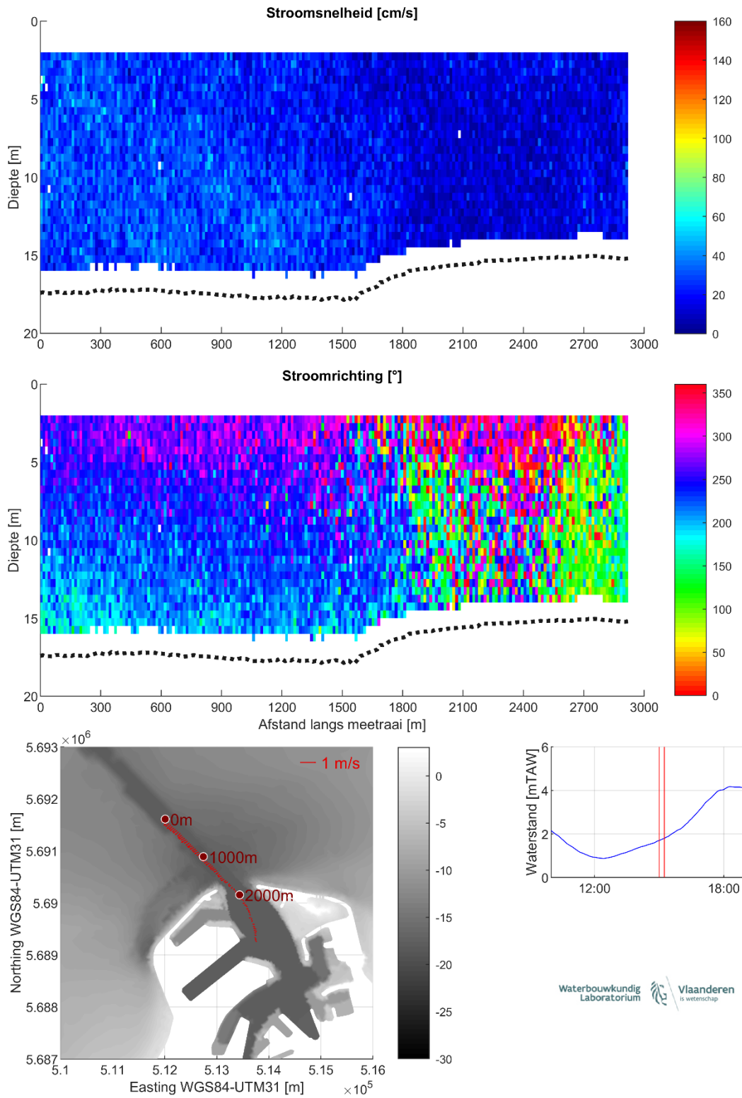
Figuur 23 – Stroomgegevens 23/08/2023 raai 18: snelheids grootte (top), -richting (midden) en diepte-gemiddelde vectoren (onder)
