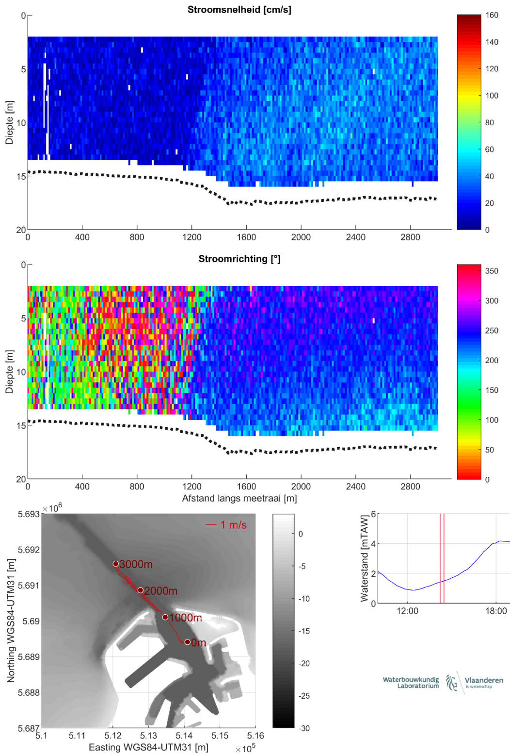
Figuur 20 – Stroomgegevens 23/08/2023 raai 15: snelheids grootte (top), -richting (midden) en diepte-gemiddelde vectoren (onder)
