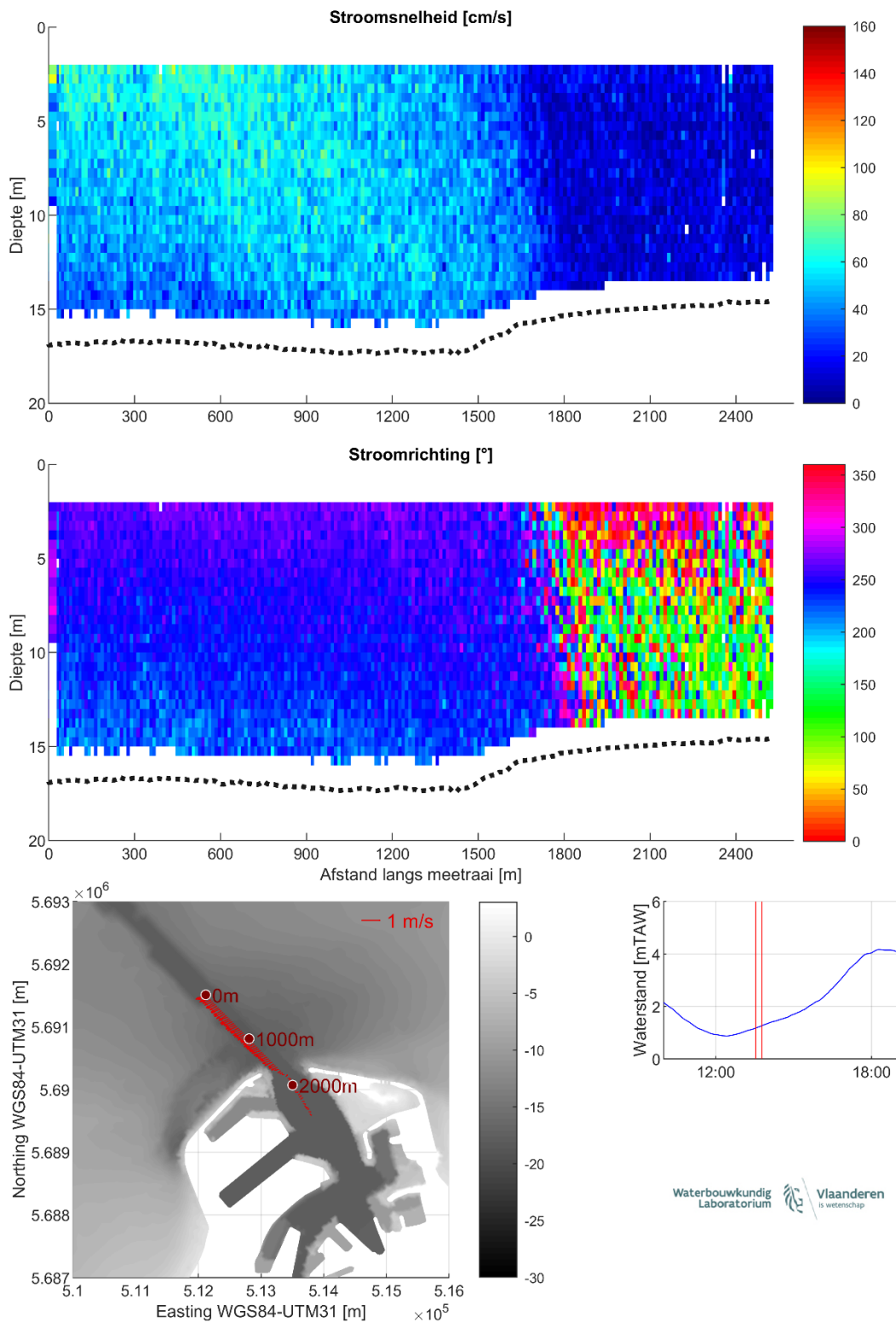
Figuur 17 – Stroomgegevens 23/08/2023 raai 12: snelheids grootte (top), -richting (midden) en diepte-gemiddelde vectoren (onder)
