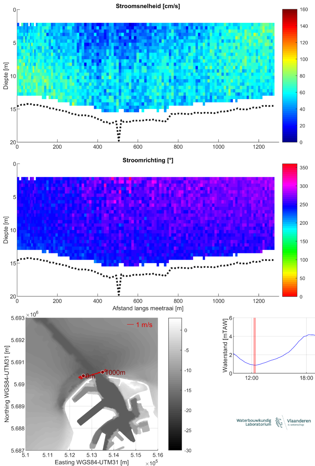
Figuur 11 – Stroomgegevens 23/08/2023 raai 6: snelheids grootte (top), -richting (midden) en diepte-gemiddelde vectoren (onder)
