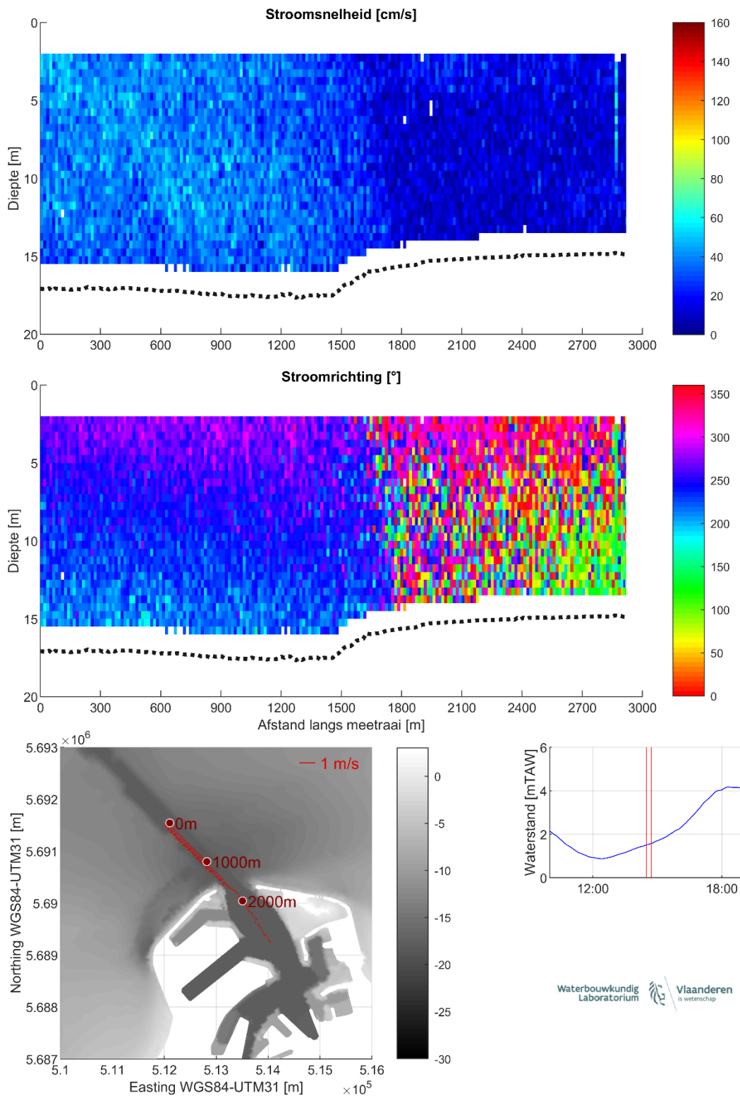
Figuur 21 – Stroomgegevens 23/08/2023 raai 16: snelheids grootte (top), -richting (midden) en diepte-gemiddelde vectoren (onder)
