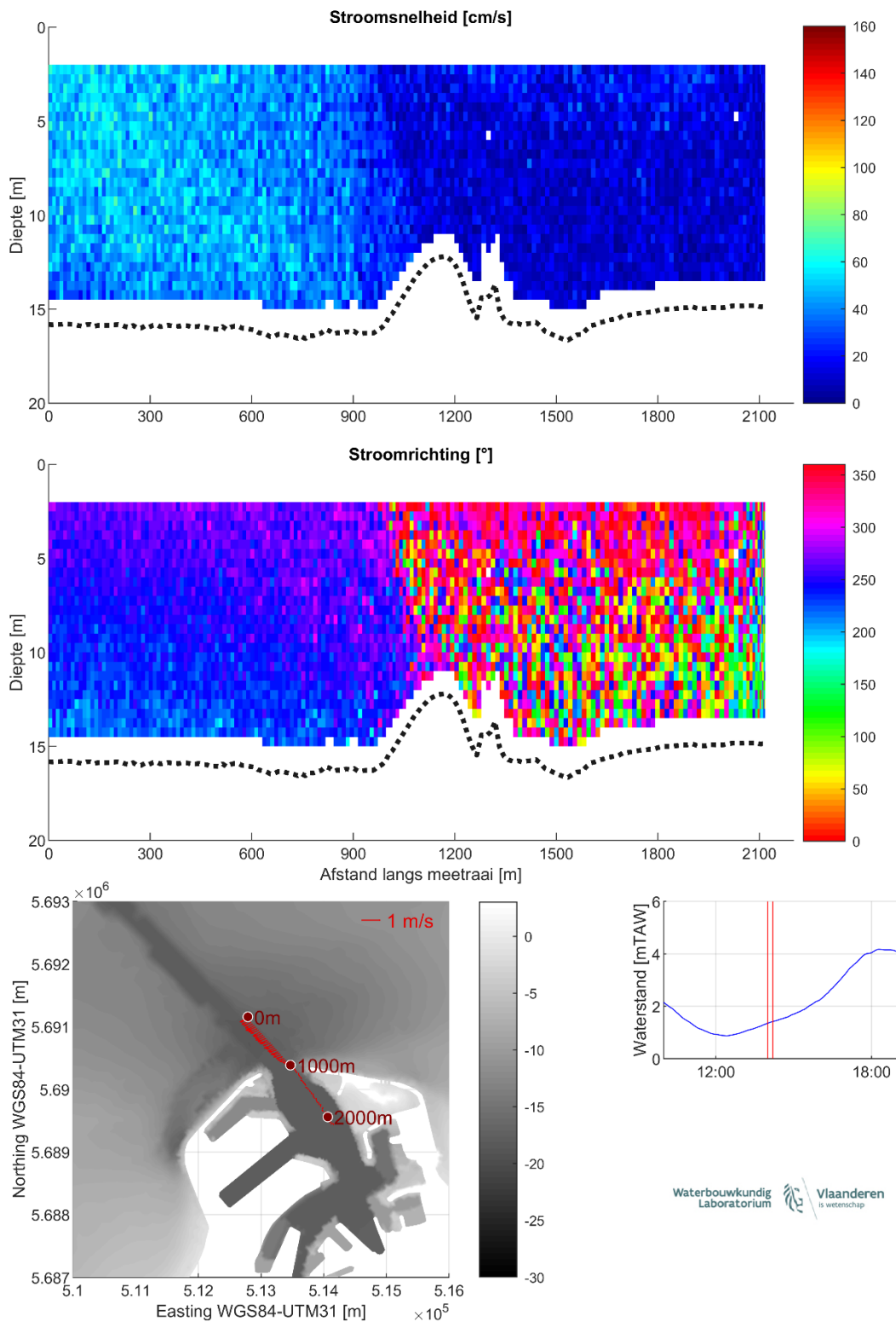
Figuur 19 – Stroomgegevens 23/08/2023 raai 14: snelheids grootte (top), -richting (midden) en diepte-gemiddelde vectoren (onder)
