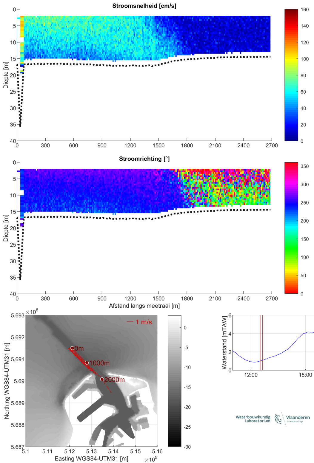
Figuur 15 – Stroomgegevens 23/08/2023 raai 10: snelheids grootte (top), -richting (midden) en diepte-gemiddelde vectoren (onder)
