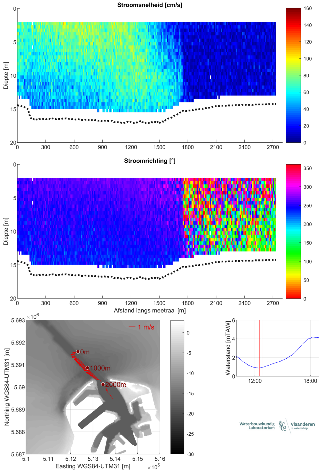
Figuur 13 – Stroomgegevens 23/08/2023 raai 8: snelheids grootte (top), -richting (midden) en diepte-gemiddelde vectoren (onder)
