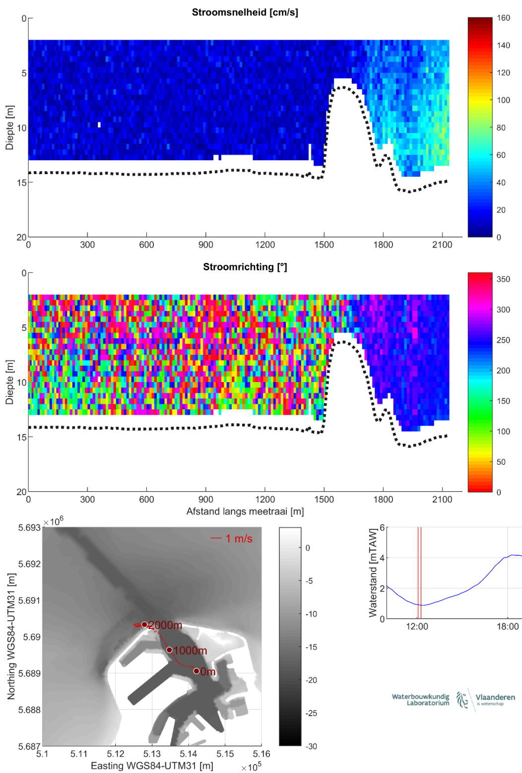
Figuur 10 – Stroomgegevens 23/08/2023 raai 5: snelheids grootte (top), -richting (midden) en diepte-gemiddelde vectoren (onder)
