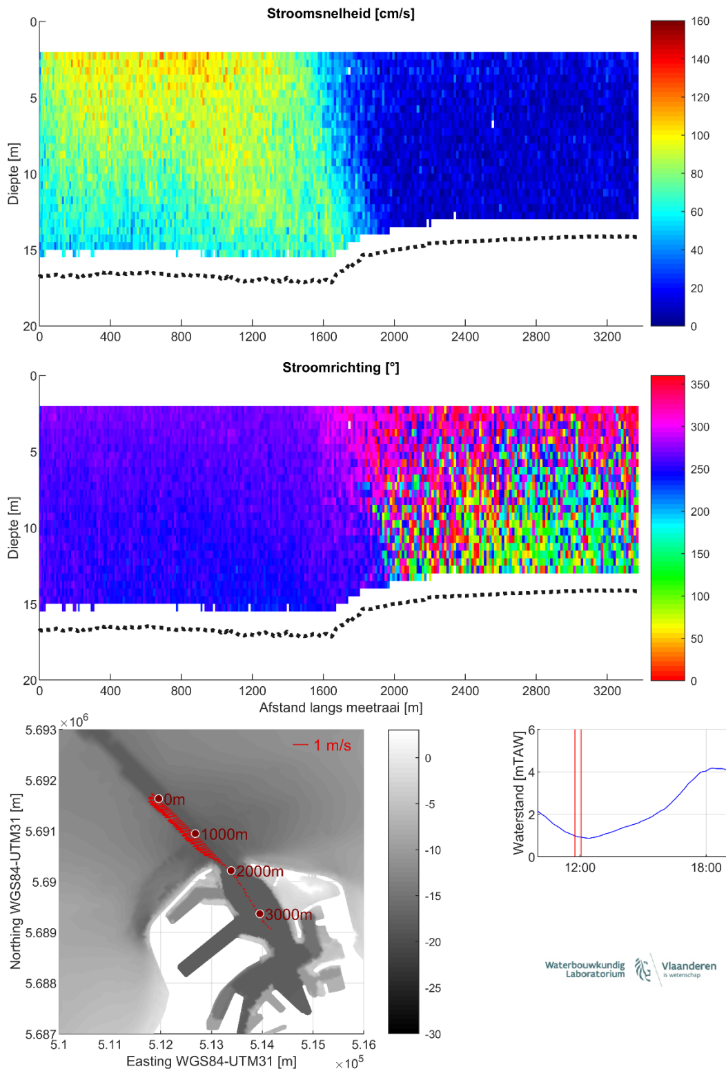
Figuur 9 – Stroomgegevens 23/08/2023 raai 4: snelheidsgrootte (top), -richting (midden) en diepte-gemiddelde vectoren (onder)
