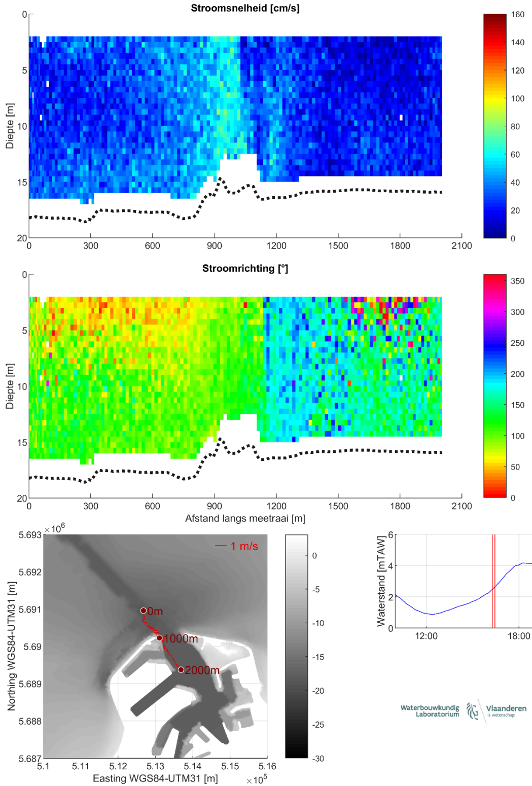
Figuur 29 – Stroomgegevens 23/08/2023 raai 24: snelheids grootte (top), -richting (midden) en diepte-gemiddelde vectoren (onder)
