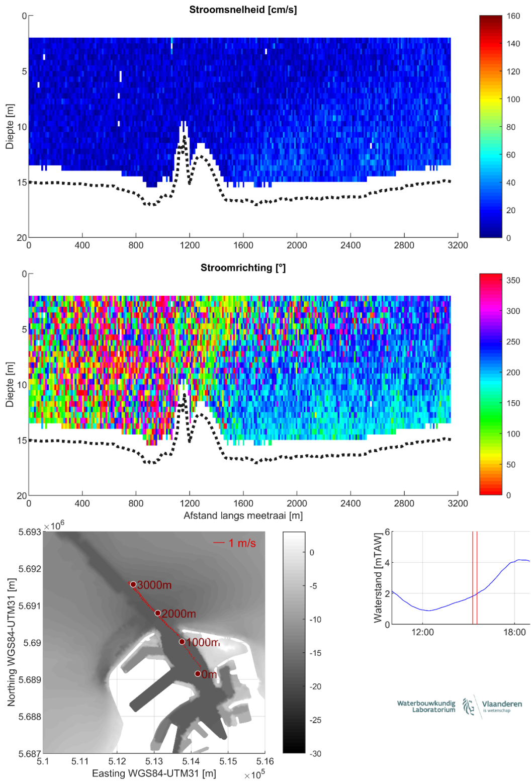
Figuur 24 – Stroomgegevens 23/08/2023 raai 19: snelheids grootte (top), -richting (midden) en diepte-gemiddelde vectoren (onder)
