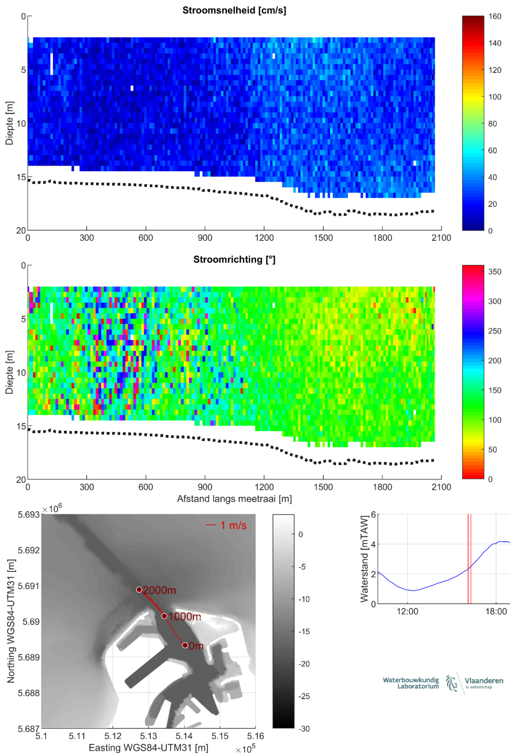
Figuur 28 – Stroomgegevens 23/08/2023 raai 23: snelheids grootte (top), -richting (midden) en diepte-gemiddelde vectoren (onder)
