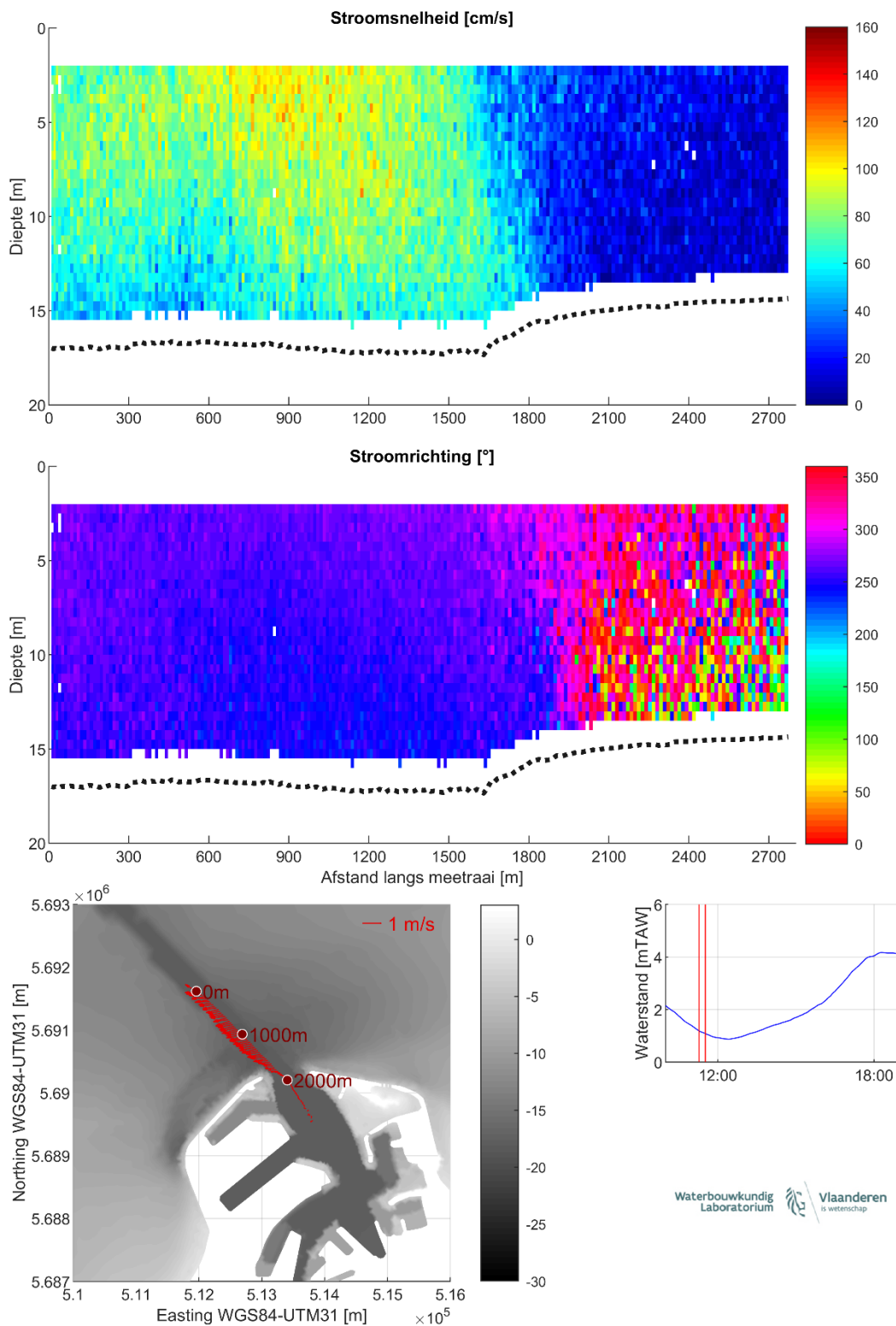
Figuur 7 – Stroomgegevens 23/08/2023 raai 2: snelheids-grootte (top), -richting (midden) en diepte-gemiddelde vectoren (onder)
