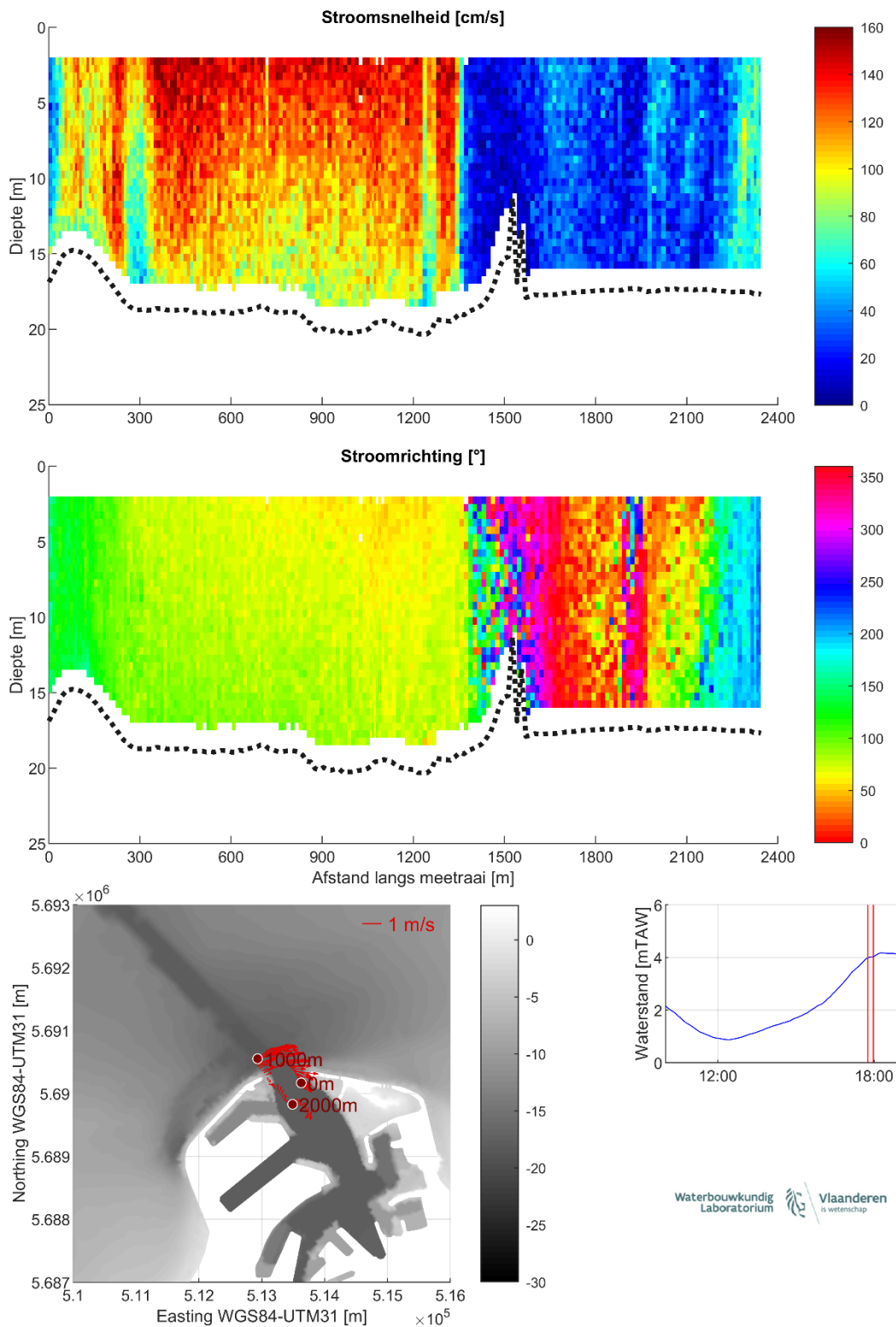
Figuur 34 – Stroomgegevens 23/08/2023 raai 29: snelheids grootte (top), -richting (midden) en diepte-gemiddelde vectoren (onder)
