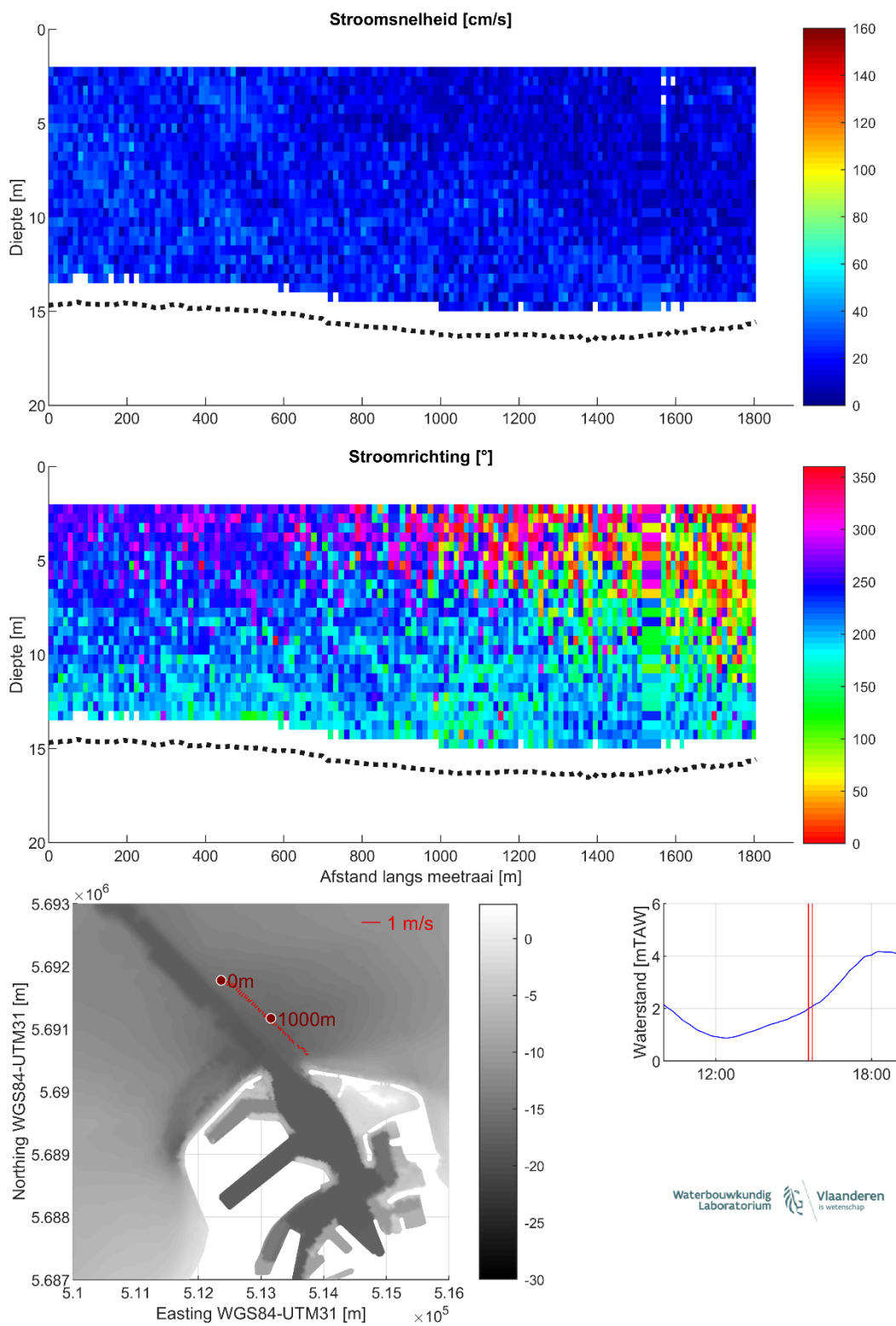
Figuur 25 – Stroomgegevens 23/08/2023 raai 20: snelheids grootte (top), -richting (midden) en diepte-gemiddelde vectoren (onder)
