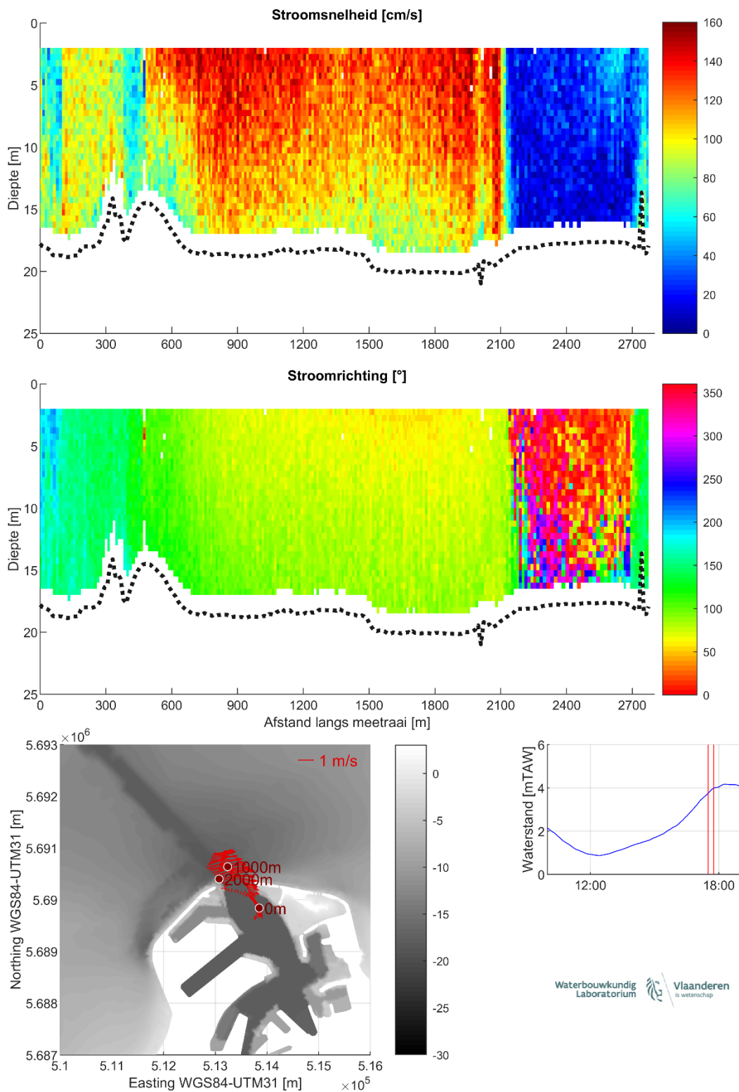
Figuur 33 – Stroomgegevens 23/08/2023 raai 28: snelheids grootte (top), -richting (midden) en diepte-gemiddelde vectoren (onder)
