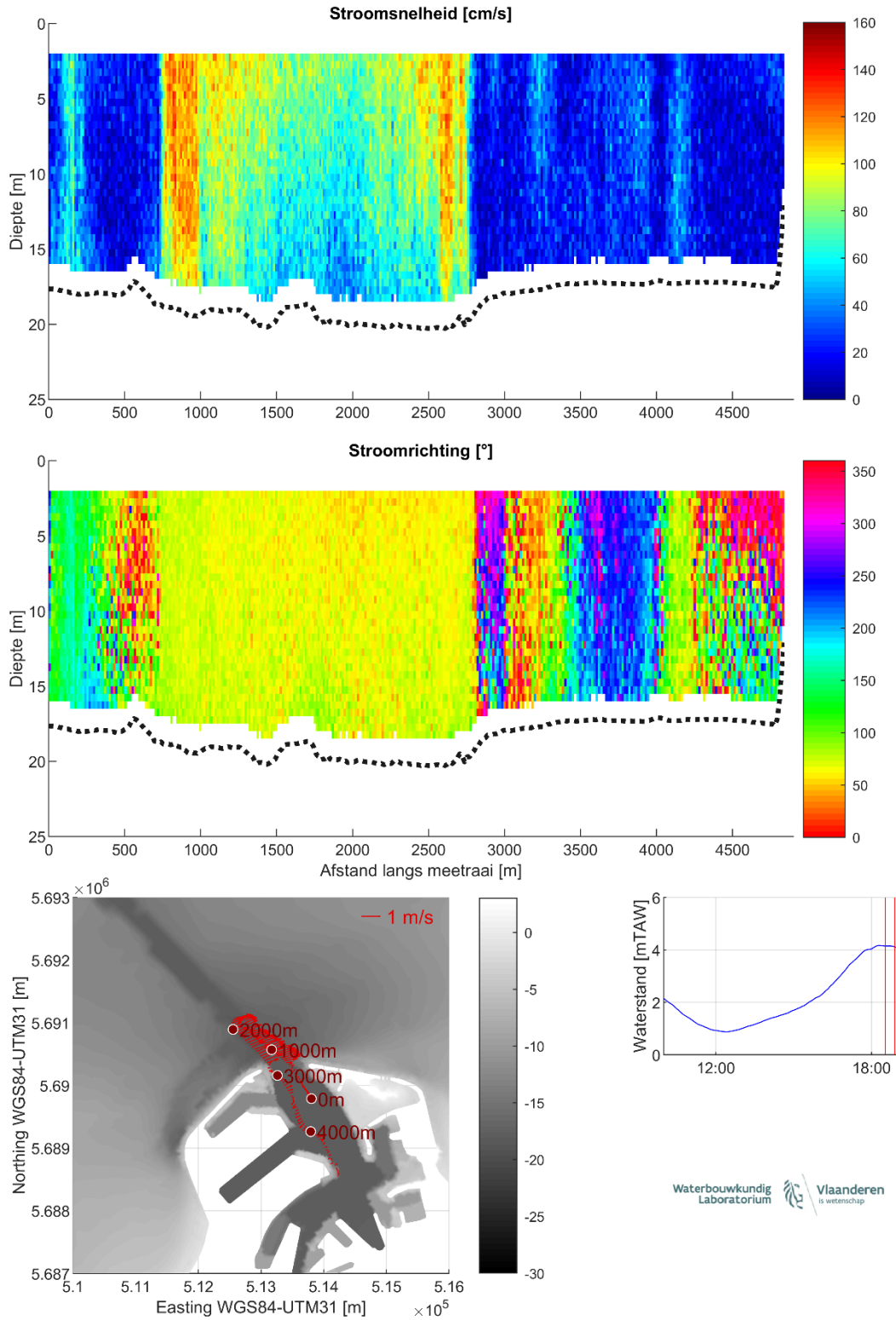
Figuur 37 – Stroomgegevens 23/08/2023 raai 32: snelheids grootte (top), -richting (midden) en diepte-gemiddelde vectoren (onder)
