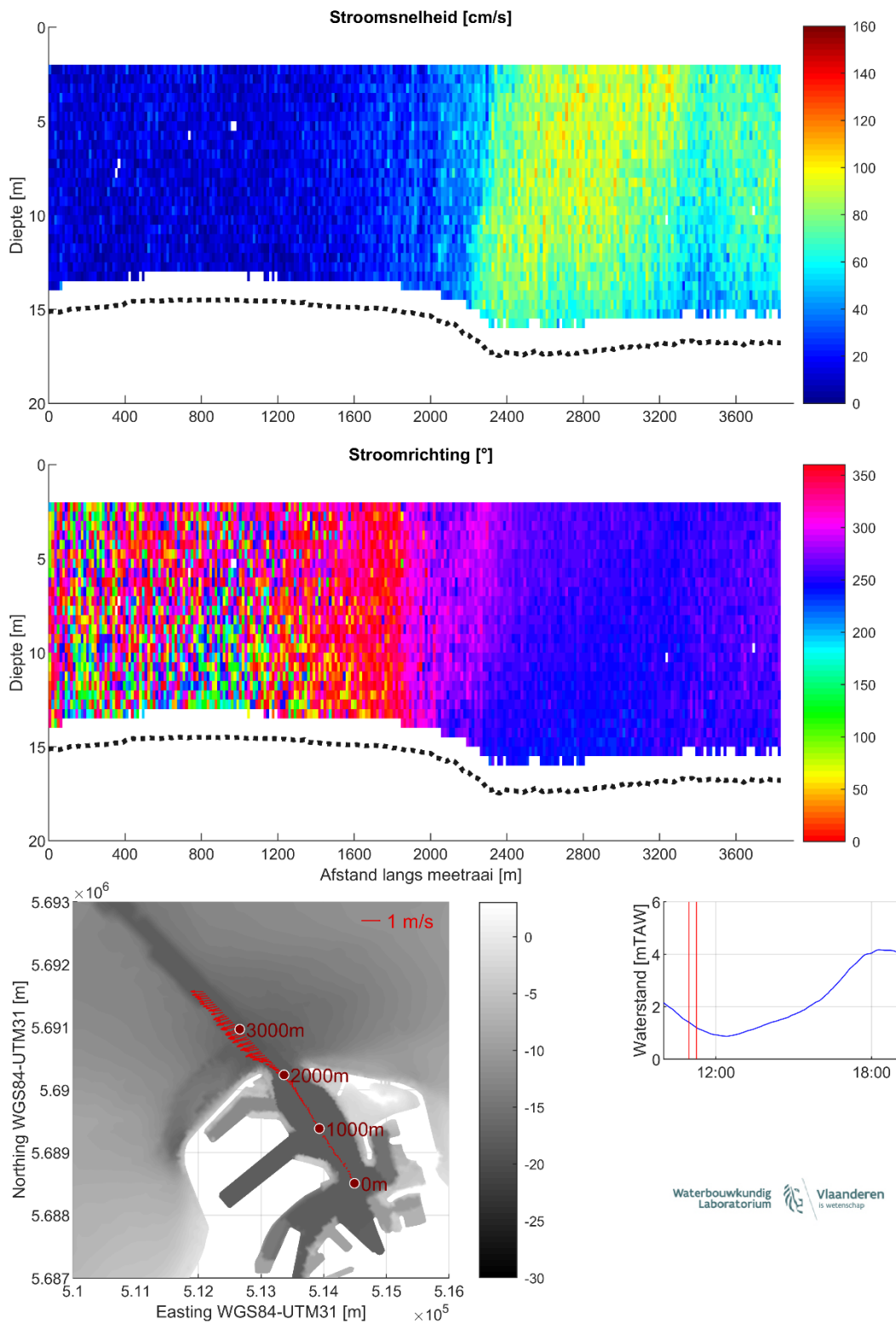
Figuur 6 – Stroomgegevens 23/08/2023 raai 1: snelheids grootte (top), -richting (midden) en diepte-gemiddelde vectoren (onder)
