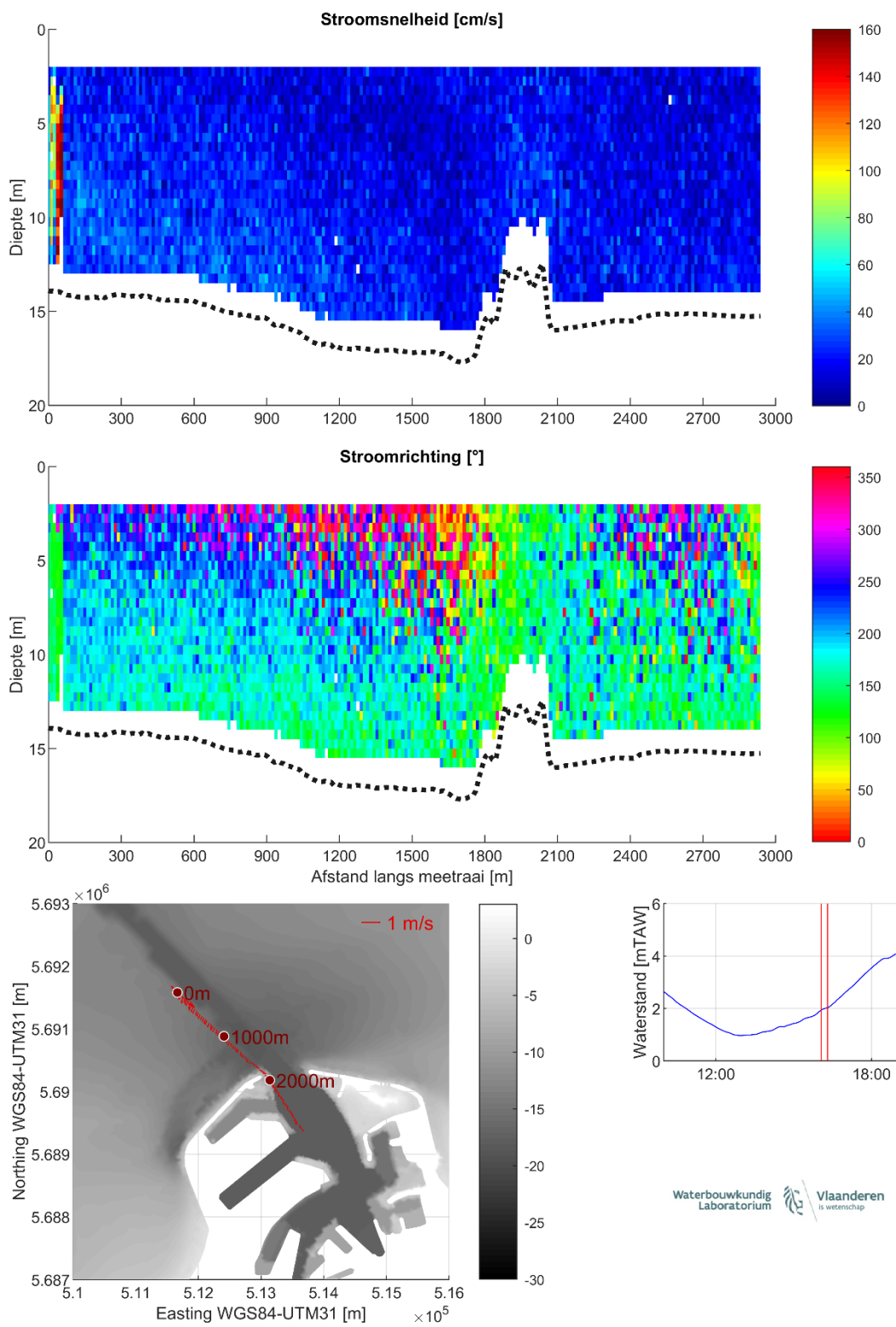
Figuur 25 – Stroomgegevens 24/08/2023 raai 20: snelheids grootte (top), -richting (midden) en diepte-gemiddelde vectoren (onder)
