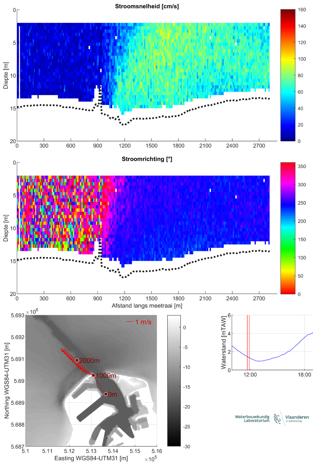
Figuur 10 – Stroomgegevens 24/08/2023 raai 5: snelheids grootte (top), -richting (midden) en diepte-gemiddelde vectoren (onder)
