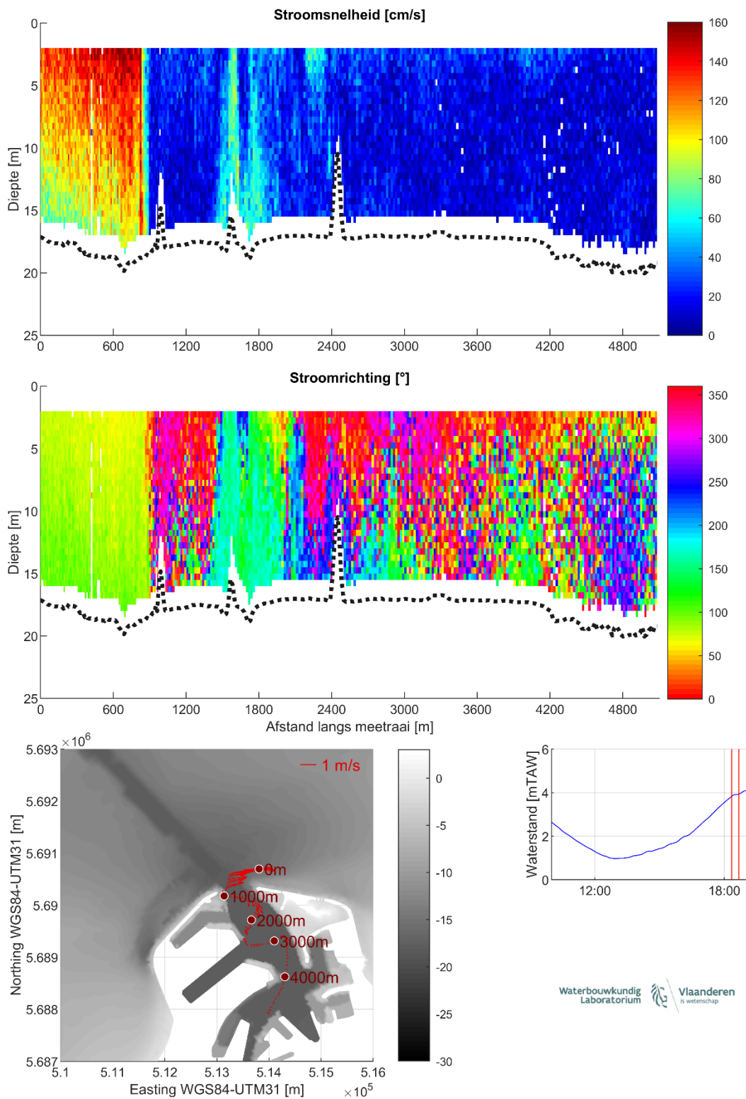
Figuur 34 – Stroomgegevens 24/08/2023 raai 29: snelheids grootte (top), -richting (midden) en diepte-gemiddelde vectoren (onder)
