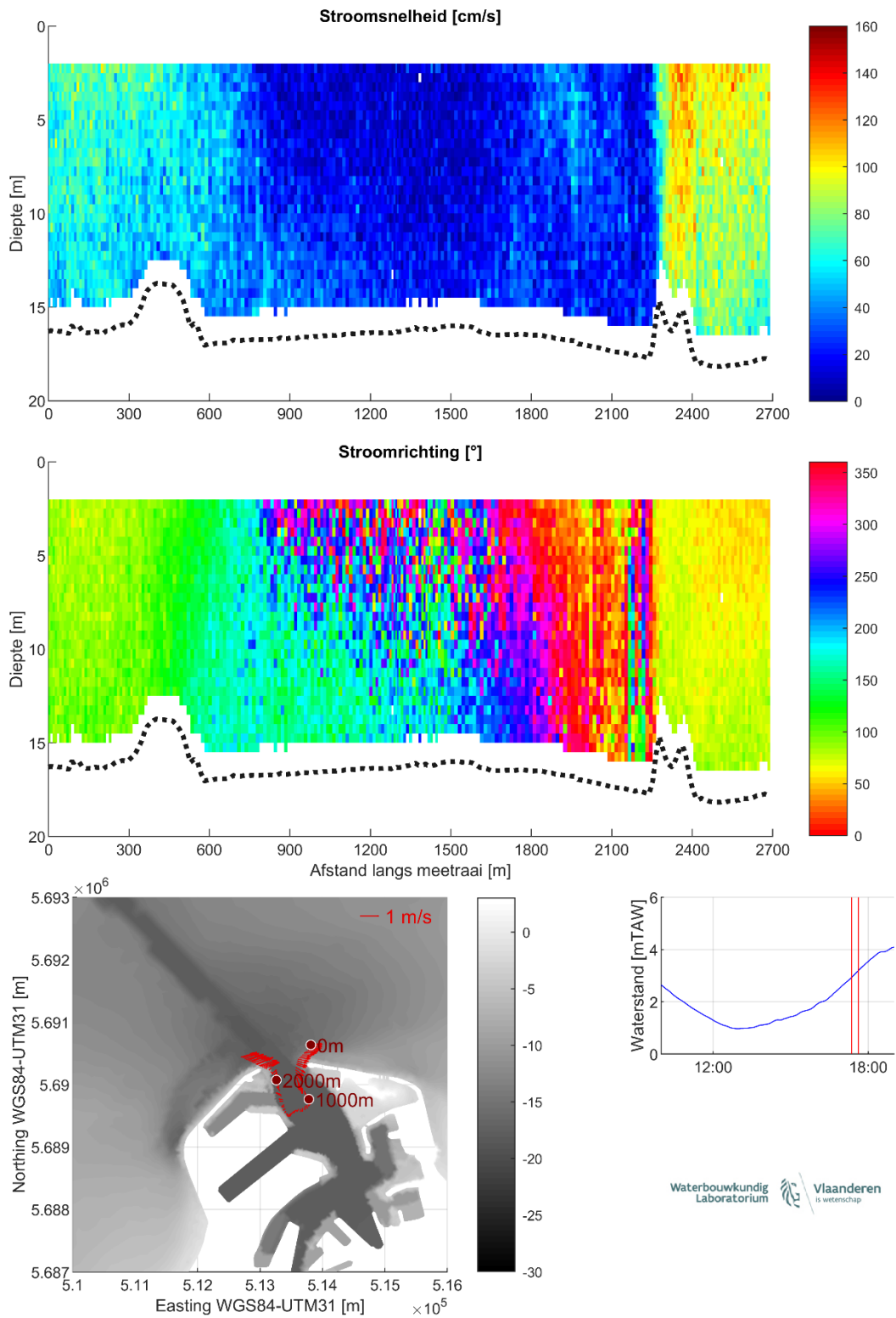
Figuur 30 – Stroomgegevens 24/08/2023 raai 25: snelheids grootte (top), -richting (midden) en diepte-gemiddelde vectoren (onder)
