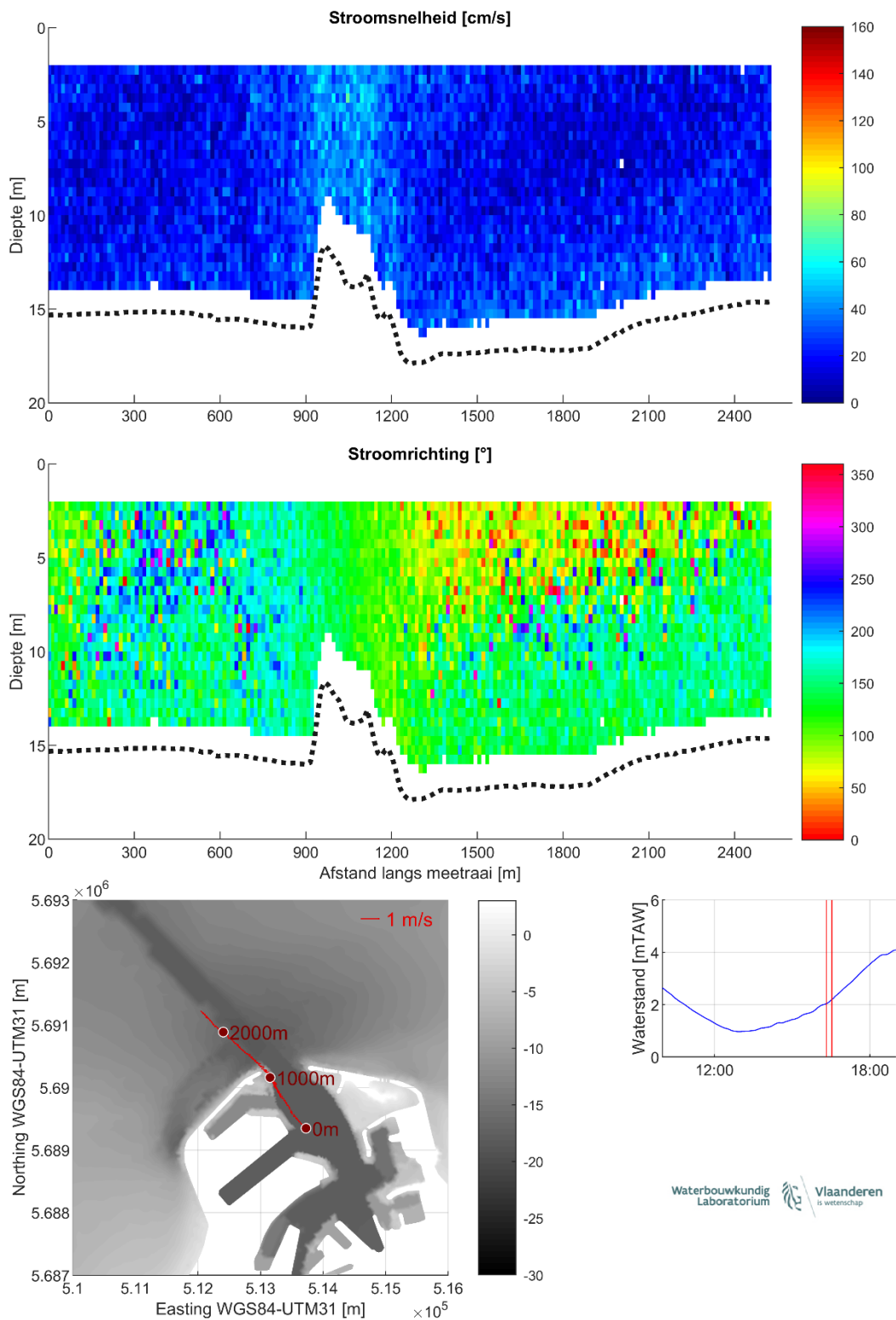
Figuur 26 – Stroomgegevens 24/08/2023 raai 21: snelheids grootte (top), -richting (midden) en diepte-gemiddelde vectoren (onder)
