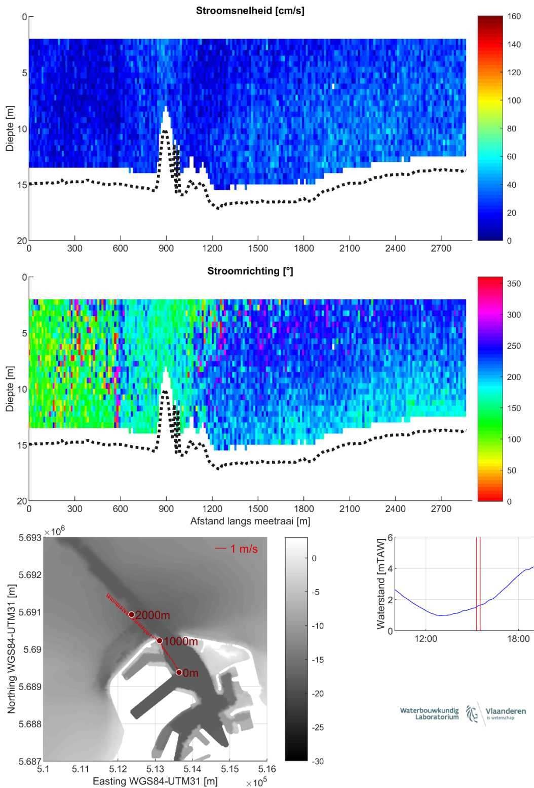
Figuur 22 – Stroomgegevens 24/08/2023 raai 17: snelheids grootte (top), -richting (midden) en diepte-gemiddelde vectoren (onder)
