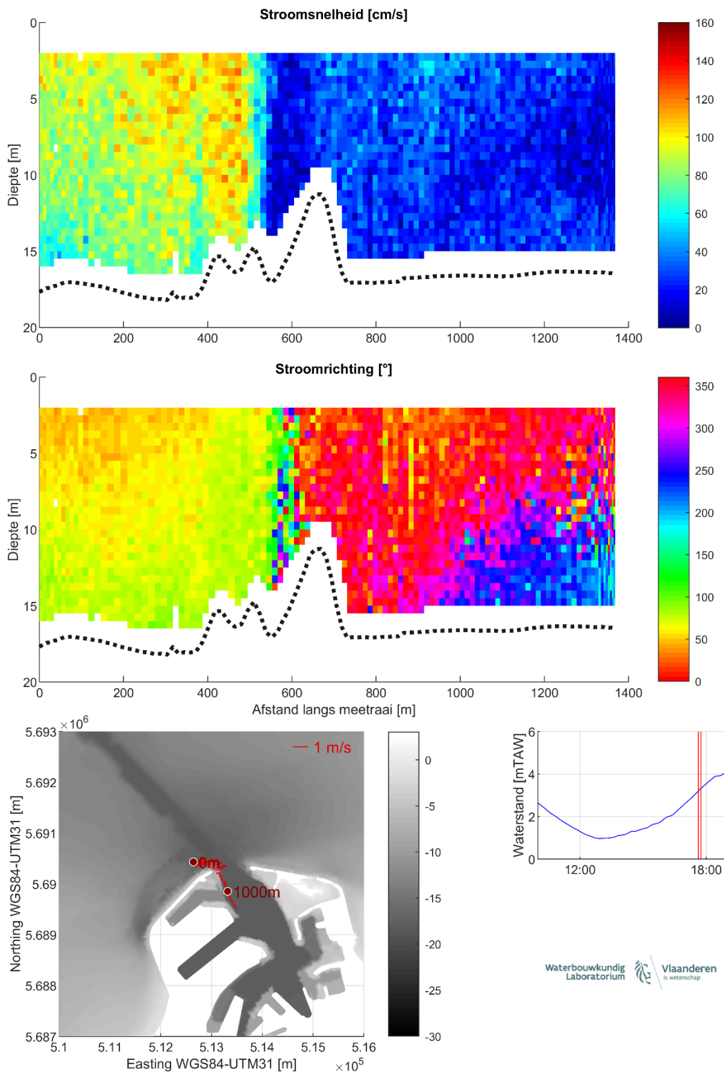
Figuur 31 – Stroomgegevens 24/08/2023 raai 26: snelheids grootte (top), -richting (midden) en diepte-gemiddelde vectoren (onder)
