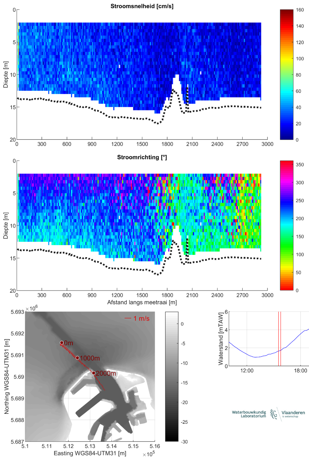
Figuur 23 – Stroomgegevens 24/08/2023 raai 18: snelheids grootte (top), -richting (midden) en diepte-gemiddelde vectoren (onder)
