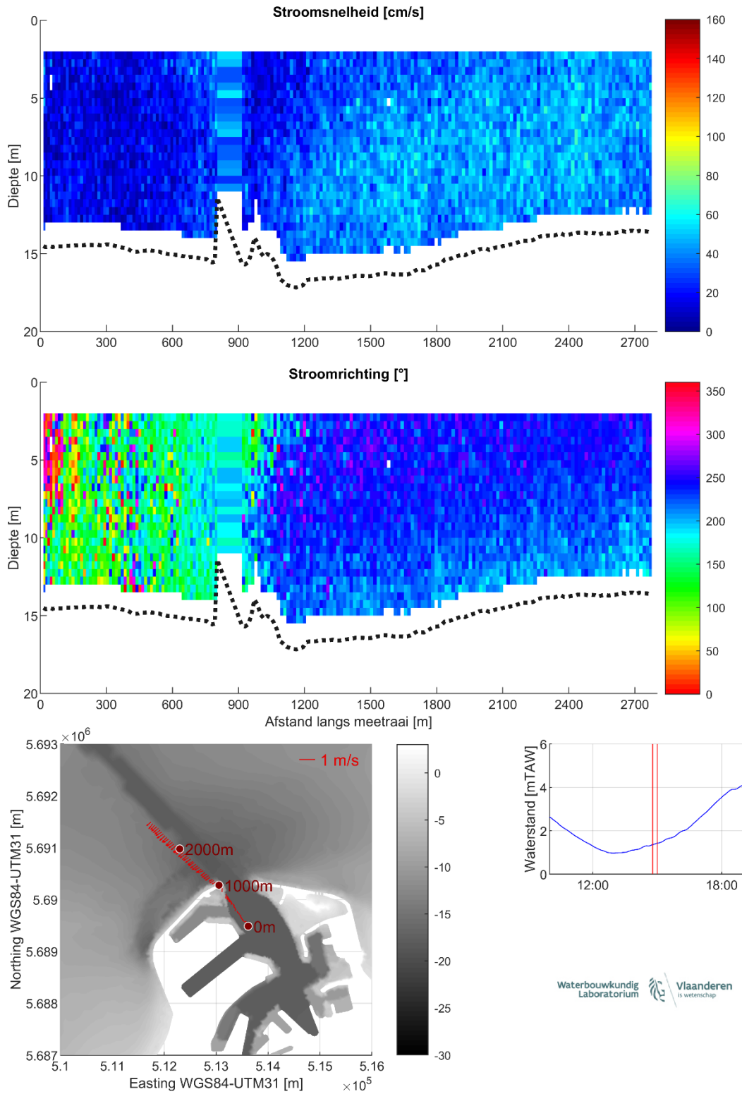
Figuur 20 – Stroomgegevens 24/08/2023 raai 15: snelheids grootte (top), -richting (midden) en diepte-gemiddelde vectoren (onder)
