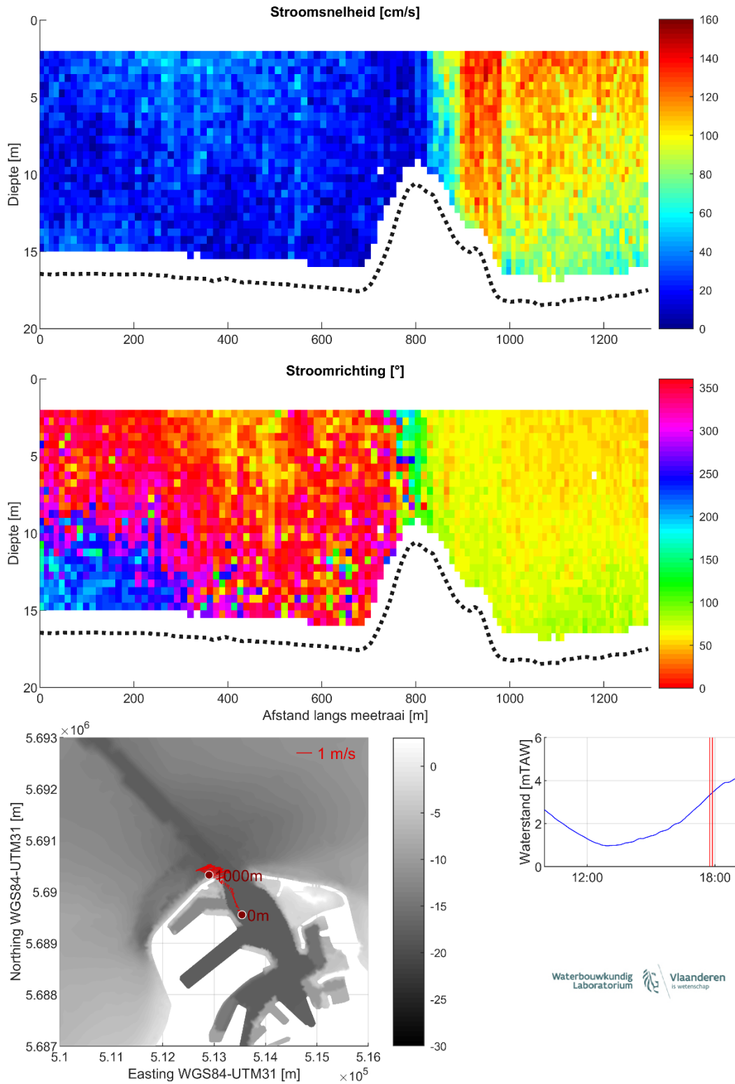
Figuur 32 – Stroomgegevens 24/08/2023 raai 27: snelheids grootte (top), -richting (midden) en diepte-gemiddelde vectoren (onder)
