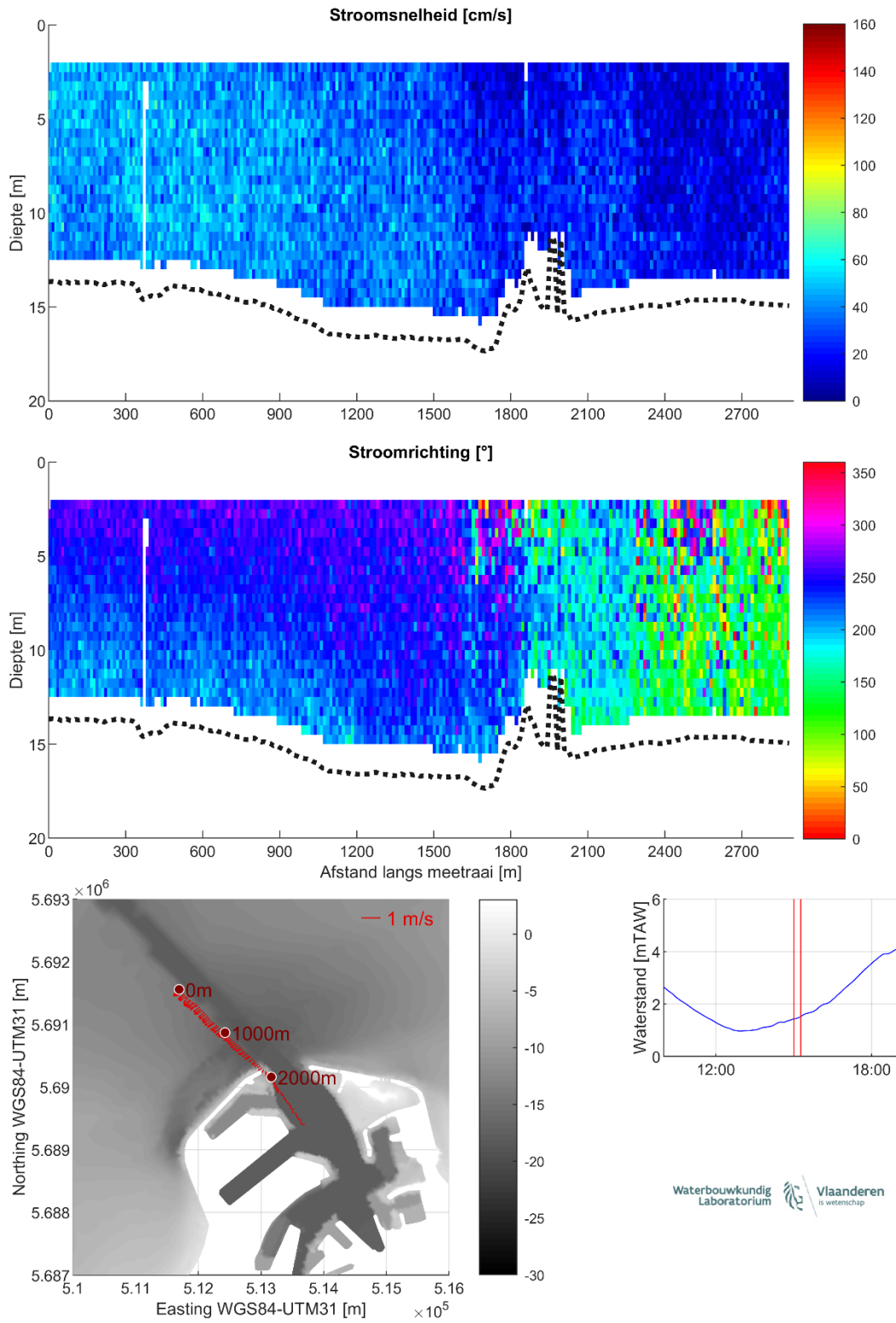
Figuur 21 – Stroomgegevens 24/08/2023 raai 16: snelheids grootte (top), -richting (midden) en diepte-gemiddelde vectoren (onder)
