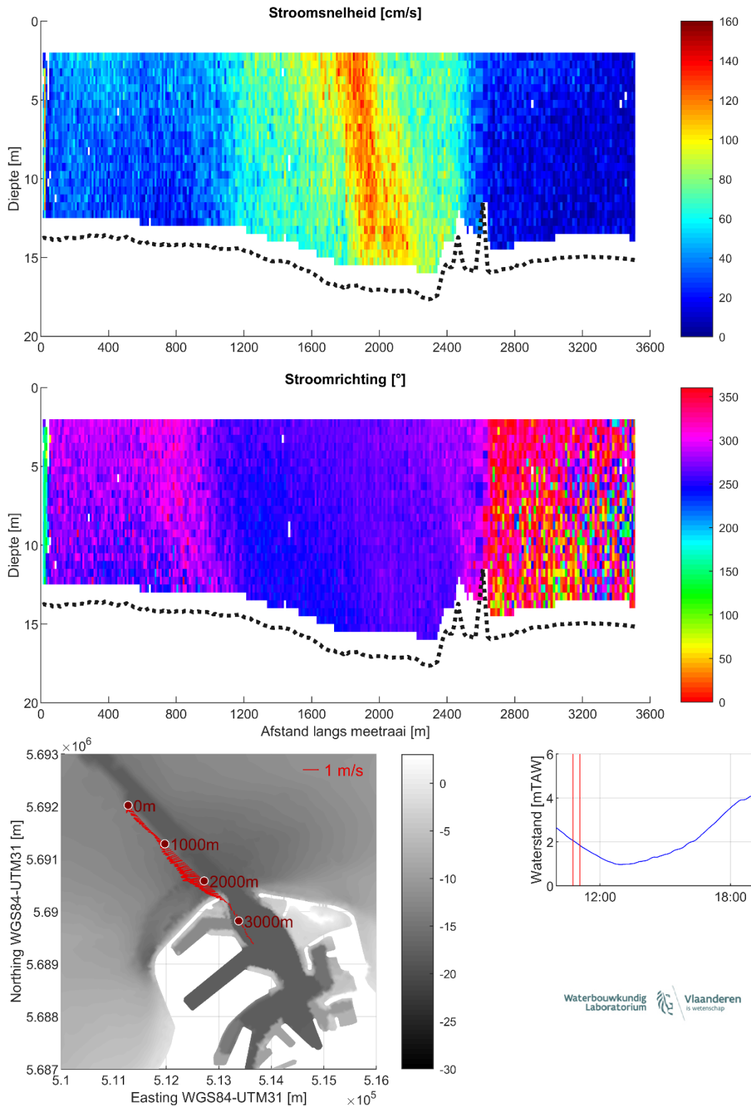
Figuur 7 – Stroomgegevens 24/08/2023 raai 2: snelheidsgrootte (top), -richting (midden) en diepte-gemiddelde vectoren (onder)
