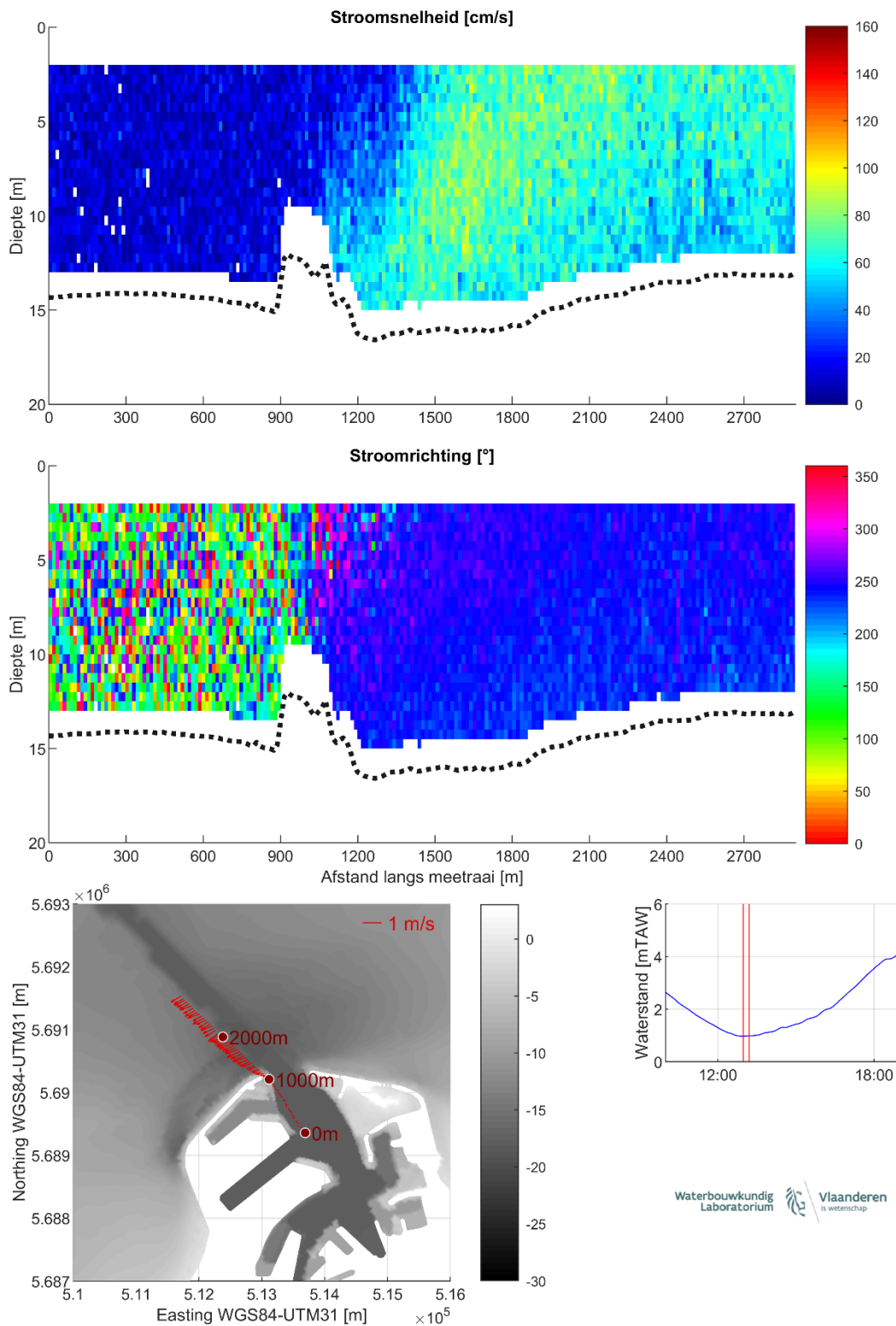
Figuur 14 – Stroomgegevens 24/08/2023 raai 9: snelheids grootte (top), -richting (midden) en diepte-gemiddelde vectoren (onder)
