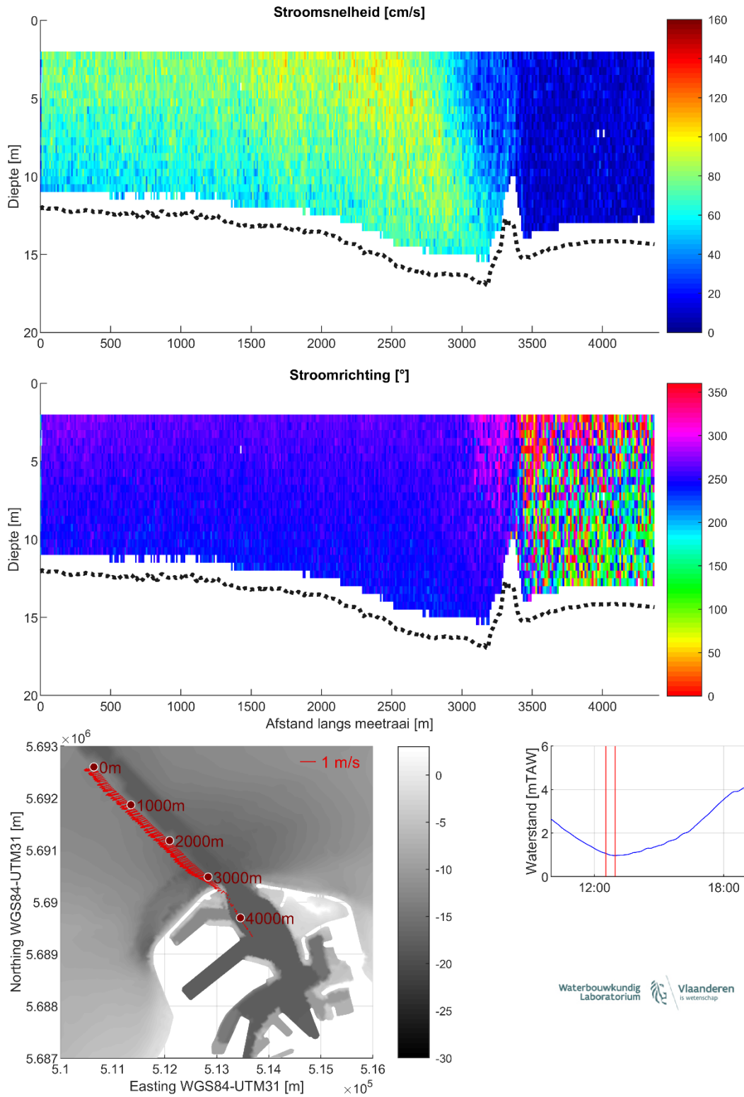
Figuur 13 – Stroomgegevens 24/08/2023 raai 8: snelheids grootte (top), -richting (midden) en diepte-gemiddelde vectoren (onder)
