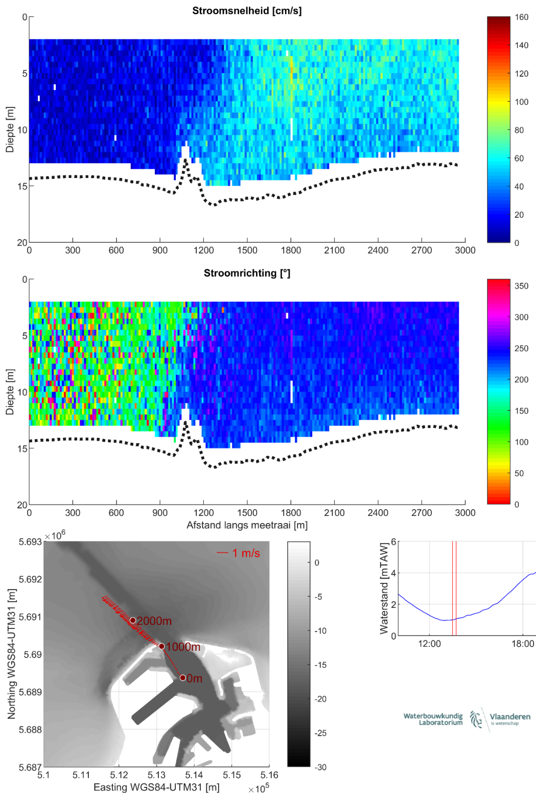
Figuur 16 – Stroomgegevens 24/08/2023 raai 11: snelheids grootte (top), -richting (midden) en diepte-gemiddelde vectoren (onder)
