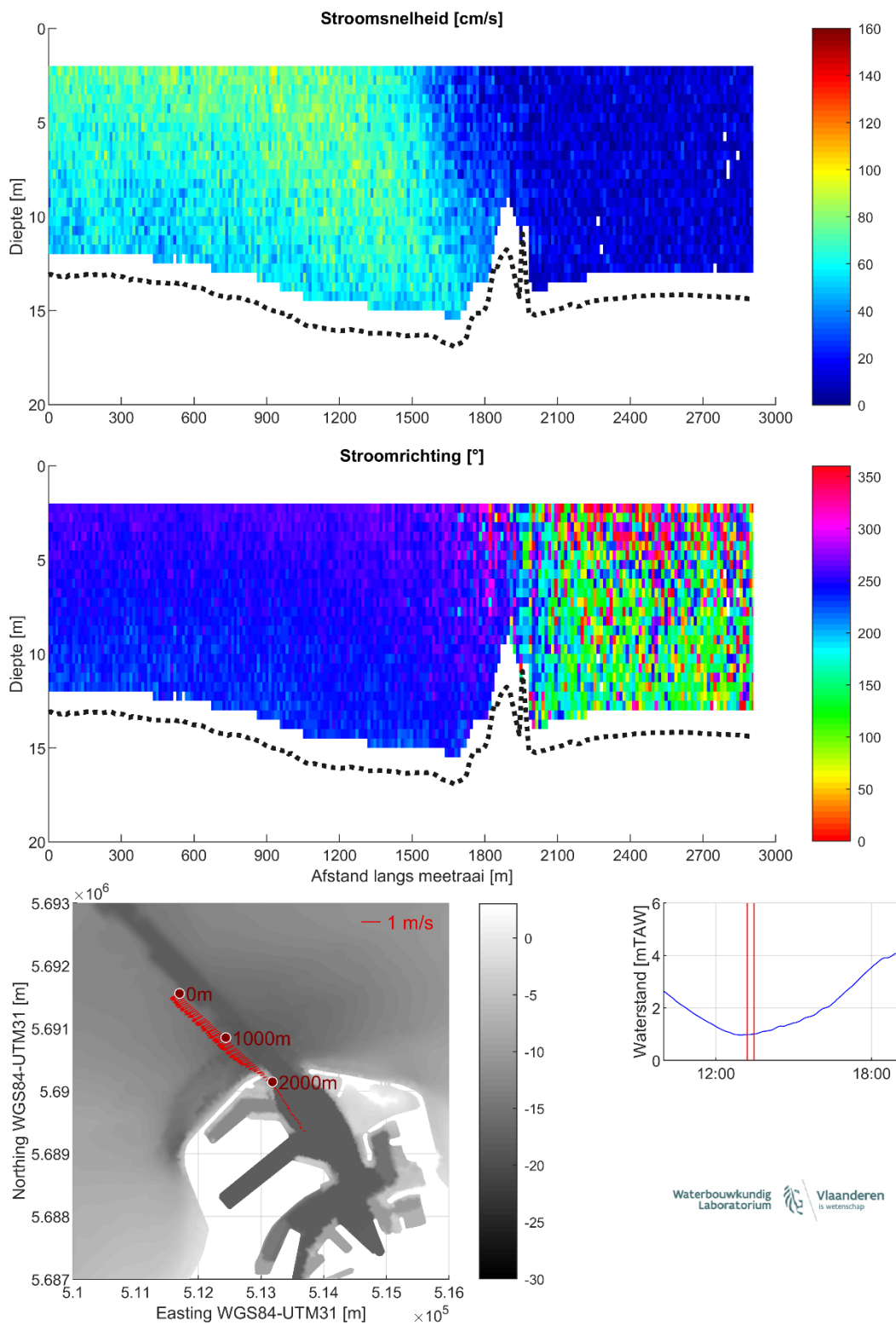
Figuur 15 – Stroomgegevens 24/08/2023 raai 10: snelheids grootte (top), -richting (midden) en diepte-gemiddelde vectoren (onder)
