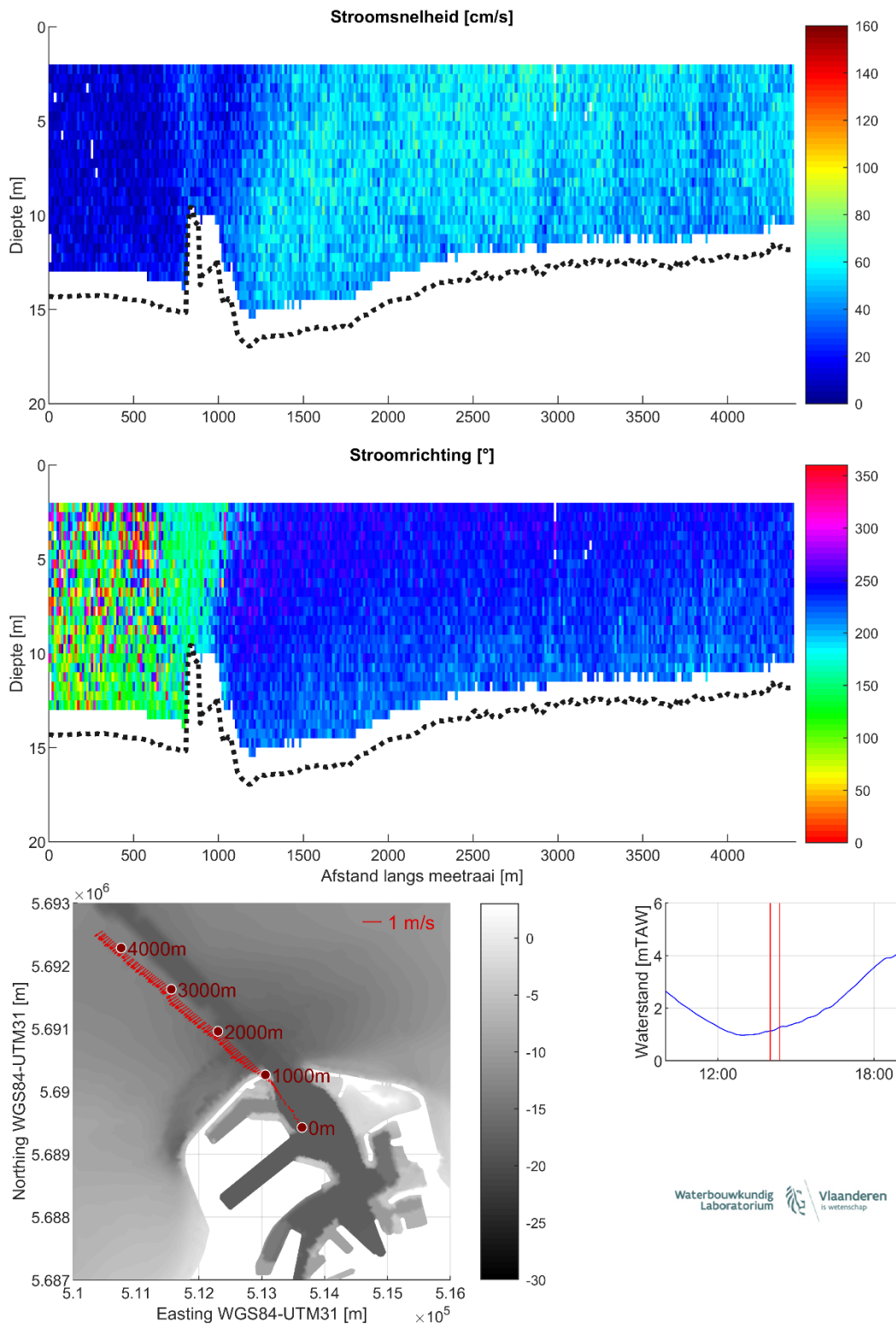
Figuur 18 – Stroomgegevens 24/08/2023 raai 13: snelheids grootte (top), -richting (midden) en diepte-gemiddelde vectoren (onder)
