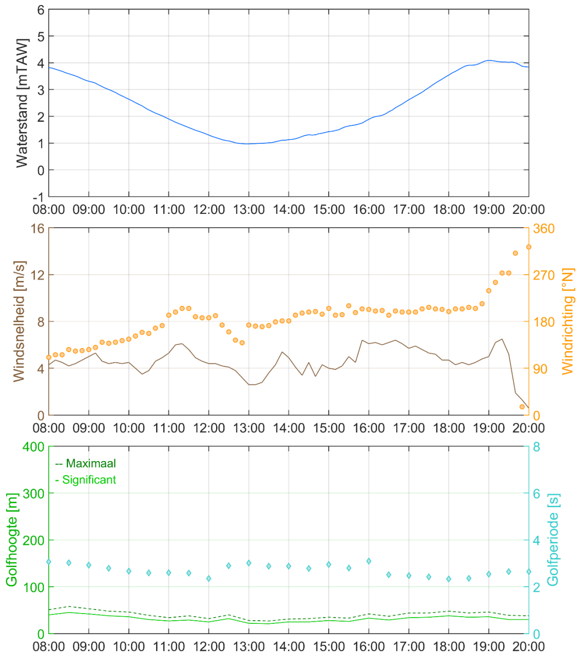
Figuur 5 – Verloop van de omgevingscondities tijdens meetcampagne Waterstand te Zeebrugge Leopold II-dam (boven) | wind te Zeebrugge Januskop (midden) | golfcondities te Bol van Heist (onder)
