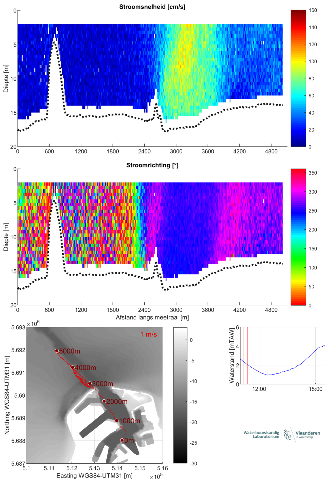
Figuur 6 – Stroomgegevens 24/08/2023 raai 1: snelheidsgrootte (top), -richting (midden) en diepte-gemiddelde vectoren (onder)
