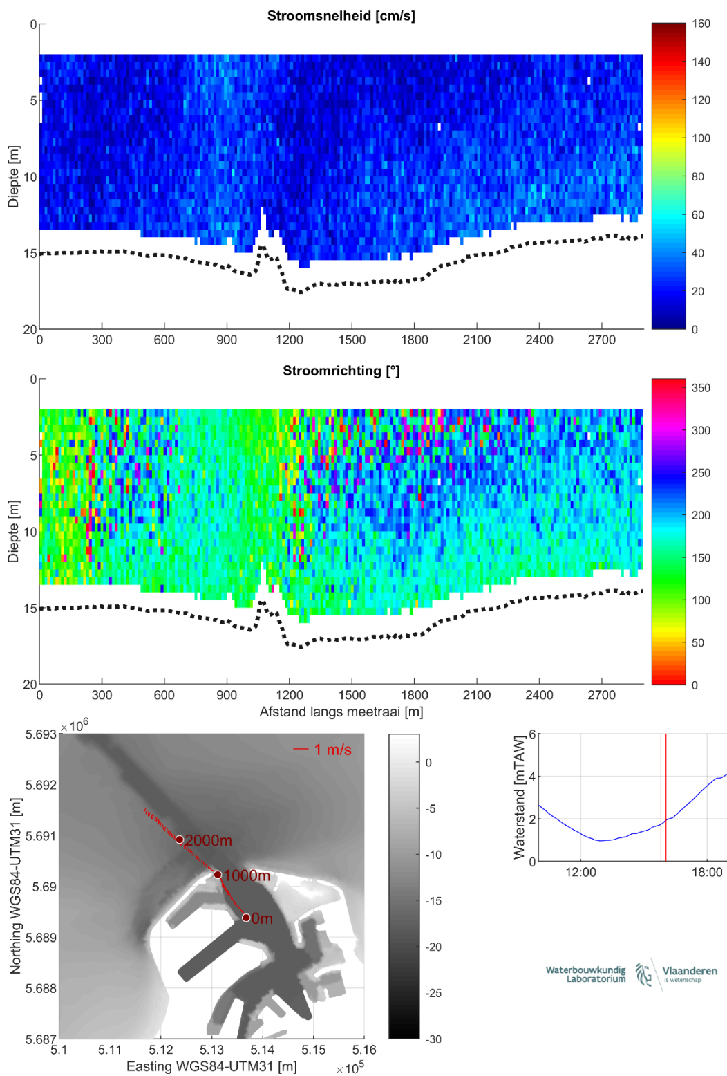
Figuur 24 – Stroomgegevens 24/08/2023 raai 19: snelheids grootte (top), -richting (midden) en diepte-gemiddelde vectoren (onder)
