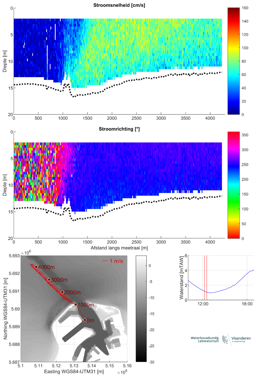
Figuur 12 – Stroomgegevens 24/08/2023 raai 7: snelheids grootte (top), -richting (midden) en diepte-gemiddelde vectoren (onder)
