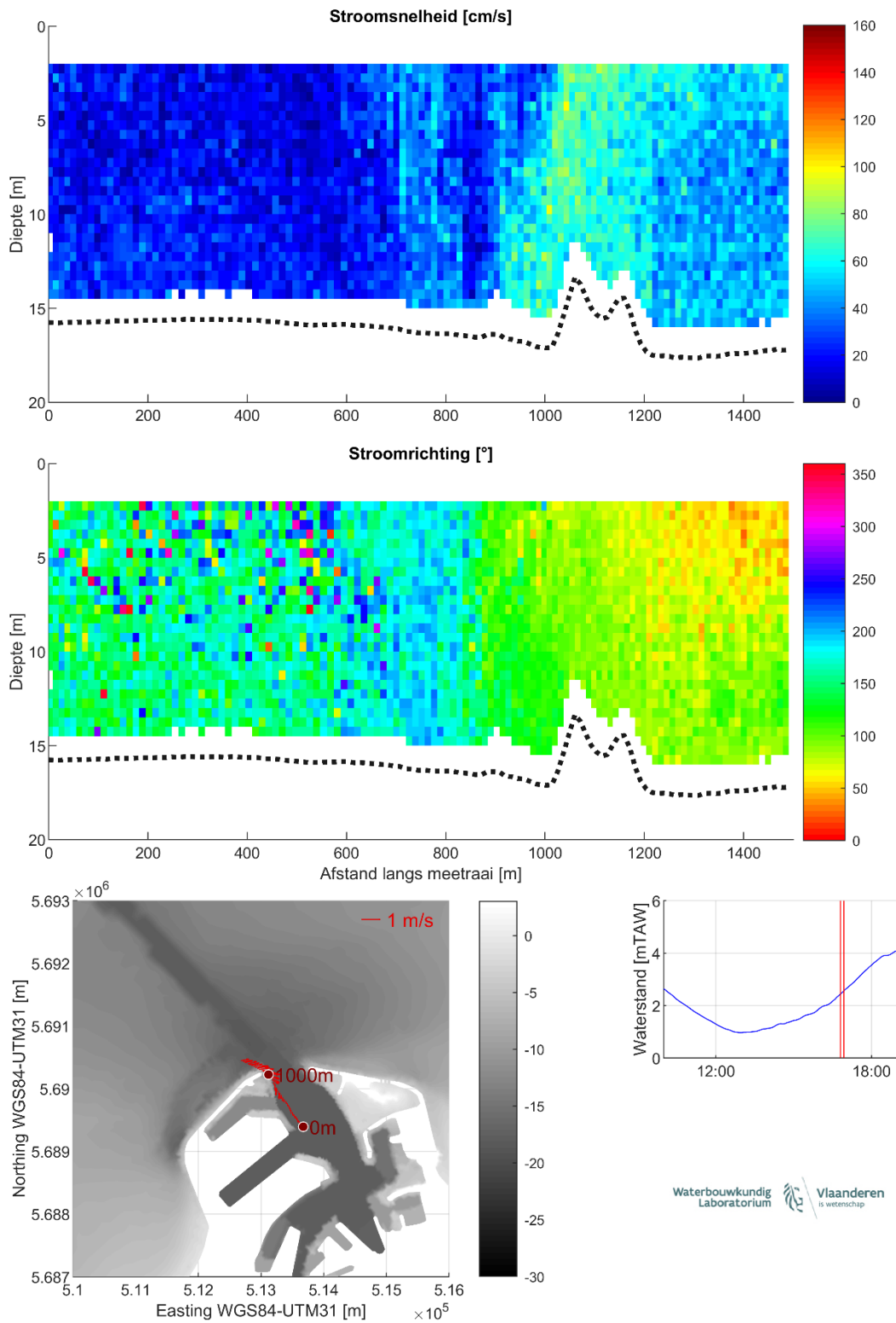
Figuur 28 – Stroomgegevens 24/08/2023 raai 23: snelheids grootte (top), -richting (midden) en diepte-gemiddelde vectoren (onder)
