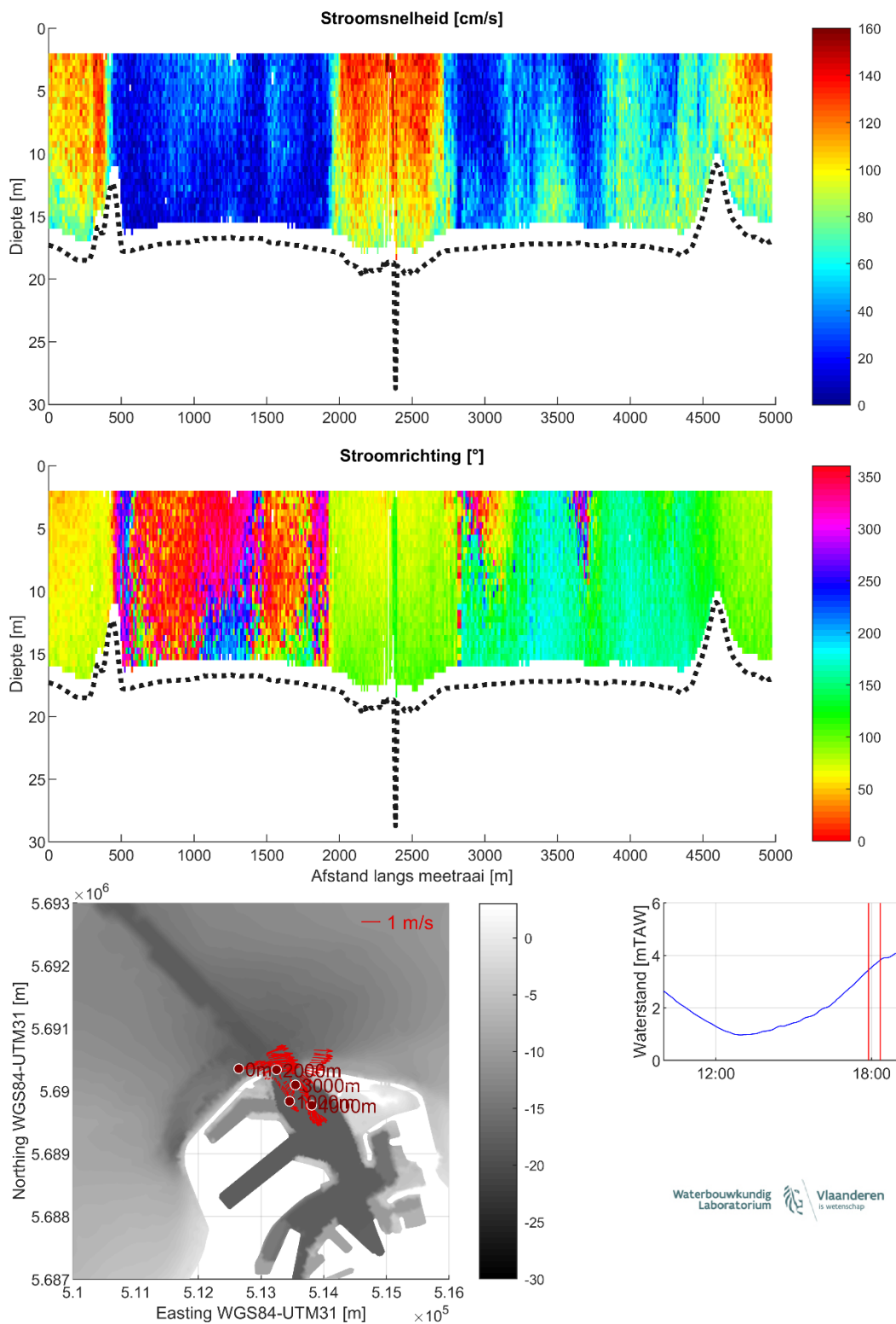
Figuur 33 – Stroomgegevens 24/08/2023 raai 28: snelheids grootte (top), -richting (midden) en diepte-gemiddelde vectoren (onder)
