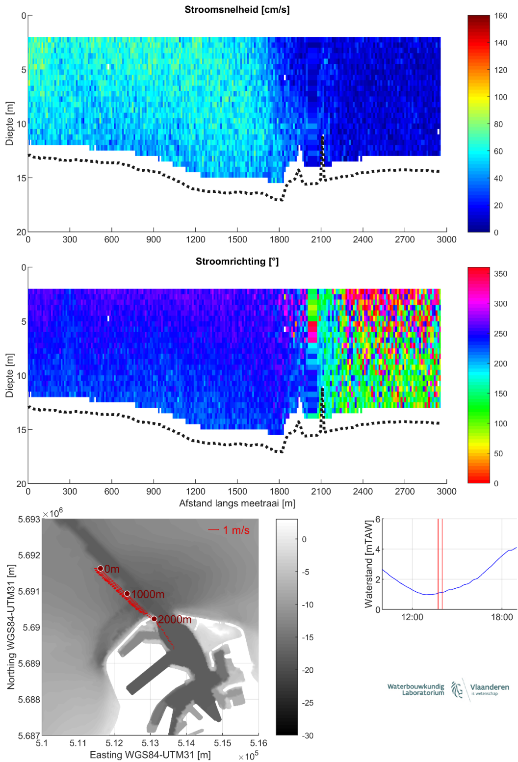
Figuur 17 – Stroomgegevens 24/08/2023 raai 12: snelheids grootte (top), -richting (midden) en diepte-gemiddelde vectoren (onder)
