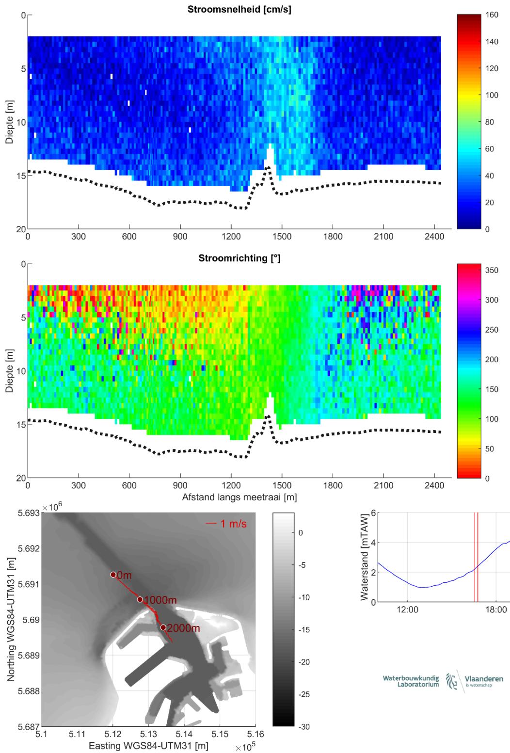
Figuur 27 – Stroomgegevens 24/08/2023 raai 22: snelheids grootte (top), -richting (midden) en diepte-gemiddelde vectoren (onder)
