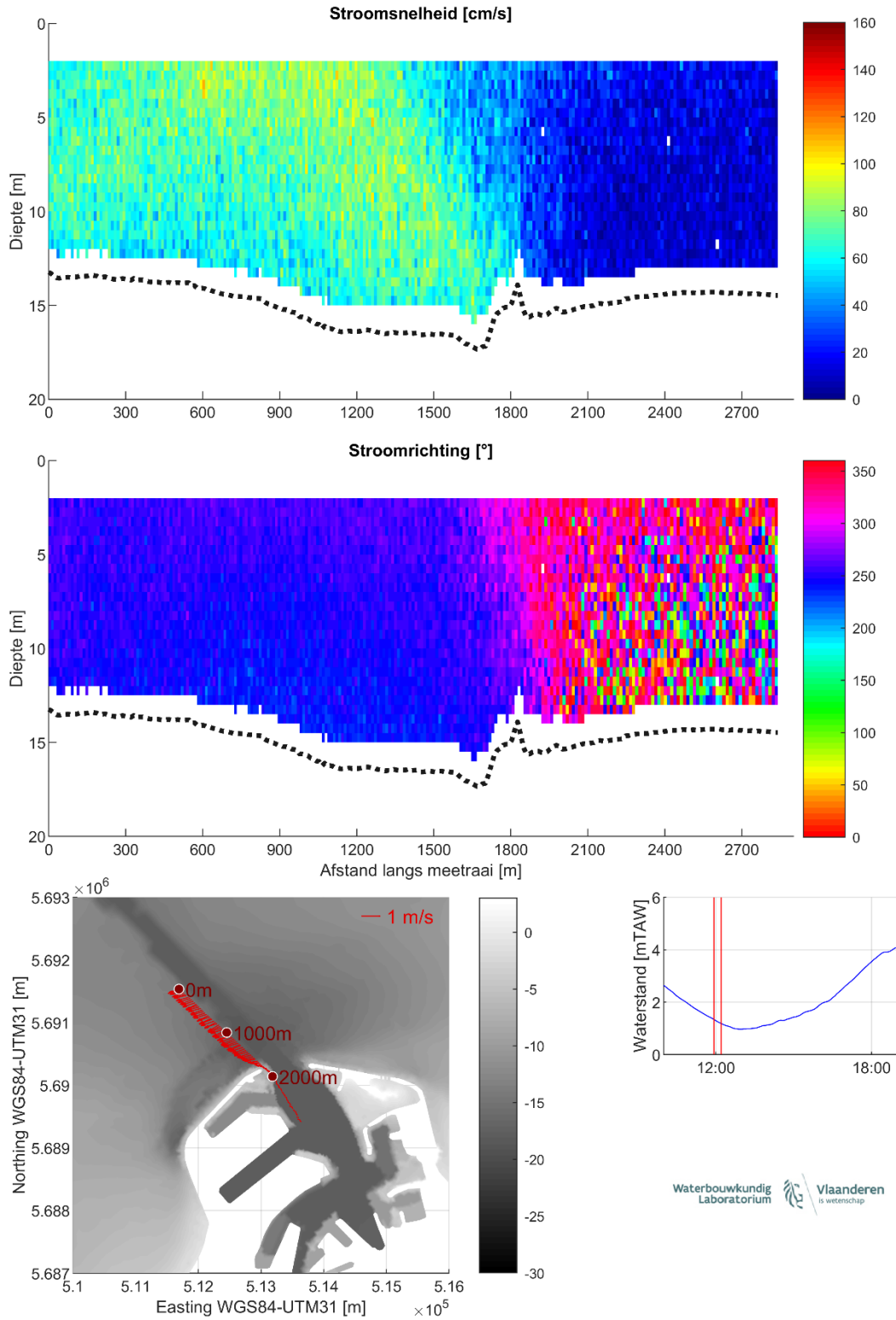
Figuur 11 – Stroomgegevens 24/08/2023 raai 6: snelheids grootte (top), -richting (midden) en diepte-gemiddelde vectoren (onder)
