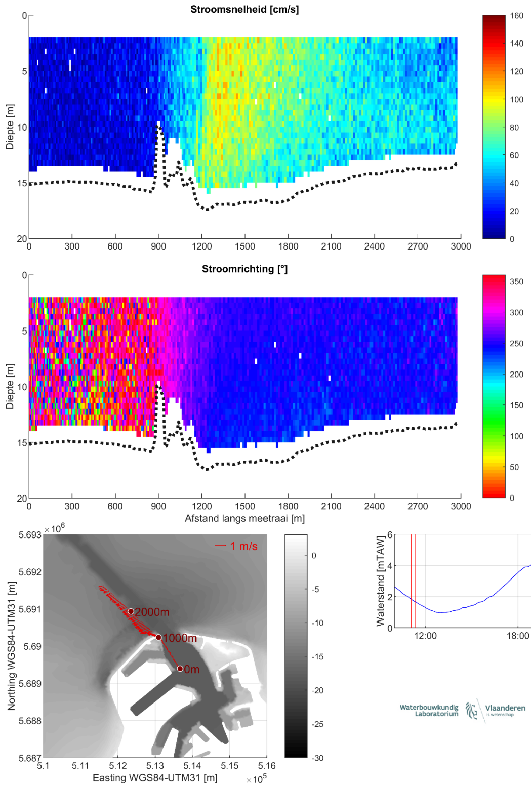
Figuur 8 – Stroomgegevens 24/08/2023 raai 3: snelheids grootte (top), -richting (midden) en diepte-gemiddelde vectoren (onder)
