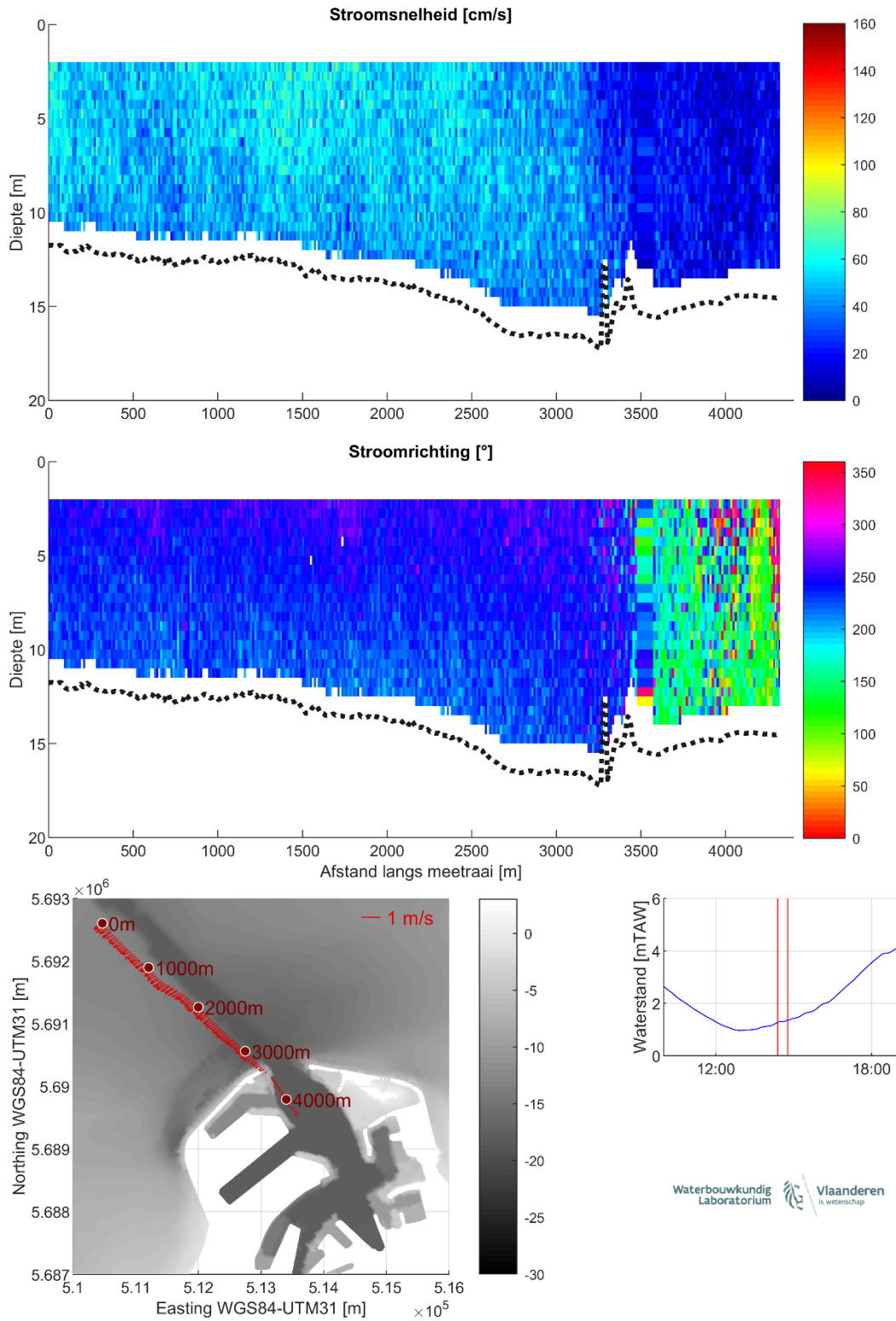
Figuur 19 – Stroomgegevens 24/08/2023 raai 14: snelheids grootte (top), -richting (midden) en diepte-gemiddelde vectoren (onder)
