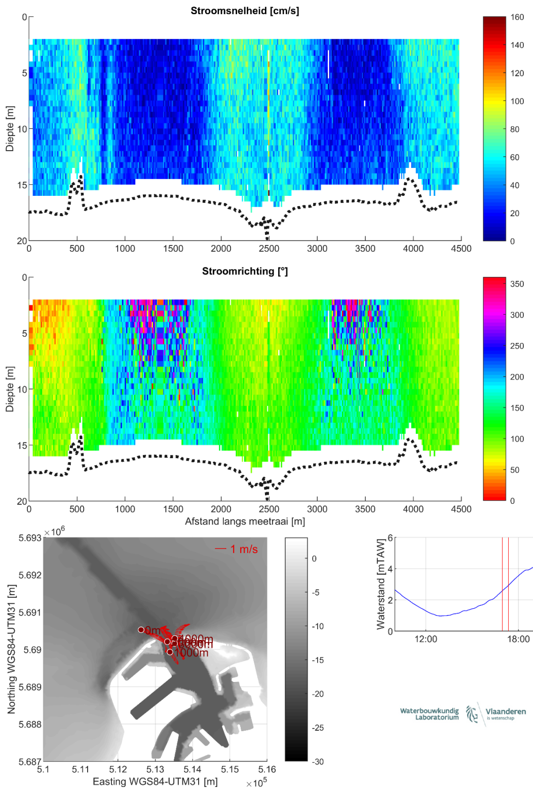
Figuur 29 – Stroomgegevens 24/08/2023 raai 24: snelheids grootte (top), -richting (midden) en diepte-gemiddelde vectoren (onder)
