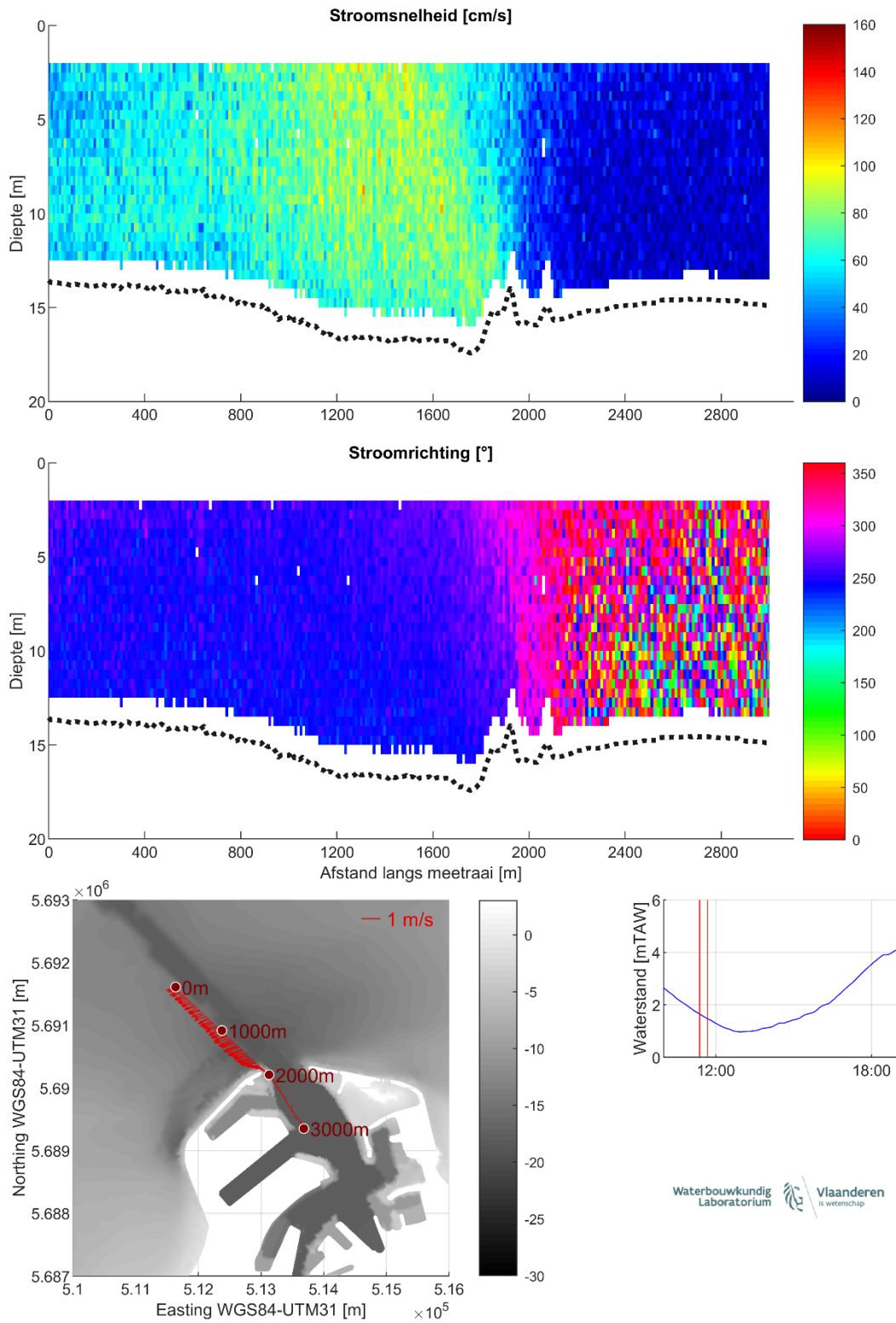
Figuur 9 – Stroomgegevens 24/08/2023 raai 4: snelheidsgrootte (top), -richting (midden) en diepte-gemiddelde vectoren (onder)
