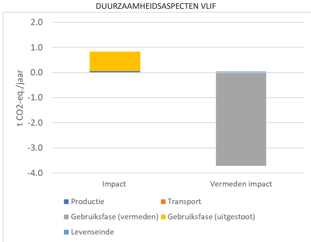
Figuur 2: Jaarlijkse impact broeikasgasemissie (t CO 2 -eq./jaar) warmtepomp
