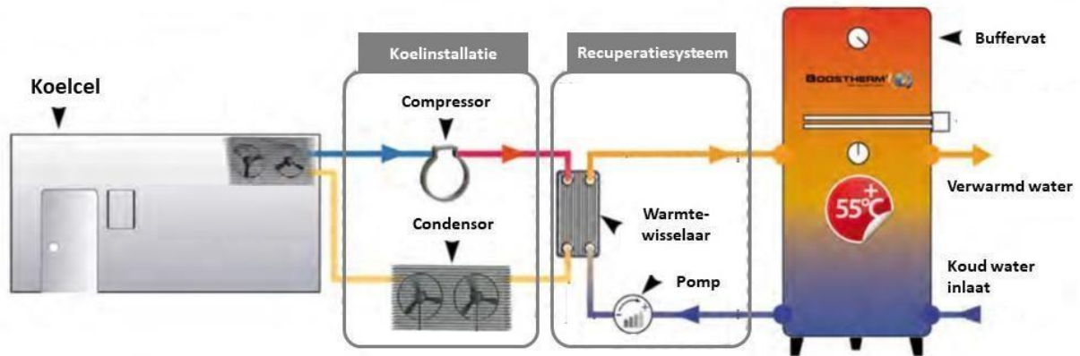
Figuur 9: Schematische voorstelling van een warmterecuperatiesysteem bij een koelinstallatie. 64
