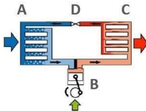
Figuur 8: Schematische voorstelling van een koelinstallatie 63
