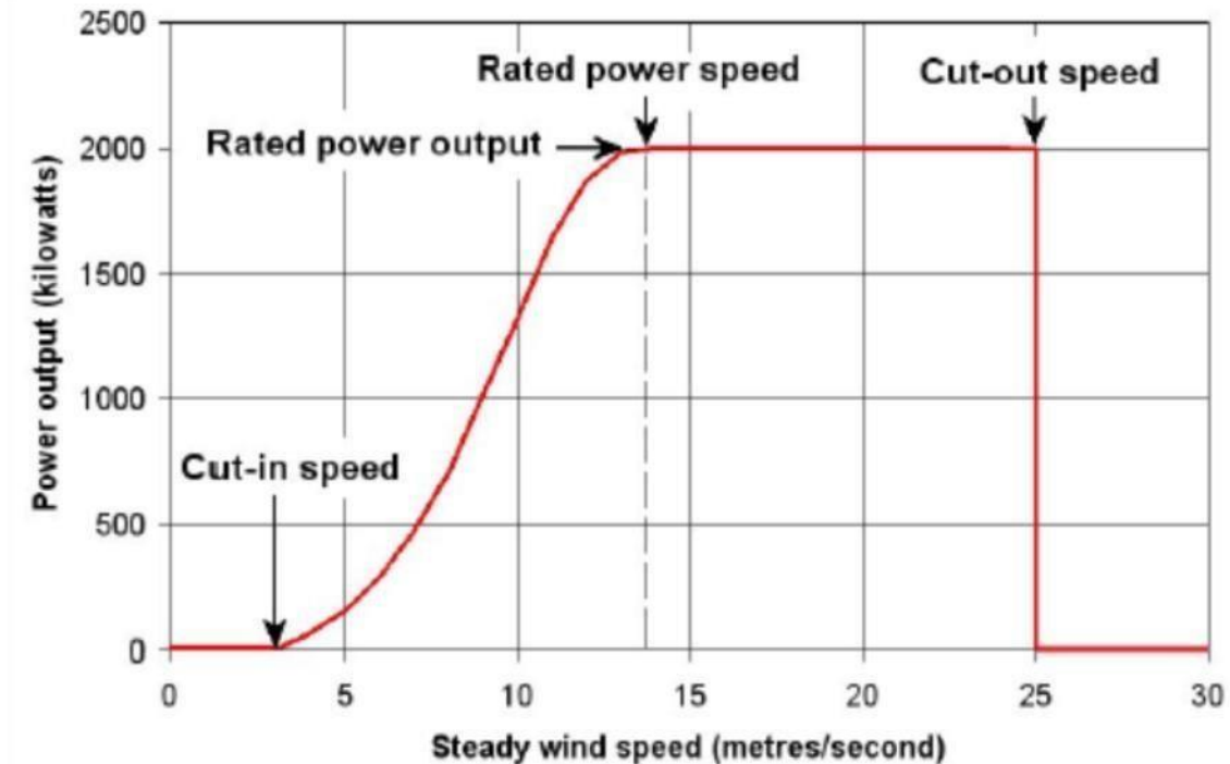
Figuur 3: Power curve van een windmolen
