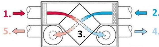
Figuur 5: Schematische voorstelling van een kruisstroomwarmtewisselaar.
