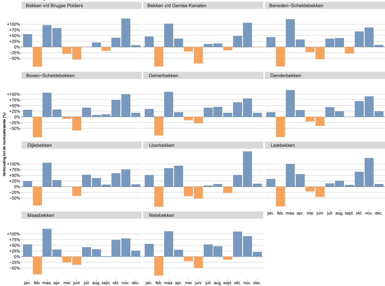
Gemiddelde maandelijkse neerslaghoeveelheden tussen januari en december 2023 voor de rivierbekkens van Vlaanderen Verhouding tot de maandelijkse normaalwaarde 1991-2020
