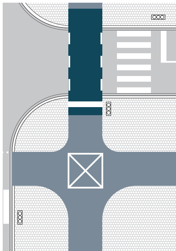
Fig. 3: Markering van het kruisingvlak.
