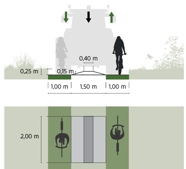
Fig. 1: Voorbehouden weg met tractorsluit
