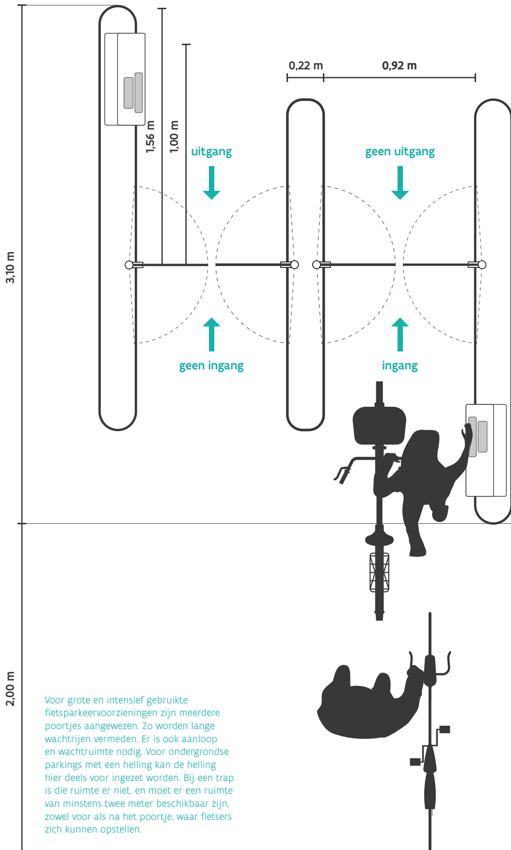
Fig. 1. Bovenaanzicht toegangscntrole
