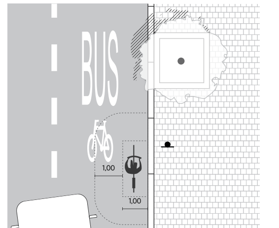
Fig. 4: busbaan met open profiel
