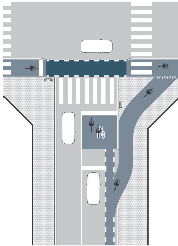
Fig. 1: Detailvoorbeeld bypass
