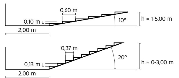
Fig. 4: Luie fietstrap met optimale maten (boven) en maximale maten (onder)
