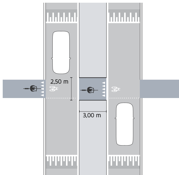
Fig. 5: Oversteek met middeneiland
