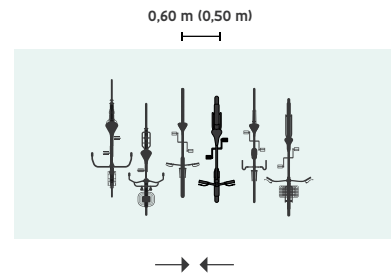
Fig. 8: Ruimte-inname hoog-laag-systeem
