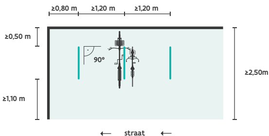
Fig. 11: Toepassing hoh-afstand van 1,20 m met fietsen en kinderfietsen eraan
