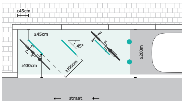
Fig. 12: Toepassing fietsfietsbeugel met lagere tussenbuis
