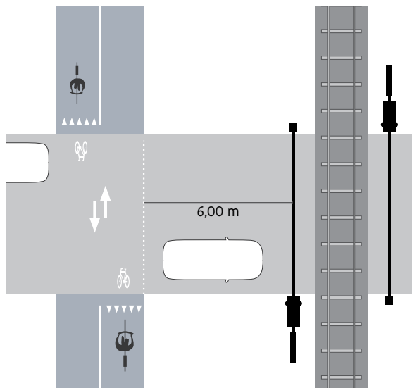
Fig. 6: Oversteek naast een langsliggend spoor
