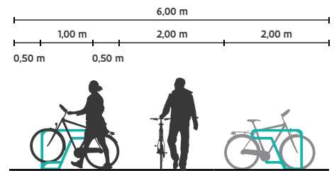
Fig. 9: Hoog-laag voorziening
