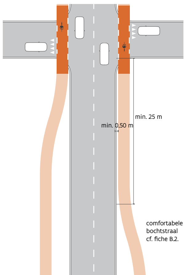
Fig. 3: Inbuigend eenrichtingsfietspad
