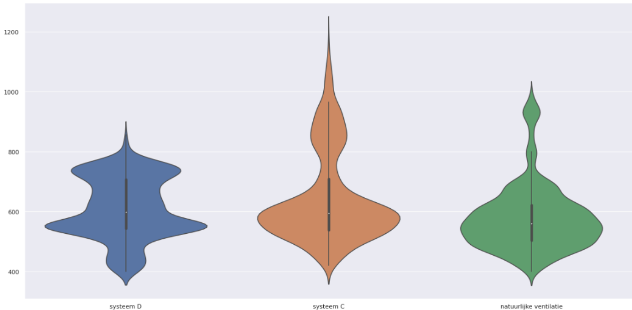
Figuur 11: Violinplot van de datapunten voor de bewonerskamers, opgesplitst per ventilatiesysteem, tijdens de ochtenduren (Y-as is de CO 2 -waarde in ppm; data ruimtes met D, C en natuurlijke ventilatie/A). De medianen zijn de witte punten op de figuren.
