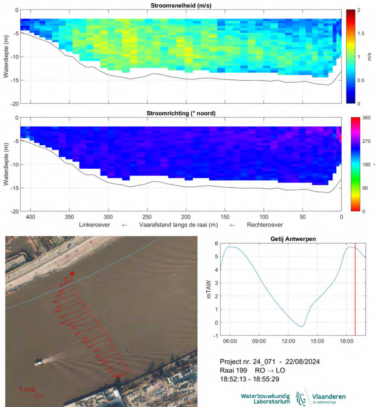
Figuur 208: Strooming opwaarts Kennedytunnel 22/08/2024 - Raai 199 - 18:52:13-18:55:29
