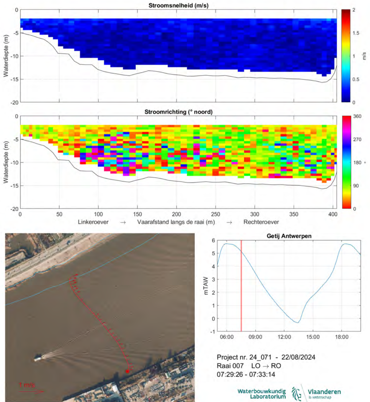
Figuur 18: Strooming opwaarts Kennedytunnel 22/08/2024 - Raai 007 - 07:29:26-07:33:14
