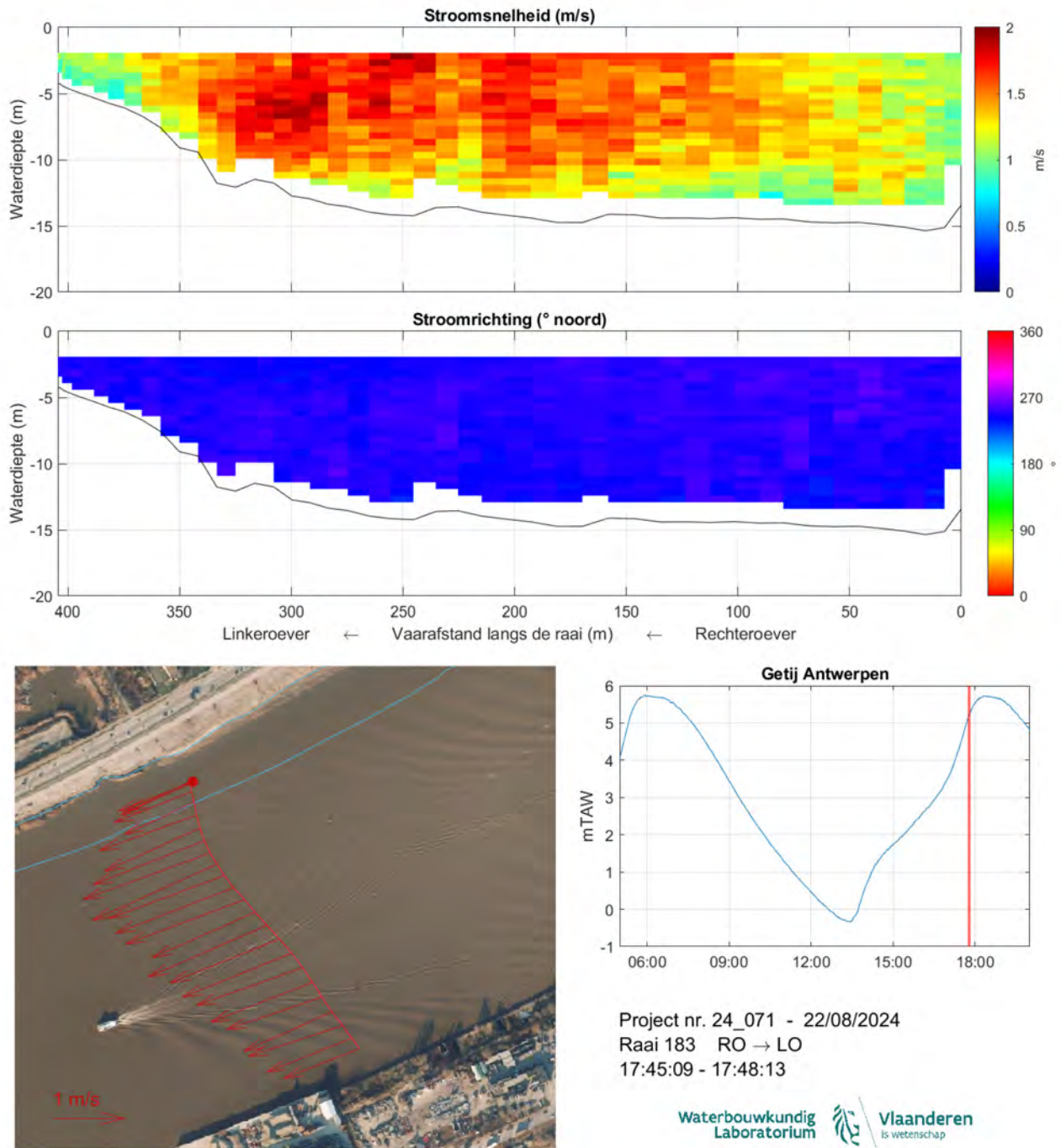
Figuur 192: Strooming opwaarts Kennedytunnel 22/08/2024 - Raai 183 - 17:45:09-17:48:13
