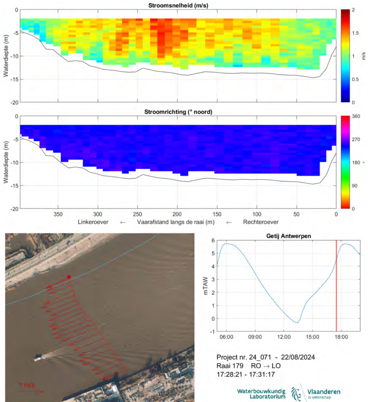
Figuur 188: Strooming opwaarts Kennedytunnel 22/08/2024 - Raai 179 - 17:28:21-17:31:17
