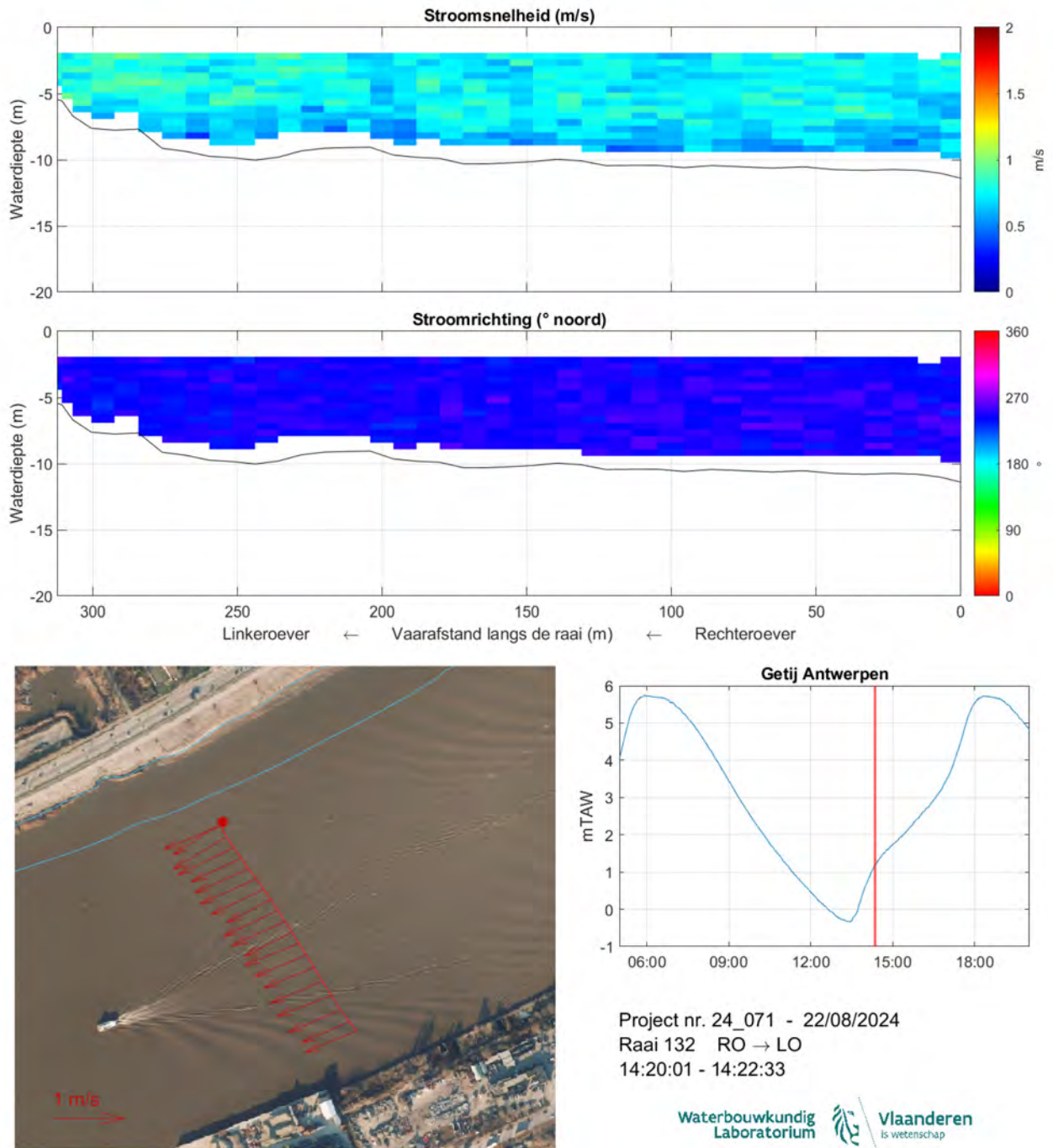
Figuur 142: Strooming opwaarts Kennedytunnel 22/08/2024 - Raai 132 - 14:20:01-14:22:33
