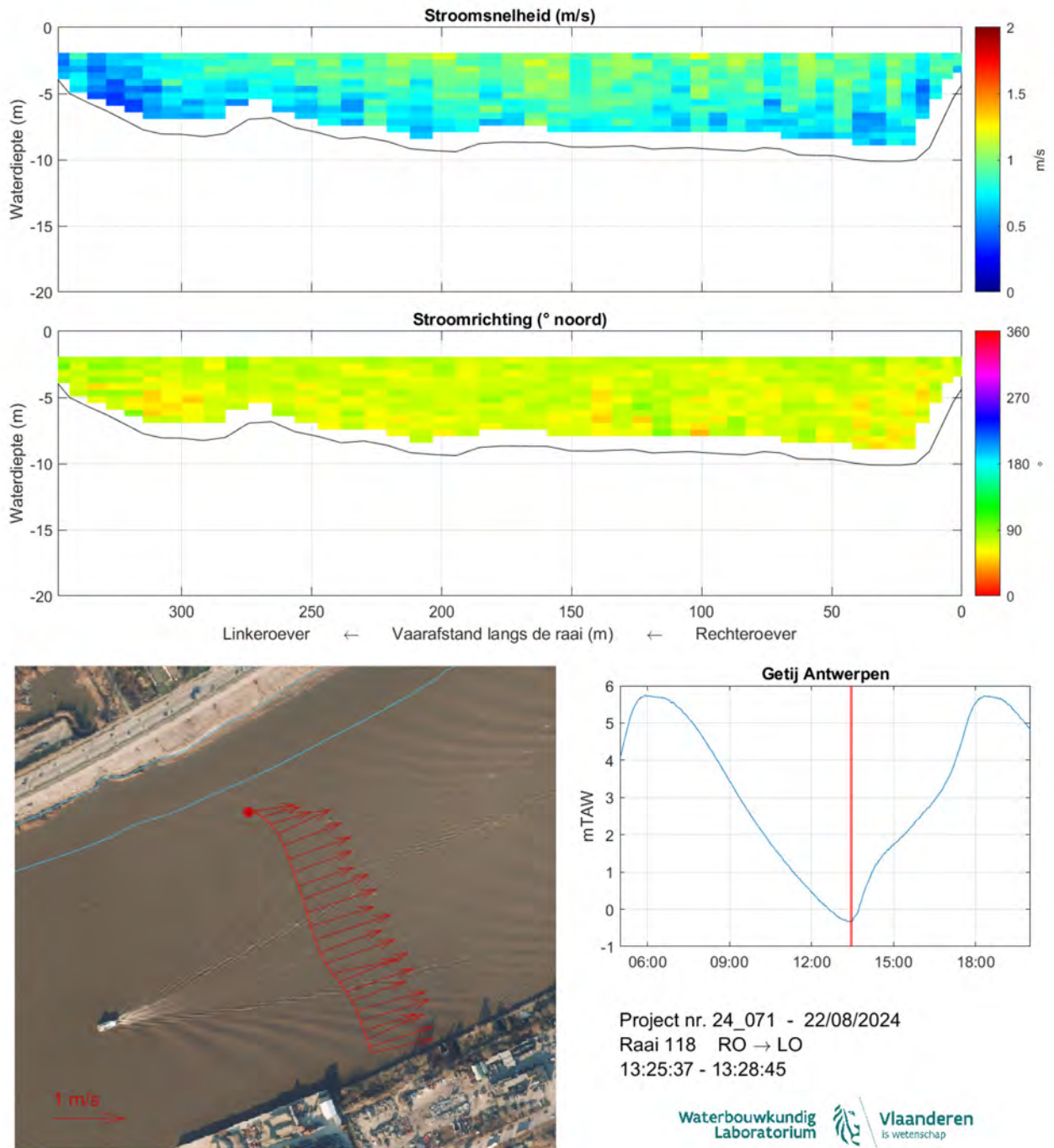
Figuur 128: Strooming opwaarts Kennedytunnel 22/08/2024 - Raai 118 - 13:25:37-13:28:45
