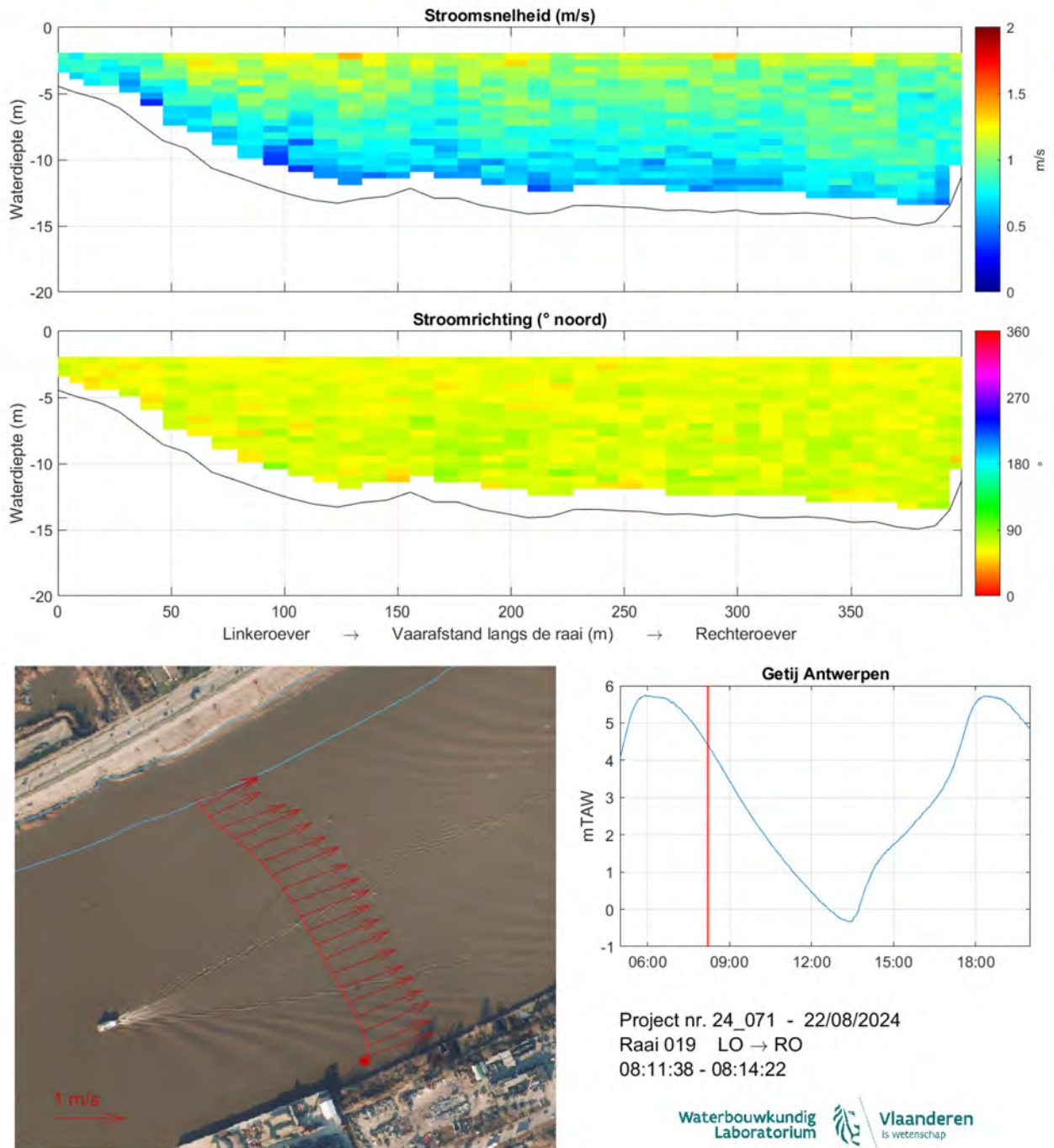
Figuur 30: Strooming opwaarts Kennedytunnel 22/08/2024 - Raai 019 - 08:11:38-08:14:22
