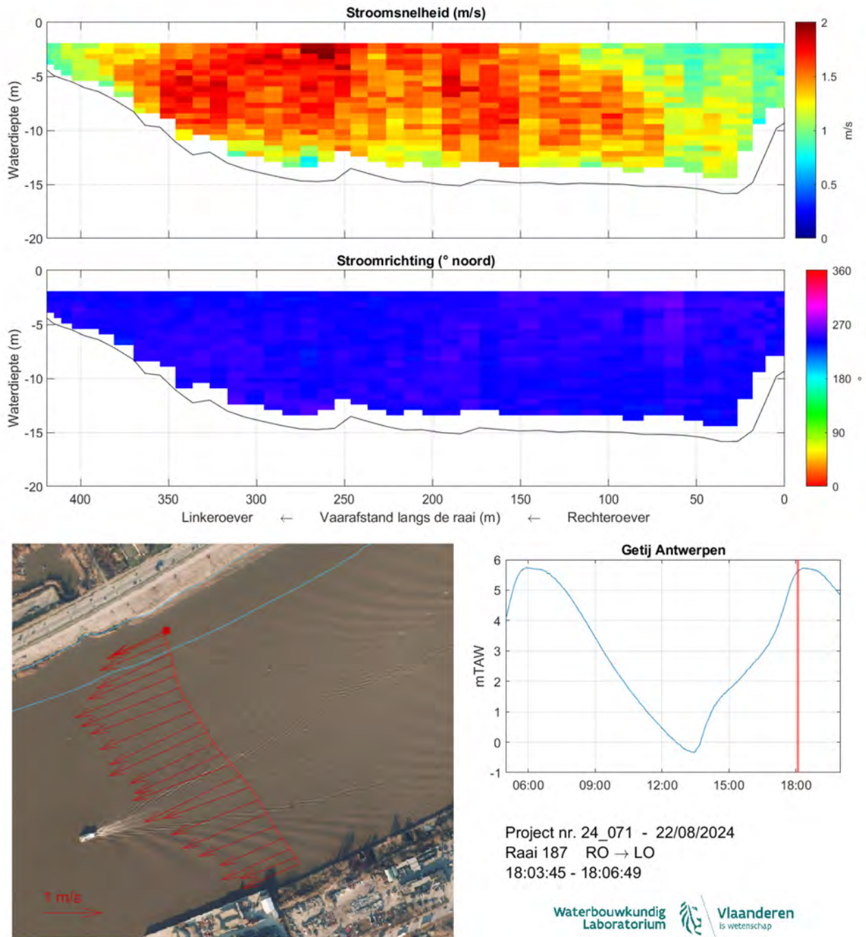
Figuur 196: Strooming opwaarts Kennedytunnel 22/08/2024 - Raai 187 - 18:03:45-18:06:49
