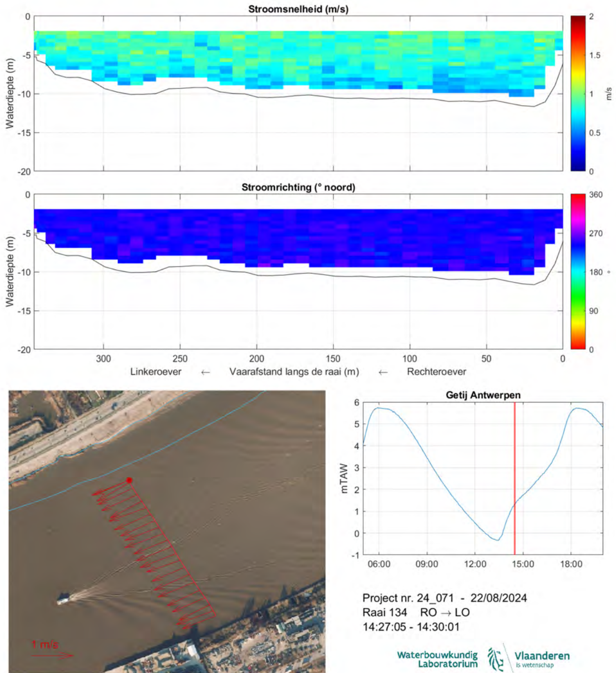
Figuur 144: Strooming opwaarts Kennedytunnel 22/08/2024 - Raai 134 - 14:27:05-14:30:01
