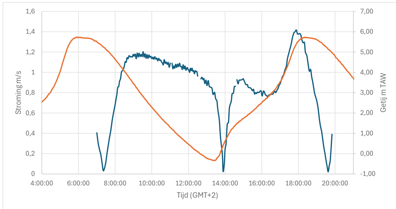
Figuur 10: Getij Antwerpen en sectiegemiddelde stroming
