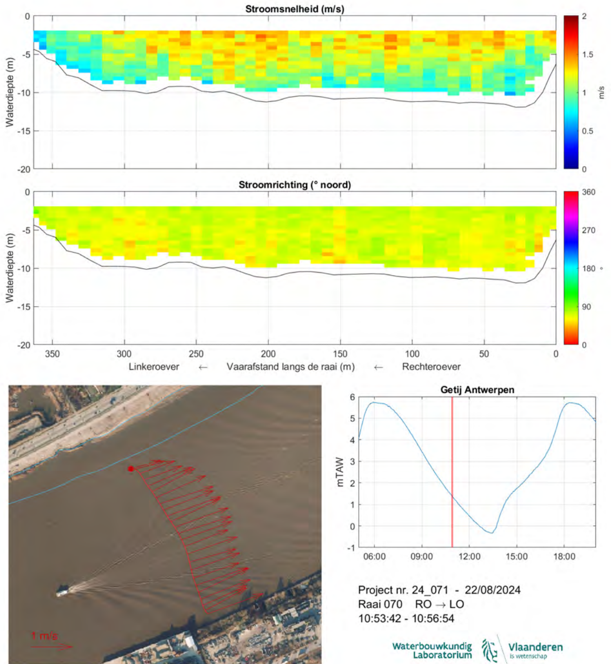
Figuur 81: Strooming opwaarts Kennedytunnel 22/08/2024 - Raai 070 - 10:53:42-10:56:54
