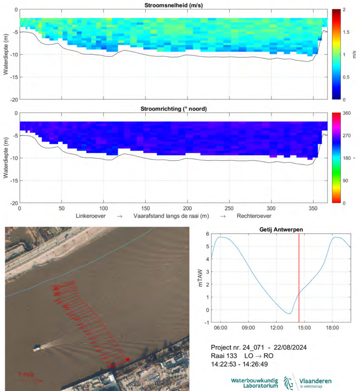
Figuur 143: Strooming opwaarts Kennedytunnel 22/08/2024 - Raai 133 - 14:22:53-14:26:49
