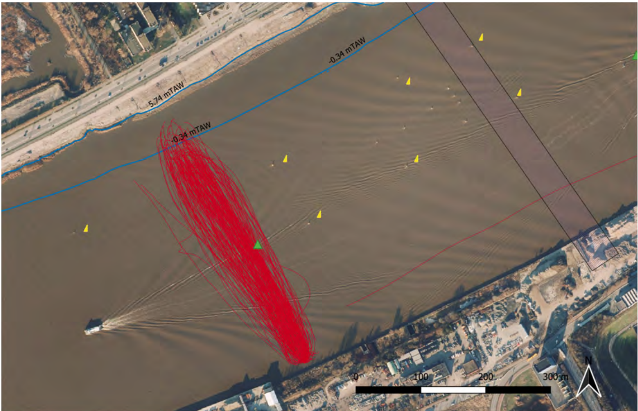
Figuur 7: GPS tracks van alle gevaren raai
