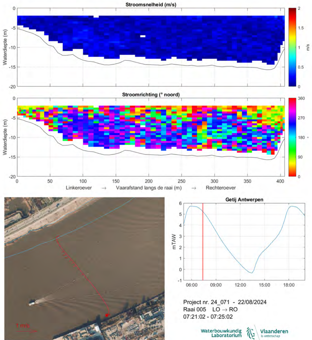
Figuur 16: Stroming opwaarts Kennedytunnel 22/08/2024 - Raai 005 - 07:21:02-07:25:02
