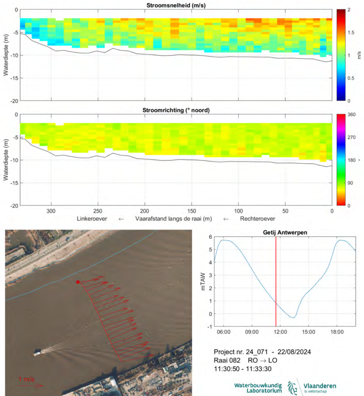
Figuur 93: Strooming opwaarts Kennedytunnel 22/08/2024 - Raai 082 - 11:30:50-11:33:30
