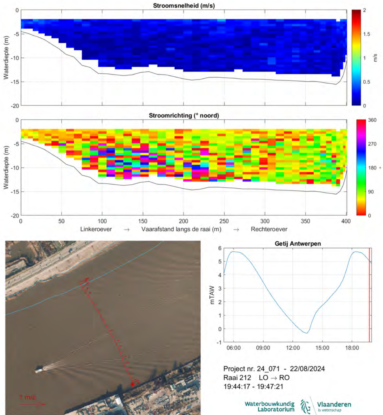
Figuur 221: Strooming opwaarts Kennedytunnel 22/08/2024 - Raai 212 - 19:44:17-19:47:21
