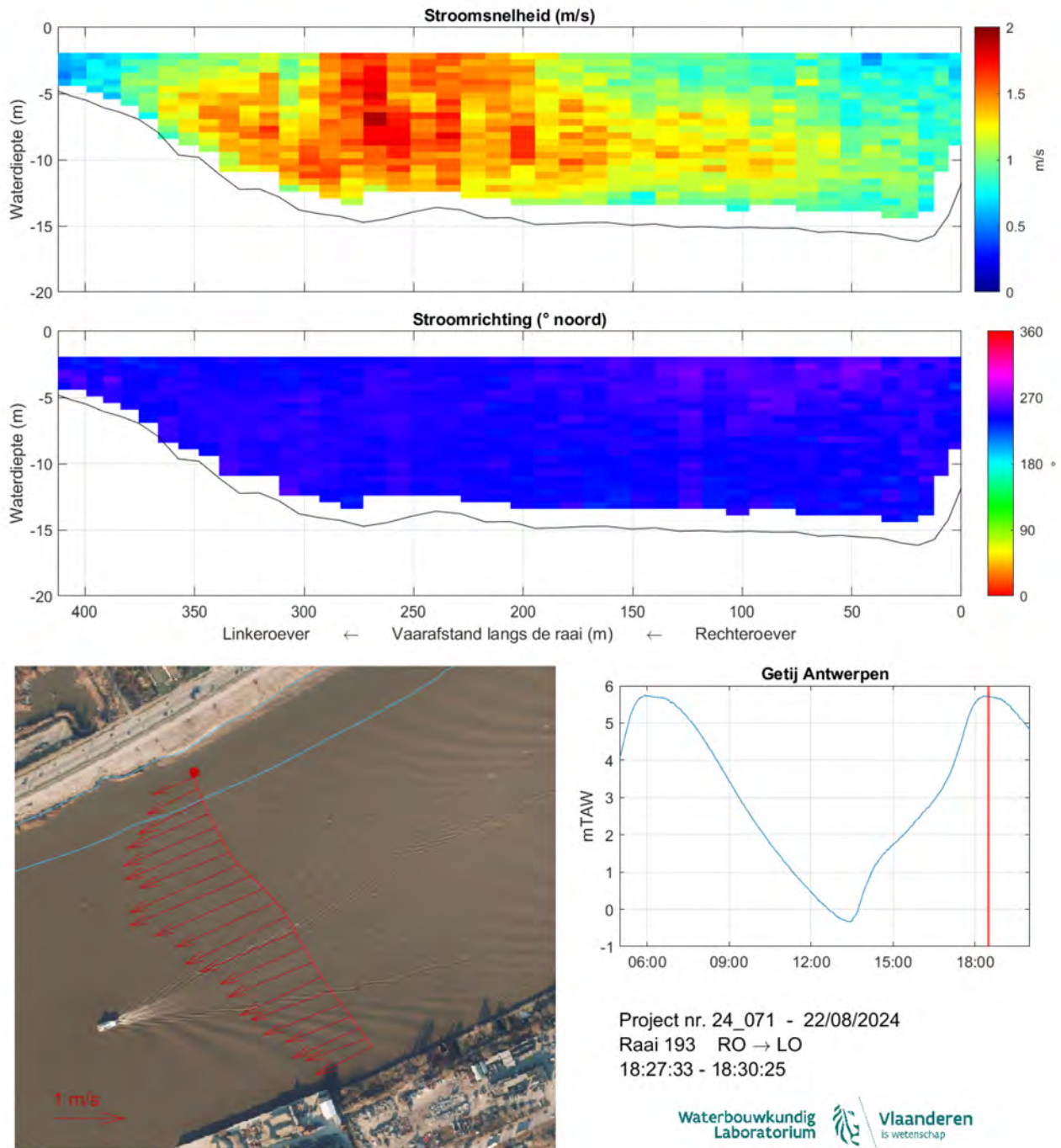
Figuur 202: Strooming opwaarts Kennedytunnel 22/08/2024 - Raai 193 - 18:27:33-18:30:25
