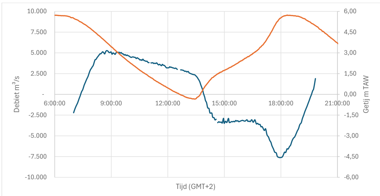
Figuur 9: Getij Antwerpen en berekend debiet
