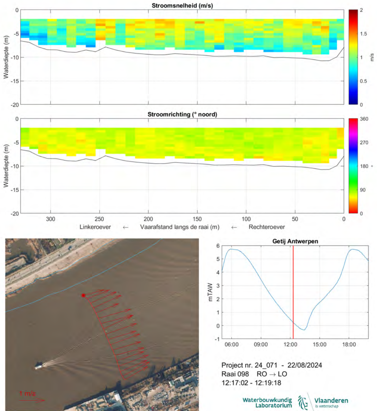
Figuur 109: Strooming opwaarts Kennedytunnel 22/08/2024 - Raai 098 - 12:17:02-12:19:18
