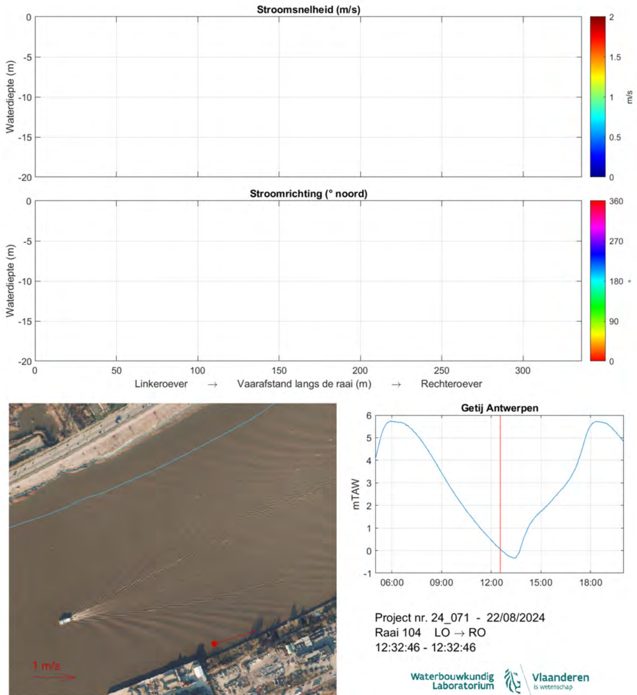
Figuur 222: Strooming opwaarts Kennedytunnel 22/08/2024 - Raai 104 - 12:32:46-12:32:46
