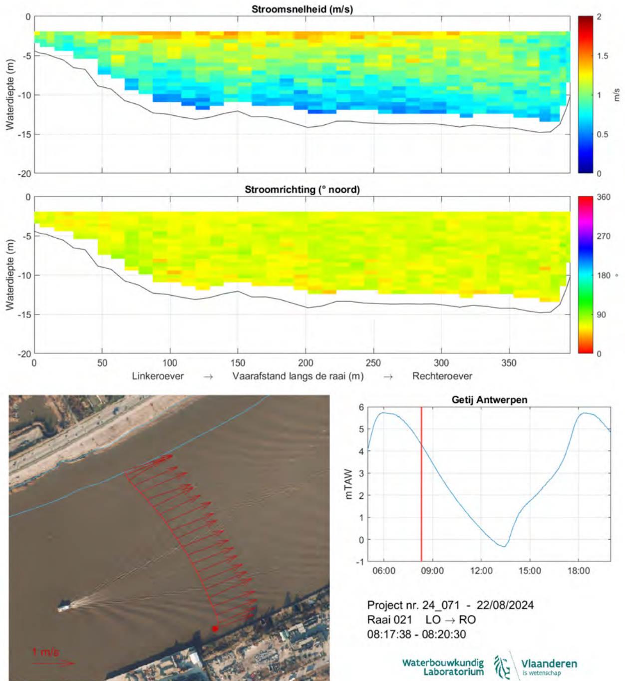
Figuur 32: Strooming opwaarts Kennedytunnel 22/08/2024 - Raai 021 - 08:17:38-08:20:30
