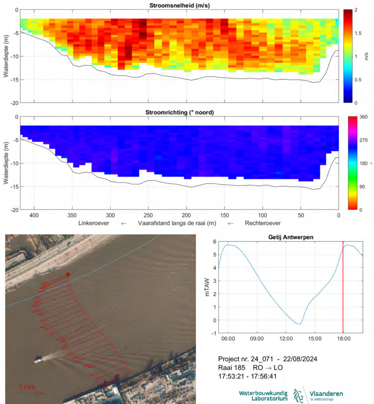
Figuur 194: Strooming opwaarts Kennedytunnel 22/08/2024 - Raai 185 - 17:53:21-17:56:41
