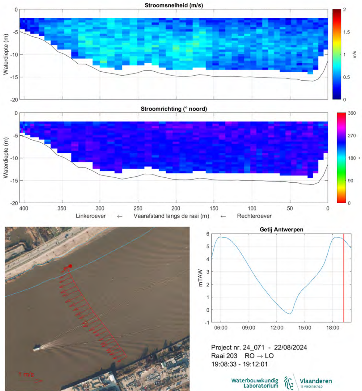
Figuur 212: Strooming opwaarts Kennedytunnel 22/08/2024 - Raai 203 - 19:08:33-19:12:01
