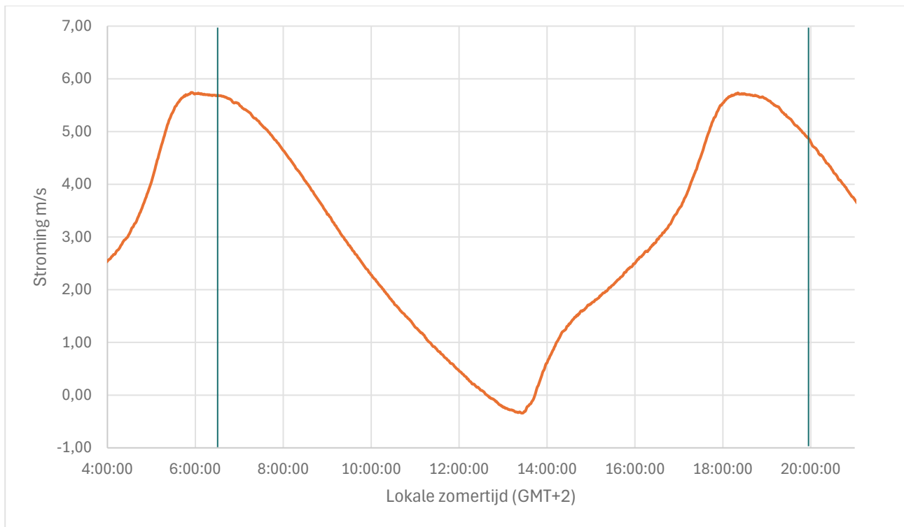
Figuur 5: Getij Antwerpen 22/8/2024 met begin en eindmarkering meetcampagne
