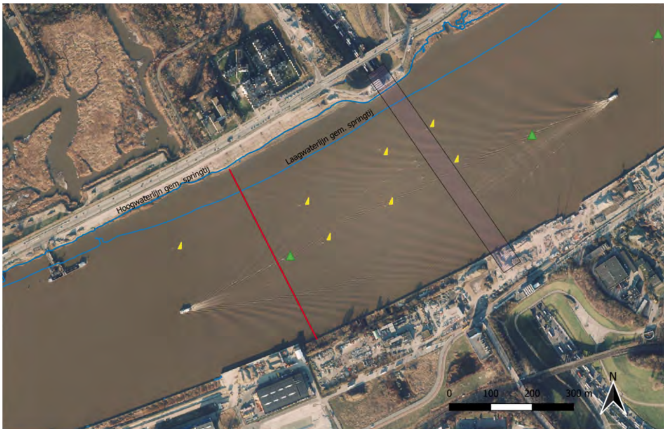
Figuur 2: Locatie van de meetraai (rode lijn). De gele bebakening geeft de locatie van de heiproef weer.
