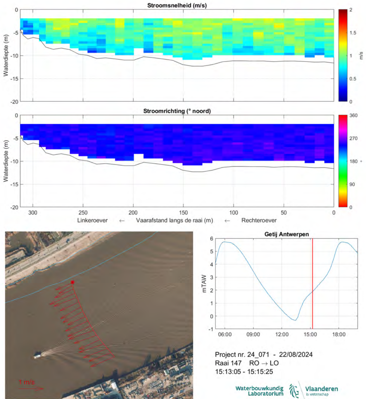
Figuur 156: Strooming opwaarts Kennedytunnel 22/08/2024 - Raai 147 - 15:13:05-15:15:25
