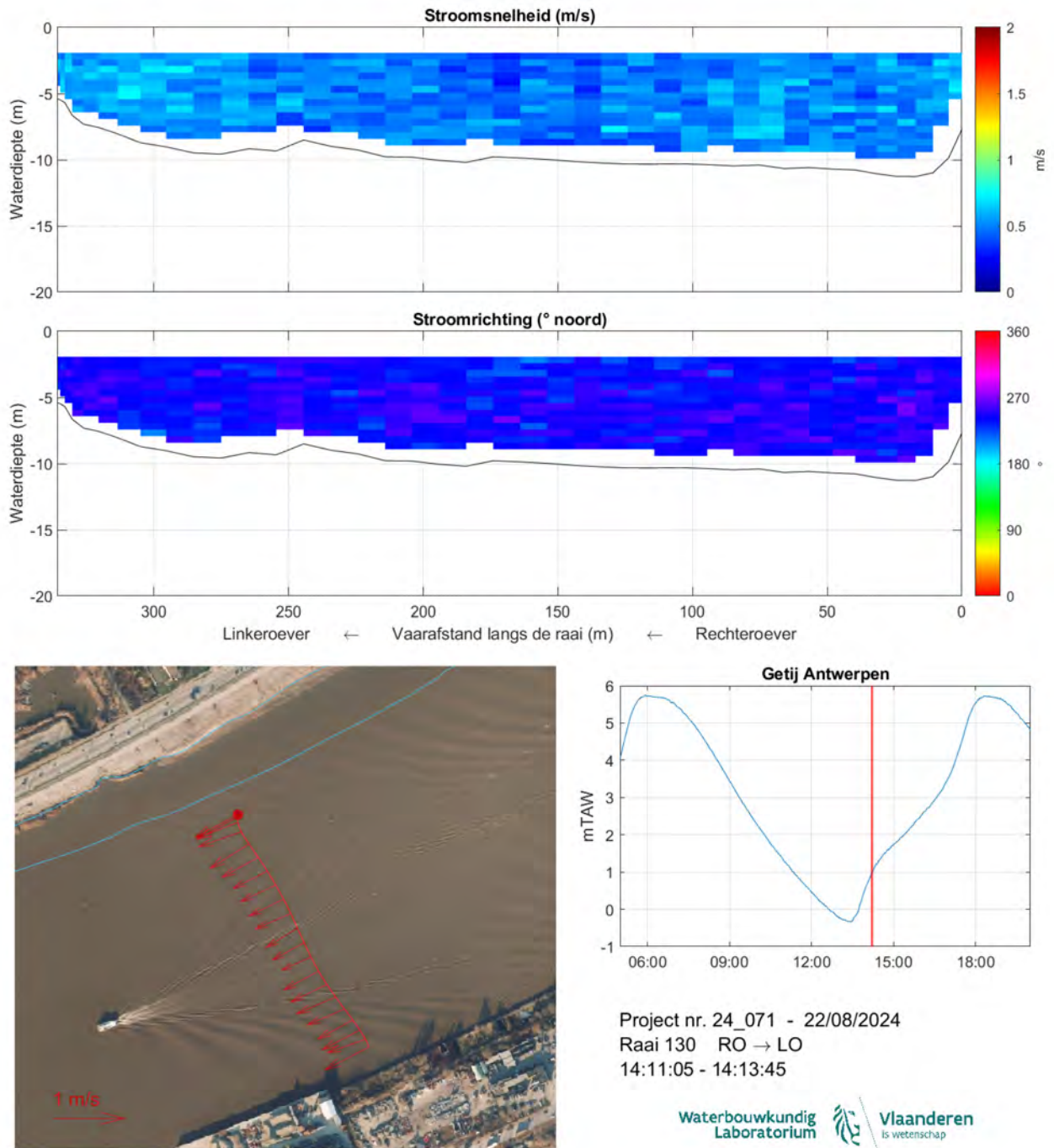
Figuur 140: Strooming opwaarts Kennedytunnel 22/08/2024 - Raai 130 - 14:11:05-14:13:45
