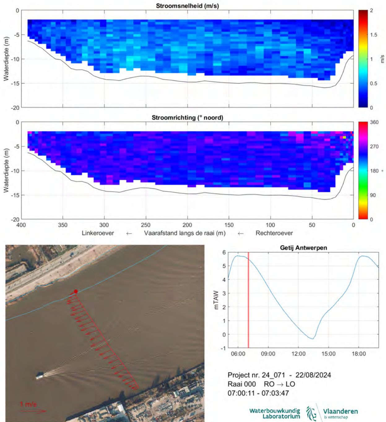
Figuur 11: Stroming opwaarts Kennedytunnel 22/08/2024 - Raai 000 - 07:00:11-07:03:47
