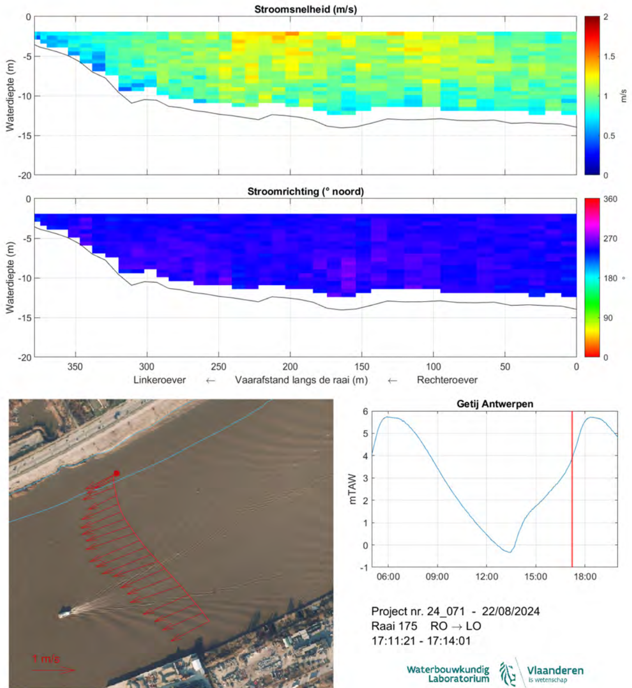
Figuur 184: Strooming opwaarts Kennedytunnel 22/08/2024 - Raai 175 - 17:11:21-17:14:01
