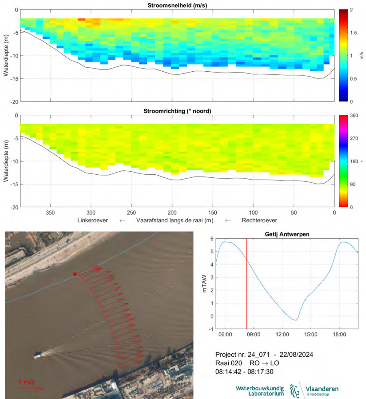
Figuur 31: Strooming opwaarts Kennedytunnel 22/08/2024 - Raai 020 - 08:14:42-08:17:30
