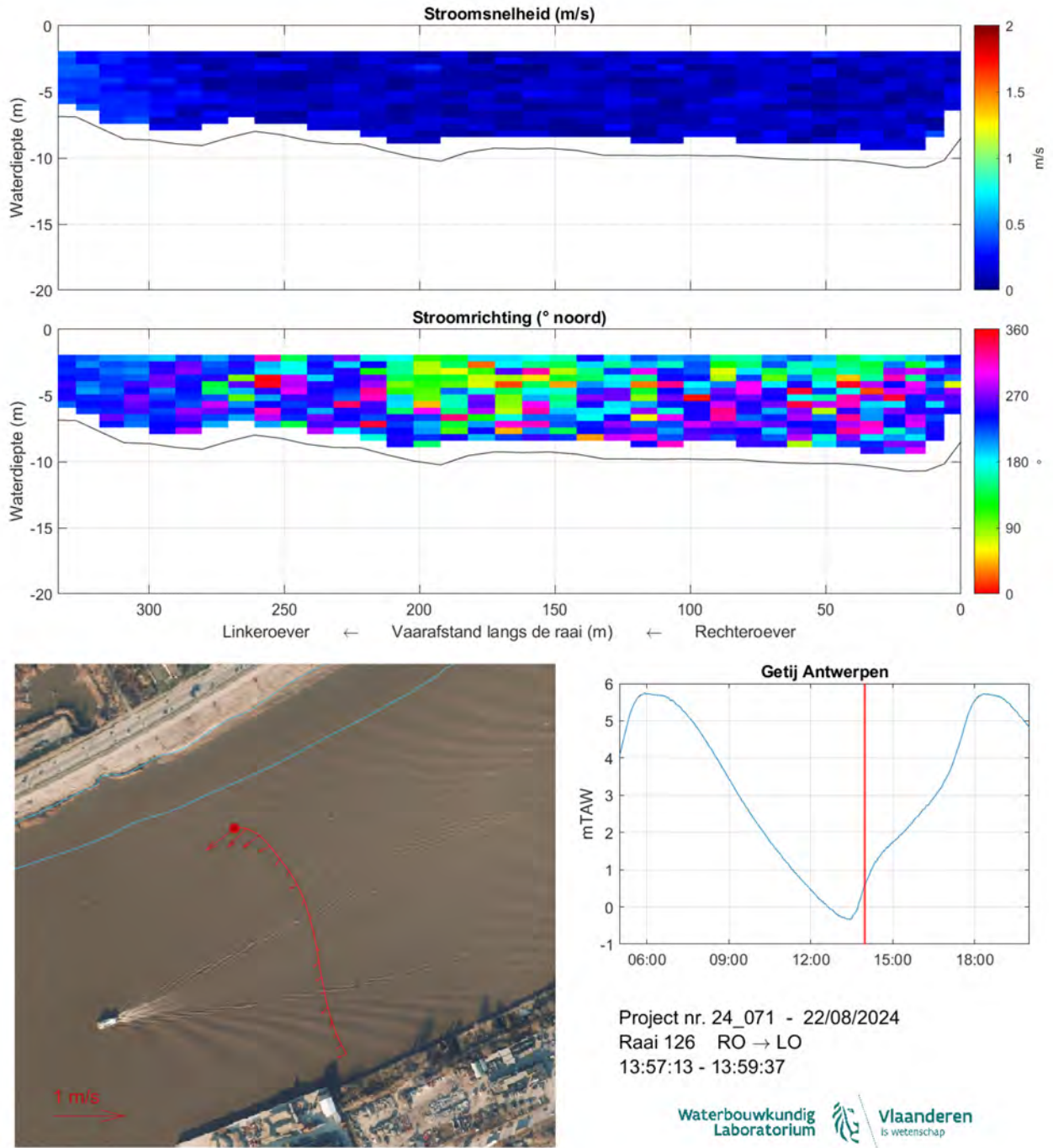
Figuur 136: Strooming opwaarts Kennedytunnel 22/08/2024 - Raai 126 - 13:57:13-13:59:37
