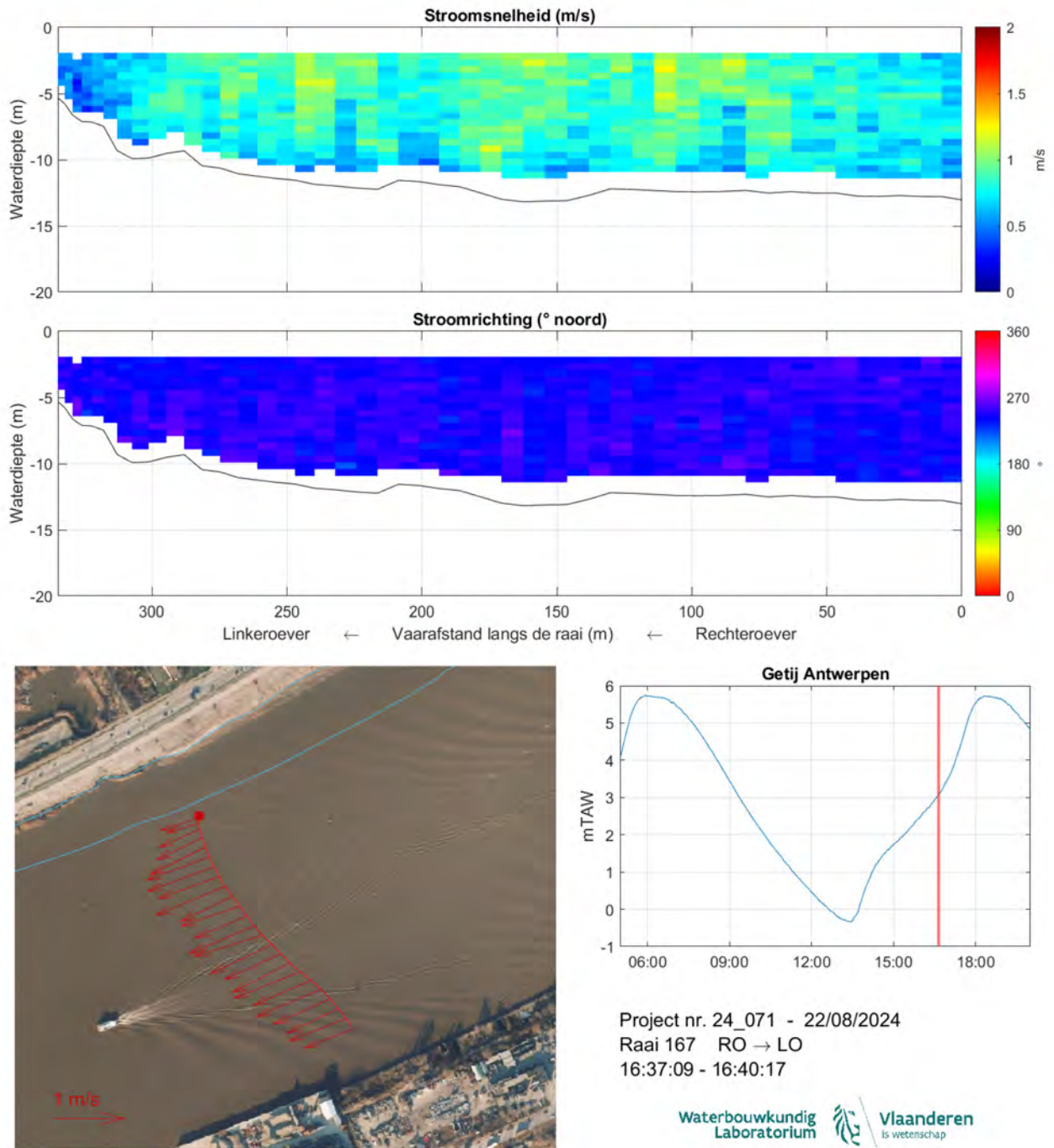
Figuur 176: Strooming opwaarts Kennedytunnel 22/08/2024 - Raai 167 - 16:37:09-16:40:17
