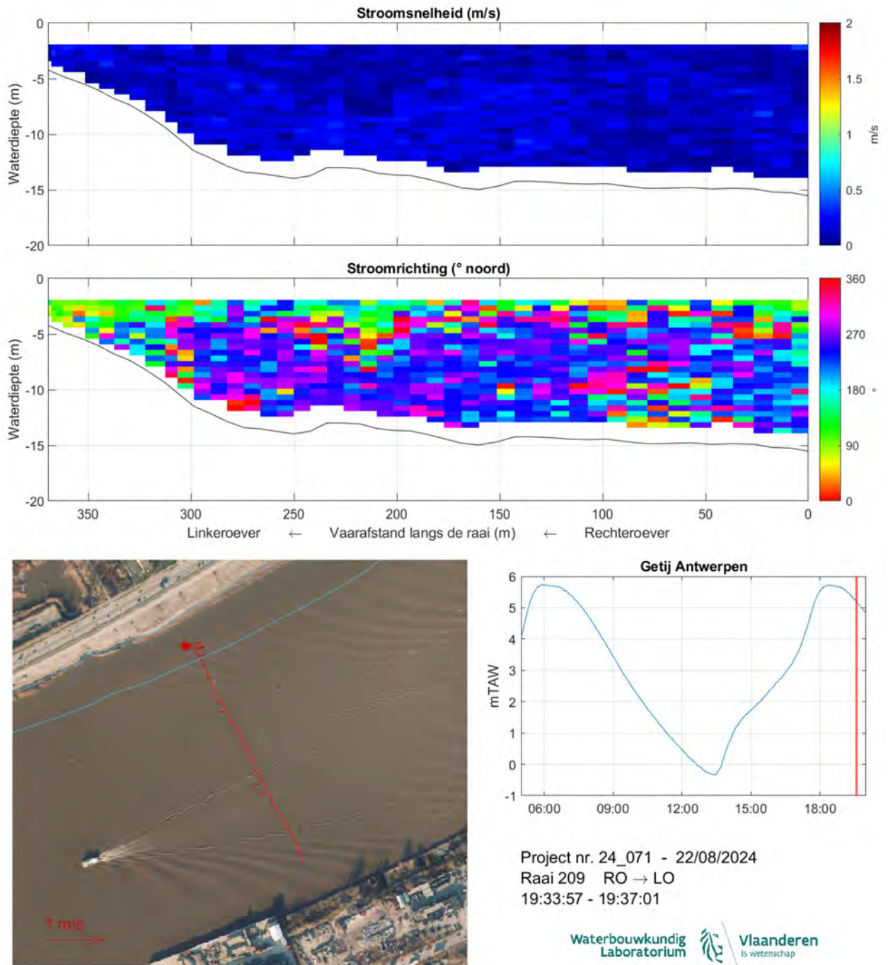
Figuur 218: Strooming opwaarts Kennedytunnel 22/08/2024 - Raai 209 - 19:33:57-19:37:01
