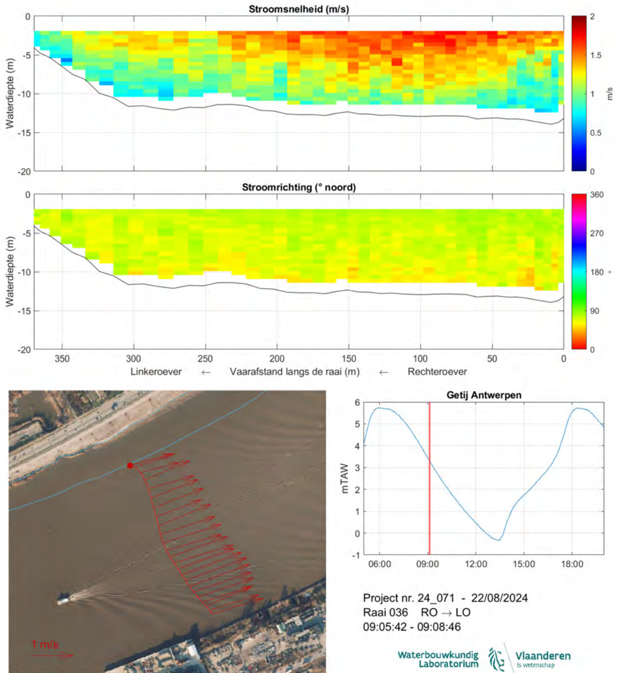
Figuur 47: Strooming opwaarts Kennedytunnel 22/08/2024 - Raai 036 - 09:05:42-09:08:46
