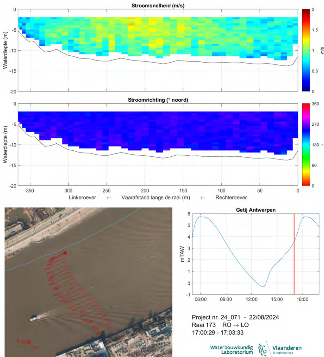
Figuur 182: Strooming opwaarts Kennedytunnel 22/08/2024 - Raai 173 - 17:00:29-17:03:33
