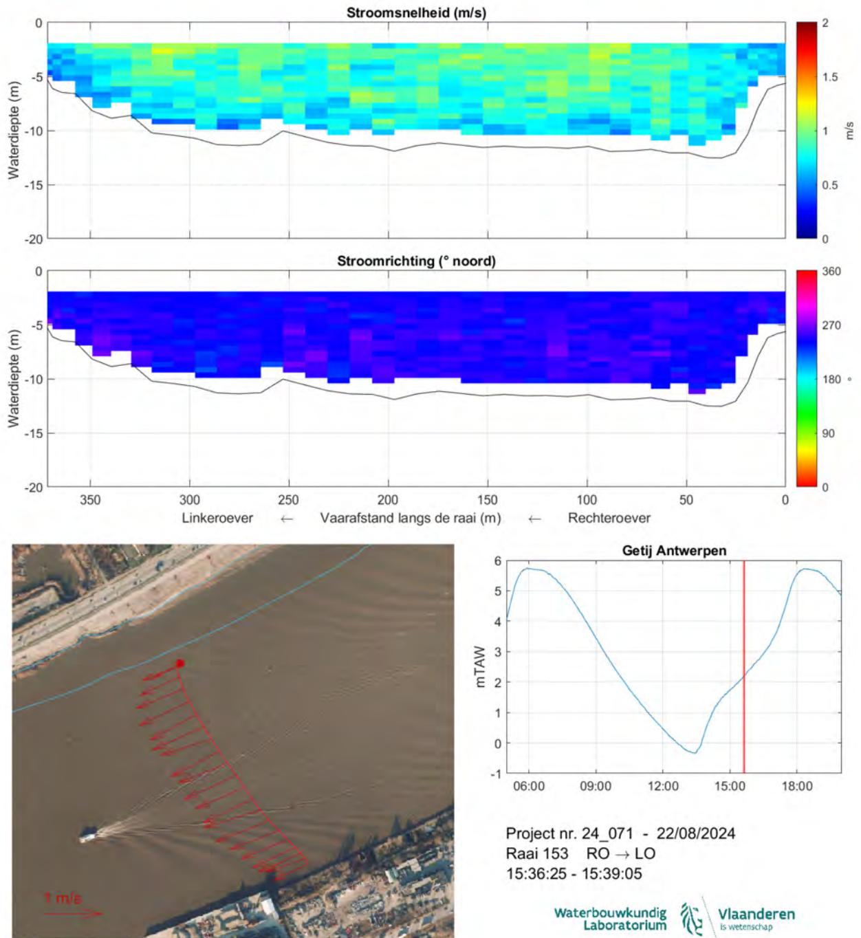
Figuur 162: Strooming opwaarts Kennedytunnel 22/08/2024 - Raai 153 - 15:36:25-15:39:05
