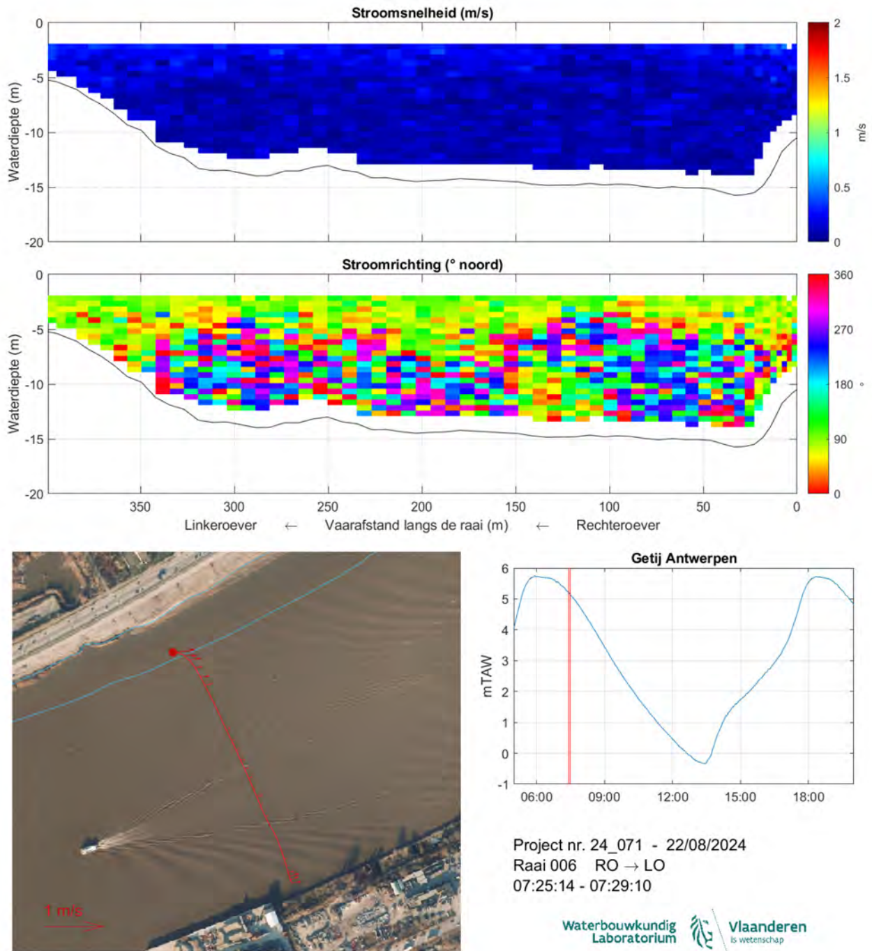
Figuur 17: Stroming opwaarts Kennedytunnel 22/08/2024 - Raai 006 - 07:25:14-07:29:10
