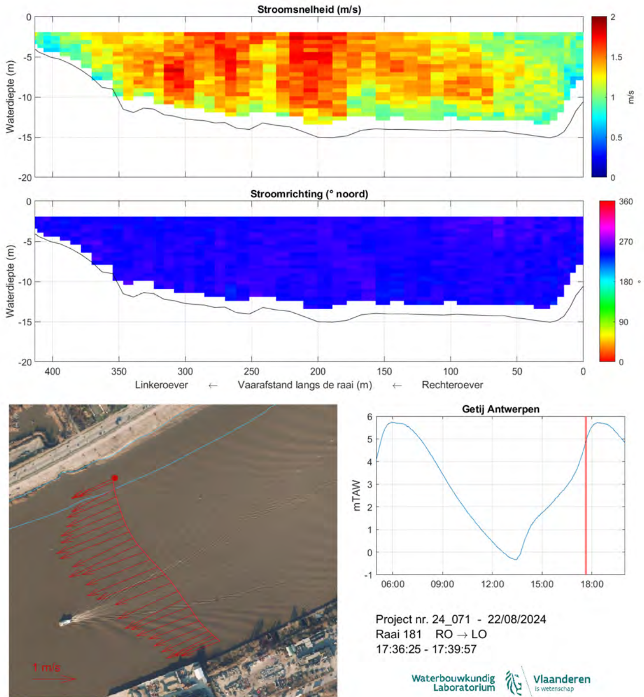
Figuur 190: Strooming opwaarts Kennedytunnel 22/08/2024 - Raai 181 - 17:36:25-17:39:57
