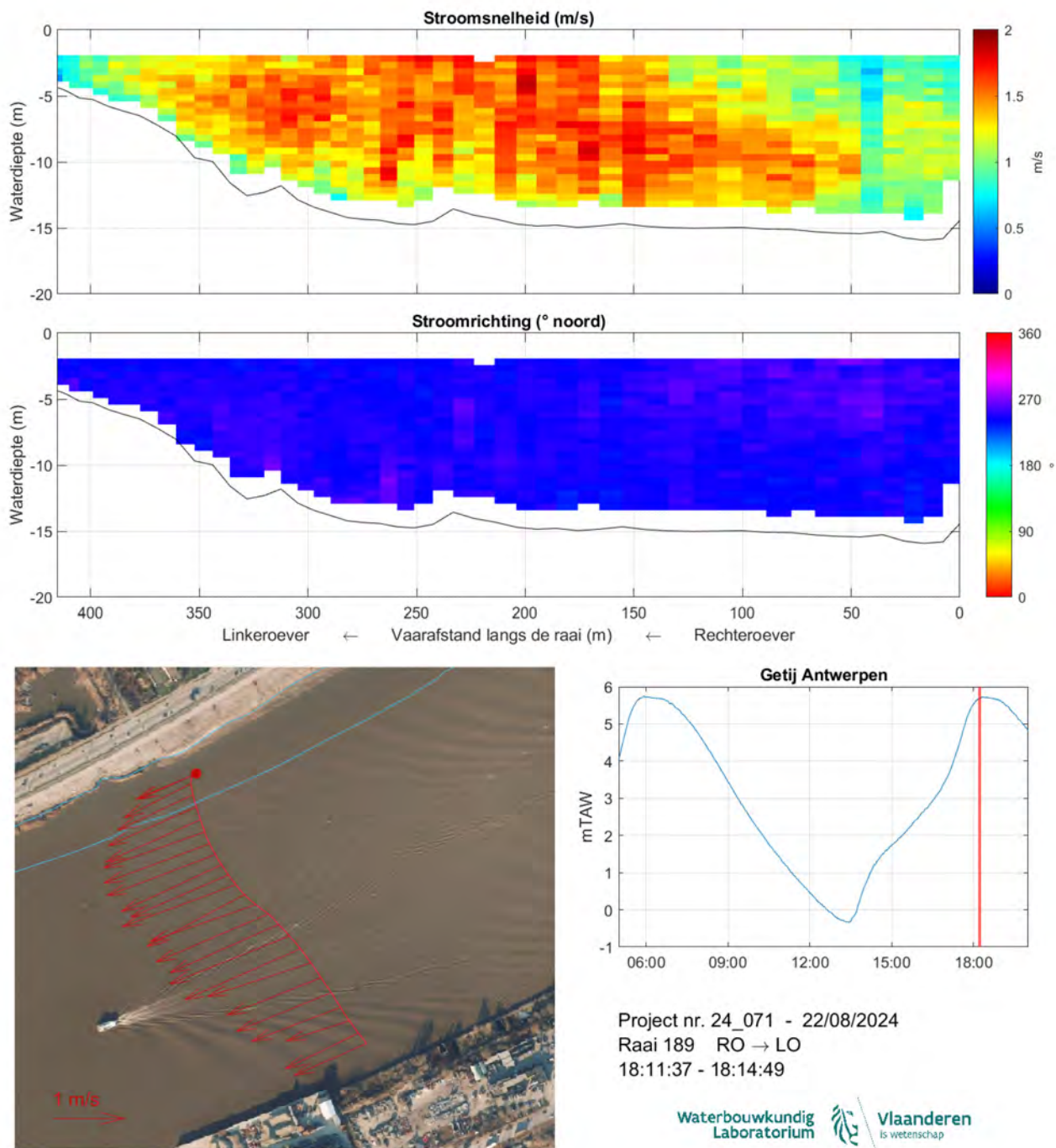
Figuur 198: Strooming opwaarts Kennedytunnel 22/08/2024 - Raai 189 - 18:11:37-18:14:49
