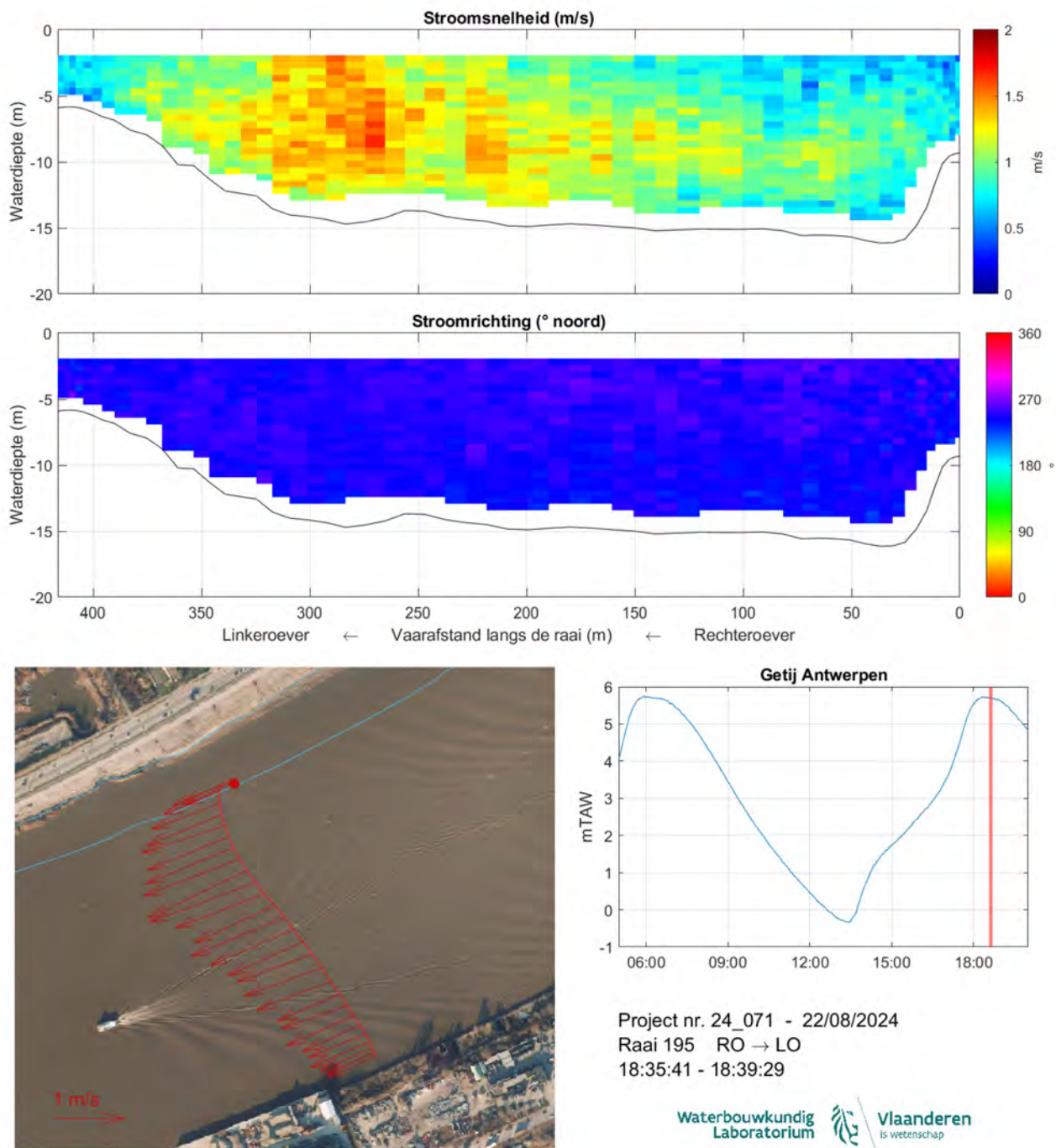
Figuur 204: Strooming opwaarts Kennedytunnel 22/08/2024 - Raai 195 - 18:35:41-18:39:29
