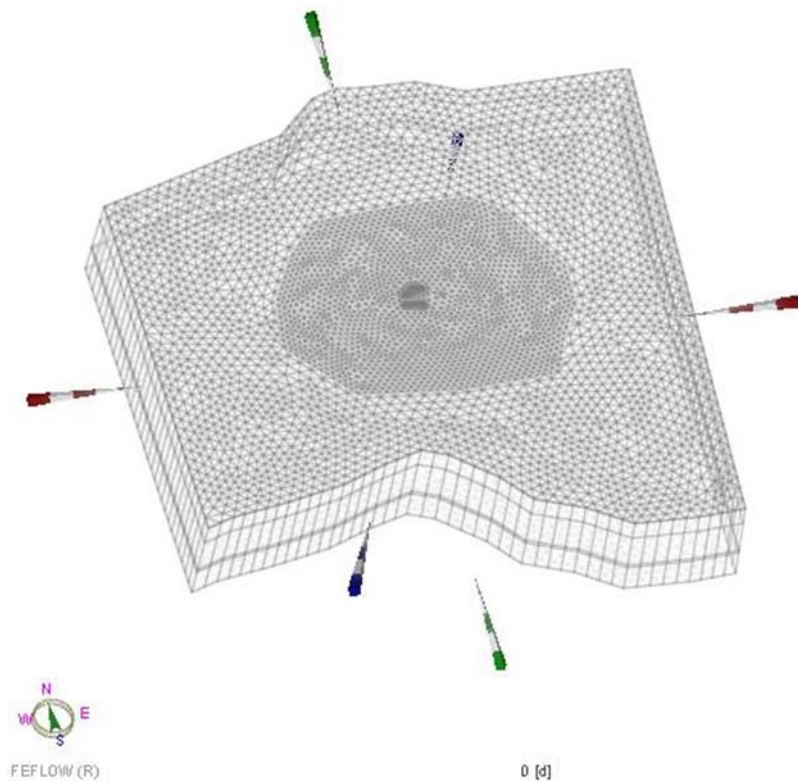
Figuur 3-13: 3D-rastering van de software FeFlow.
