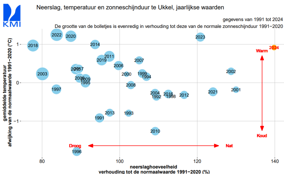
Figuur 3 Neerslag, temperatuur en zonneshijnduur gemeten te Ukkel voor de jaren 1991-2024 (bron: KMI)
